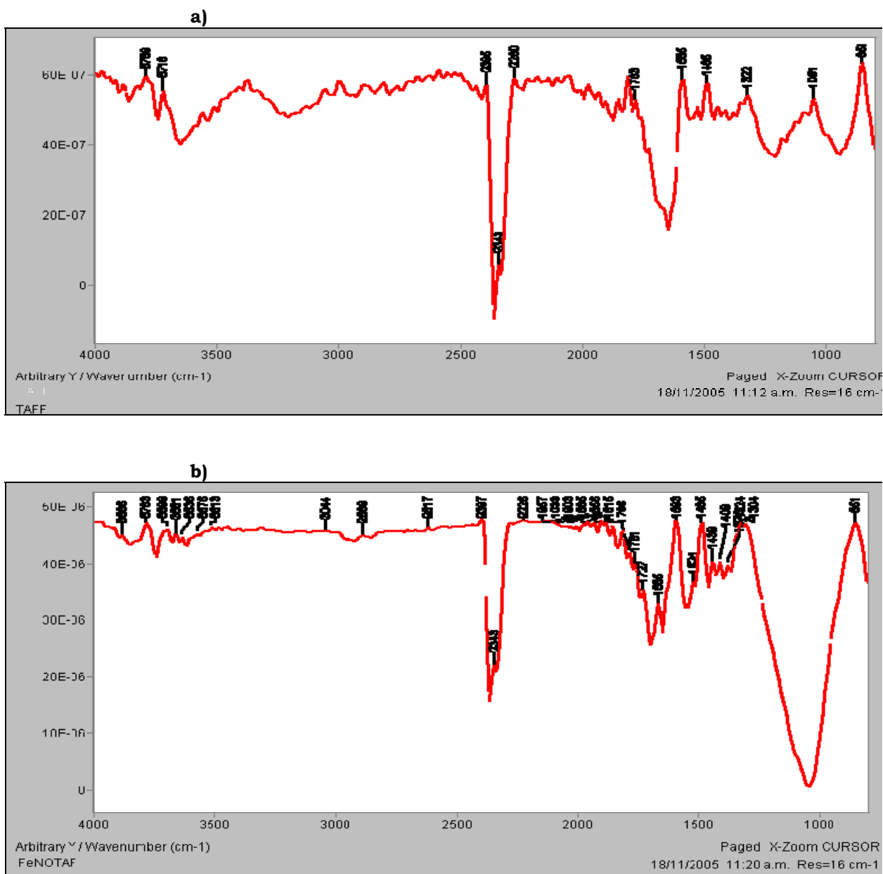
Figura 17. Espectros de absorción infrarroja a) TAFF, b) Fe(NO 3 ) 3 /TAFF
