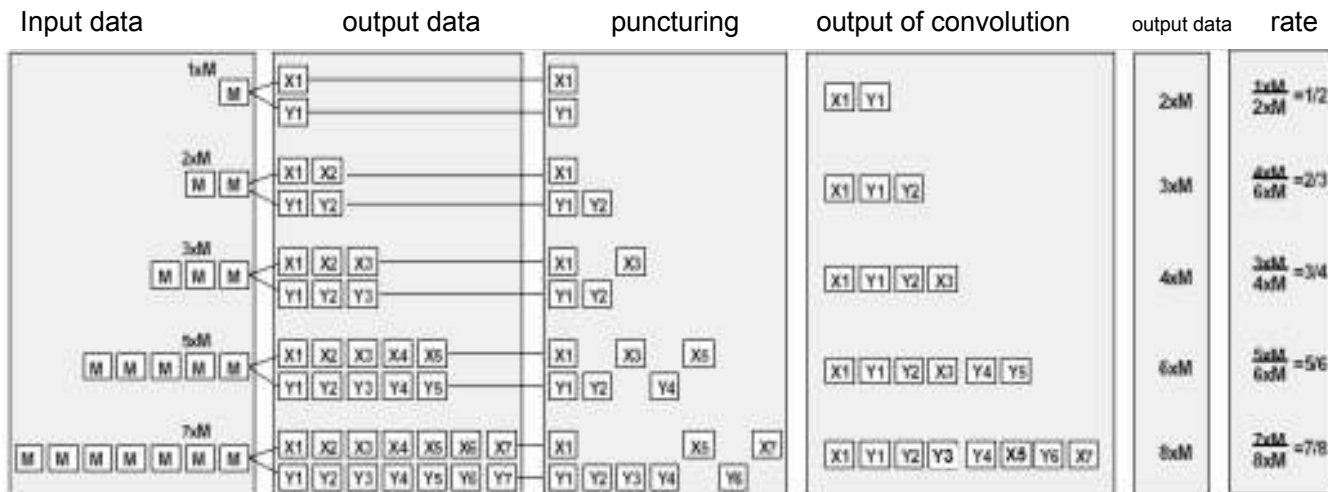
Figura 3-8 Esquema de punteo y secuencia transmitida en la salida serie.
