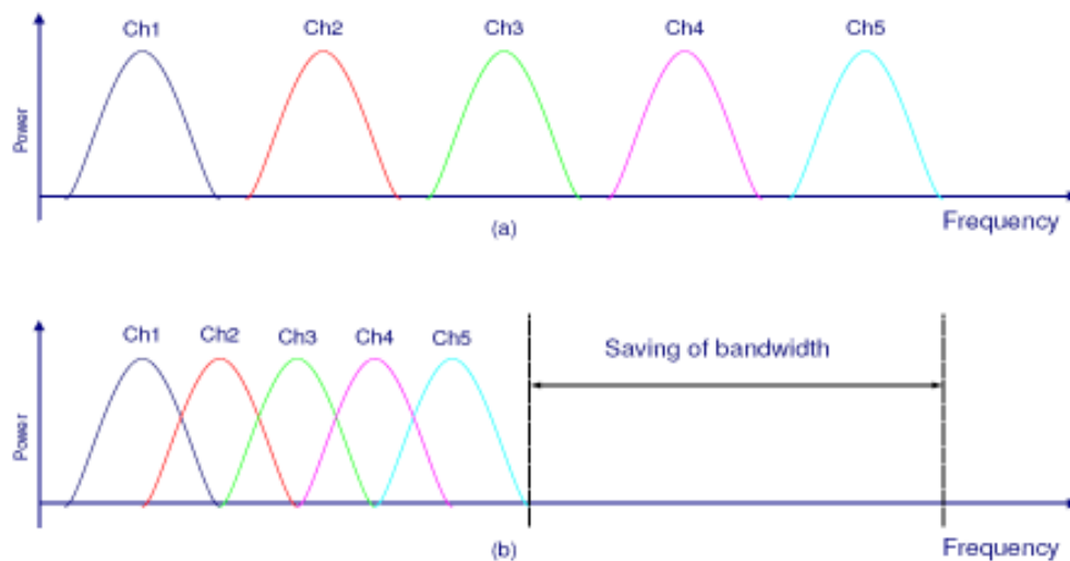
Figura 3-7 Acceso Múltiple por División Ortogonal de Frecuencia: a) Técnica Multiportadora convencional, b) Modulación con portadoras ortogonales.
