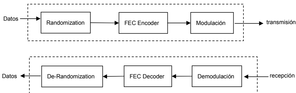
Figura 4-1 Diagrama conceptual del modelo WiMAX.
