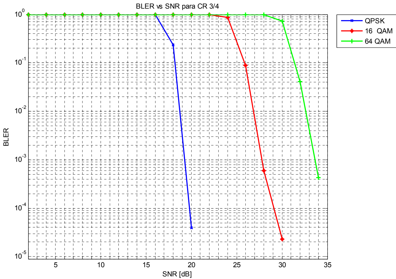
Figura 4-4 BLER vs SNR para CR \frac{3}{4}
