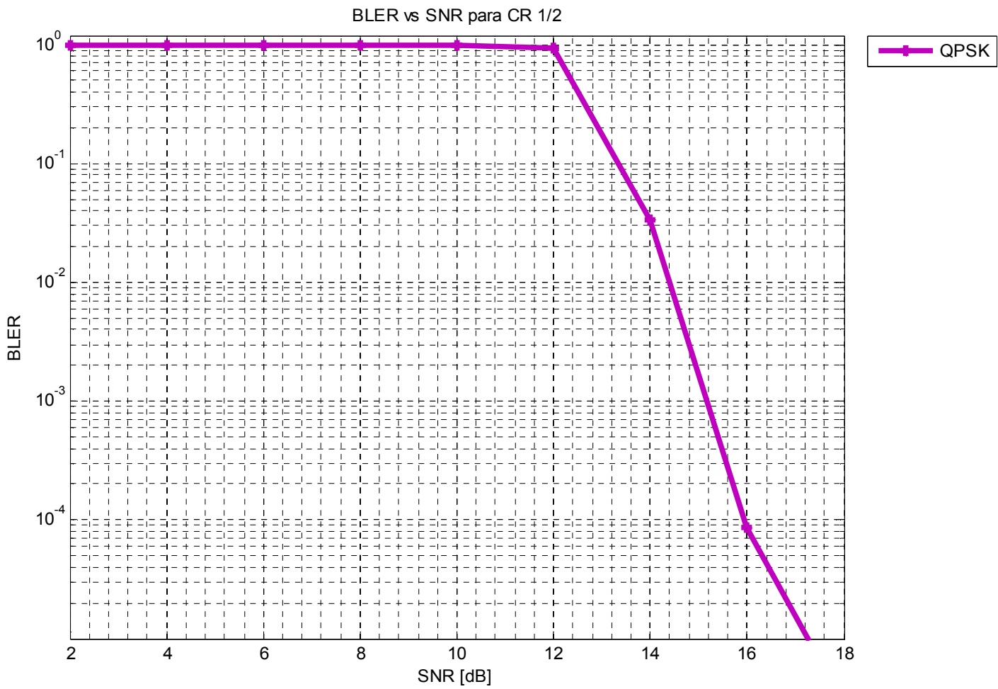
Figura 4-6 BLER vs SNR para CR 1/2
