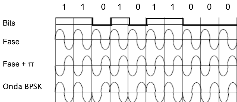
Figura 3-2 Esquema de modulación BPSK.
