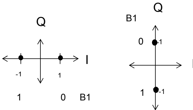
Figura 3-3 Constelación de la modulación BPSK.
