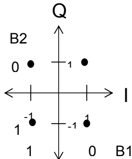
Figura 3-4 Constelación de la modulación QPSK.
