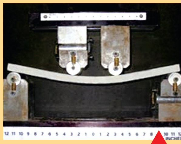
Imagen 3. Hormigón bajo flexión. Un refuerzo con alto contenido de fibras produce un hormigón “flexible”.
