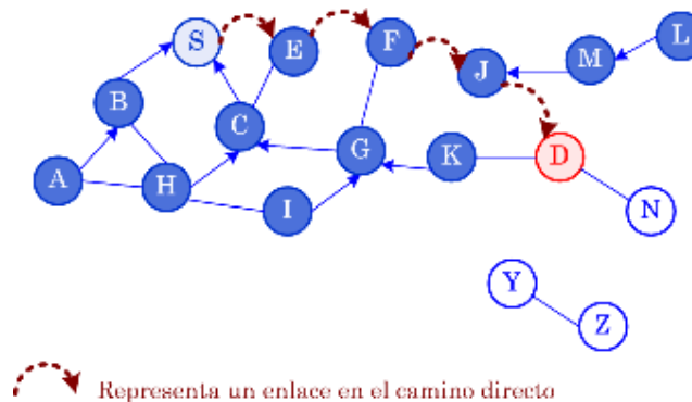
Figura 5.8 Se crea la ruta del nodo S al nodo D
