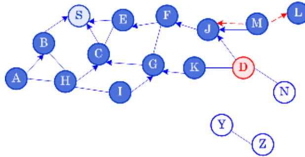
Figura 5.6 El nodo D no reenvía el RREQ
