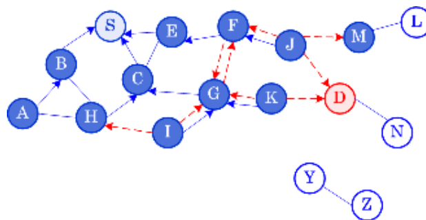
Figura 5.5 Llegada de la petición a RREQ a nodo D
