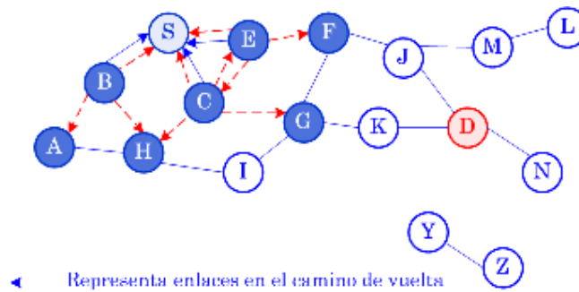
Figura 5.3 Flooding del Mensaje RREQ
