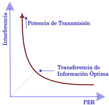
Figura 7.7 Relación entre Interferencia, PER y Potencia de Transmisión
