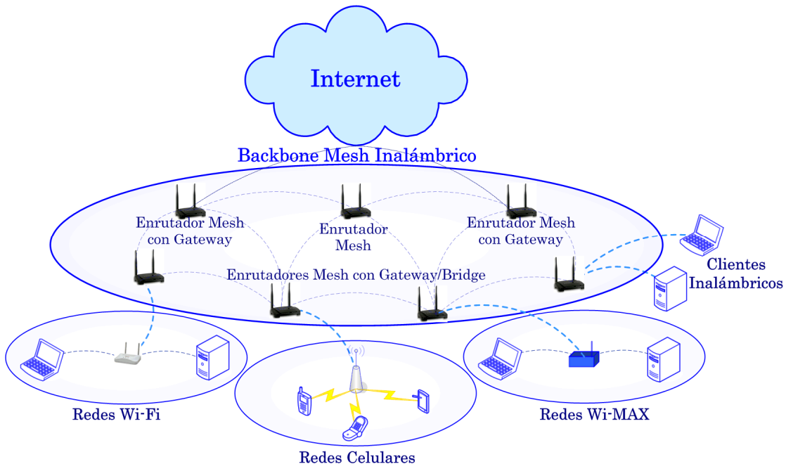
Figura 6.2. Infraestructura/Backbone de las WMNs
