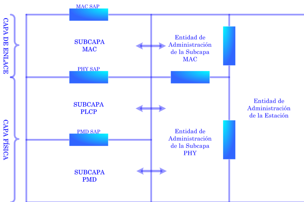
Figura 2.4 Modelo Básico de Referencia
