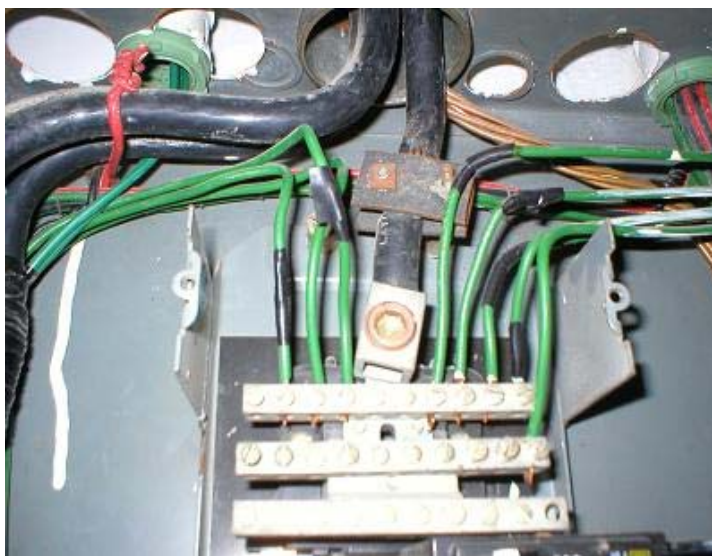
Figura 3.7 Alimentador del neutro con empalme mal hecho.
