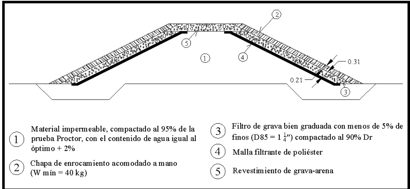
Figura 94. Sección de bordo propuesta para lagunas de sedimentación.
