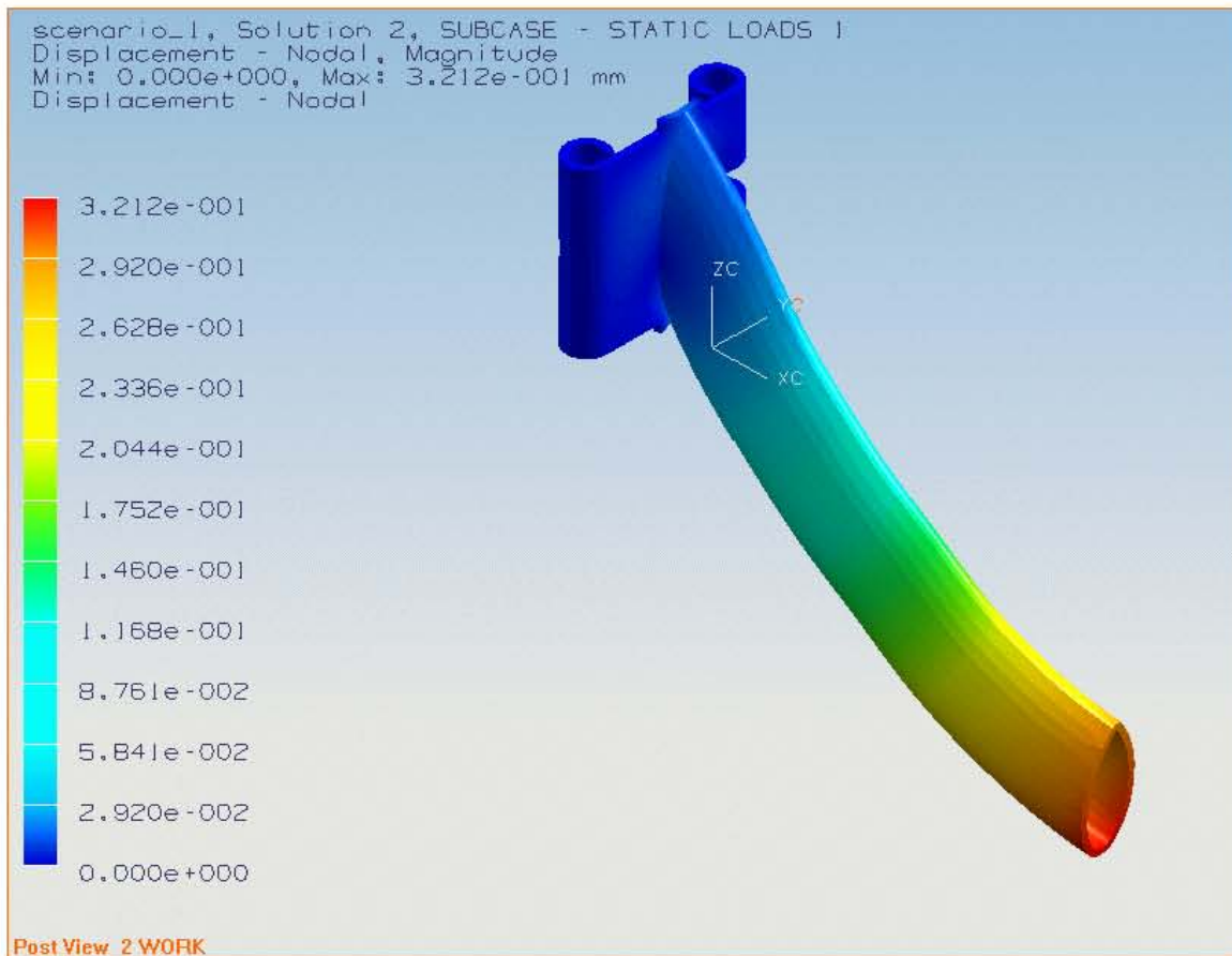
Fig. 5.19 Análisis por elemento finito del tubo central lado derecho, desplazamiento. Solución 2.
