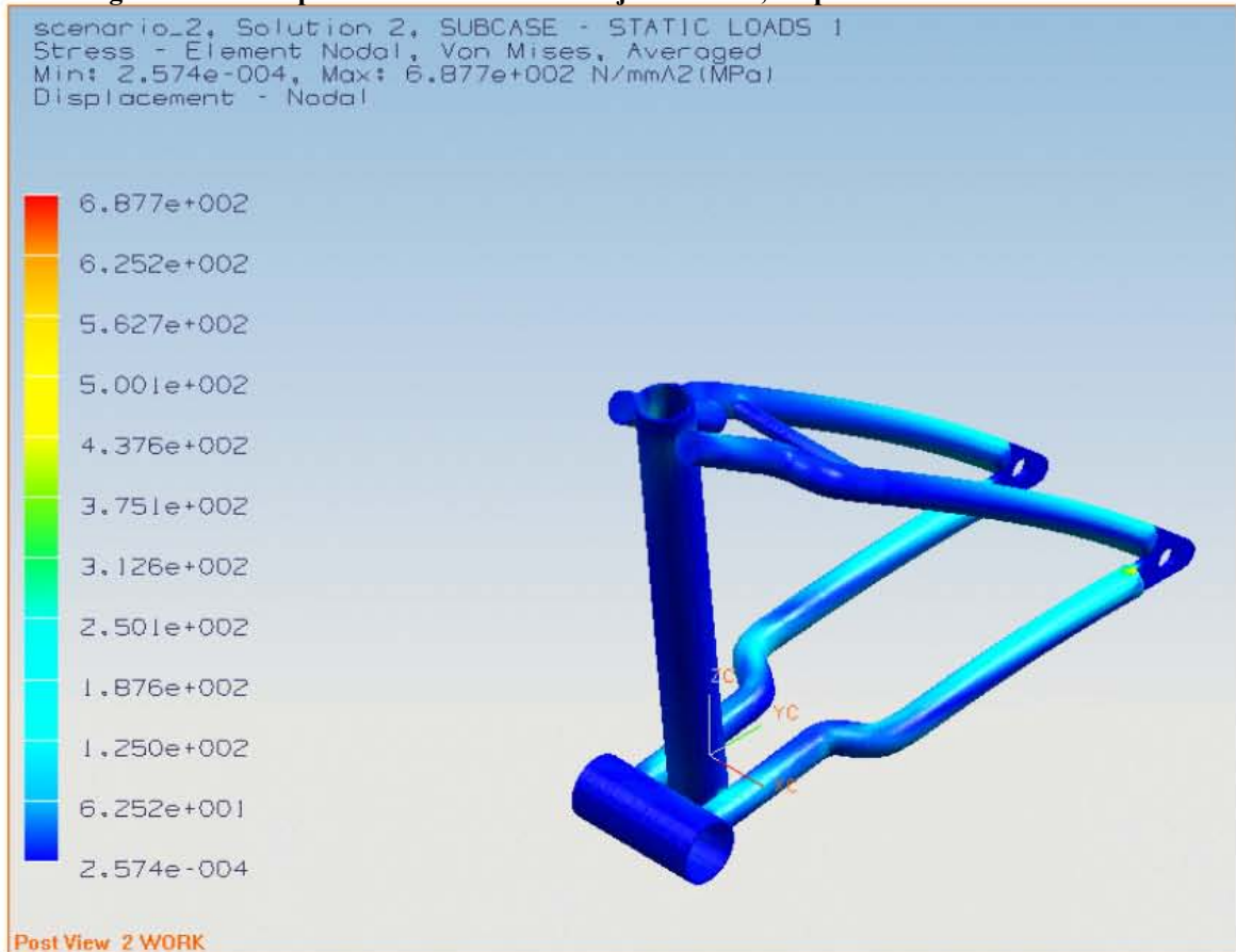
Fig. 5.14 Análisis por elemento finito de la tijera trasera, esfuerzo Von mises. Solución 2.
