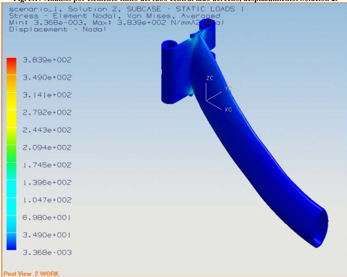
Fig. 5.20 Análisis por elemento finito del tubo central lado derecho, esfuerzo Von mises. Solución 2.
