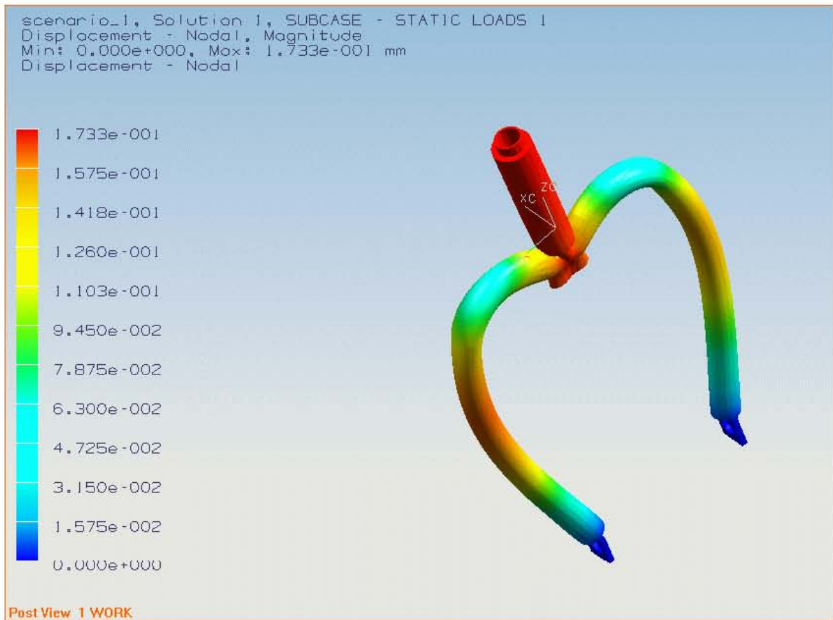
Fig. 5.7 Análisis por elemento finito tijera delantera, desplazamiento.
