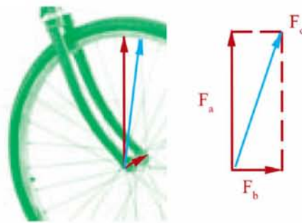
Fig. 5.6 Componentes horizontal y vertical en los radios de la rueda.
