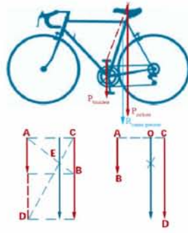
Fig. 5.5-b El peso del ciclista y la bici que se consideran.
