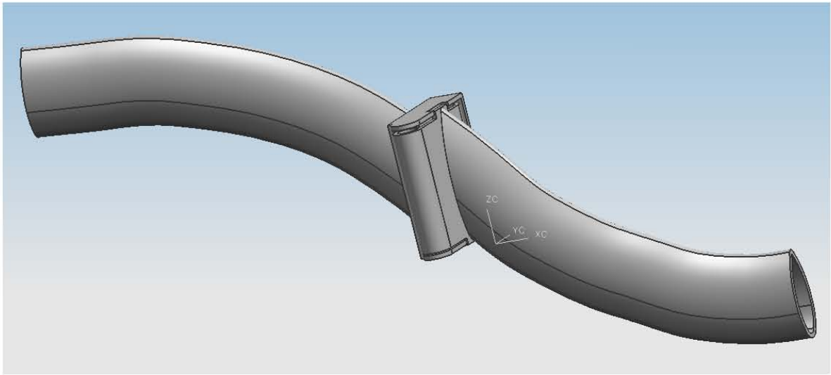
Fig. 5.4 Modelo en 3D Tubo central, ensamble.
