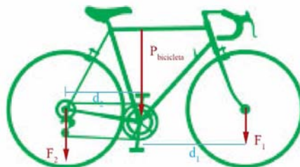
Fig. 5.5a. Fuerzas ejercidas sobre la bicicleta.
