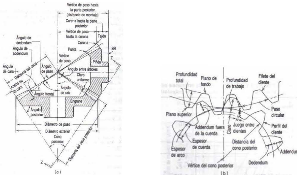
Fig. 4.20 a-b Engranajes cónicos rectos.
