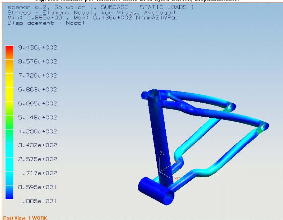
Fig. 5.12 Análisis por elemento finito de la tijera trasera, esfuerzo Von mises.
