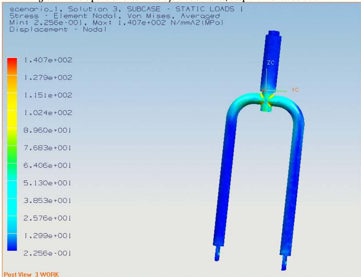
Fig. 5.10 Análisis por elemento finito tijera de enfrente, esfuerzo Von mises. Solución 2
