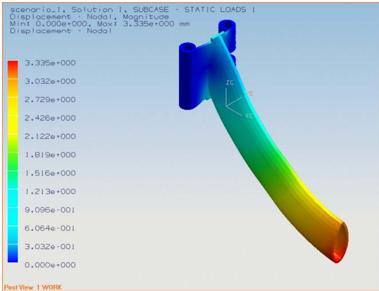
Fig. 5.17 Análisis por elemento finito del tubo central lado derecho, desplazamiento. Solución 1.
