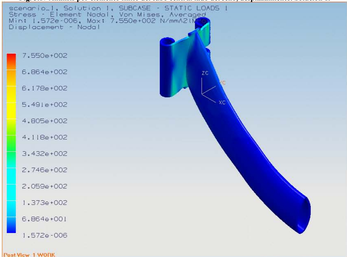
Fig. 5.18 Análisis por elemento finito del tubo central lado derecho, esfuerzo Von mises. Solución 1.
