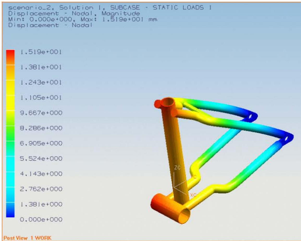
Fig. 5.11 Análisis por elemento finito de la tijera trasera, desplazamiento.
