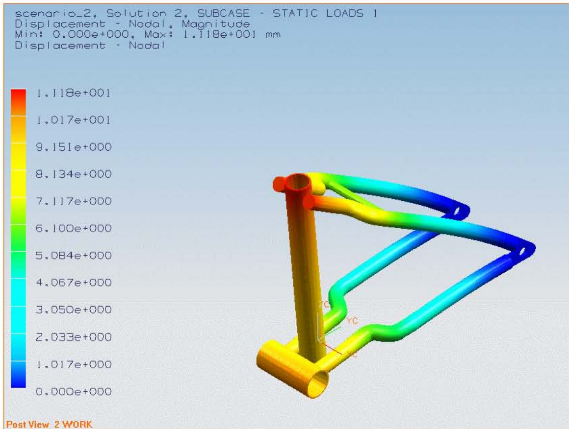
Fig. 5.13 Análisis por elemento finito de la tijera trasera, desplazamiento. Solución 2.
