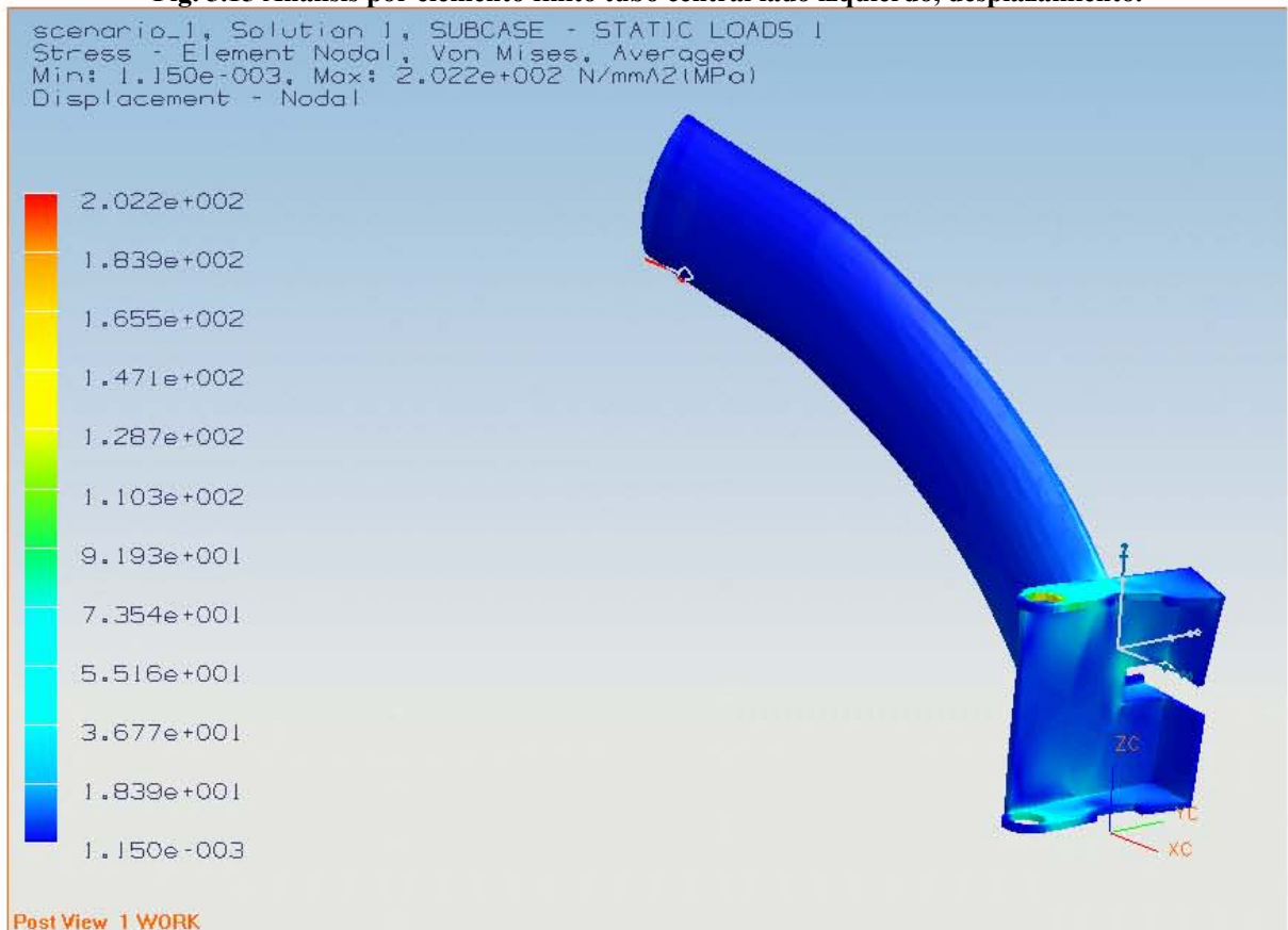
Fig. 5.16 Análisis por elemento finito del tubo central izquierdo, esfuerzo Von mises.
