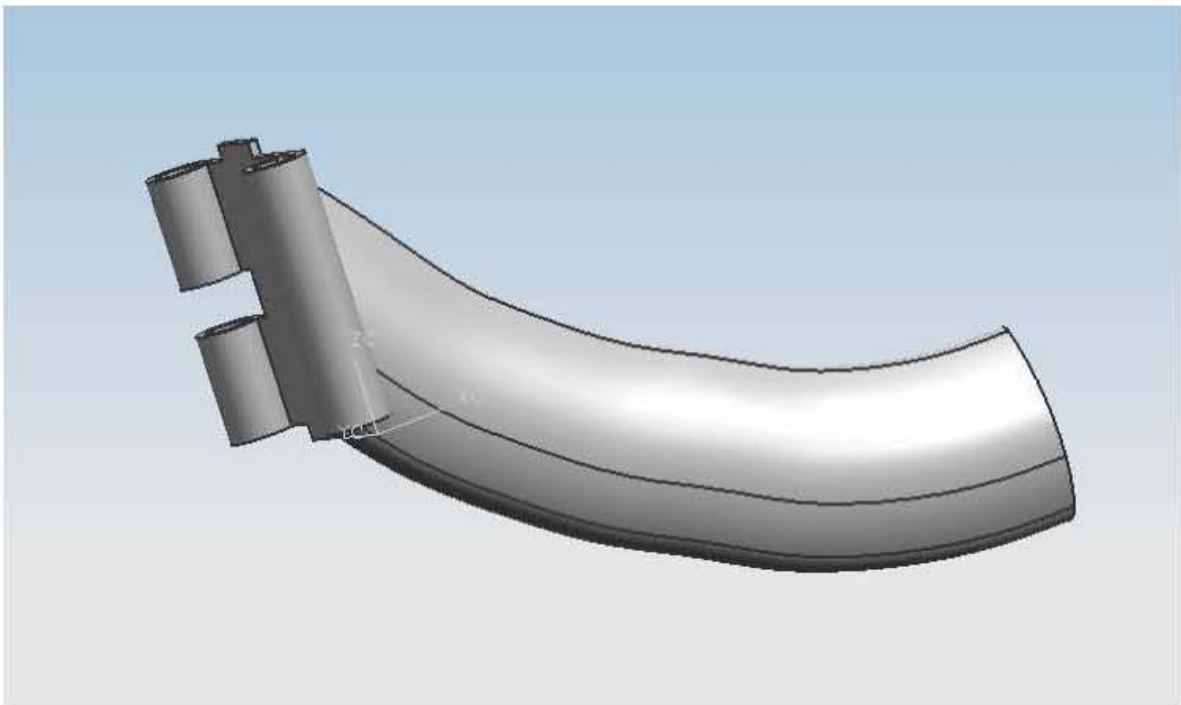
Fig. 5.3 Modelo en 3D. Tubo central parte derecha.
