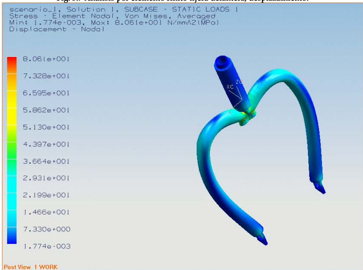
Fig. 5.8 Análisis por elemento finito tijera delantera, esfuerzo Von mises.
