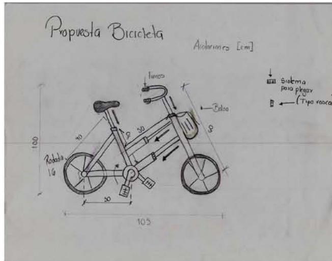
Fig. 3.5-b Boceto de la primera propuesta.
