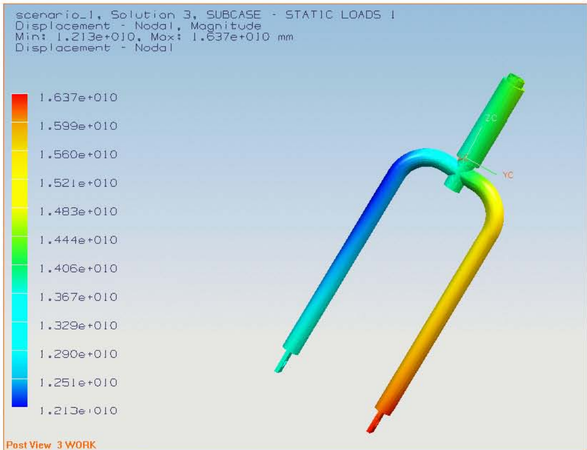
Fig. 5.9 Análisis por elemento finito tijera de enfrente, desplazamiento. Solución 2.
