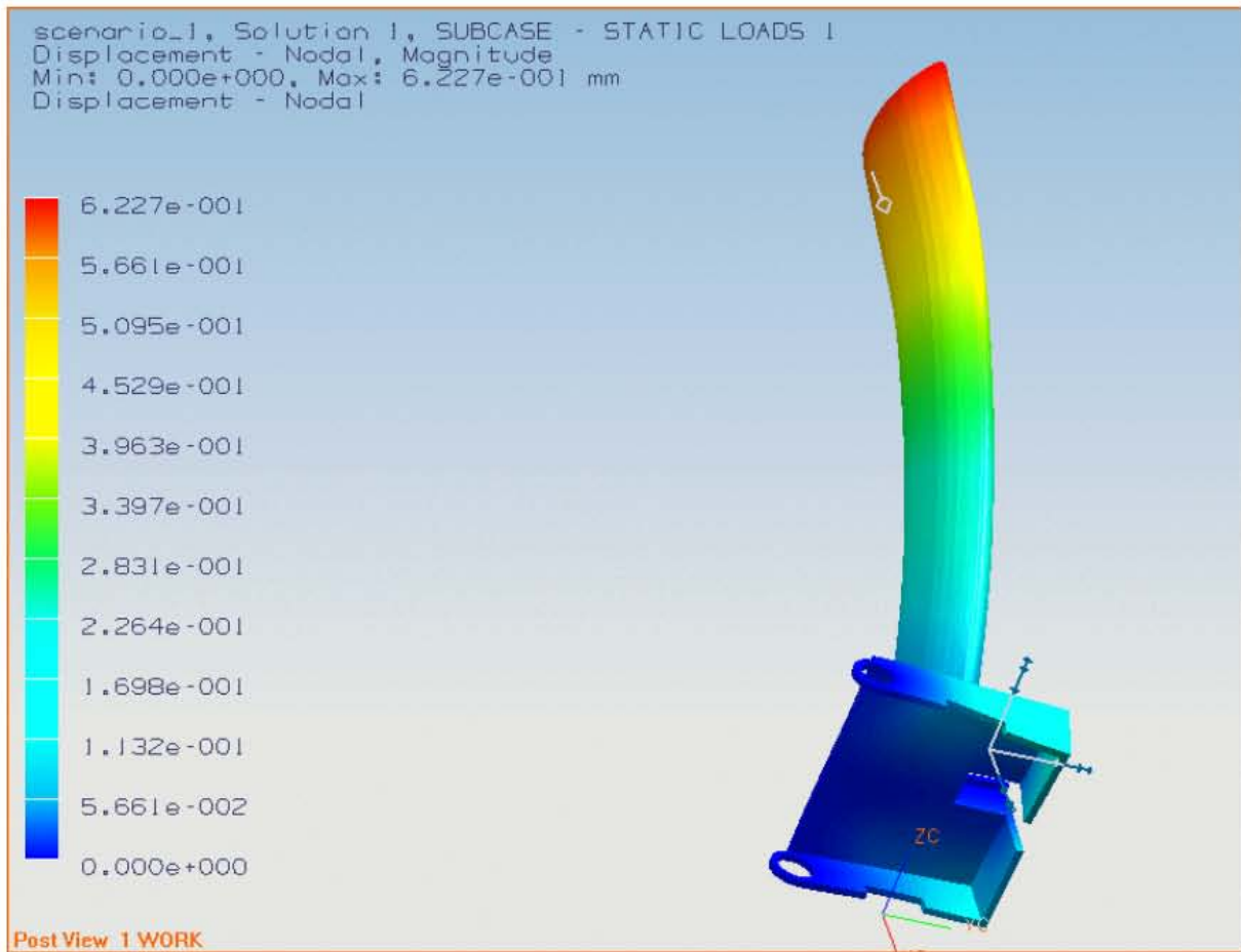
Fig. 5.15 Análisis por elemento finito tubo central lado izquierdo, desplazamiento.
