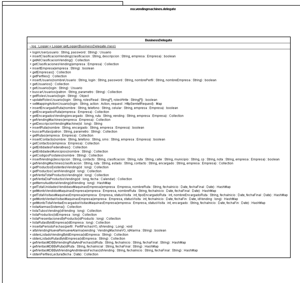
Figura 5.40 Diagrama de Clases 5
