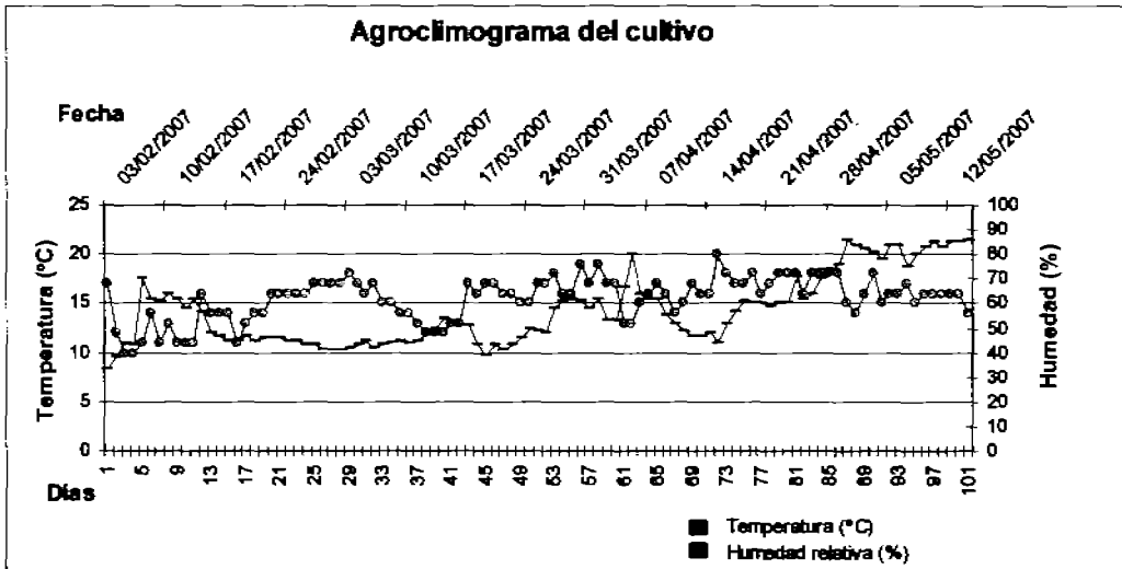
Fig. 4.10. Agroclimograma completo del cultivo.
