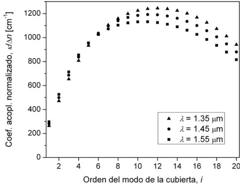
Figura 4.2 Coeficientes de acoplamiento cruzado normalizados para modos de la cubierta LP_{0i} , i = 1 \dots 20 , y diferente longitud de onda \lambda .
