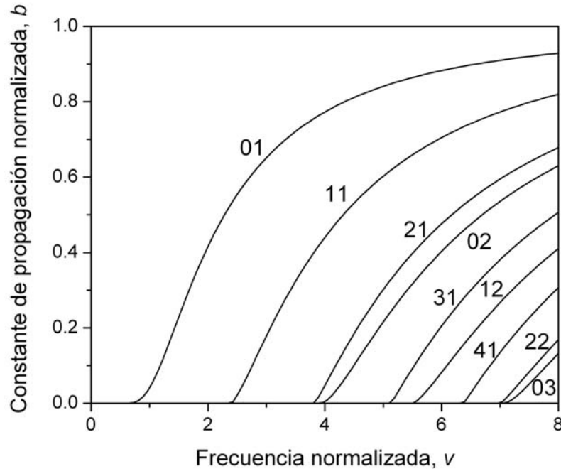
Figura 3.6 Constante de propagación normalizada en función de la frecuencia normalizada para diferentes modos LP.
