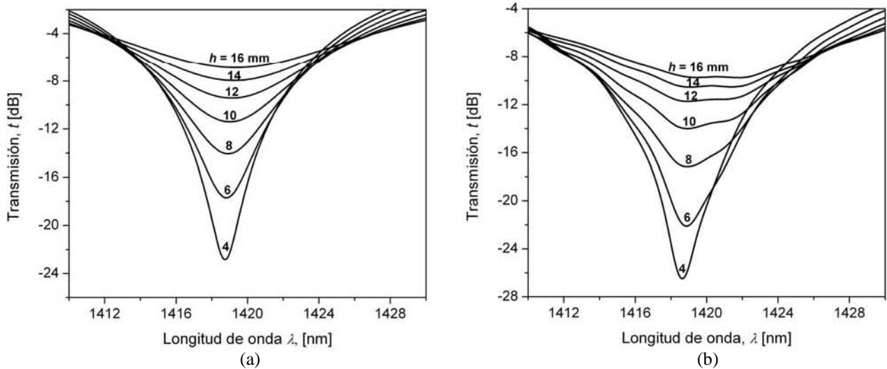
Figura 5.9 Espectros de transmisión de la rejilla de período largo variable para diferentes valores del nivel del líquido h . (a) Espectros obtenidos con la simulación; (b) Espectros medidos experimentalmente.
