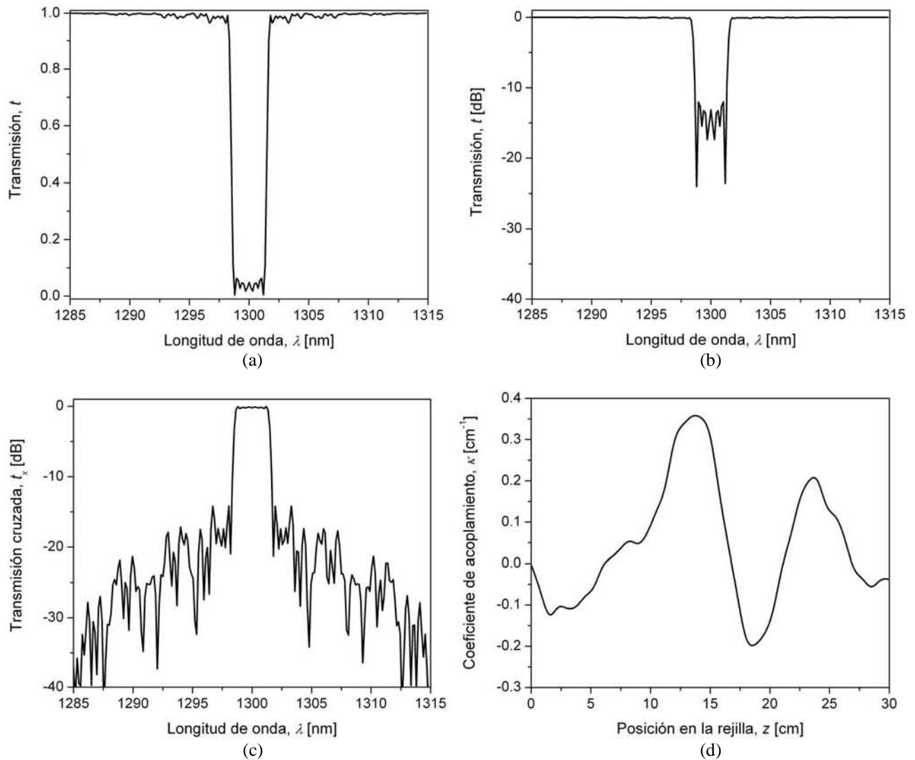
Figura 4.18 Rejilla sintetizada con \lambda_c = 1300 nm y banda de rechazo de 3 nm. (a) Transmisión t(\lambda) ; (b) Transmisión en decibels t(\lambda) ; (c) Transmisión cruzada en decibels t_x(\lambda) ; (d) Perfil del coeficiente de acoplamiento \kappa(z) .
