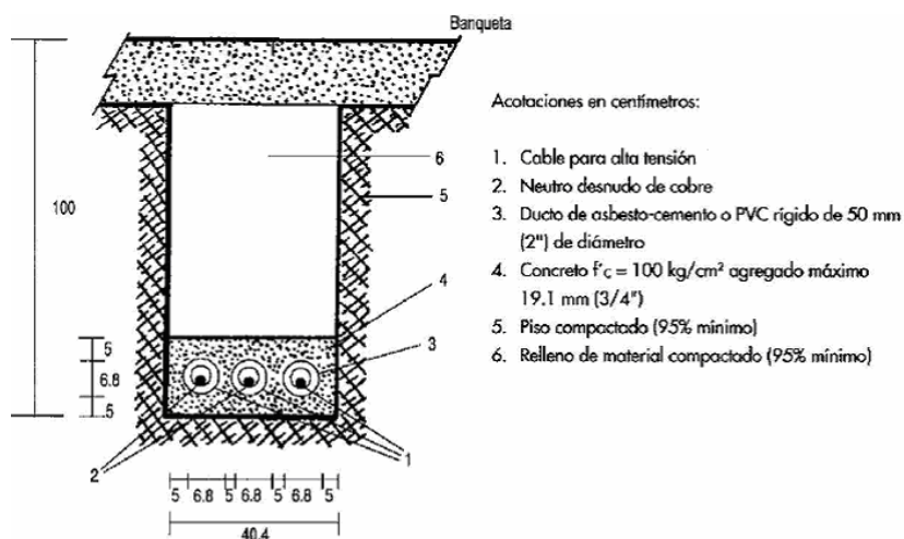
FIGURA 32. DUCTOS
