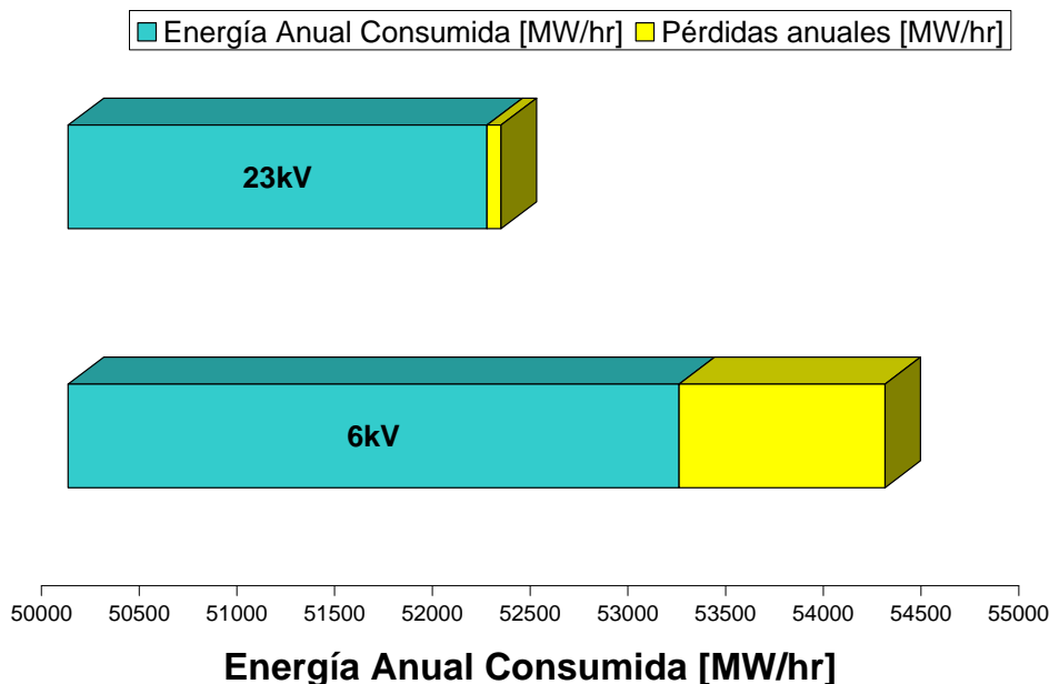
GRAFICA 40. COMPARATIVA DE LA ENERGÍA ANUAL CONSUMIDA ENTRE TENSIONES.
