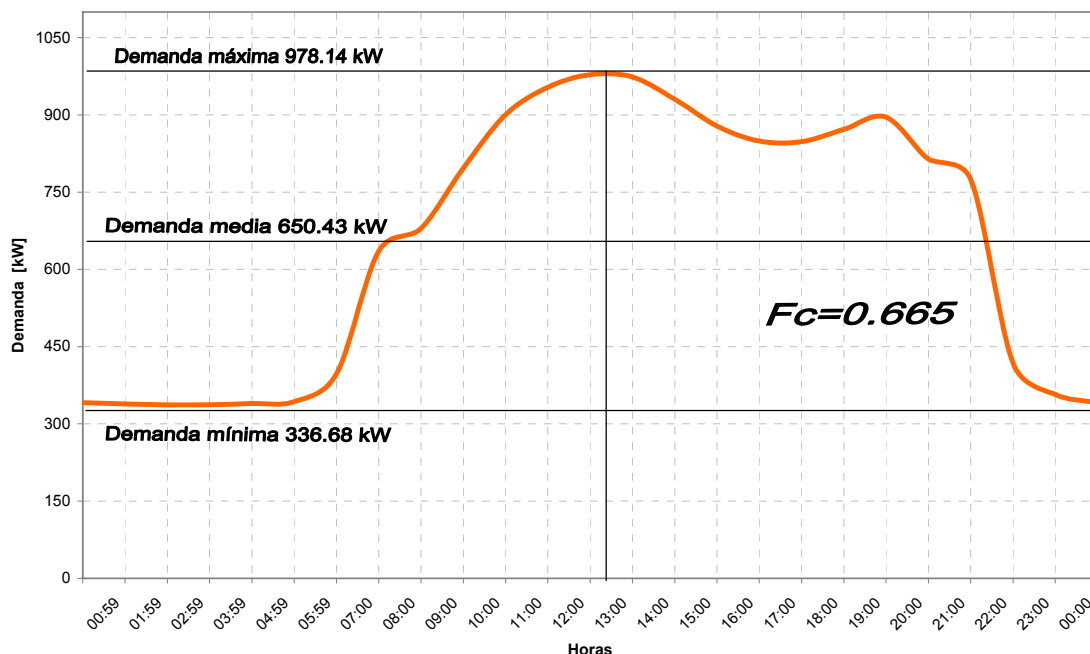
GRAFICA 28. CURVA DE DEMANDA PROMEDIO DIARIA ANUAL DEL ALIMENTADOR "J".
