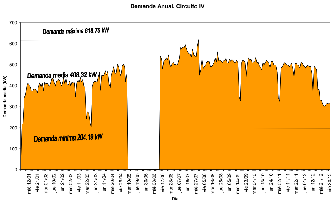
GRAFICA 39. CURVA DE DEMANDA ANUAL DEL CIRCUITO "IV"
