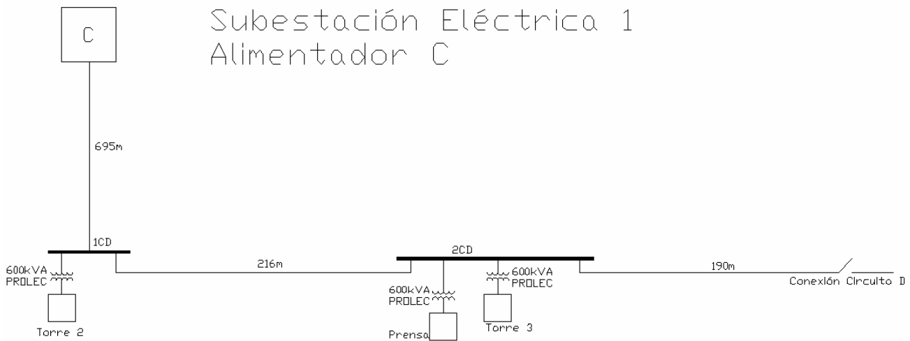
DIAGRAMA 18. DIAGRAMA UNIFILAR DEL ALIMENTADOR "C"
