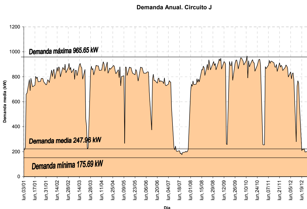
GRAFICA 29. CURVA DE DEMANDA ANUAL DEL ALIMENTADOR "J"
