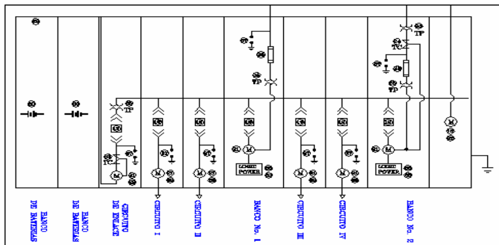
DIAGRAMA 30. ALIMENTADORES DERIVADOS SUBESTACIÓN GENERAL No. 2
