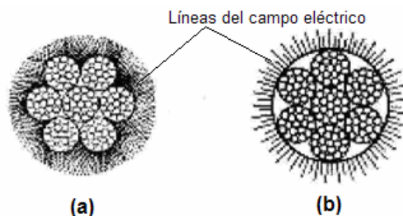
FIGURA 20. (a) CONDUCTOR SIN PANTALLA SEMICONDUCTORA SOBRE EL CONDUCTOR. (b) CONDUCTOR CON PANTALLA SEMICONDUCTORA SOBRE EL CONDUCTOR.
