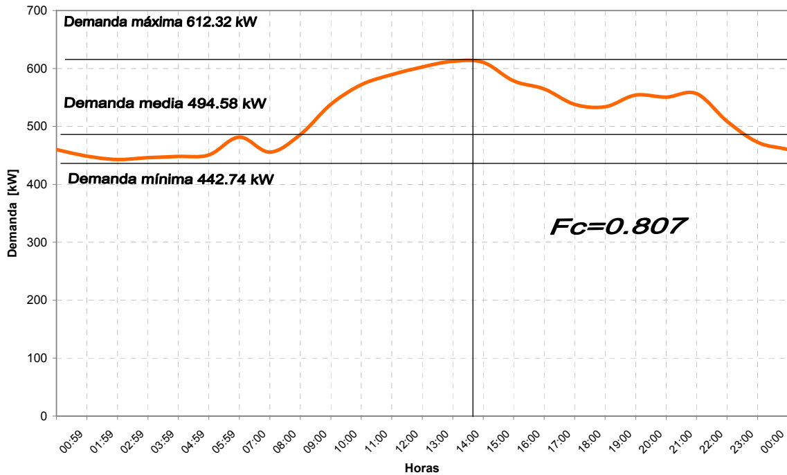
GRAFICA 13. CURVA DE DEMANDA PROMEDIO DIARIA DURANTE UN AÑO DEL ALIMENTADOR "F"
