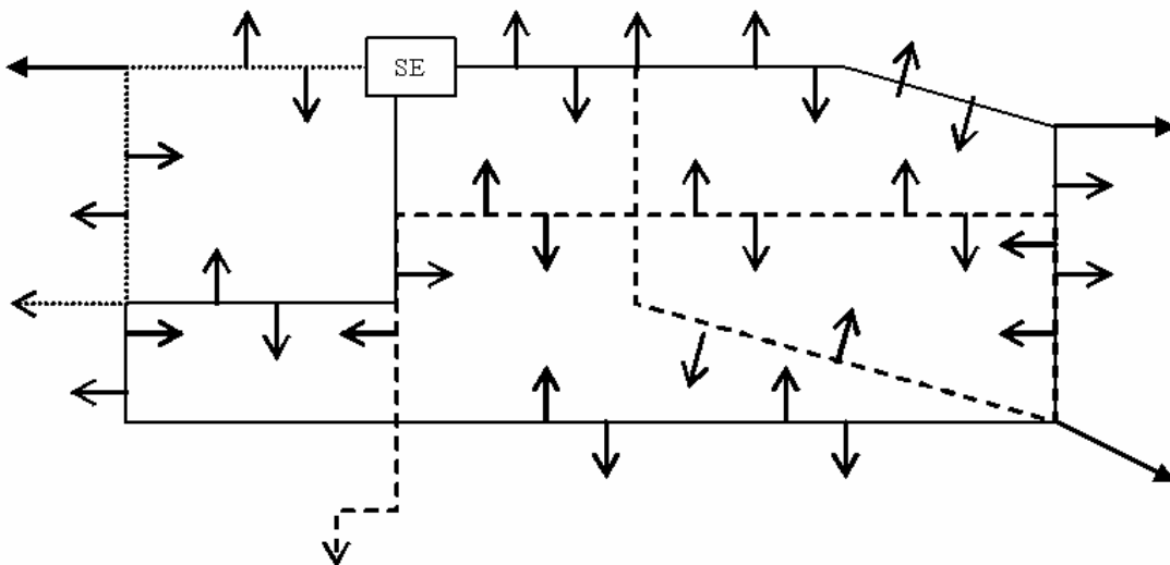
DIAGRAMA 5. SECCIONAMIENTO DE UNA ESTRUCTURA RADIAL
