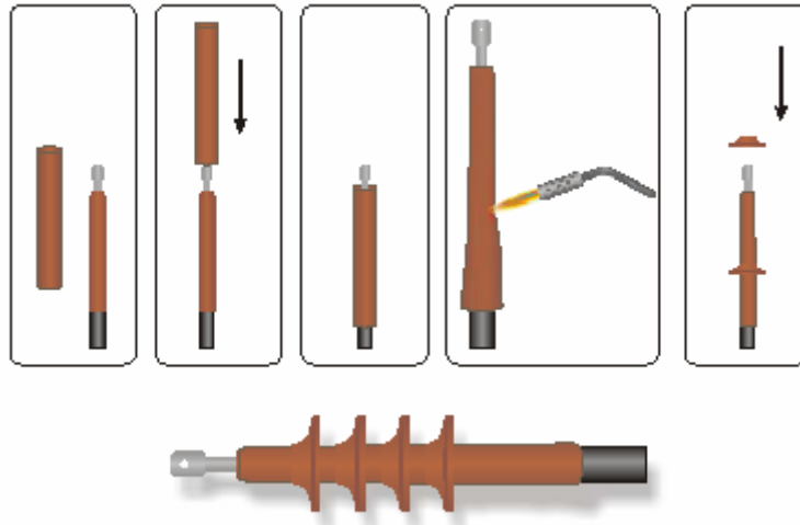
FIGURA 27. TERMINAL TIPO TERMOCONTRÁCTIL MT
