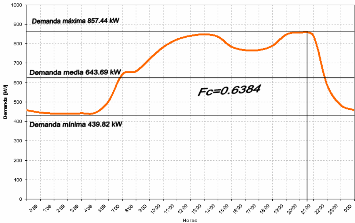
GRAFICA 17. CURVA DE DEMANDA PROMEDIO DIARIA DURANTE UN AÑO DEL ALIMENTADOR "G"
