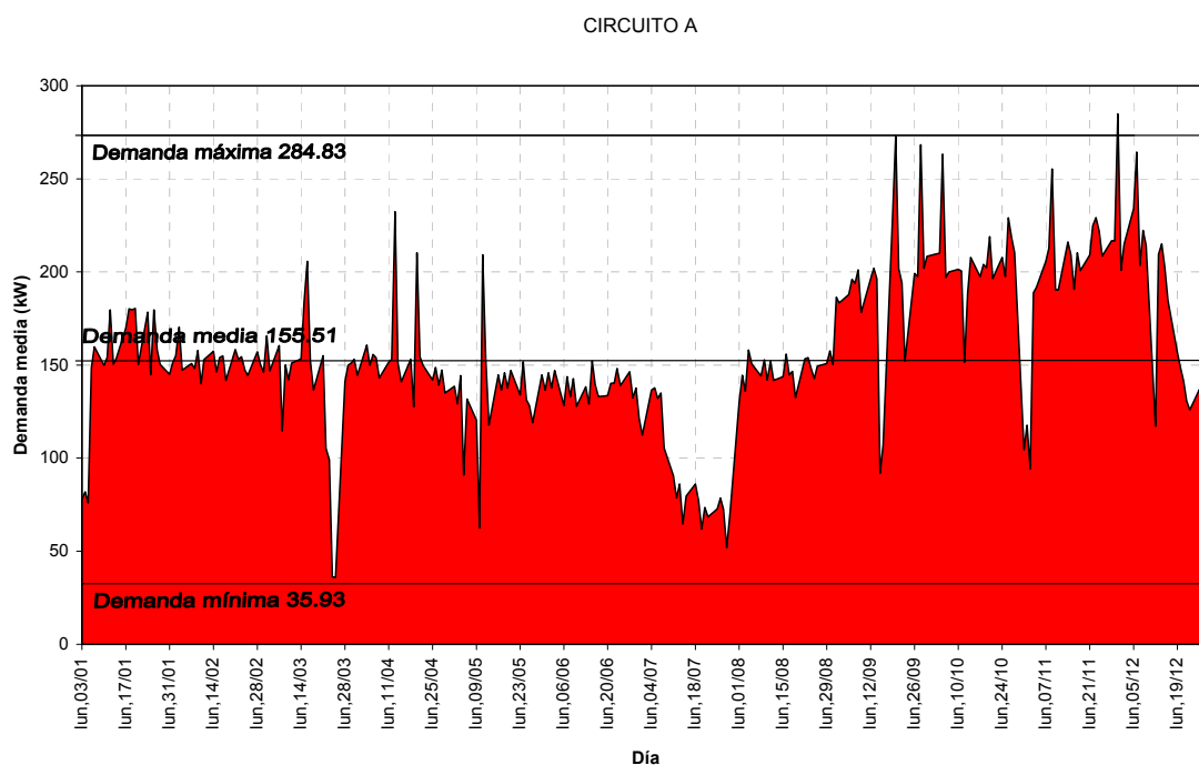
GRAFICA 8. CURVA DE DEMANDA ANUAL DEL ALIMENTADOR "A"
