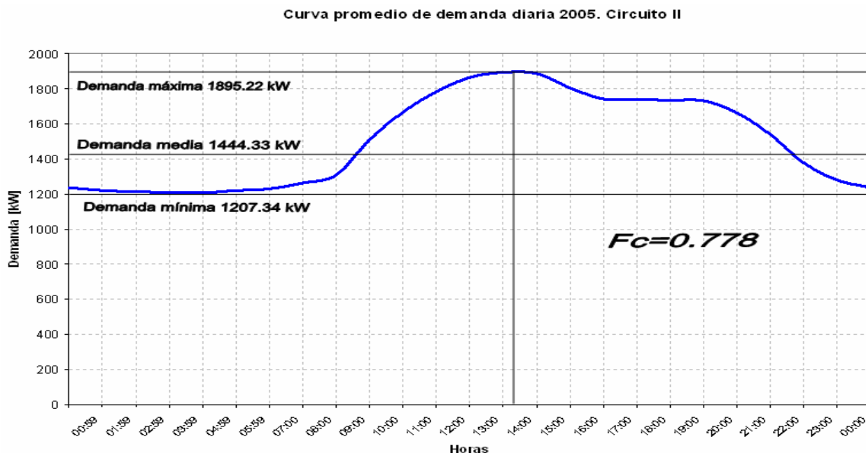
GRAFICA 34. CURVA DE DEMANDA PROMEDIO DIARIA DURANTE UN AÑO DEL CIRCUITO "II"
