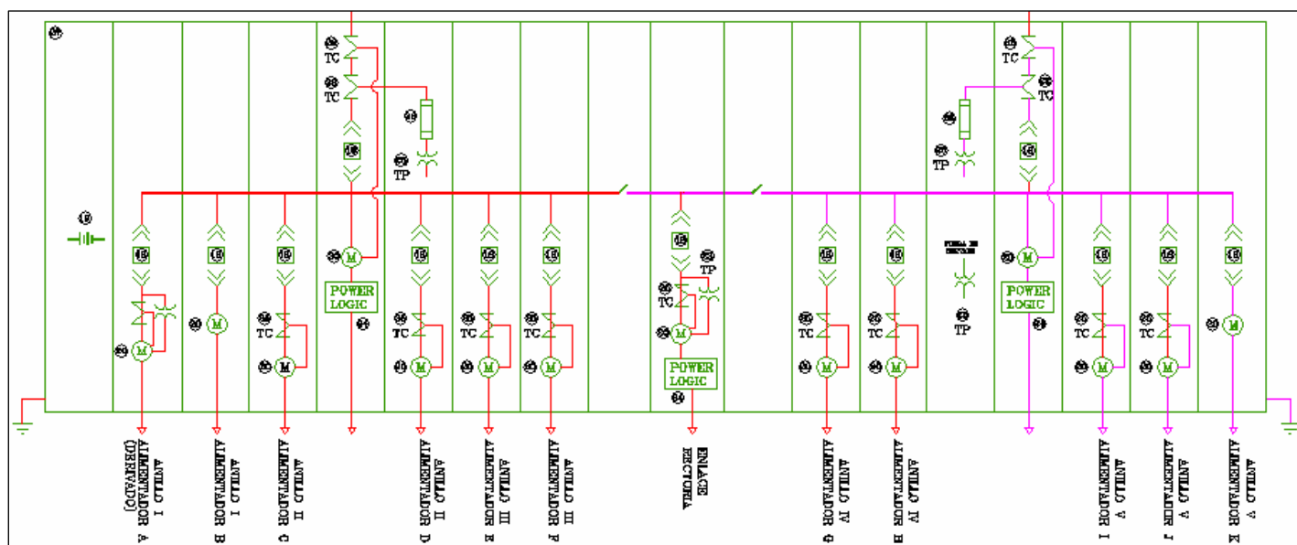
DIAGRAMA 15. ALIMENTADORES DERIVADOS DE LA SUBESTACIÓN GENERAL No. 1
