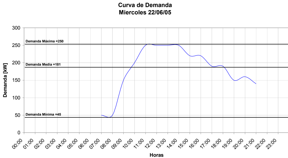
GRAFICA 21. CURVA DE DEMANDA DE UN DÍA EXTRAORDINARIO DE ACTIVIDADES DEL ALIMENTADOR "H"
