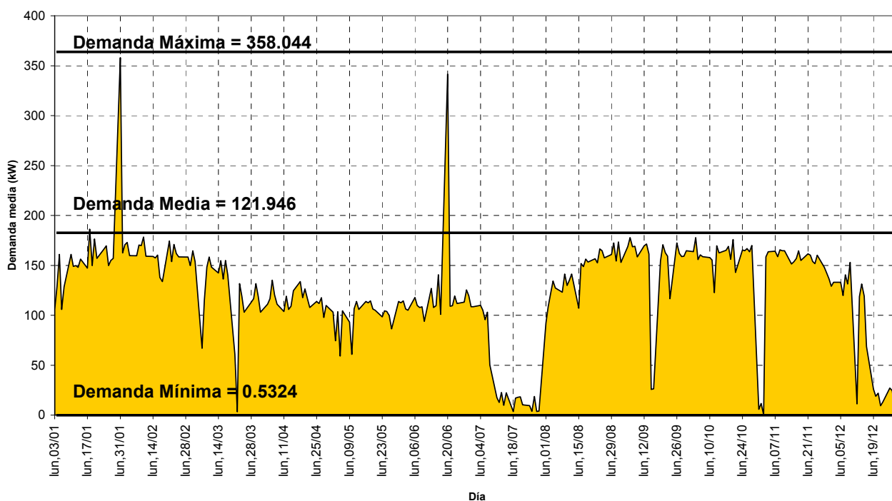
GRAFICA 25. CURVA DE DEMANDA ANUAL DEL ALIMENTADOR "H"
