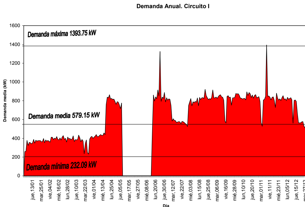
GRAFICA 33. CURVA DE DEMANDA ANUAL DEL CIRCUITO "I"
