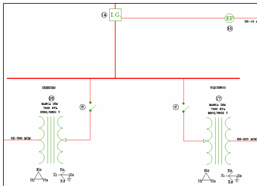
DIAGRAMA 14. TRANSFORMADORES DE LA SUBESTACIÓN GENERAL No. 1
