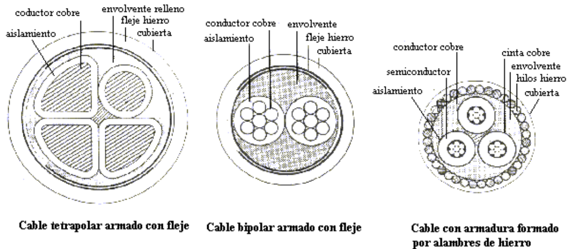
FIGURA 22. CLASIFICACIÓN DE CABLES SUBTERRÁNEOS MULTIPOLARES
