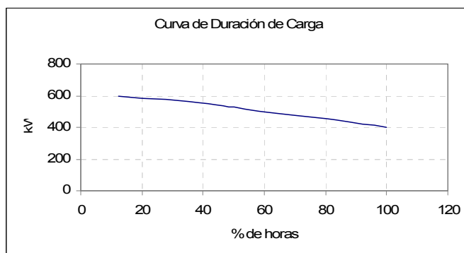
GRAFICA 14. CURVA DE DURACIÓN DE CARGA EN EL ALIMENTADOR "F"
