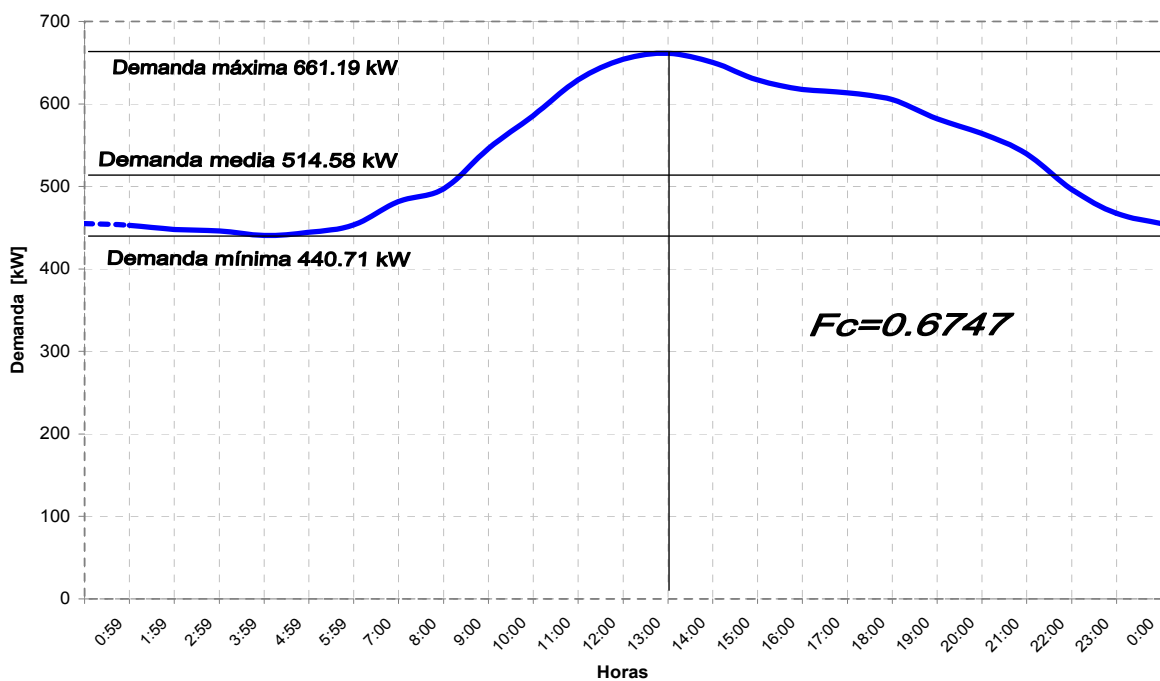
GRAFICA 36. CURVA DE DEMANDA PROMEDIO DIARIA DURANTE UN AÑO DEL CIRCUITO "III"
