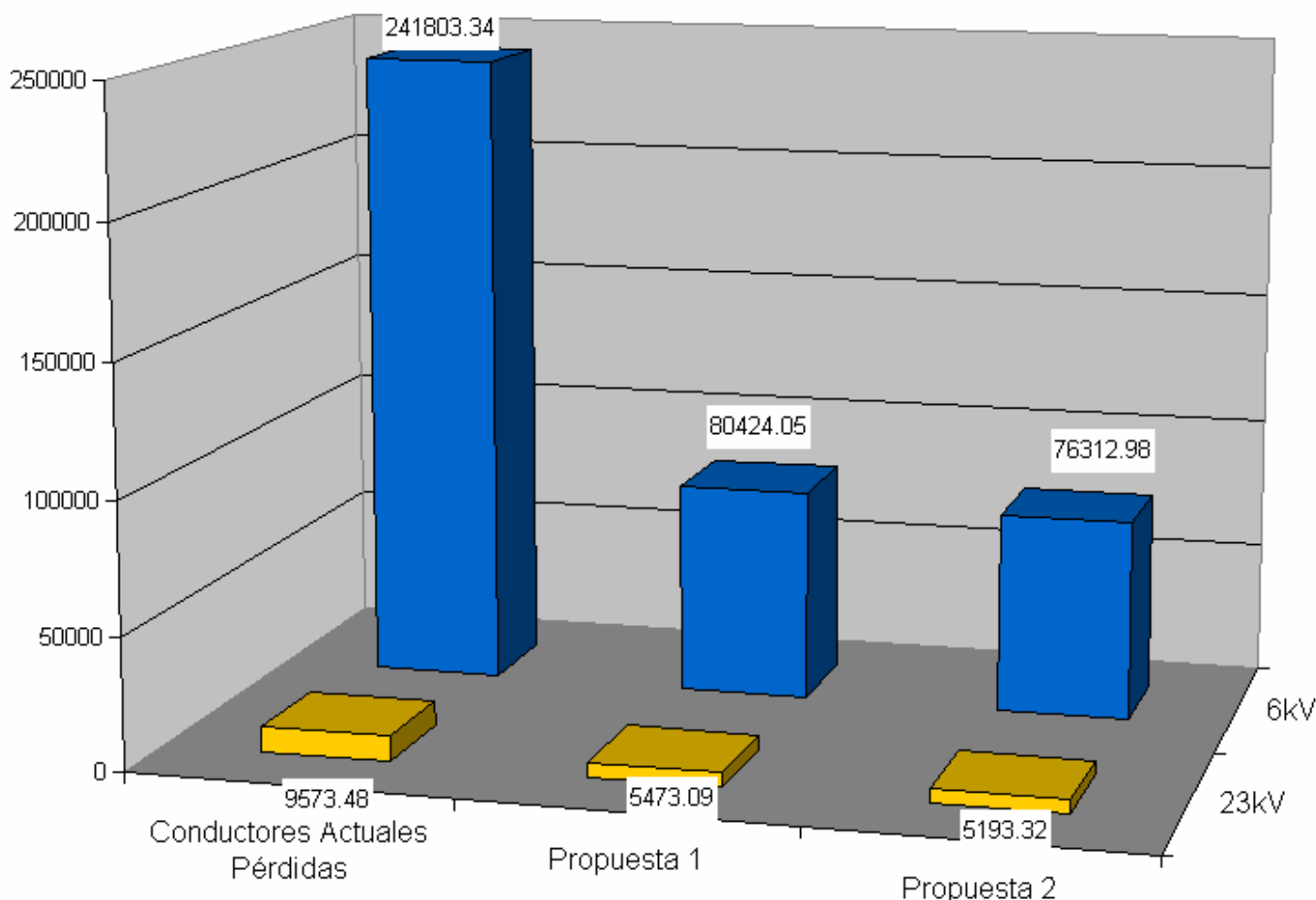
GRAFICA 41. REDUCCIÓN DE PÉRDIDAS
