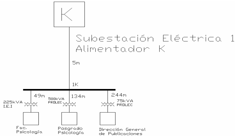
DIAGRAMA 26. DIAGRAMA UNIFILAR DEL ALIMENTADOR "K"
