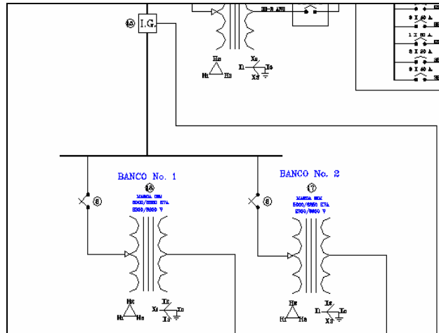
DIAGRAMA 29. TRANSFORMADORES SUBESTACIÓN GENERAL No. 2
