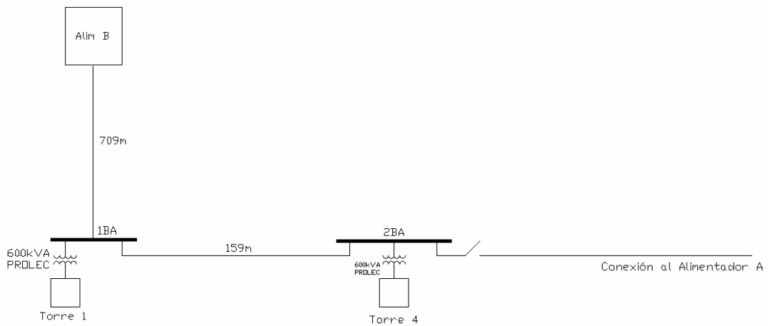
DIAGRAMA 17. DIAGRAMA UNIFILAR DEL ALIMENTADOR "B"
