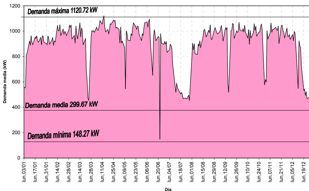
Demanda Anual. Circuito I
