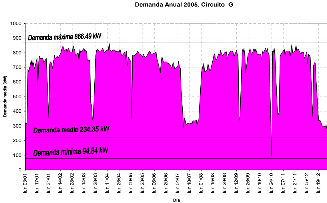
GRAFICA 18. CURVA DE DEMANDA DURANTE UN AÑO DEL ALIMENTADOR "G"
