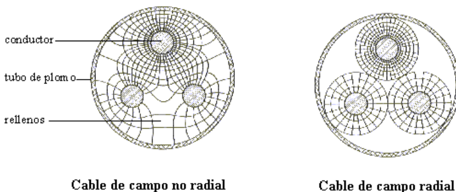
FIGURA 23. CLASIFICACIÓN DE CABLES SUBTERRÁNEOS POR TIPO DE CAMPO
