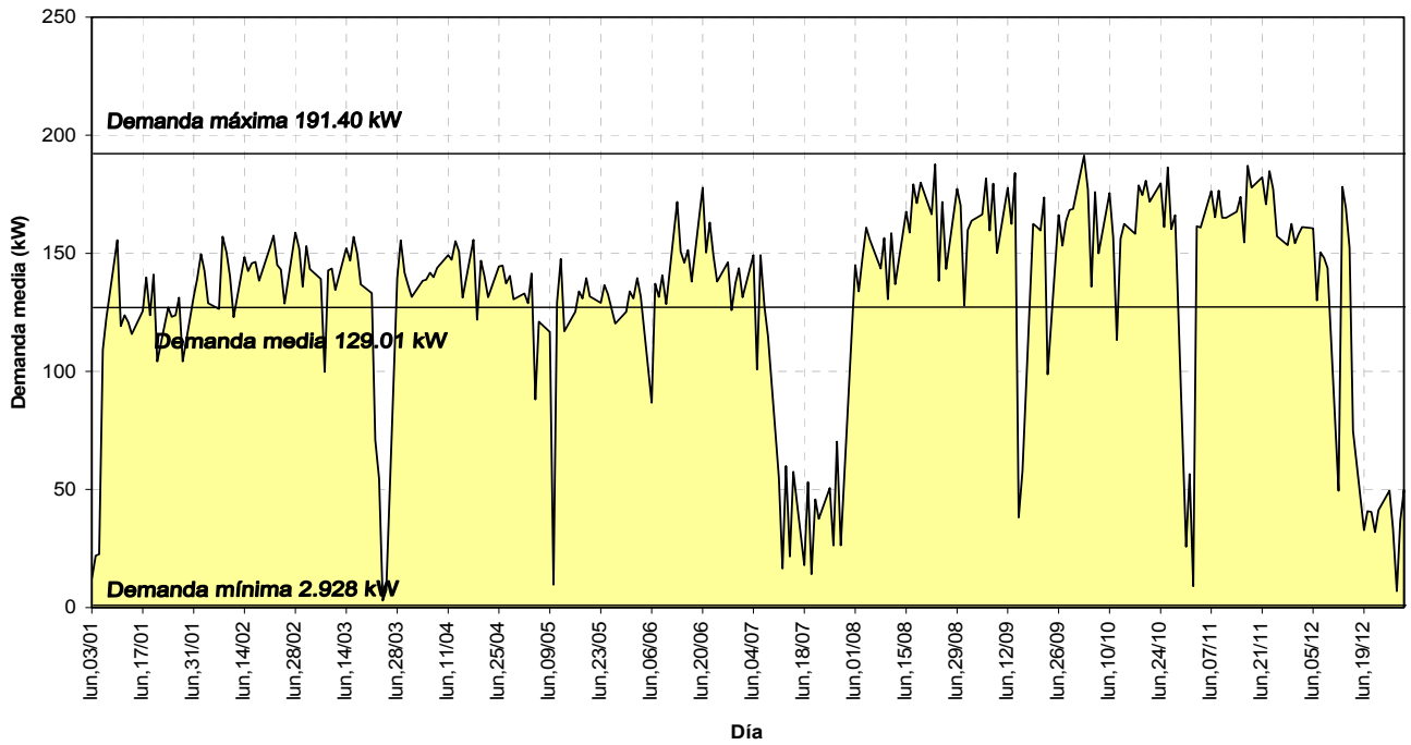
GRAFICA 31. CURVA DE DEMANDA ANUAL DEL ALIMENTADOR "K"
