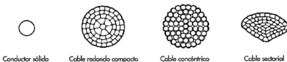
FIGURA 18 . FORMAS DE CONDUCTORES
