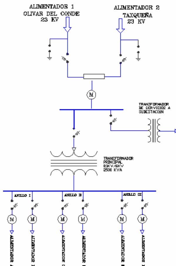
DIAGRAMA 1. SUBESTACIÓN PRINCIPAL No. 1. 1952
