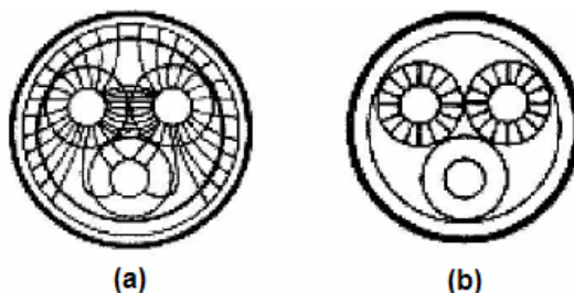
FIGURA 21. ESFUERZOS ELÉCTRICOS EN: (a) CABLE SIN PANTALLA SOBRE EL AISLAMIENTO (b) CABLE CON PANTALLA SOBRE EL AISLAMIENTO
