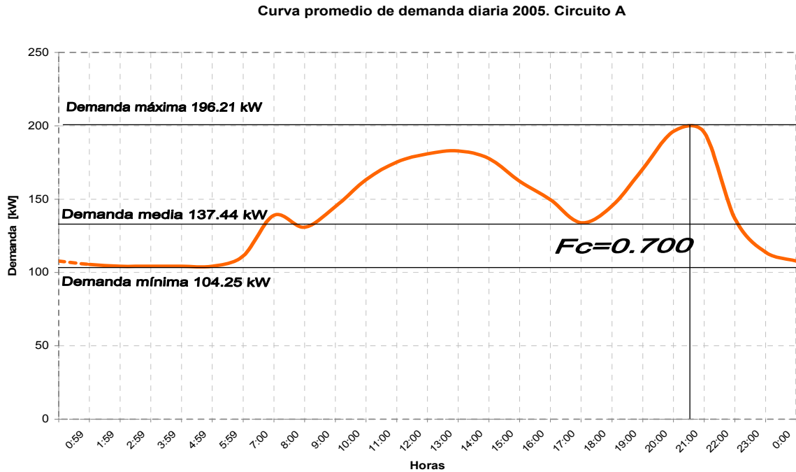
GRAFICA 5. CURVA DE DEMANDA PROMEDIO DIARIA EL ALIMENTADOR "A"
