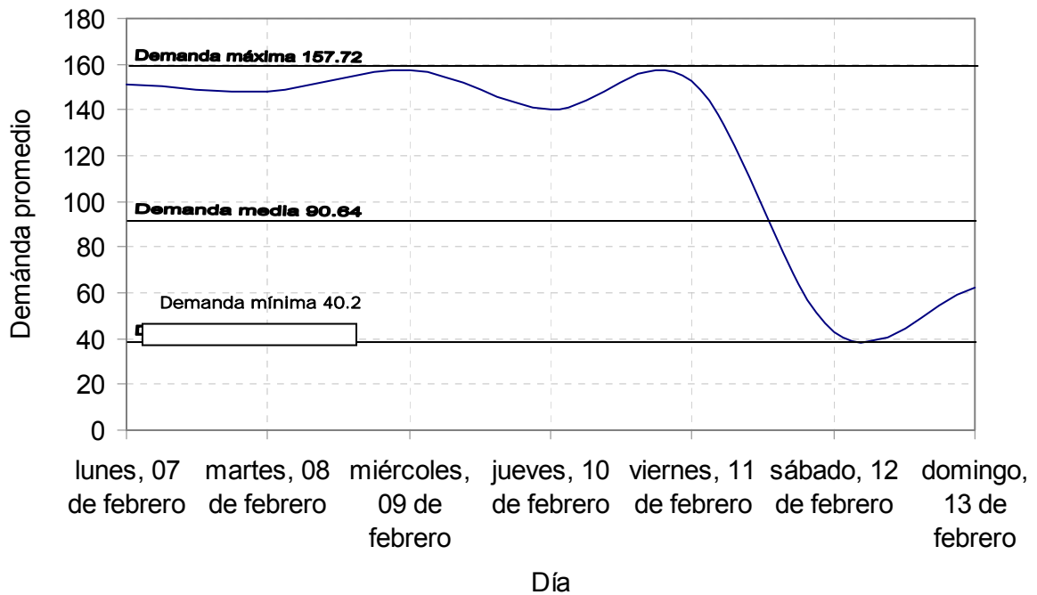
GRAFICA 7. CURVA DE DEMANDA SEMANAL DEL ALIMENTADOR "A"
