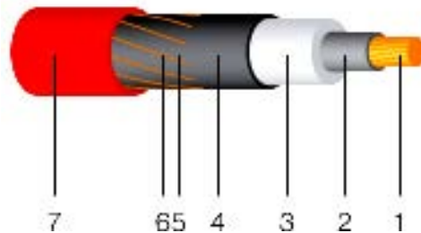
FIGURA 17. SECCIÓN DE UN CABLE SUBTERRÁNEO DE ENERGÍA
