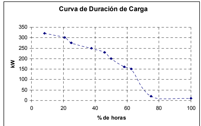
GRAFICA 20. CURVA DE DURACIÓN DE CARGA DE UN DÍA ORDINARIO DE ACTIVIDADES EN EL ALIMENTADOR "H"
