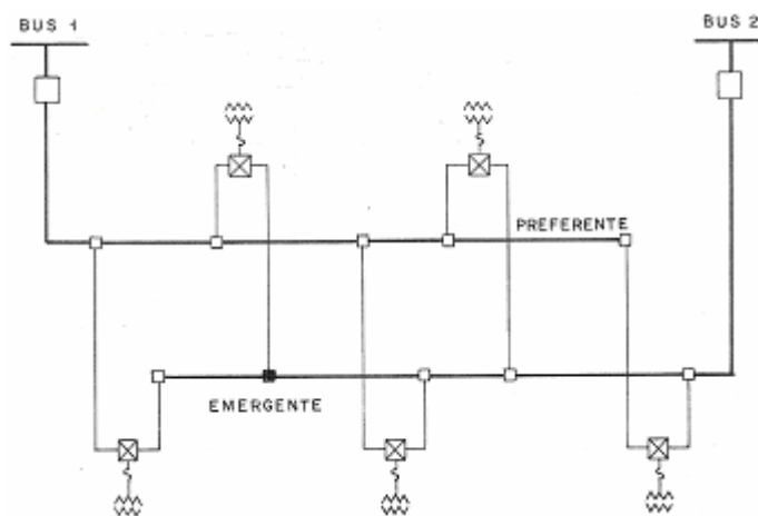
DIAGRAMA 9. ESTRUCTURA EN DOBLE DERIVACIÓN
