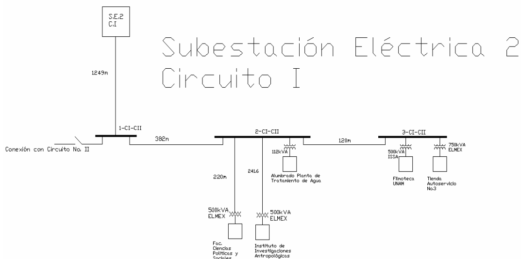
DIAGRAMA 31. DIAGRAMA UNIFILAR CIRCUITO "I"
