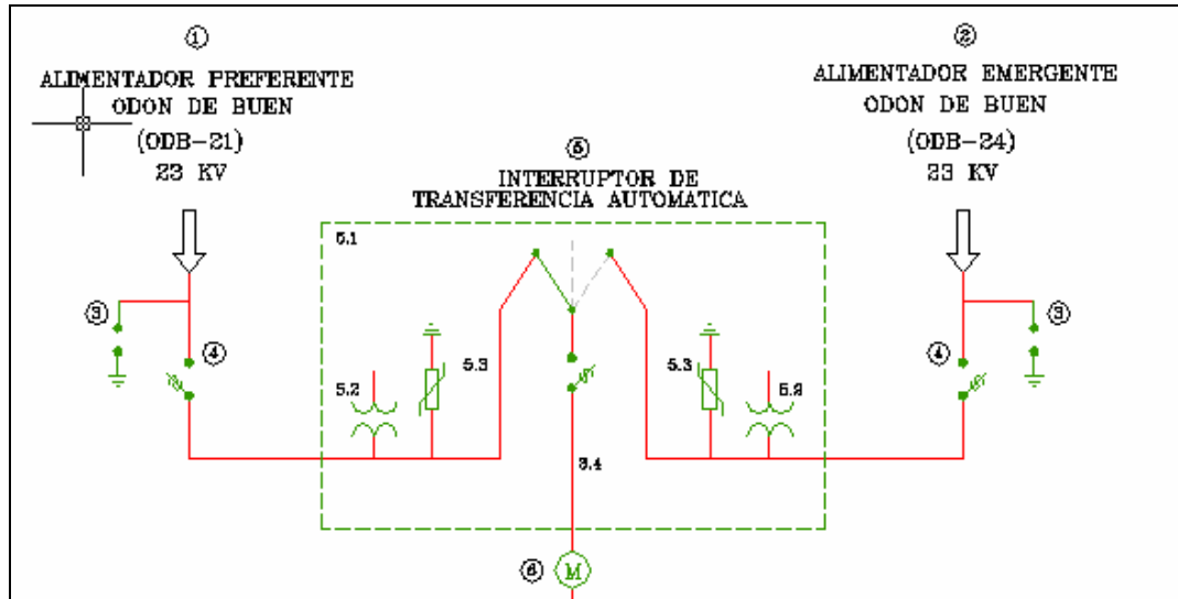
DIAGRAMA 13. ACOMETIDA DE LA SUBESTACIÓN GENERAL No. 1
