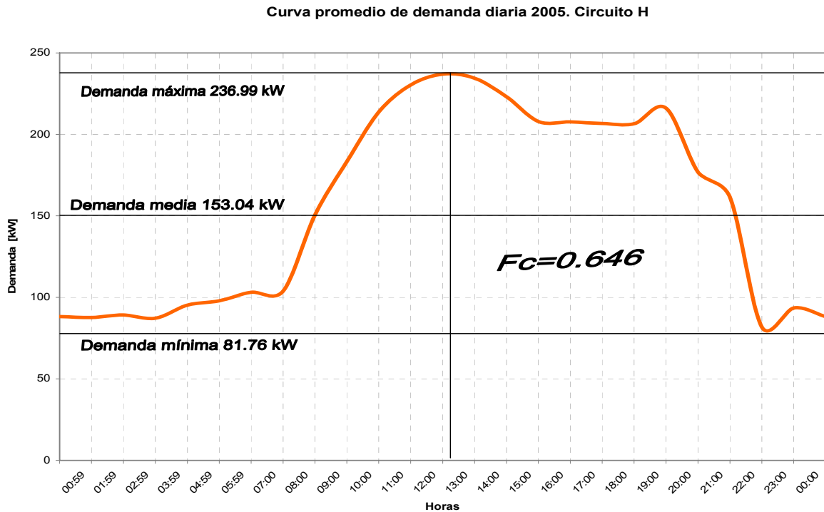
GRAFICA 23. CURVA DE DEMANDA PROMEDIO DIARIA ANUAL DEL ALIMENTADOR "H"
