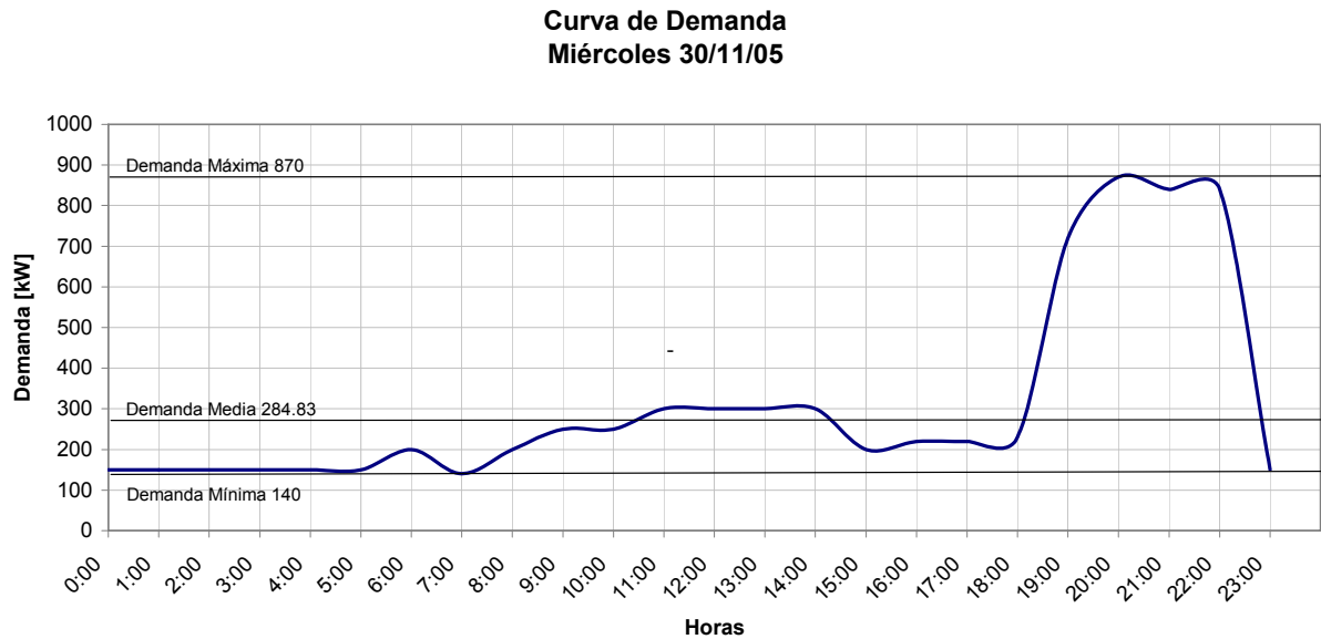
GRAFICA 3. CURVA DE DEMANDA DE UN DÍA EXTRAORDINARIO DE ACTIVIDADES DEL ALIMENTADOR "A"
