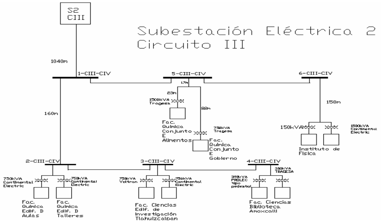
DIAGRAMA 33. DIAGRAMA UNIFILAR CIRCUITO "III".
