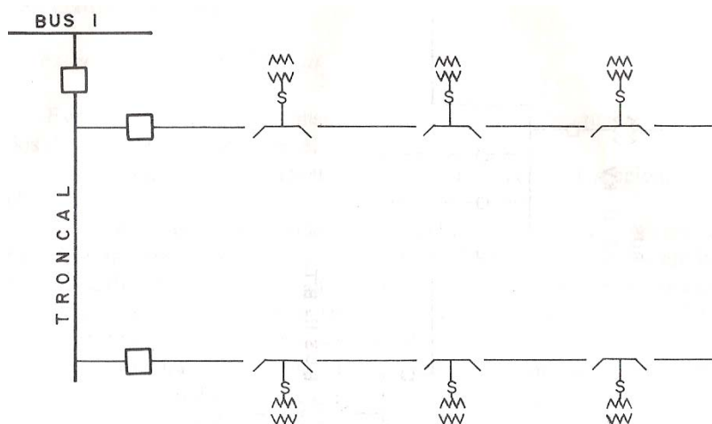
DIAGRAMA 6. RED EN ANILLO CON UNA SOLA FUENTE DE ALIMENTACIÓN
