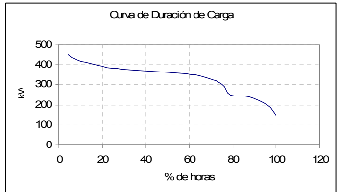
GRAFICA 12. CURVA DE DURACIÓN DE CARGA DE UN DÍA EXTRAORDINARIO DE ACTIVIDADES EN EL ALIMENTADOR "F"
