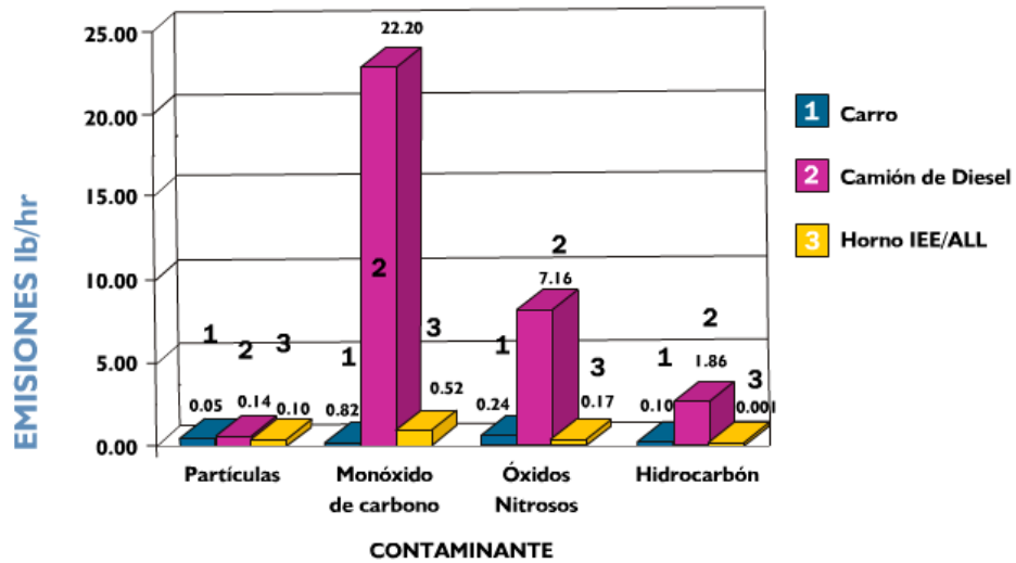
Gráfica. 1. Tabla comparativa de emisiones entre horno crematorio y camión diesel.
