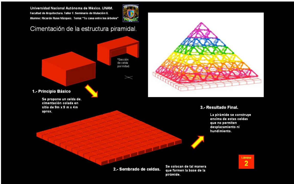
Figura 5. Concepto general de cimentación por conformación de terreno.
