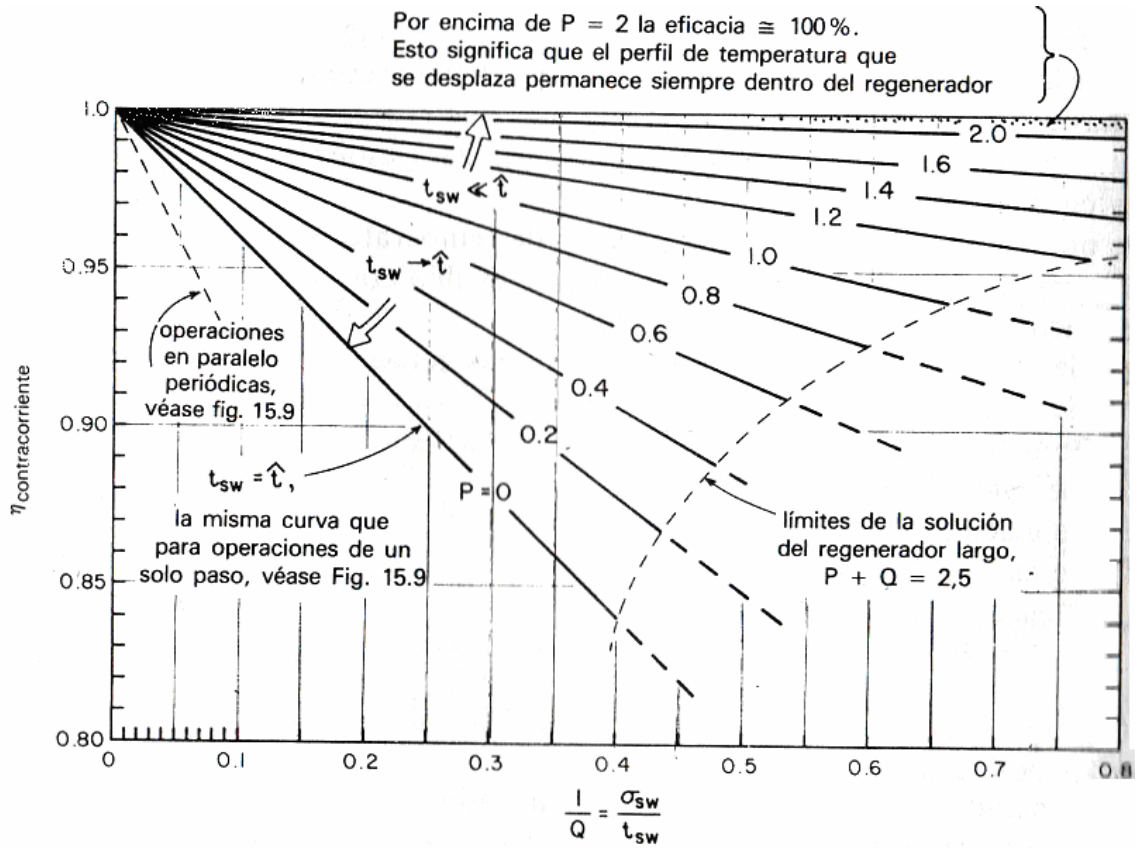
Diagrama de eficiencia de Mills.
