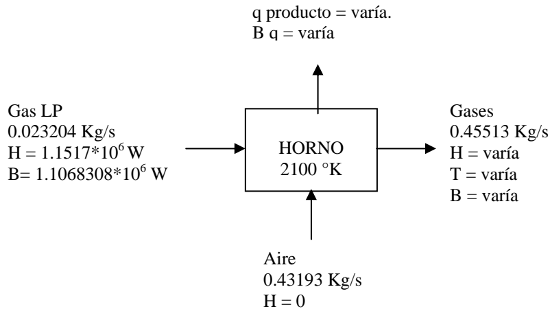
Figura 2.1 Diagrama de procesos originales.
