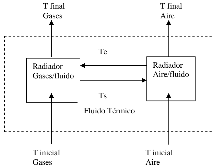
Figura 5.1 Diagrama de recuperador de doble radiador.
