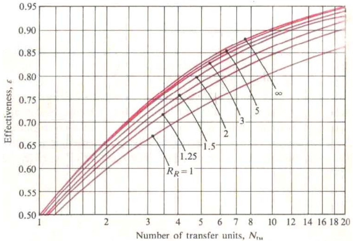
Diagrama de eficiencia de Mills.
