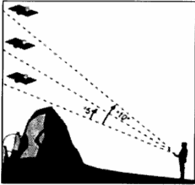
Fig. 1 Visibilidad sin obstáculos
