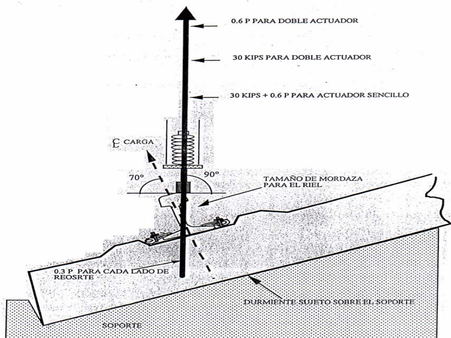
FIG. 6 PRUEBA DE CARGA REPETITIVA EN FIJACION DEL RIEL.
