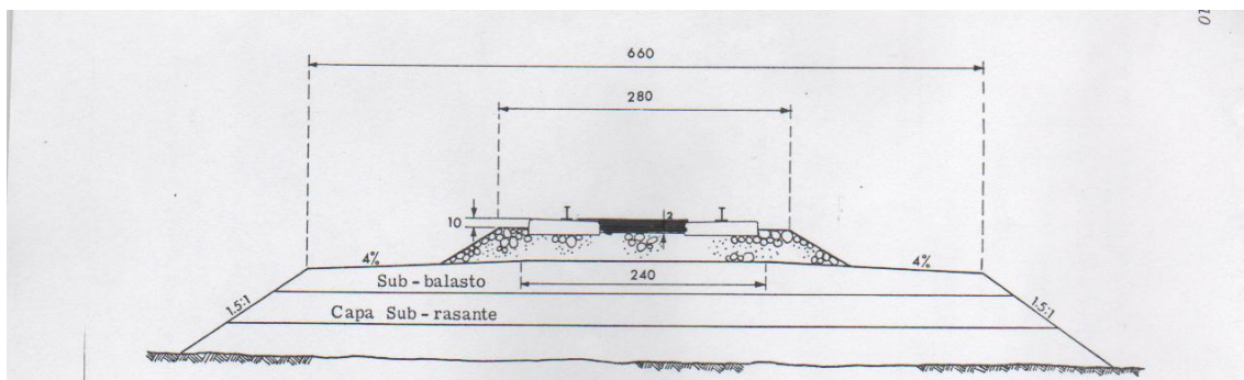
TERRAPLEN CON CAPAS DE SUB-BALASTO Y SUBRASANTE.
