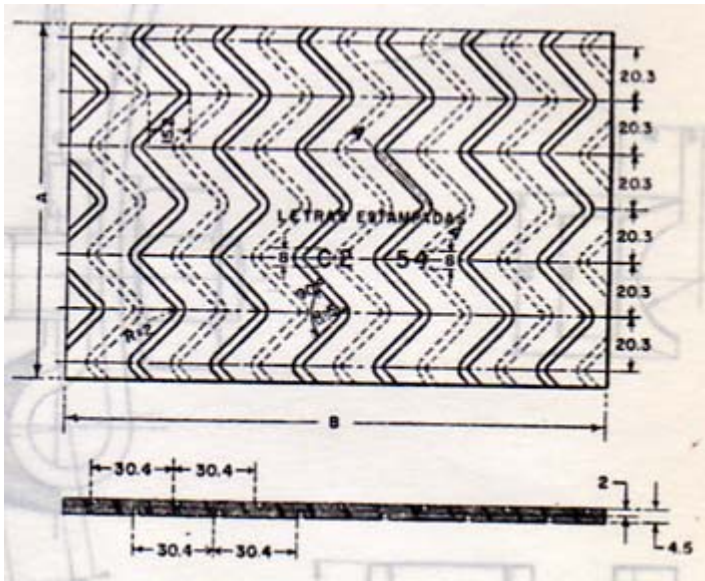
Placa de Hule Neopreno tipo Chevron
