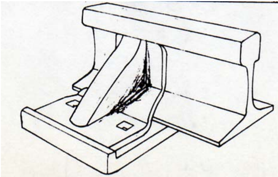
Silleta de Refuerzo.
