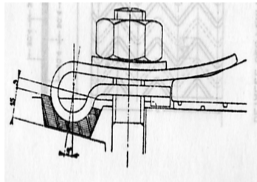
Cojinete amortiguador
