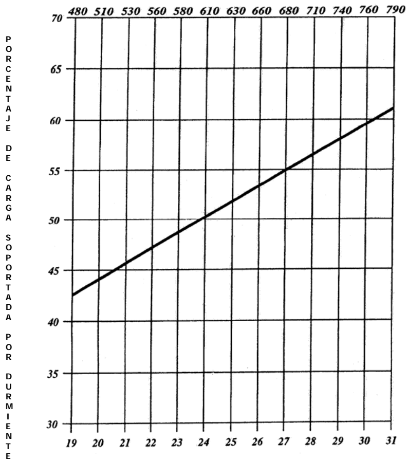
SEPARACION DE CENTRO A CENTRO DE DURMIENTE EN PULGADAS.
