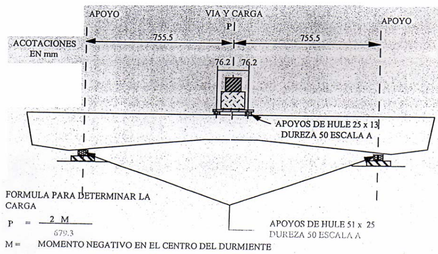
FIG.3 MOMENTO NEGATIVO EN EL CENTRO DEL DURMIENTE.
