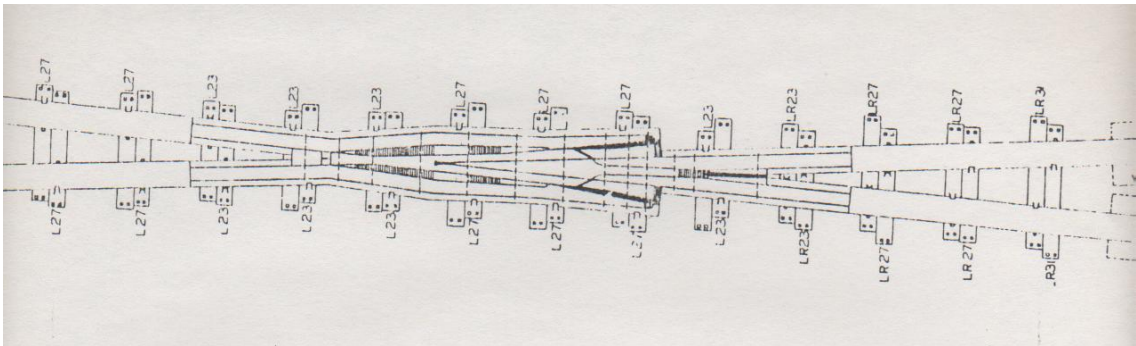
Sapo inserto corazón acero manganeso
