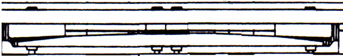
Contra riel de 11' o 13' de longitud
