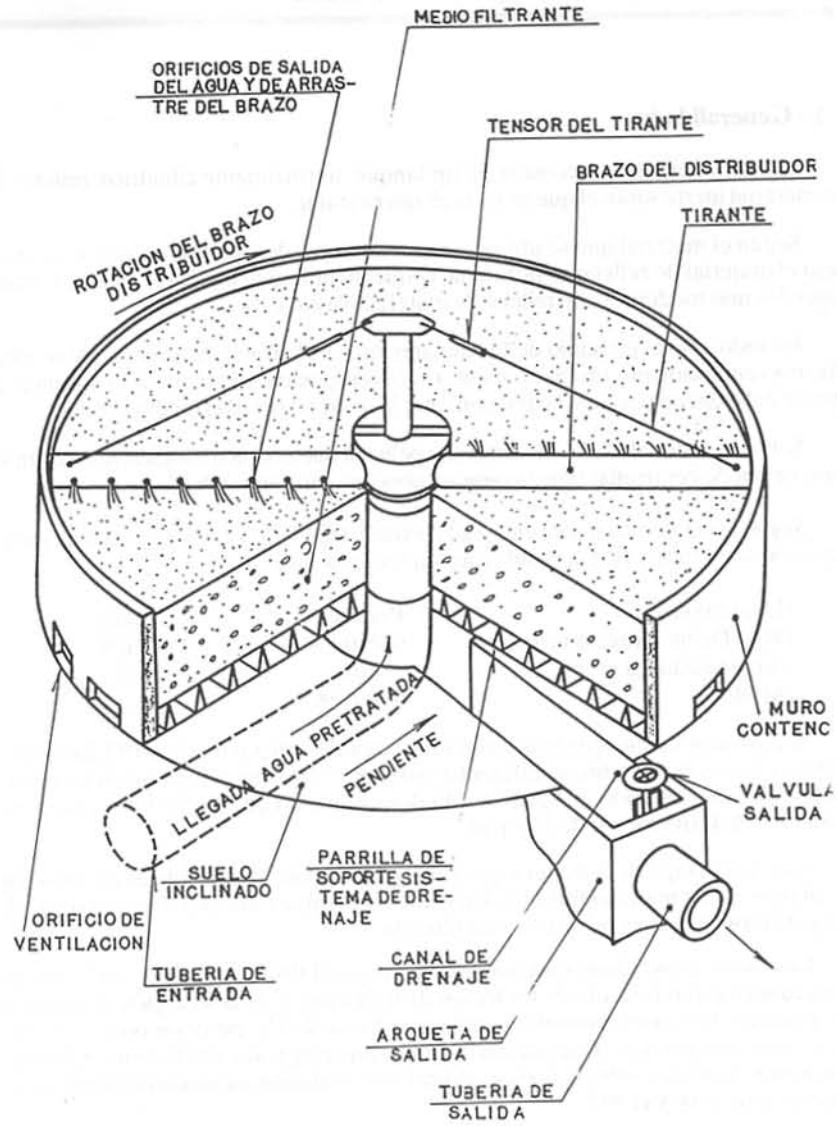
Fig. 1 Esquema general de un filtro percolador.
