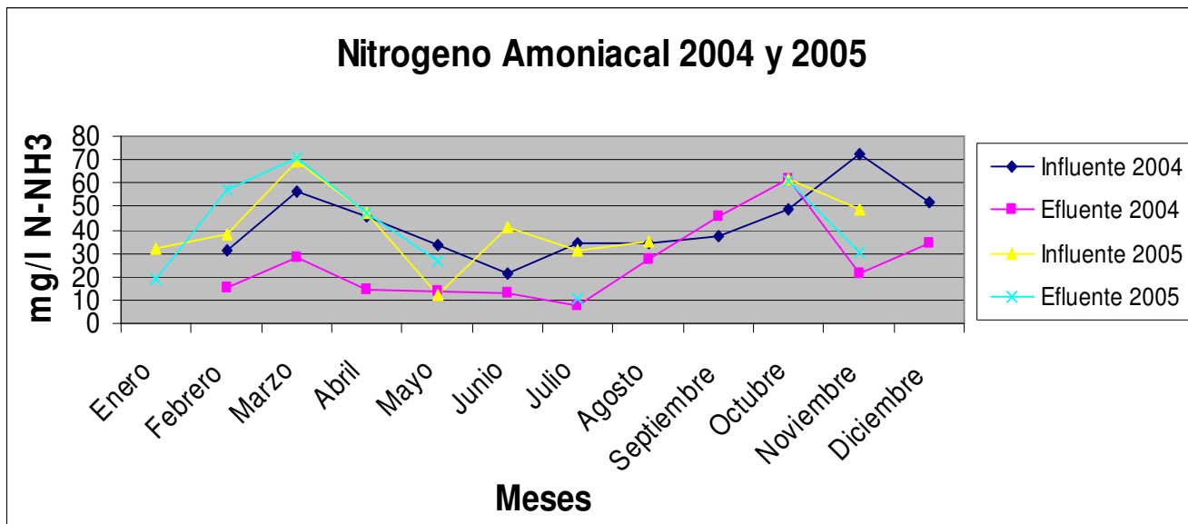
Figura 15. Comparación de los valores de nitrógeno amoniacal del influente y el efluente del 2004 y 2005.
