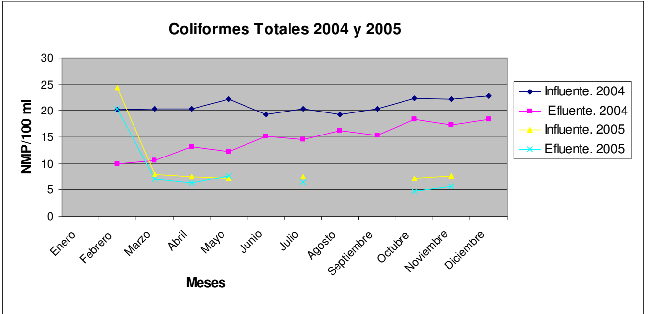
Figura 11. Comparación de los valores de coliformes totales del influente y el efluente del 2004 y 2005.
