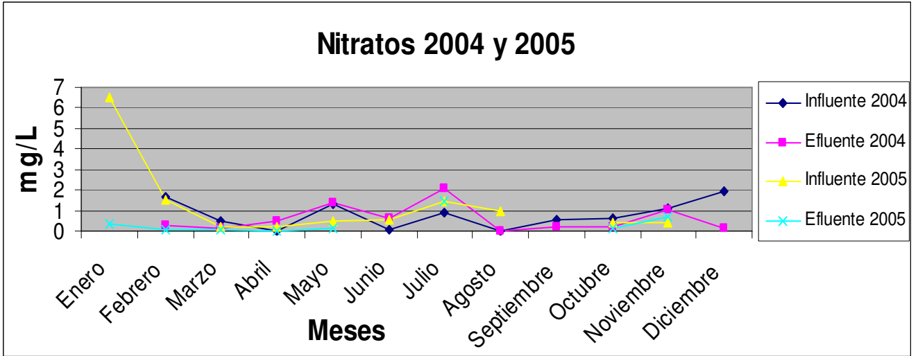
Figura 16. Comparación de los valores de nitratos del influente y el efluente del 2004 y 2005.
