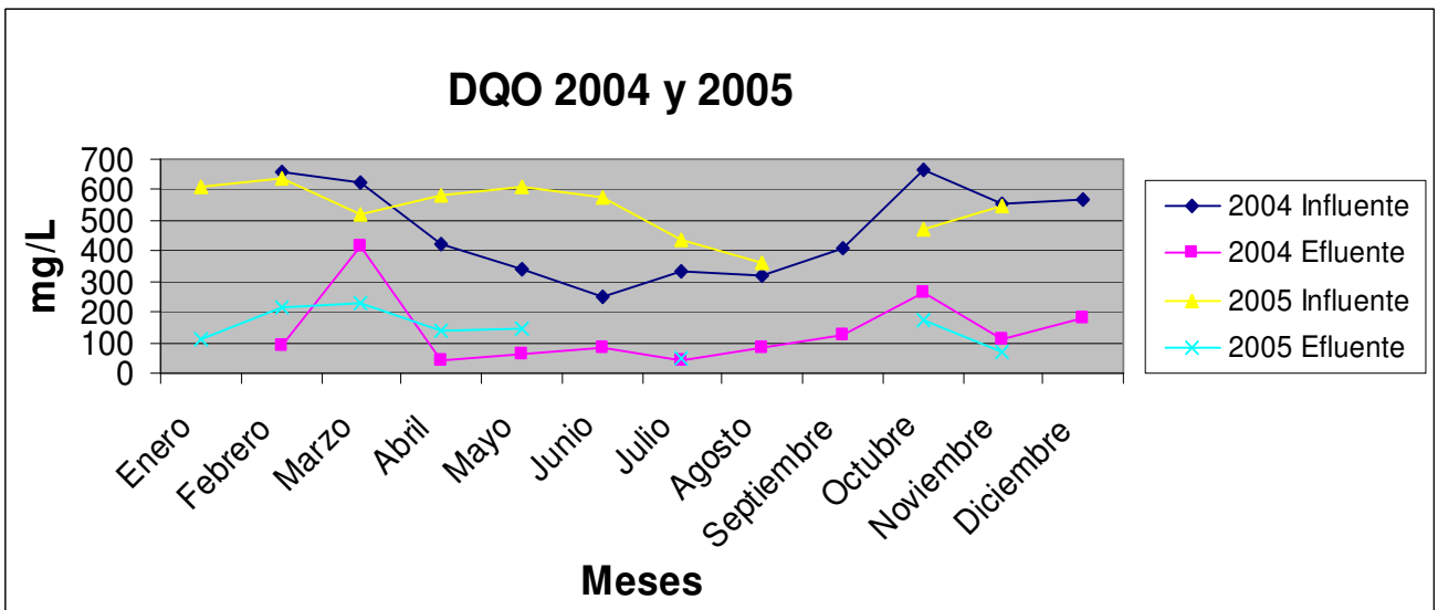
Figura 14. Comparación de los valores de DQO del influente y el efluente del 2004 y 2005.
