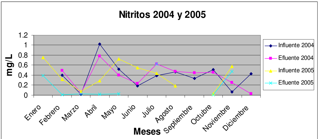
Figura 17. Comparación de los valores de nitritos del influente y el efluente del 2004 y 2005.
