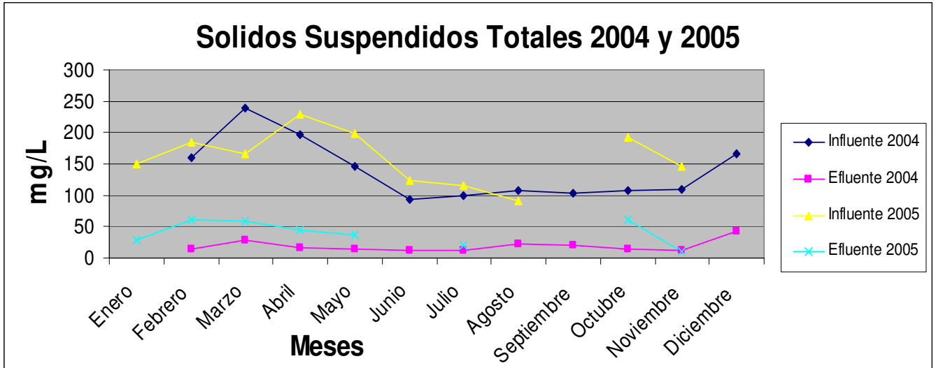
Figura 21. Comparación de los valores de sólidos suspendidos totales del influente y el efluente del 2004 y 2005.
