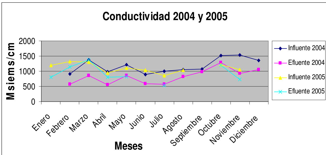
Figura 20. Comparación de los valores de conductividad del influente y el efluente del 2004 y 2005.
