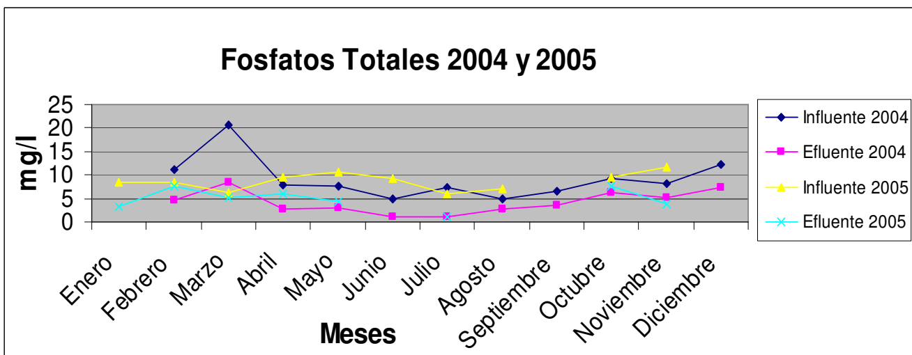
Figura 19. Comparación de los valores de fosfatos totales del influente y el efluente del 2004 y 2005.
