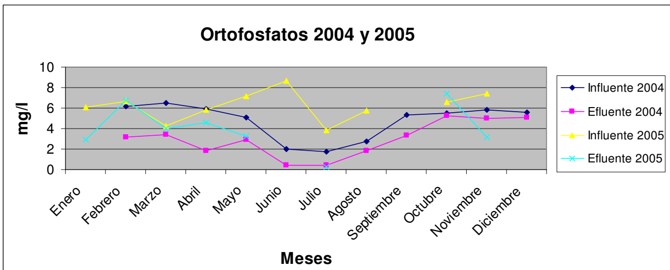
Figura 18. Comparación de los valores de ortofosfatos del influente y el efluente del 2004 y 2005.
