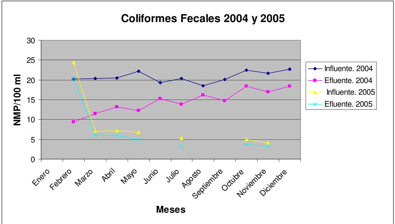
Figura 12. Comparación de los valores de coliformes fecales del influente y el efluente del 2004 y 2005.
