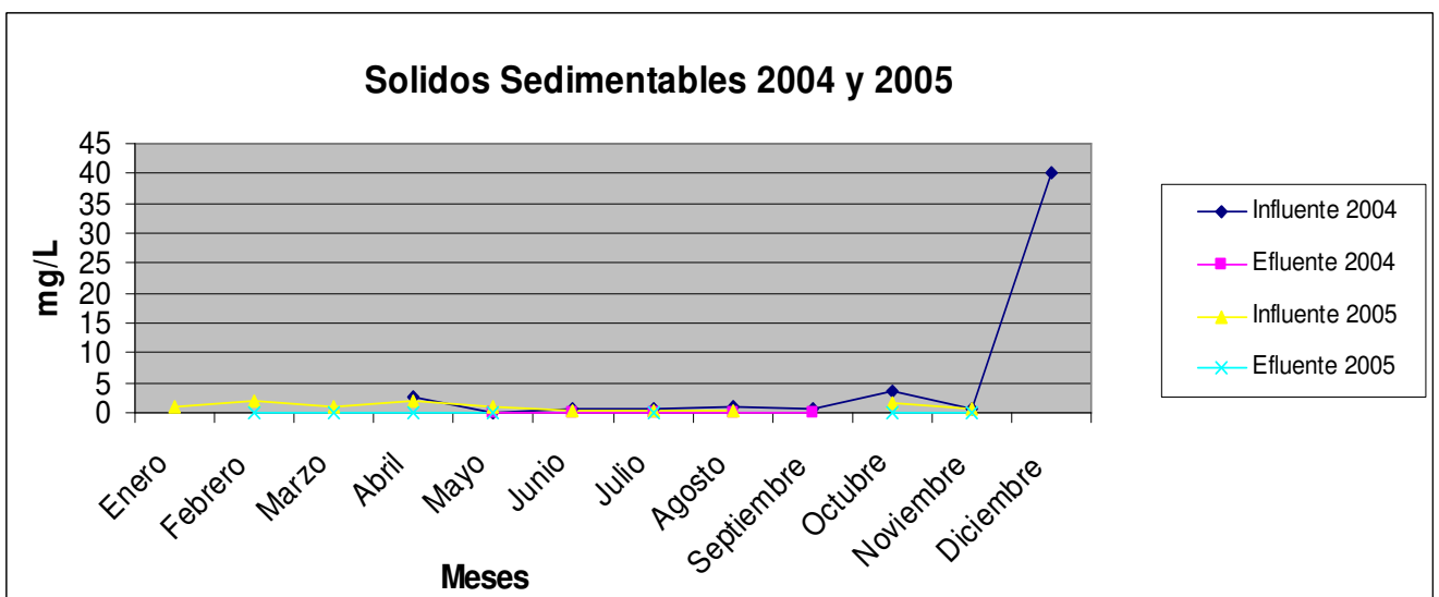
Figura 22. Comparación de los valores de sólidos sedimentables del influente y el efluente del 2004 y 2005.
