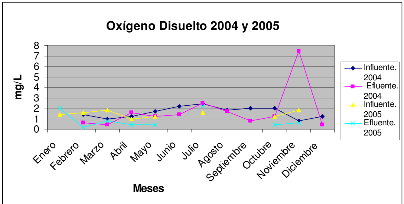
Figura 10. Comparación de los valores de oxígeno disuelto del influente y el efluente del 2004 y 2005.
