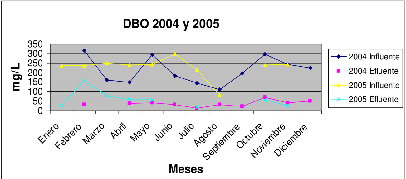
Figura 13. Comparación de los valores de DBO 5 del influente y el efluente del 2004 y 2005.
