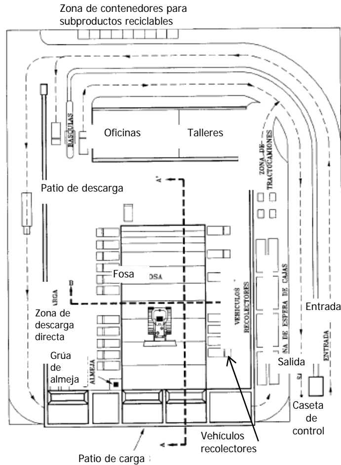
Figura 2.3 Planta de conjunto tipo de estaciones de transferencia con descarga indirecta.
