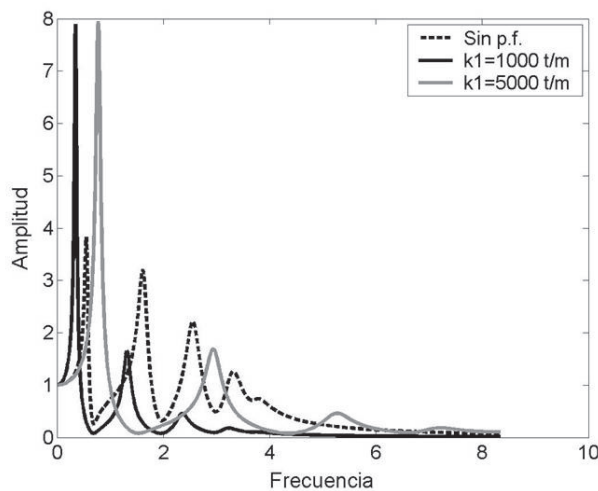
Figura 1.2 Funciones de transferencia del primer entrepiso de estructuras con y sin piso flexible.
