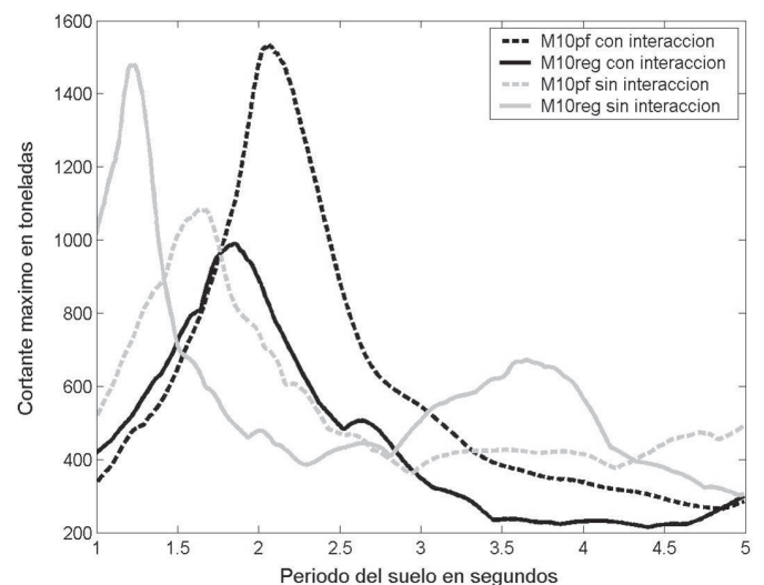
Figura 4.15. Variación del cortante basal máximo.
