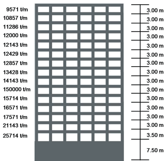
Figura 4.6. Fachada frontal del edificio base para el modelo M15reg.
