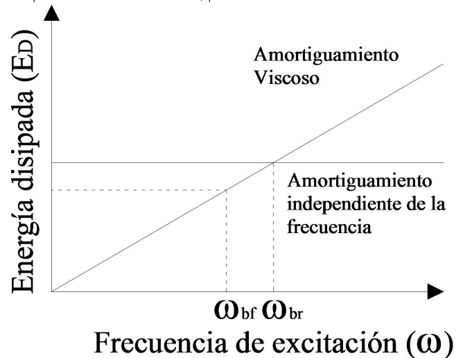
Figura 3.5. Diferencia entre el amortiguamiento con y sin ISE.
