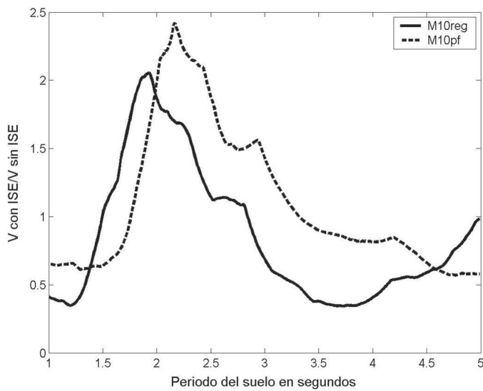
Figura 4.19. Cocientes entre los cortantes basales máximos con y sin efectos ISE de los modelos M10reg y M10pf.
