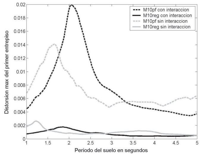
Figura 4.20. Variación de las distorsiones máximas del primer entrepiso.
