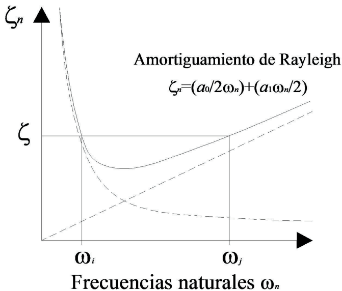
Figura 3.3. Amortiguamiento de Rayleigh
