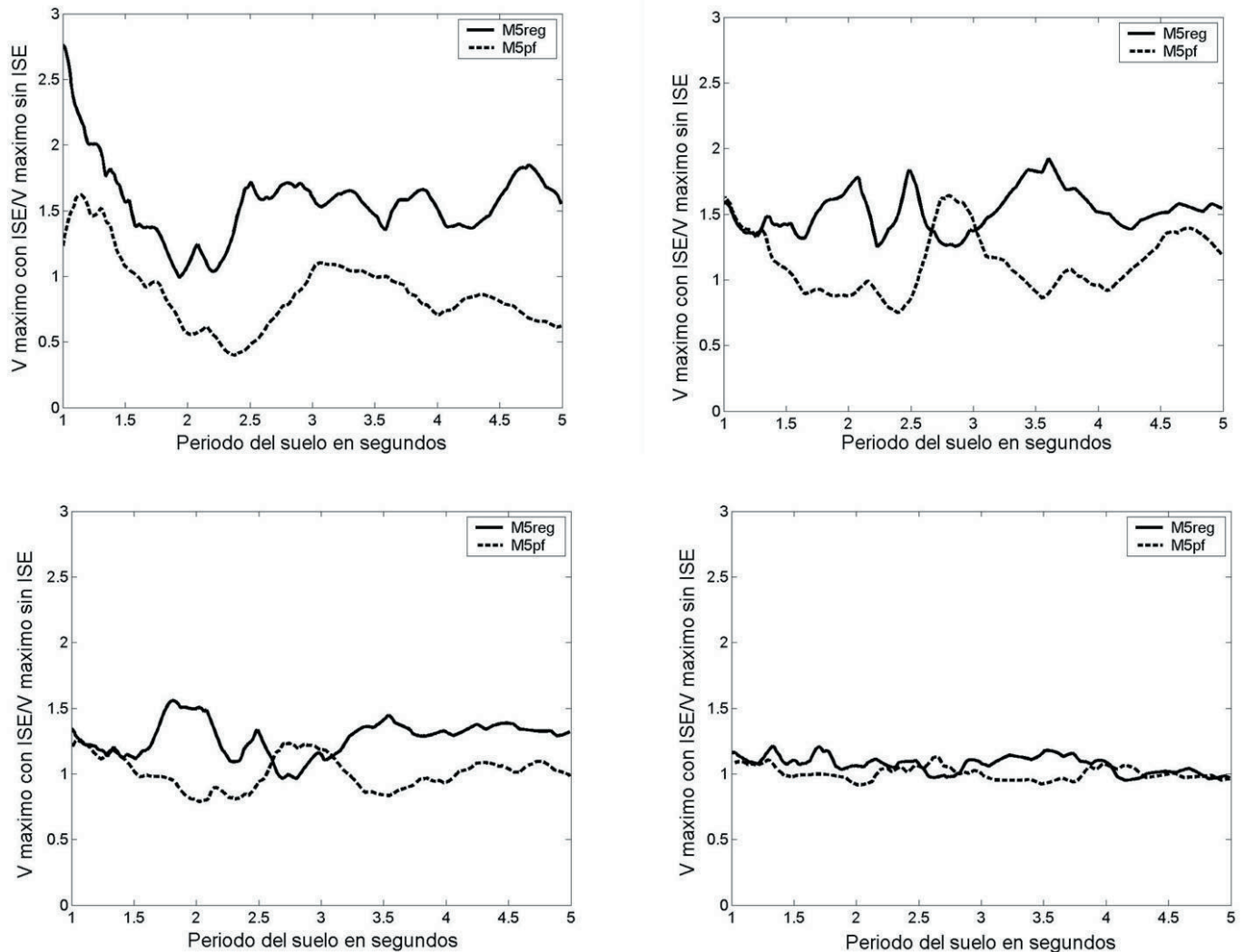
Figura 4.23. Diferentes condiciones de apoyo. ( \beta_s = 50, 75, 100 y 150 m/s)
