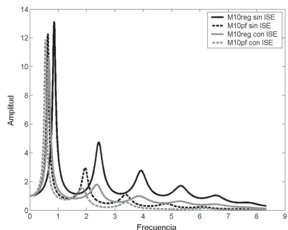
Figura 4.7. Funciones de transferencia de azotea de los modelos M10reg y M10pf con y sin ISE.
