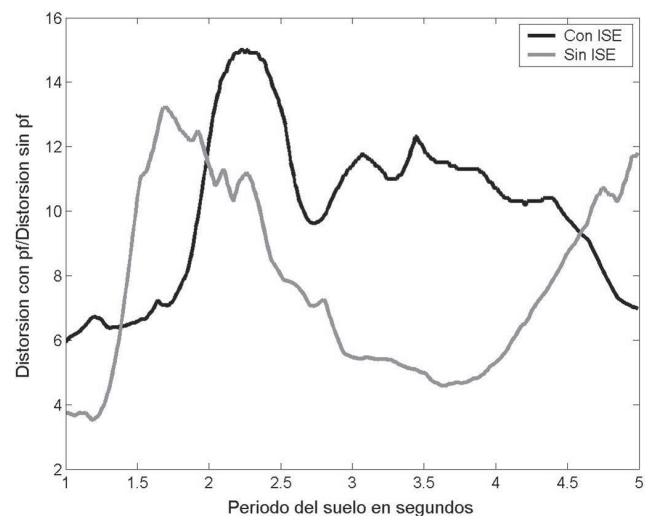
Figura 4.21. Cocientes entre las distorsiones máximas del primer entrepiso de los modelos M10pf y M10reg, con y sin efectos ISE.
