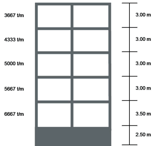
Figura 4.2. Fachada frontal del edificio base para el modelo M5reg.
