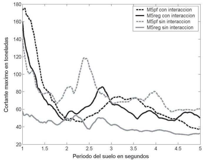
Figura 4.17. Variación de los cortantes basales máximos.
