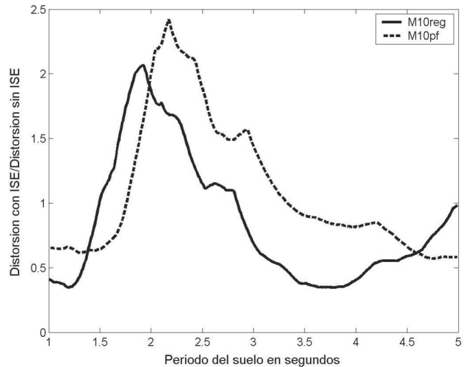
Figura 4.22. Cocientes entre las distorsiones máximas del primer entrepiso con y sin efectos ISE de los modelos M10reg y M10pf.
