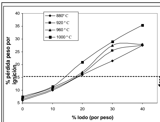
Fig. 2.3. % de pérdida por ignición de los ladrillos (Weng C. H., et al., 2003).
