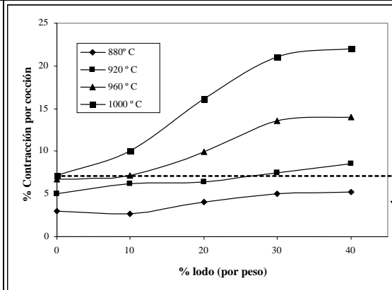
Fig. 2.2. % de contracción por secado de los ladrillos (Weng C. H., et al., 2003).
