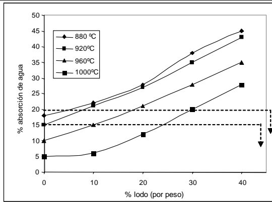
Fig. 2.1. % de absorción de agua de los ladrillos (Weng C. H., et al., 2003).
