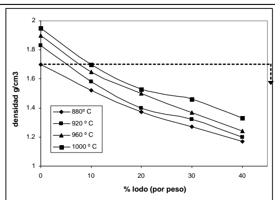
Fig. 2.4 Densidad de los ladrillos (Weng C. H., et al., 2003).
