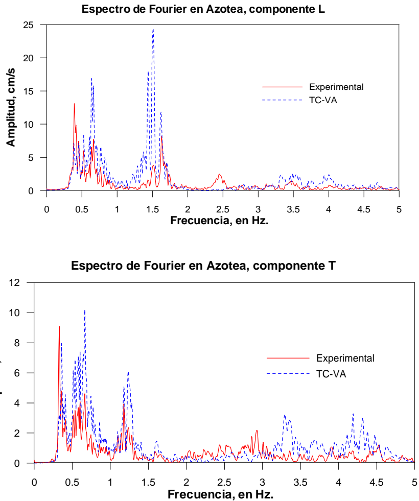
Figura 4.6 Comparación de espectros de Fourier, analítico y experimental de los componentes horizontales L y T
