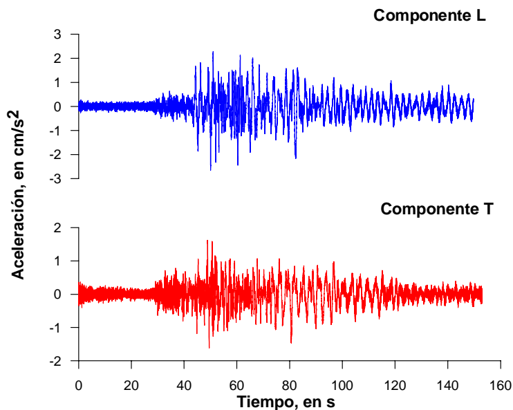
Figura 3.10 Aceleraciones experimentales de azotea registradas durante el evento sísmico TT04-3 en los componentes L y T
