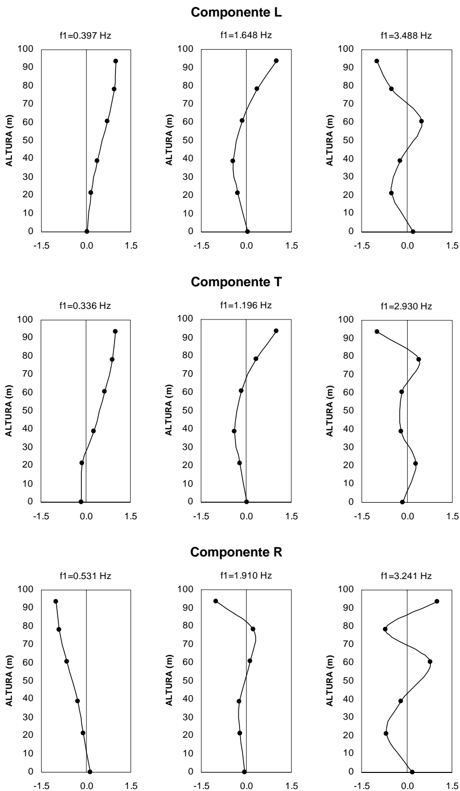
Figura 3.6 Formas modales con apéndice durante el evento sísmico TT04-3
