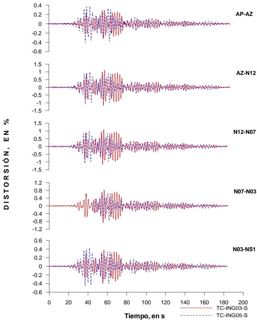
Figura 4.21 Historia de distorsiones en el componente L de modelos ingenieriles para sismo al ser sometidos a las excitaciones del sismo de septiembre de 1985
