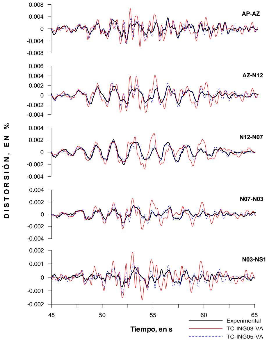
Figura 4.20 Historia de distorsiones en el componente T durante la fase intensa del evento sísmico TT04-3, modelos ingenieriles para vibración ambiental
