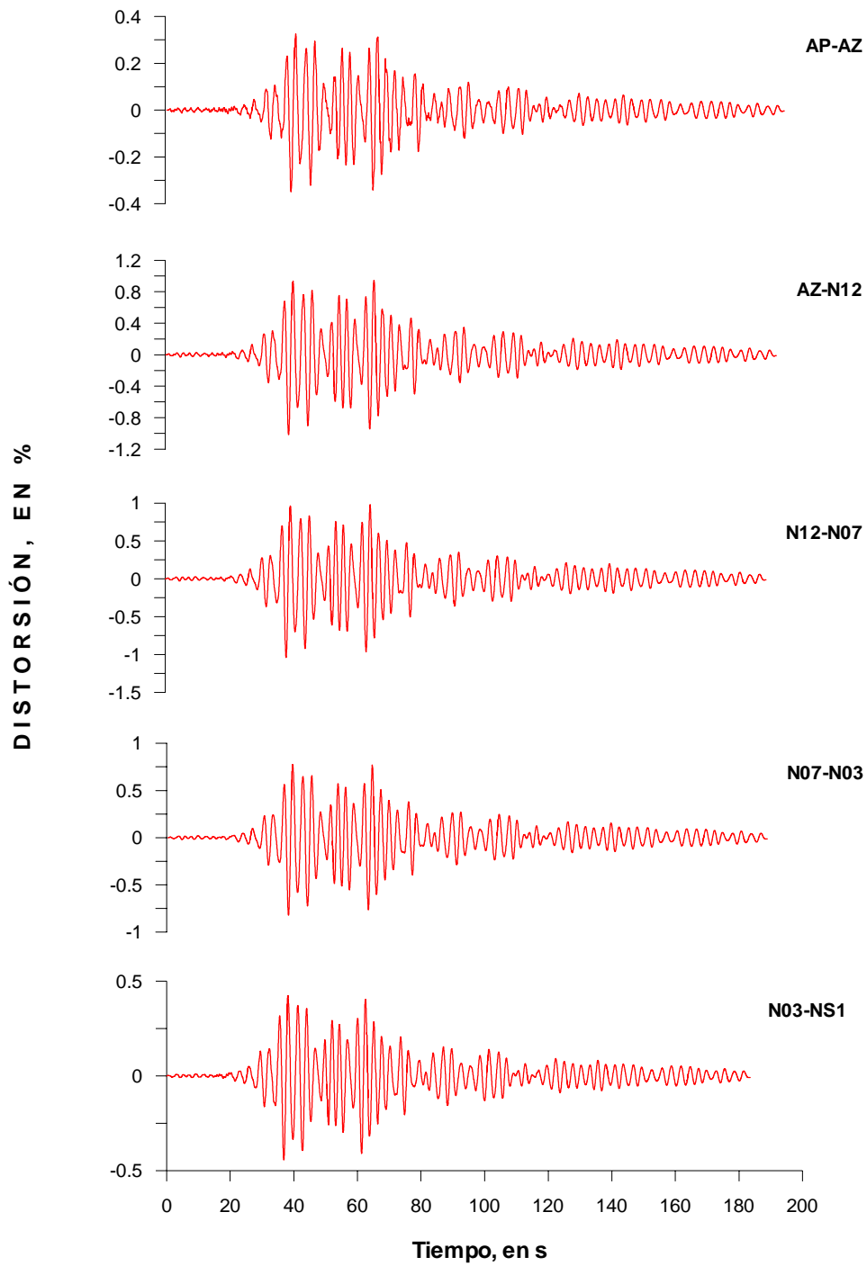
Figura 4.14 Historia de distorsiones en el componente L del modelo TC-S2, al ser sometido a las excitaciones del sismo de septiembre de 1985 ocurrido en la ciudad de México
