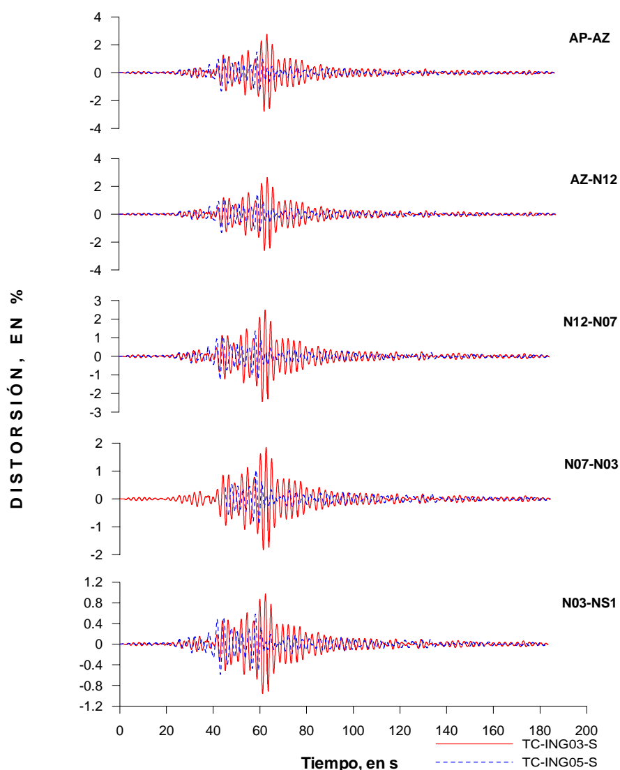
Figura 4.22 Historia de distorsiones en el componente T de modelos ingenieriles para sismo al ser sometidos a las excitaciones del sismo de septiembre de 1985
