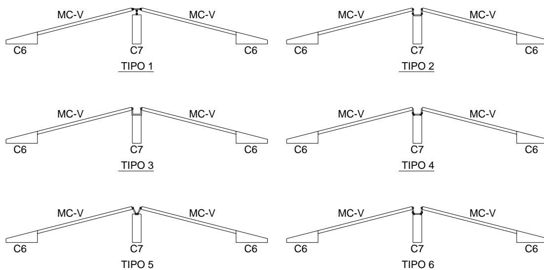
Figura C.1 Propuestas de desacoplamiento
