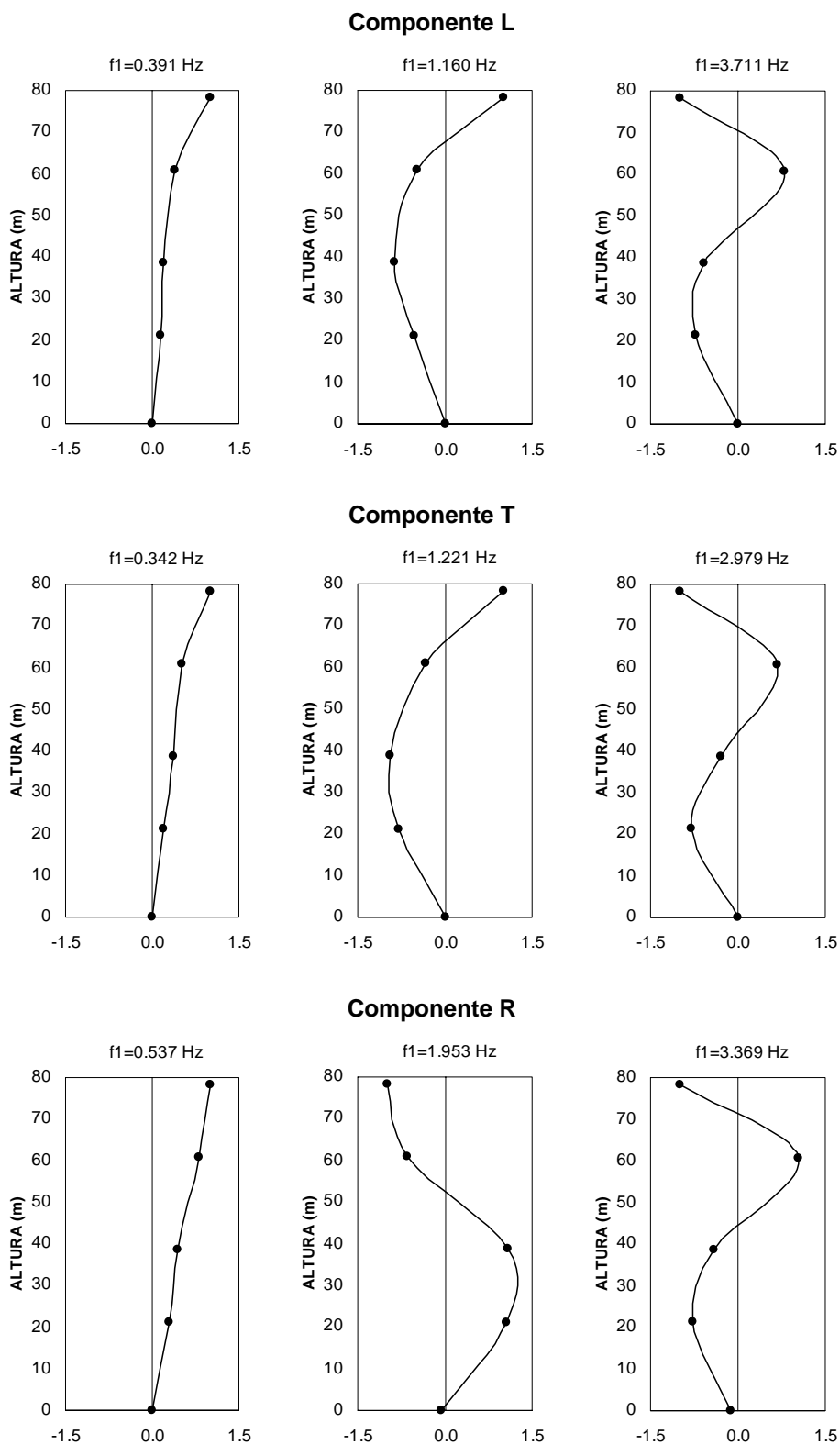
Figura 3.5 Formas modales sin apéndice para condiciones de vibración ambiental
