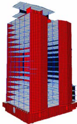
Figura 4.1 Modelo TC-VA calibrado para las condiciones de VA
