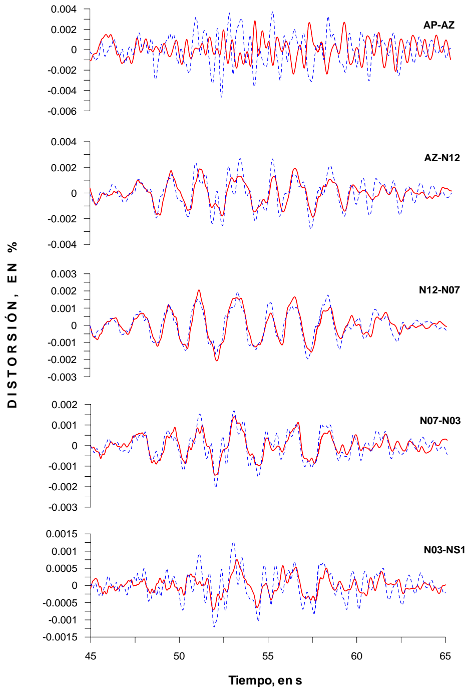
Figura 4.9 Historia de distorsiones experimental (línea continua) y analítica (línea discontinua) en el componente T durante la fase intensa del evento sísmico TT04-3, entre los niveles instrumentados
