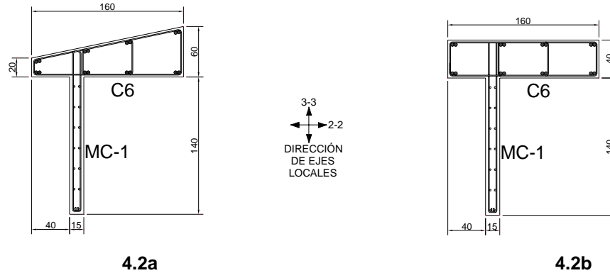
Figura 4.2 Sección y armado de acero transversal del conjunto MC-1 y C6
