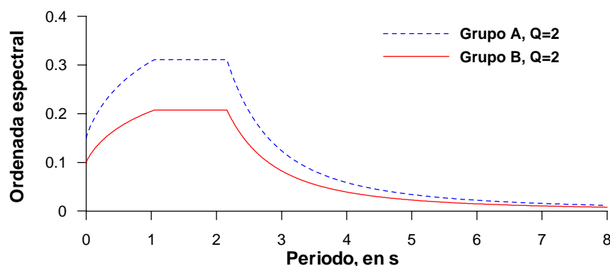
Figura 4.18 Espectro de aceleraciones de diseño del edificio, apéndice A de NTC-sismo, 2004
