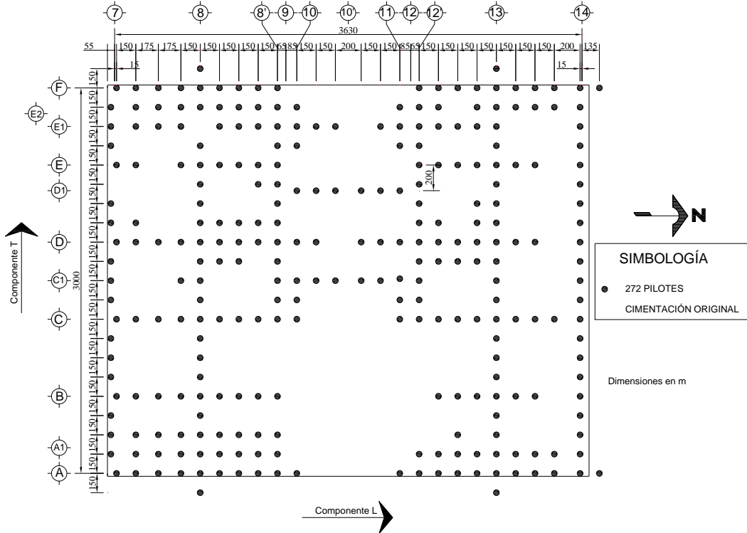
Figura 2.2 Planta Losa de Cimentación (CIM)
