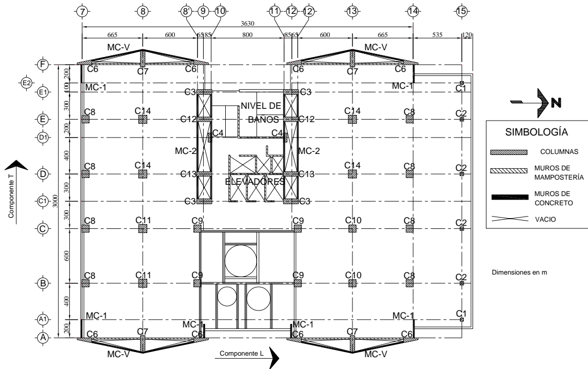
Figura 2.6 Planta nivel N3
