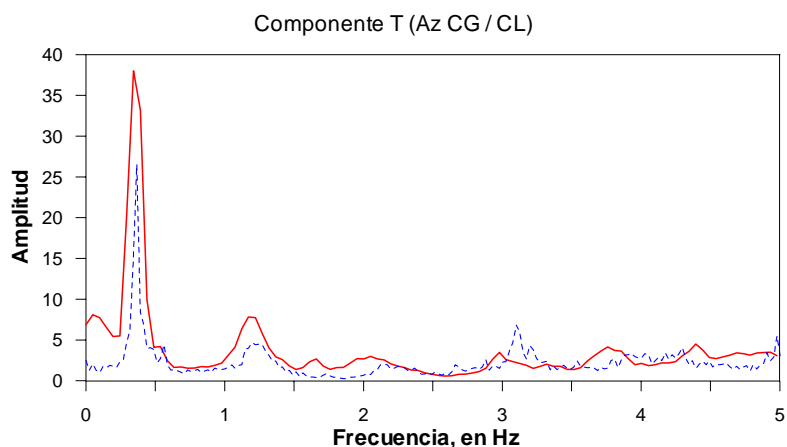
Figura 3.2 Función de transferencia entre azotea centro geométrico y terreno en componente T, para las vibraciones ambientales VA01 (línea continua) y VA03 (línea discontinua)
