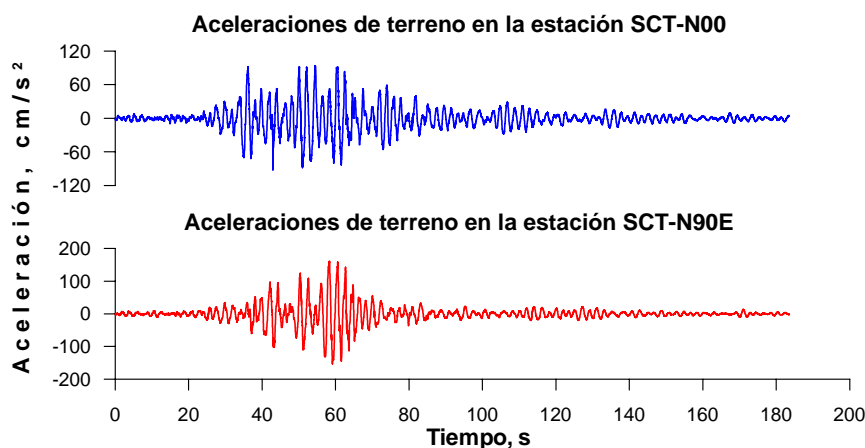
Figura 4.13 Aceleraciones de terreno en la estación de SCT, debidas al sismo ocurrido en la ciudad de México el 19 de septiembre de 1985
