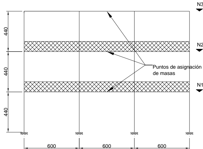
Figura B.5 Dimensiones de marco plano
