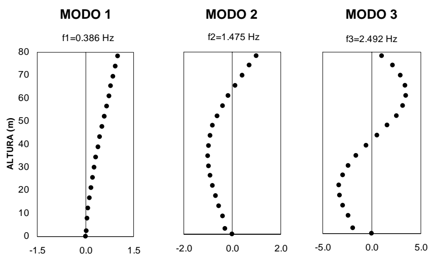
Figura 4.3 Formas modales analíticas del componente L
