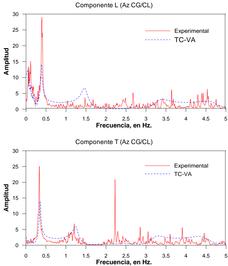
Figura 4.7 Funciones de transferencia entre Azotea y Terreno, analítica y experimental de los componentes horizontales L y T
