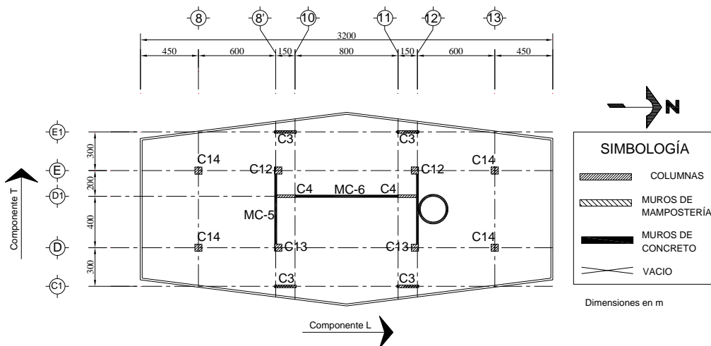
Figura 2.11 Planta nivel N18
