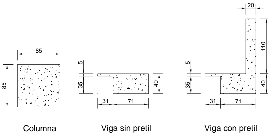
Figura B.6 Dimensiones de elementos estructurales definidos en el modelo de marco plano
