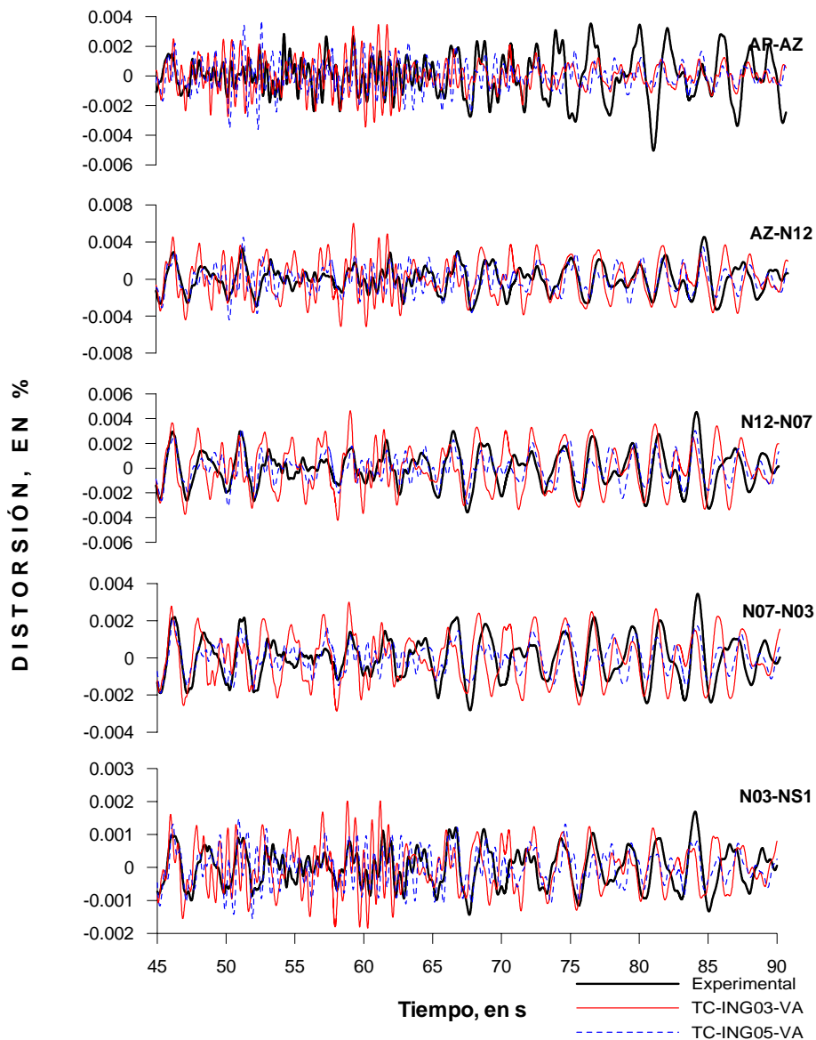
Figura 4.19 Historia de distorsiones en el componente L durante la fase intensa del evento sísmico TT04-3, modelos ingenieriles para vibración ambiental
