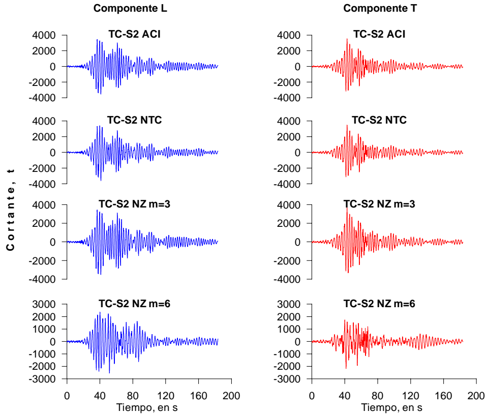
Figura 4.16 Cortante basal en los componentes L y T de los modelos TC-S2 con ZR de 50 por ciento
