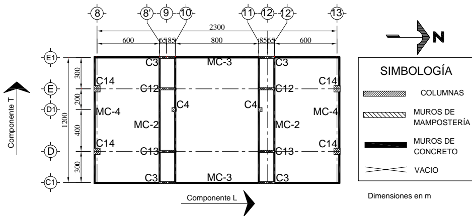
Figura 2.9 Planta nivel N16'
