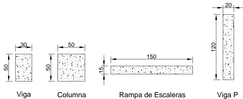
Figura B.3 Dimensiones de elementos estructurales
