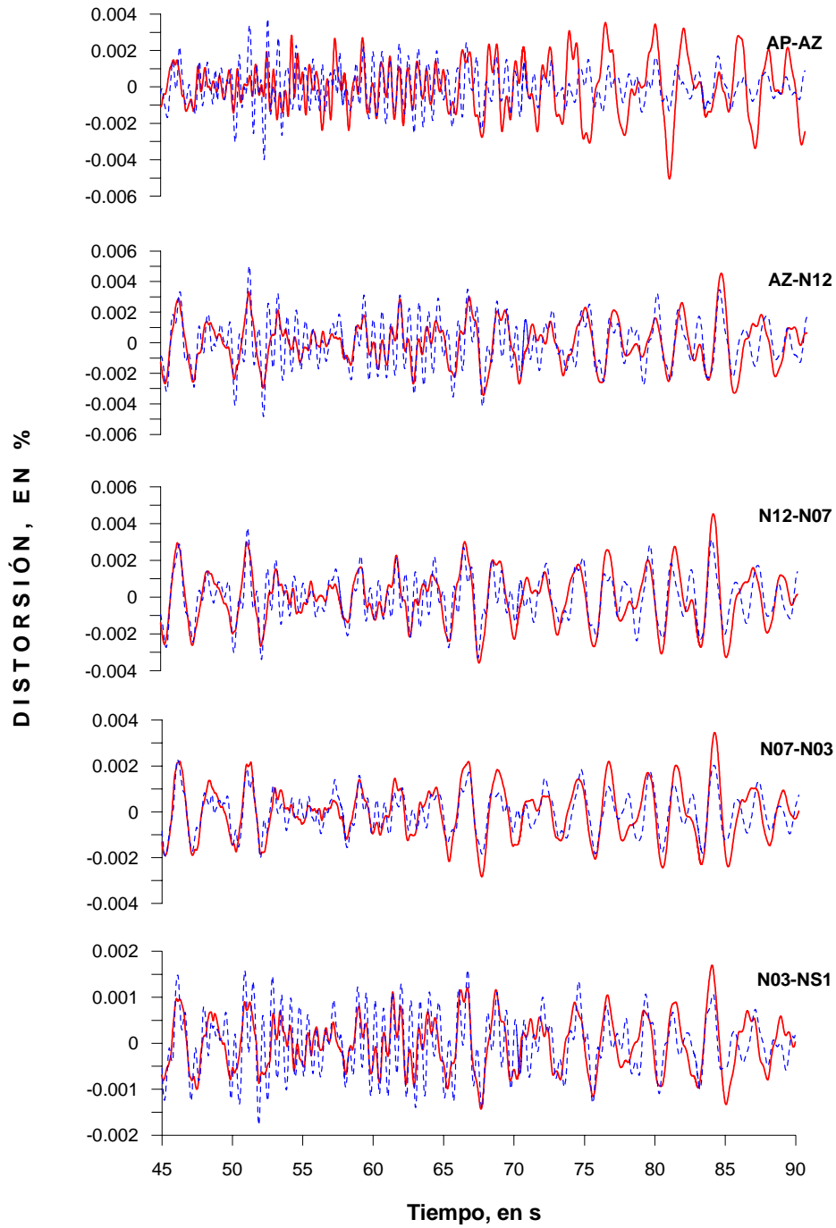
Figura 4.8 Historia de distorsiones experimental (línea continua) y analítica (línea discontinua) en el componente L durante la fase intensa del evento sísmico TT04-3, entre los niveles instrumentados
