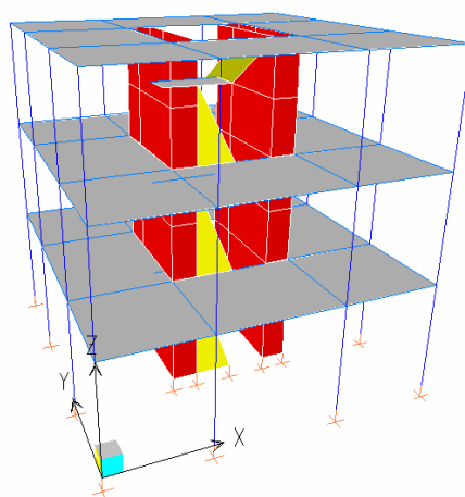
Figura B.4 Vista de modelo tridimensional elaborado en Etabs
