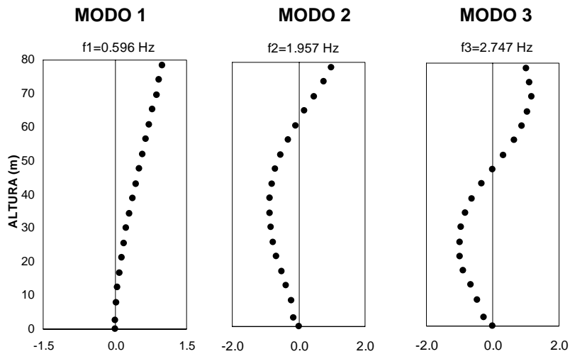
Figura 4.5 Formas modales analíticas del componente R
