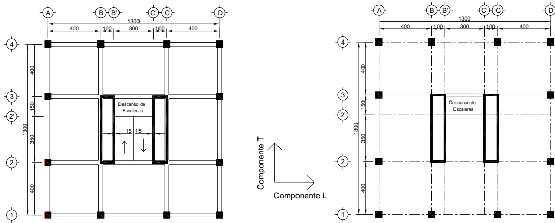
Figura B.2 Planta tipo y nivel de descanso de escaleras en los modelos.
