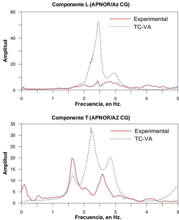
Figura 4.10 Funciones de transferencia entre apéndice y azotea (N18NN/Az CG), experimental y analítica de los componentes L y T
