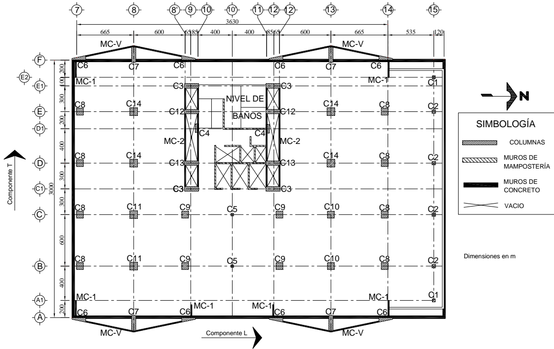
Figura 2.4 Planta Baja (PB)
