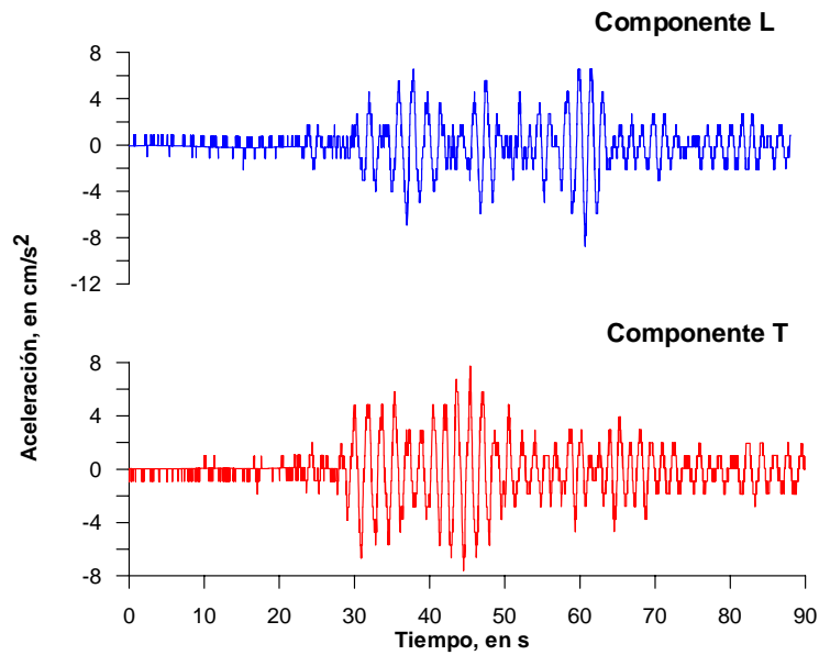
Figura 3.7 Aceleraciones experimentales de terreno registradas durante el evento sísmico TT04-1 en los componentes L y T
