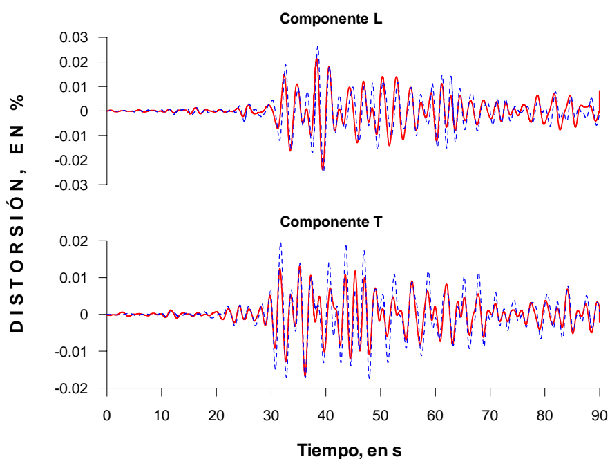
Figura 4.12 Historias de distorsiones de entrepiso experimental (línea continua) y analítica (línea discontinua) durante el evento sísmico TT04-1, entre azotea y nivel de sótano
