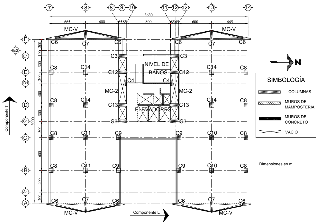
Figura 2.7 Planta tipo (N4-N15)
