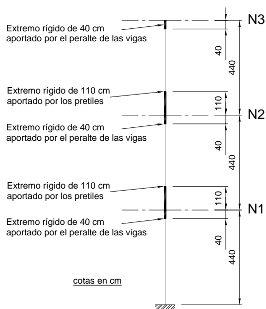
Figura B.7 Esquema para determinar la altura efectiva de las columnas en el modelo 04
