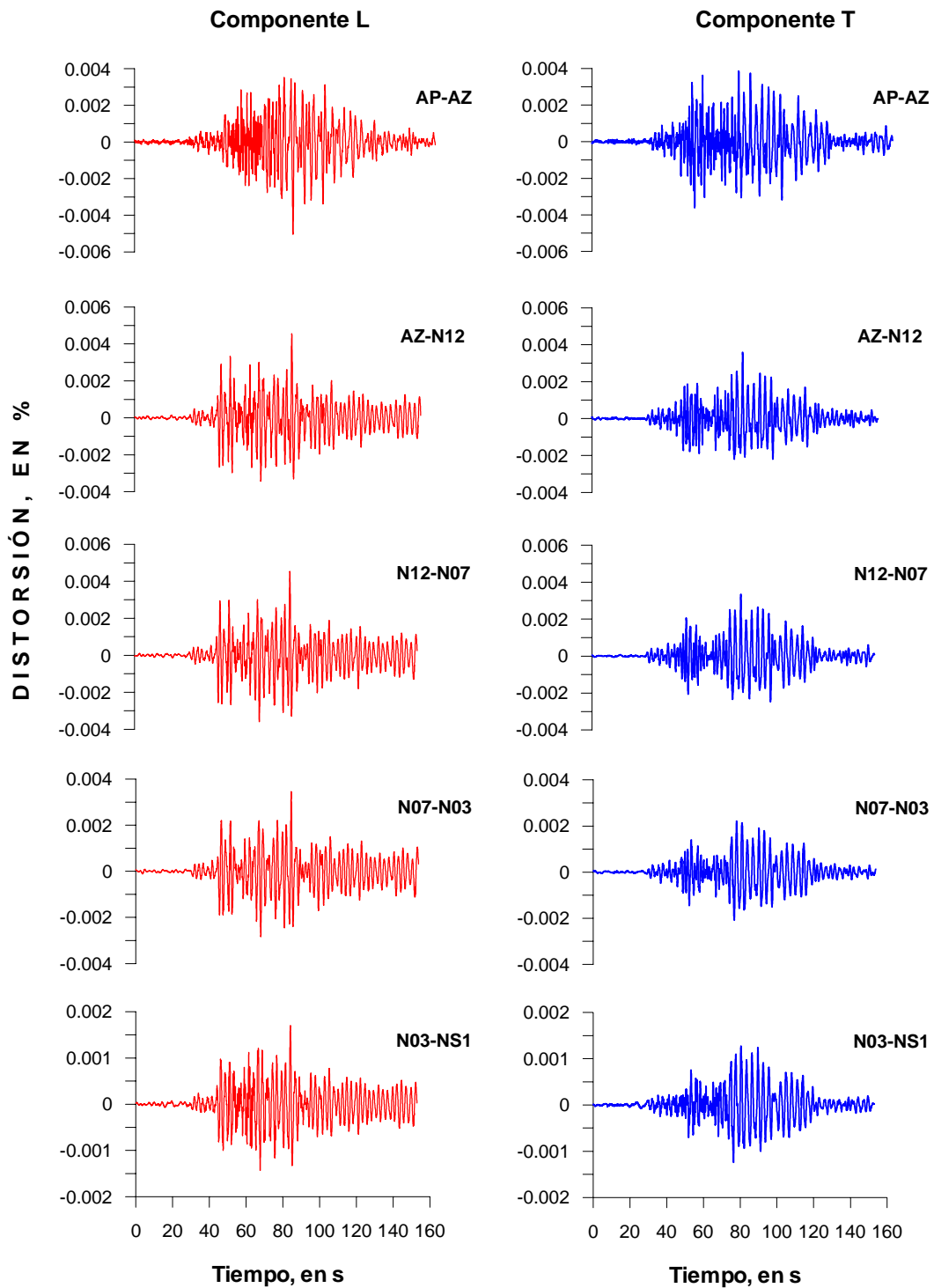
Figura 3.12 Historia de distorsiones de entrepiso durante el evento sísmico TT04-3
