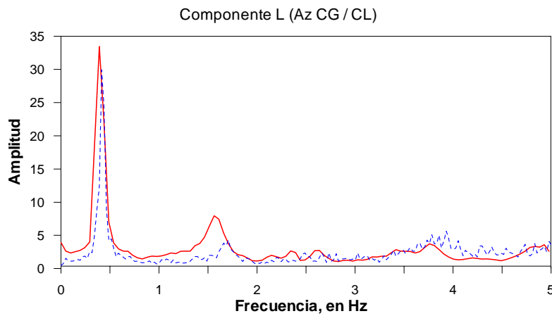
Figura 3.1 Función de transferencia entre azotea centro geométrico y terreno en componente L, para las vibraciones ambientales VA04-1 (línea continua) y VA04-3 (línea discontinua)
