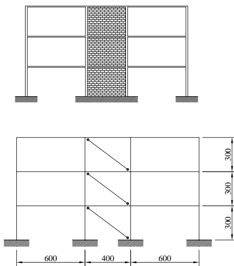
Figura B.1 Modelo de marco plano para el análisis de propuestas para el modelado de muros de mampostería por medio de diagonales equivalentes.
