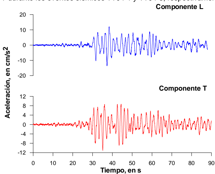
Figura 3.9 Aceleraciones experimentales de azotea registradas durante el evento sísmico TT04-1 en los componentes L y T
