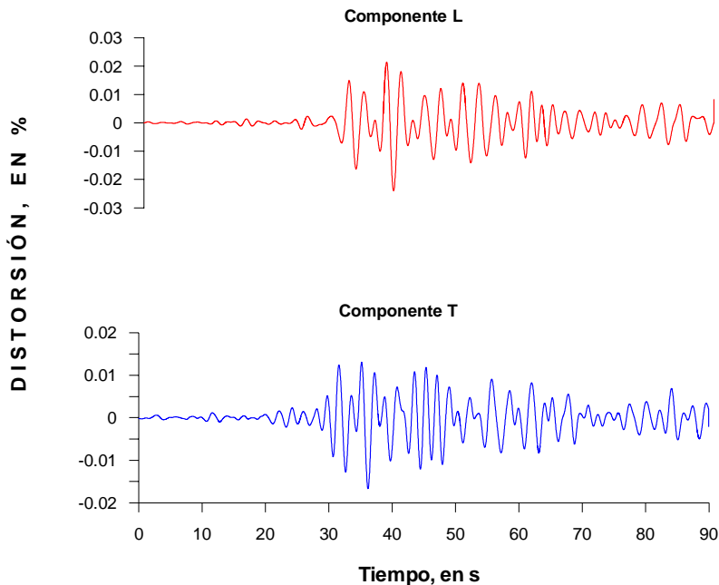
Figura 3.11 Historia de distorsiones experimentales entre azotea (AZ) y sótano (NS1) durante el evento sísmico TT04-1
