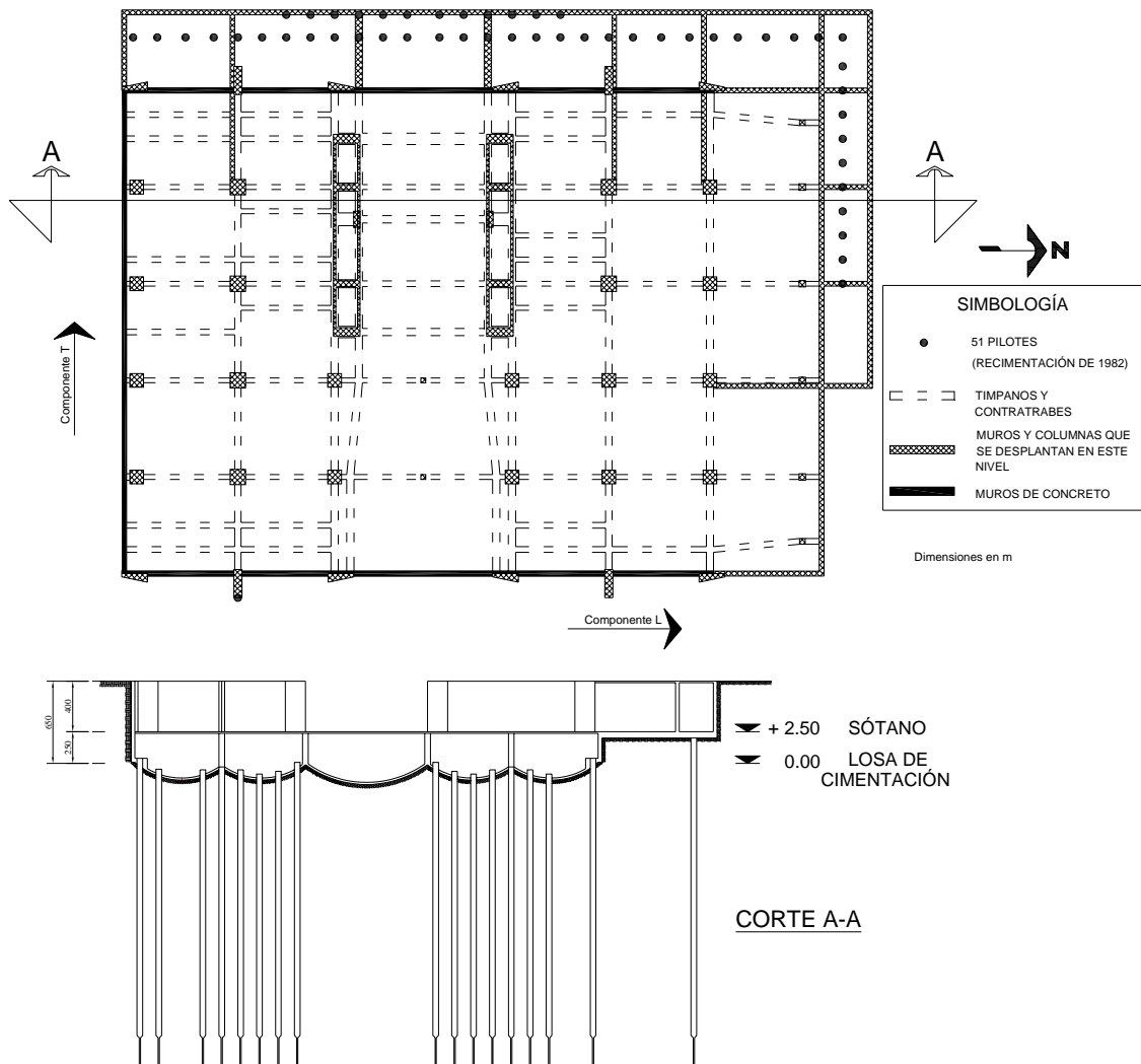
Figura 2.16 Ubicación de los 51 pilotes de la recimentación del edificio
