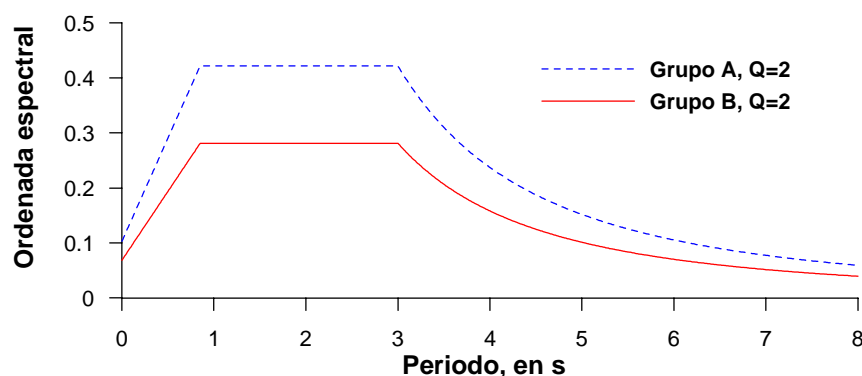
Figura 4.17 Espectro de aceleraciones de diseño del edificio, de NTC-sismo, 2004
