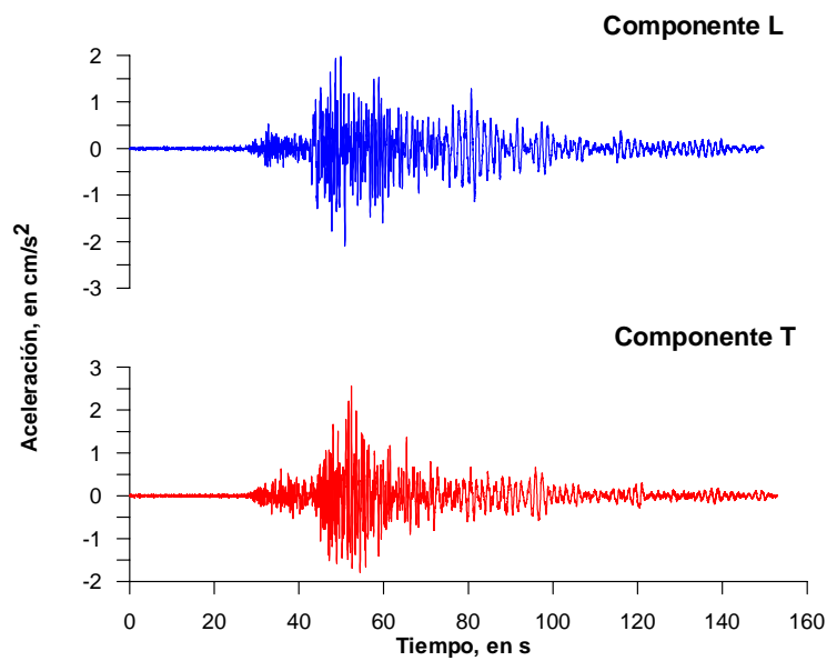
Figura 3.8 Aceleraciones experimentales de terreno registradas durante el evento sísmico TT04-3 en los componentes L y T
