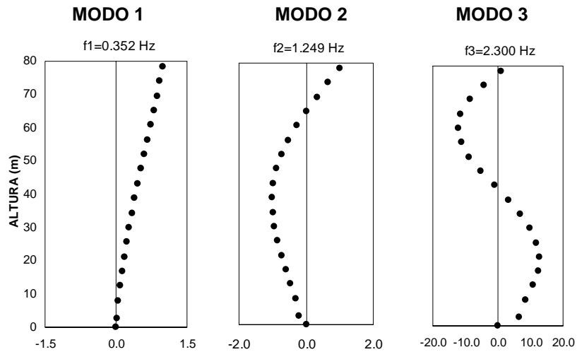
Figura 4.4 Formas modales analíticas del componente T
