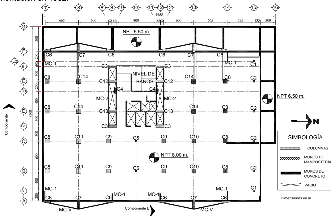
Figura 2.17 Planta Baja rehabilitada
