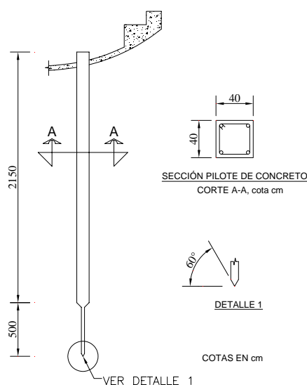
Figura 2.1 Pilotes, características geométricas
