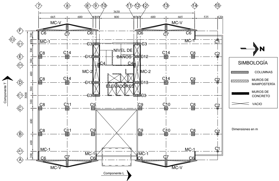
Figura 2.5 Planta niveles N1 y N2
