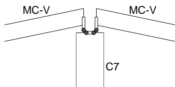
Figura 4.11 Desacoplamiento de los muros MC-V en el modelo TC-S1a
