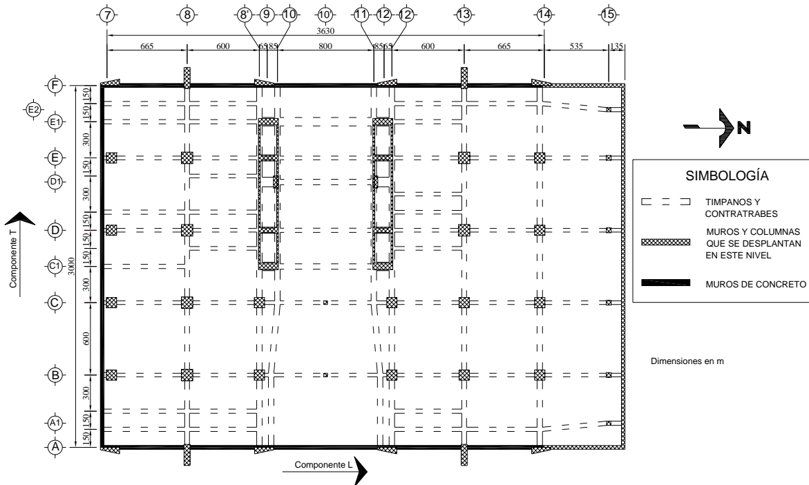
Figura 2.3 Planta nivel Sótano (NS1)
