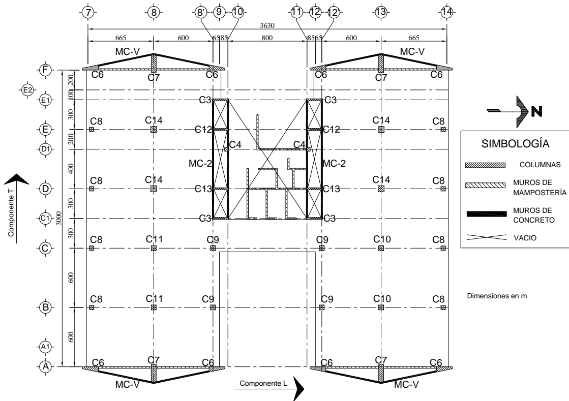
Figura 2.8 Planta nivel N16
