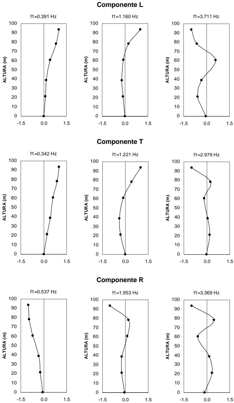
Figura 3.4 Formas modales con apéndice para condiciones de vibración ambiental
