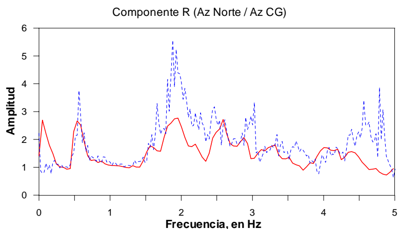
Figura 3.3 Función de transferencia entre azotea norte y azotea centro geométrico en componente T, para las vibraciones ambientales VA04-1 (línea continua) y VA04-3 (línea discontinua)
