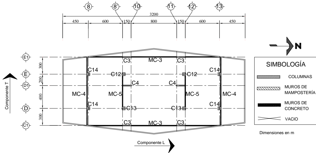
Figura 2.10 Planta nivel N17
