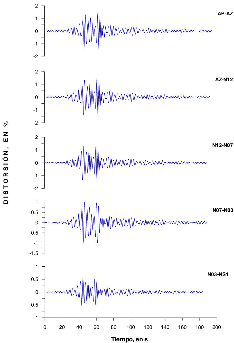
Figura 4.15 Historia de distorsiones en el componente T del modelo TC-S2, al ser sometido a las excitaciones del sismo de septiembre de 1985 ocurrido en la ciudad de México
