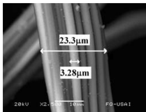
Figura 5. Micrografía del cátodo
