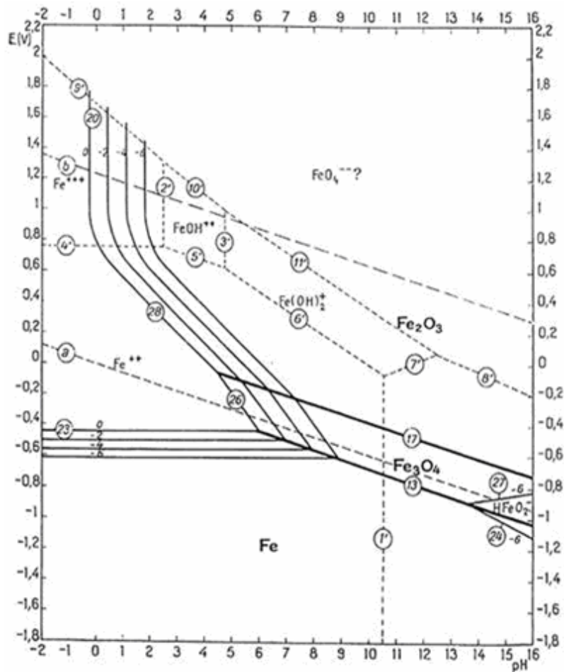
Figura 2. Diagrama de equilibrio pH-Potencial del hierro-agua a 25°C.
