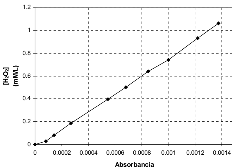
Gráfica 15. Curva de calibración del peróxido de hidrógeno.
