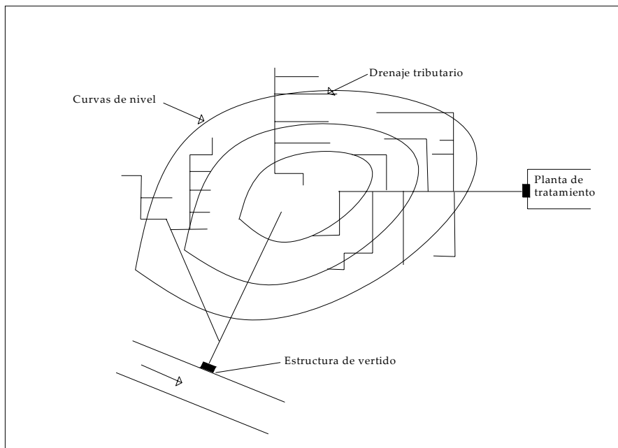
Figura 3.5 Sistema radial
