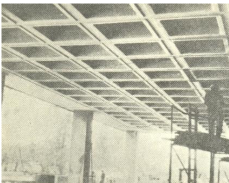
Figura III.XI Desconchamiento de una losa nervada en la planta baja de un edificio administrativo por efectos de incendio.
