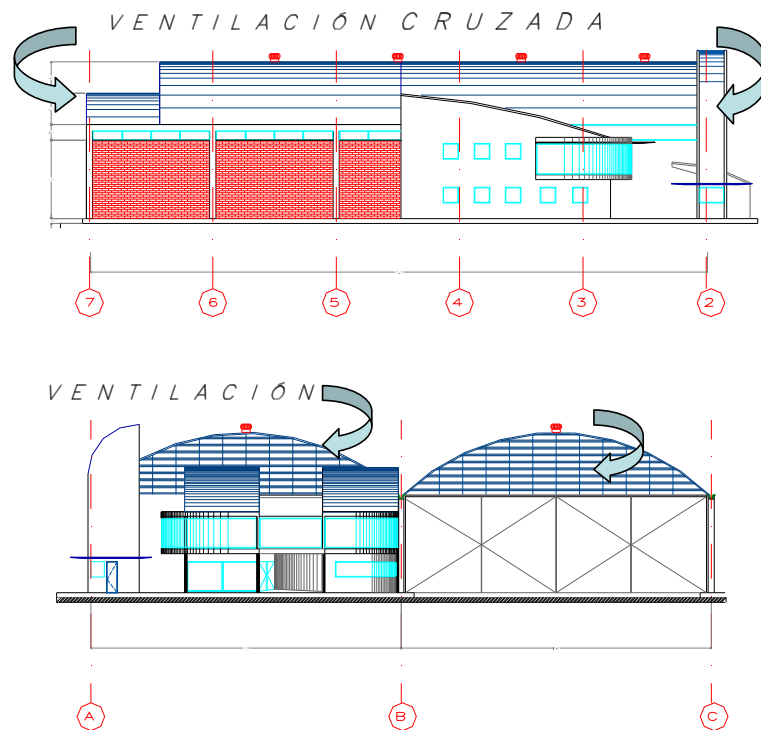
Figura II.III' Diseño de Naves industriales con tipo de ventilación para seguridad contra incendio
