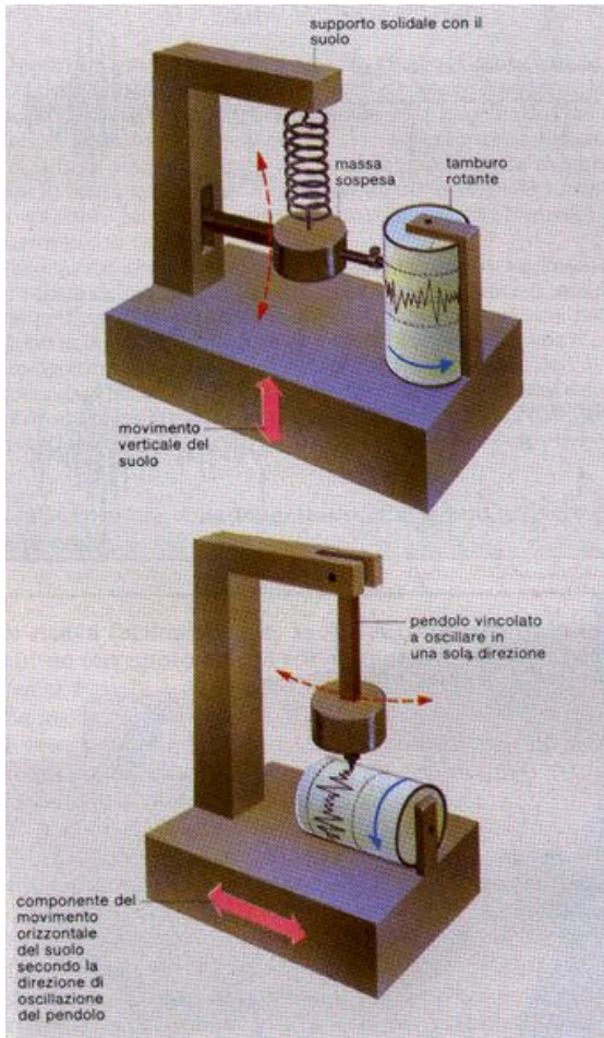
. Figura I.X Principio básico de operación y registro de un sismógrafo que mide el desplazamiento vertical del terreno.
