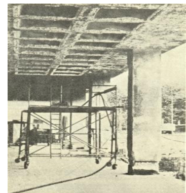
Figura III.XI Desconchamiento de una losa nervada en la planta baja de un edificio administrativo por efectos de incendio.
