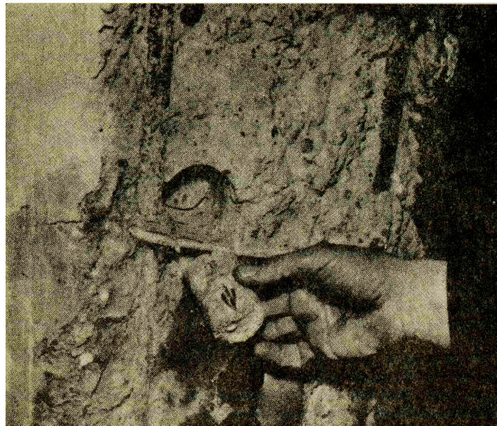
Figura III.VI Núcleos de concreto endurecido de diámetro pequeño auxilian a dimensionar adecuadamente la profundidad de la coloración rosada y los micro agrietamientos existentes.
