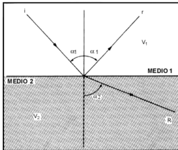
Figura I.VIII rayo incidente, r rayo reflejado, R rayo refractado.
