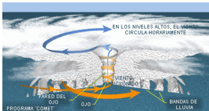
Figura I.XVIII Partes de un Huracán
