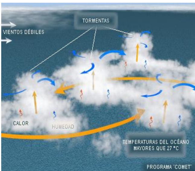
Figura I.XVII Grafica de como se forma un Huracán.
