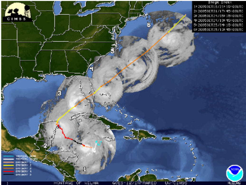
Trayectoria del huracán “wilma”. UW-CIMMS
