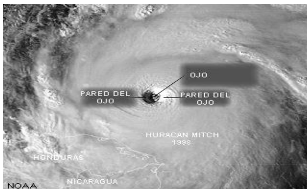
Figura I.XIX Vista de un ojo del Huracán desde un satélite.
