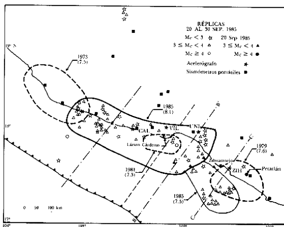
Figura I.II Áreas de ruptura y réplicas de los sismos de Michoacán de septiembre de 1985.
