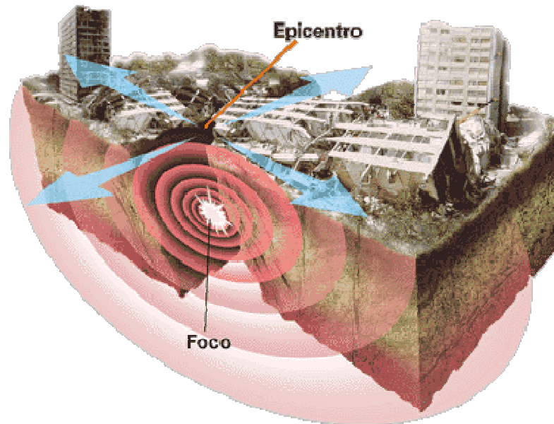
Figura I.IV Vista de epicentro y Foco en el sismo
