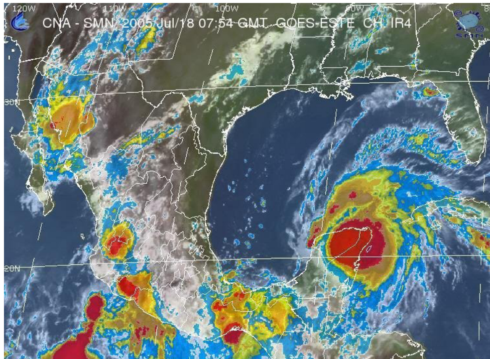
IMAGEN DEL SATÉLITE GOES-E EN CANAL INFRARROJO IR4 PRIMER IMPACTO EN MÉXICO SOBRE LA PENÍNSULA DE YUCATÁN 18 DE JULIO DE 2005 / 07:54 GMT
