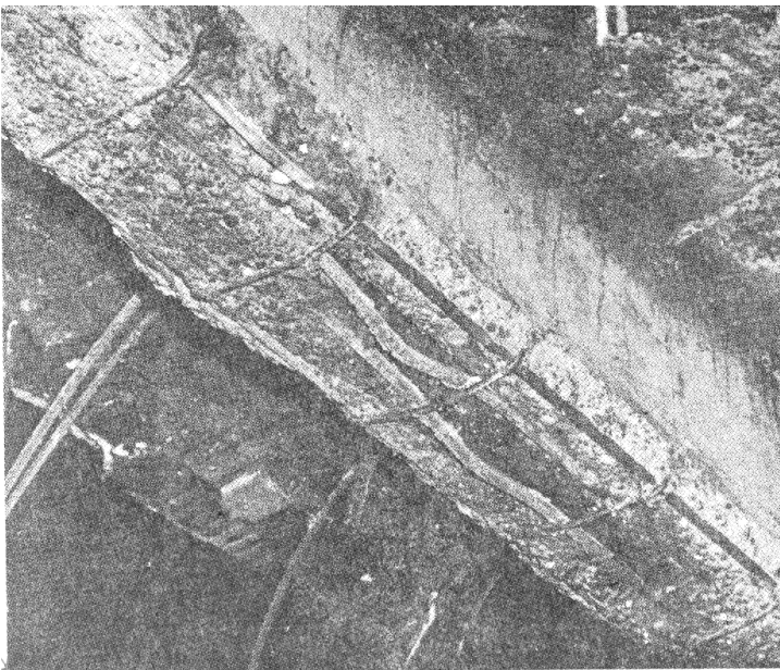
Figura III.VII Muestra del desconchamiento debido a la acción del fuego.
