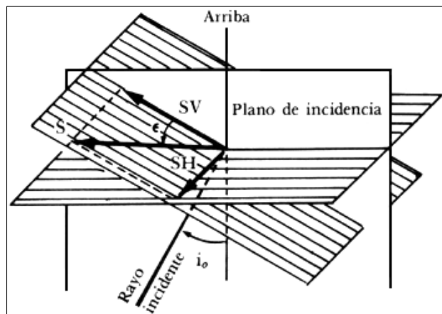
Figura I.VII. La onda S y sus componentes SV y SH.
