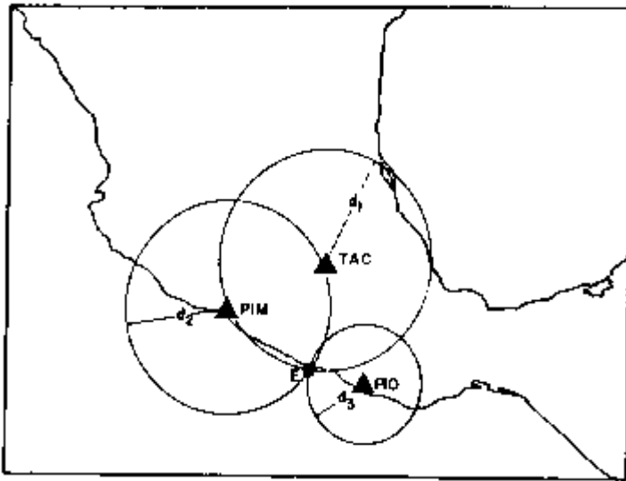
Figura I.XI Conociendo la distancia ( d ) de una estación sismológica al epicentro, ésta puede representarse como un círculo de radio d con centro en dicha estación. Si contamos con observaciones al menos en tres estaciones, el punto de intersección ( E ) de los círculos corresponde al epicentro. En la figura se representa el ejemplo de un sismo en las costas de Guerrero, localizado mediante registros de las estaciones: Tacubaya, D.F. (TAC); Presa Infiernillo, Mich. (PIM); y Pinoterpa Nacional, Oax. (PIO).
