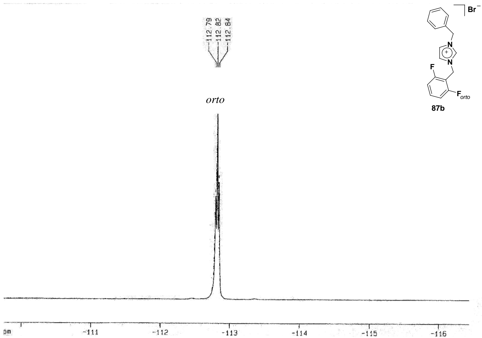
Apéndice VI. RMN 19 F (CDCl 3 ) del compuesto 87b .
