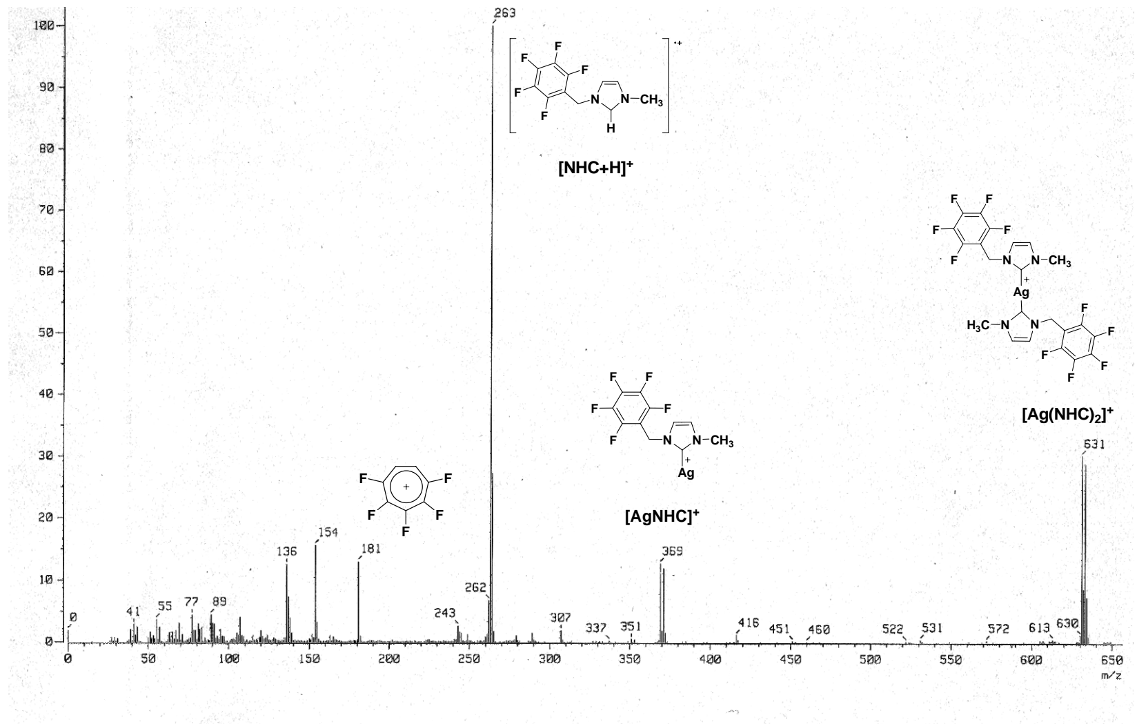
Apéndice XII. EM-FAB + del compuesto (NHC)AgBr 85a.
