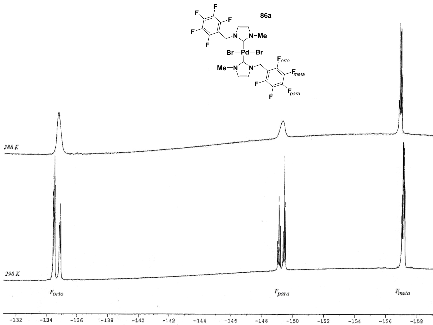
Apéndice XVII. RMN ^{19}\text{F} ( \text{CDCl}_3 ) a alta temperatura del compuesto (NHC)Pd(II) 86a .
