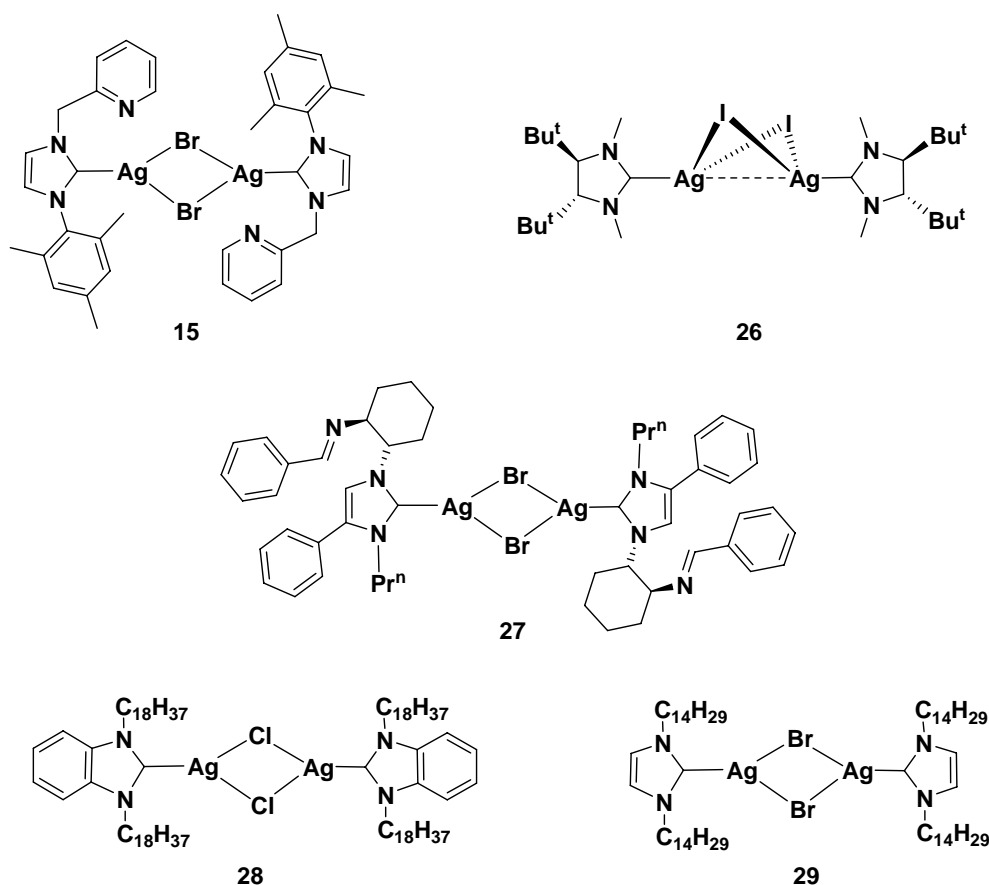
Figura. 8. Estructuras multinucleares tipo [\text{AgLX}]_2 .
