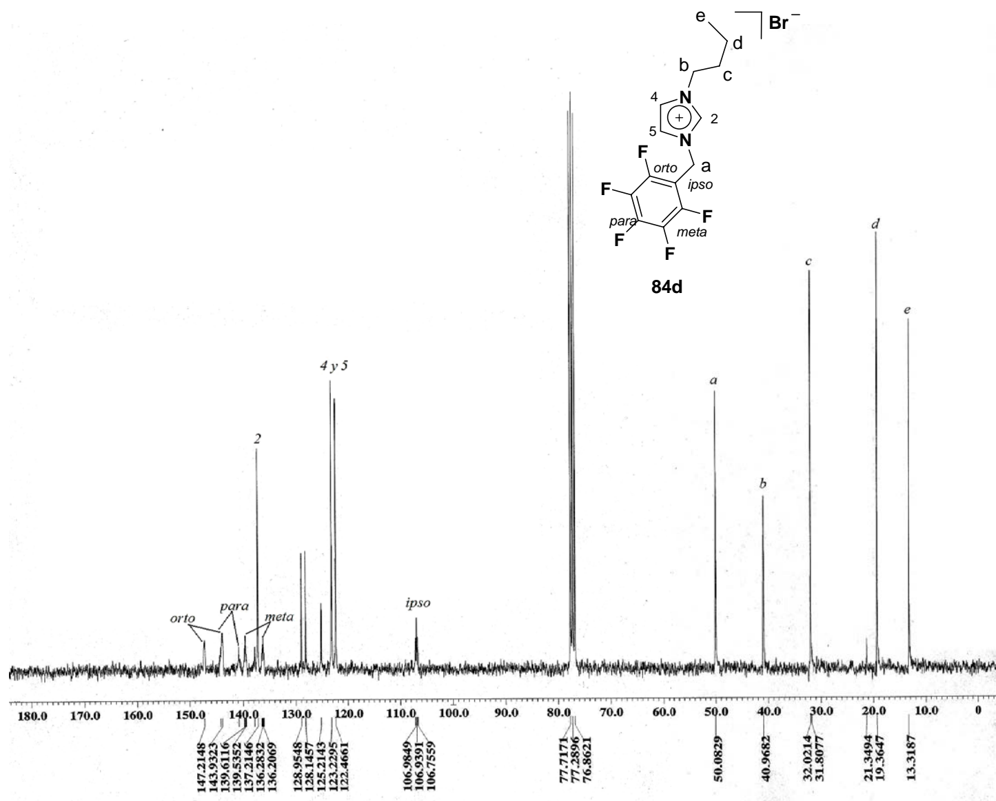
Apéndice III. RMN ^{13}\text{C}\{^1\text{H}\} ( \text{CDCl}_3 ) del compuesto 84d .
