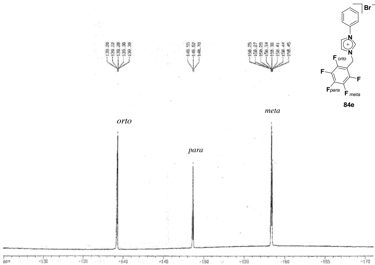
Apéndice IV. RMN ^{19}\text{F} ( \text{CDCl}_3 ) del compuesto 84e .
