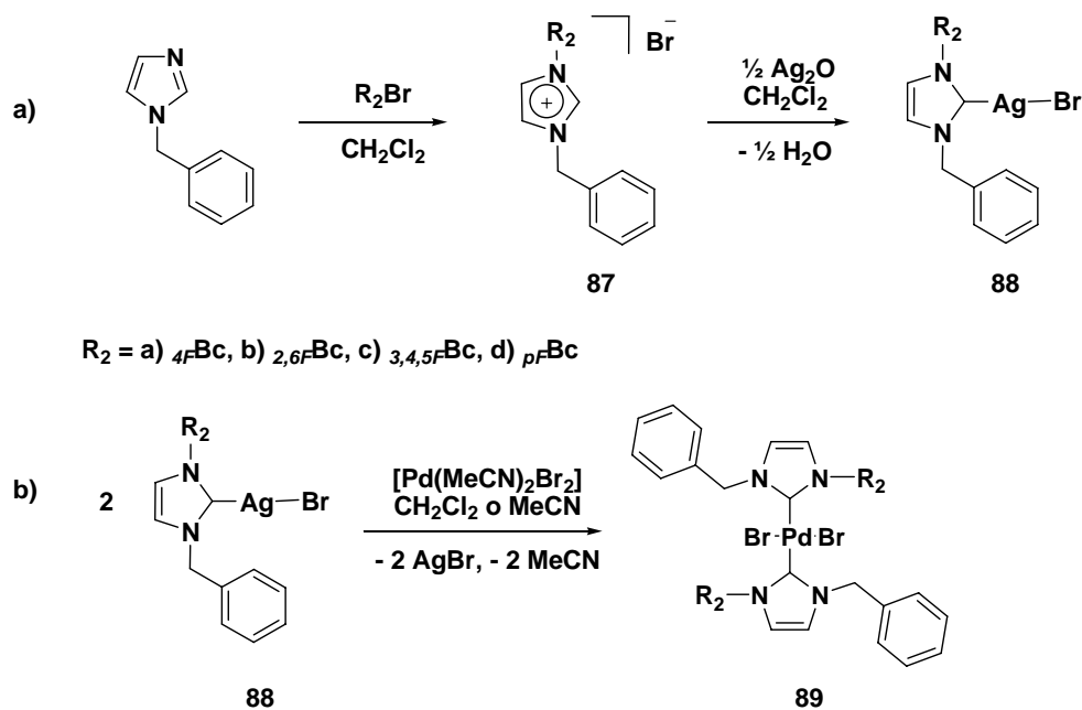
Esquema 28. a) Uso de 1-bencilimidazol y bromuros de bencilo mono, di, tri y pentafluorados para obtener compuestos NHC fluorados de Ag(I) (por simplicidad se utiliza el tipo C-Ag-X para describir las estructuras de plata 88 , pero no necesariamente pertenecen a esta clasificación). b) reacciones de transferencia con [\text{Pd}(\text{MeCN})_2\text{Br}_2] para generar carbenos N -heterocíclicos fluorados de Pd(II).
