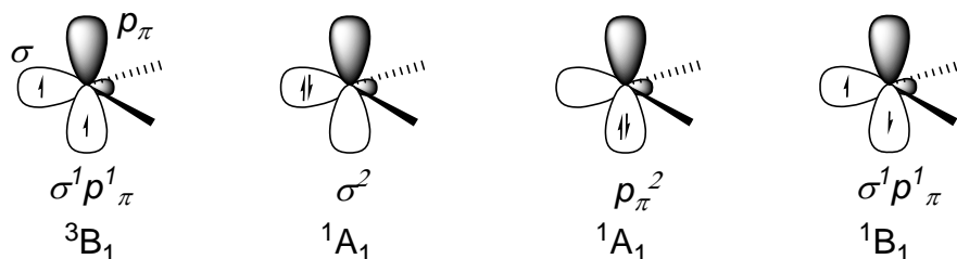
Figura 3. Configuraciones electrónicas de carbenos.
