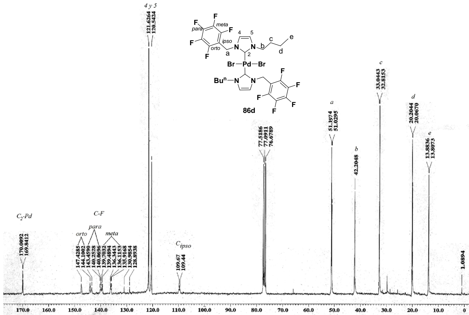
Apéndice XVI. RMN 13 C{ 1 H} (CDCl 3 ) del compuesto (NHC)Pd(II) 86d.
