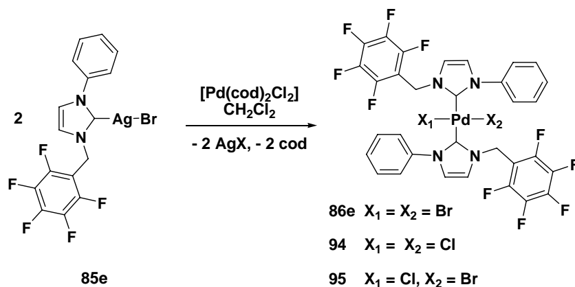
Esquema 31. Experimento de transferencia usando 85e y [\text{Pd}(\text{cod})\text{Cl}_2] que dio lugar a una mezcla de halógenos Cl y Br en los compuestos NHC de paladio(II)
