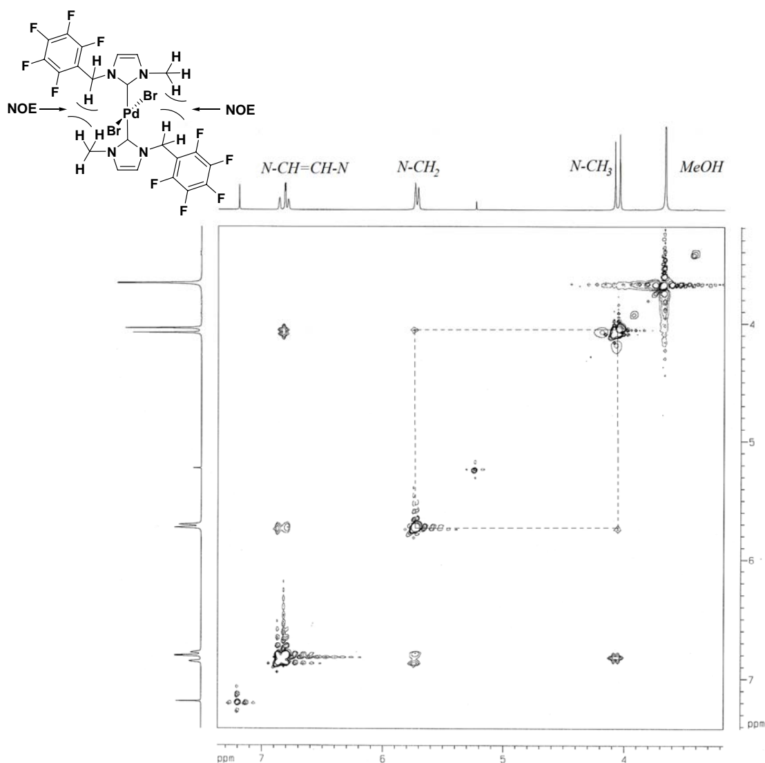
Figura 39. Experimento NOESY ^1\text{H} del compuesto 86a . La línea punteada muestra interacciones importantes mediante el efecto Nuclear Overhauser (NOE) entre los metilenos ( N\text{-CH}_2 ) y metilos ( N\text{-CH}_3 ) de los ligandos NHC.
