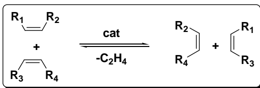
Esquema 16. El principio de la metátesis de olefinas.
