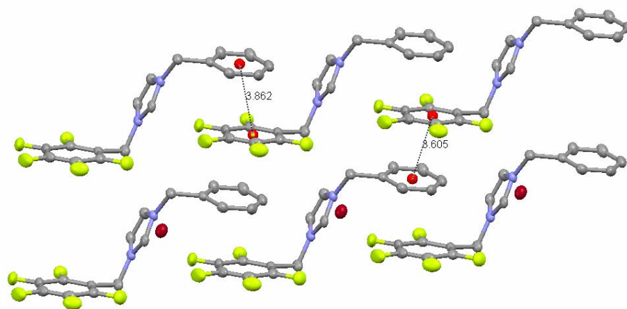
Figura 25. Arreglo supramolecular asimétrico en 3D de pF - BcBcImBr 87d . En color verde los átomos de F, en azul los átomos de N, en color rojo oscuro los átomos de Br y en color rojo claro los centroides.
