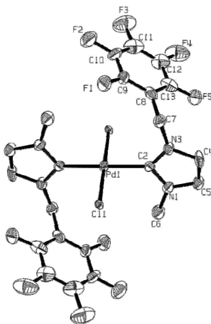
Figura 16. Diagrama ORTEP de la estructura de rayos-X del compuesto 93 .
