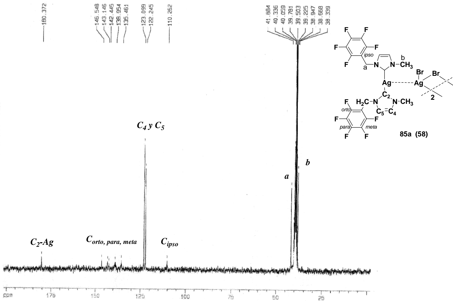
Apéndice X. RMN 13 C{ 1 H} (DMSO- d 6 ) del compuesto (NHC)AgBr 85a (58).
