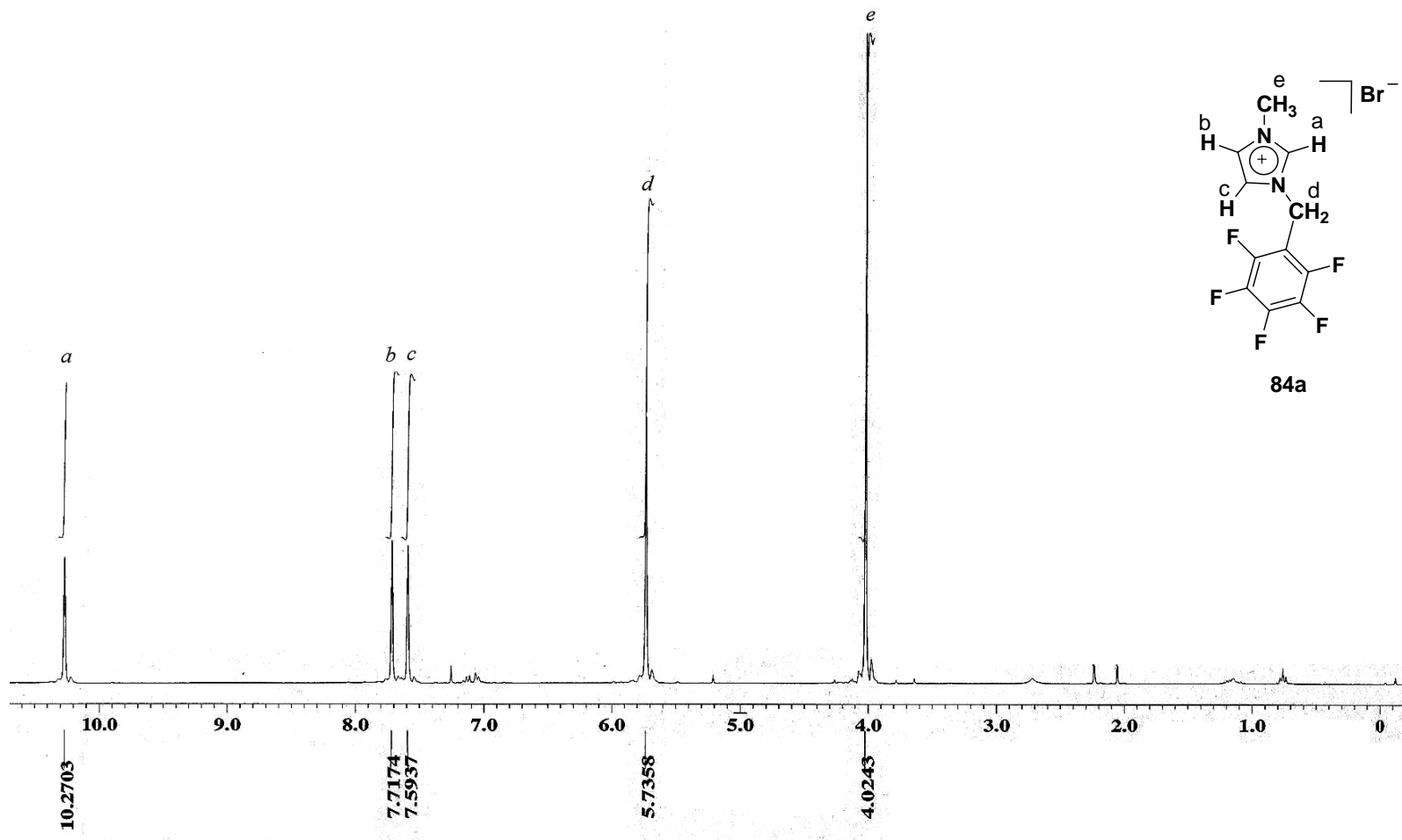
Apéndice II. RMN 1 H (CDCl 3 ) del compuesto 84a .
