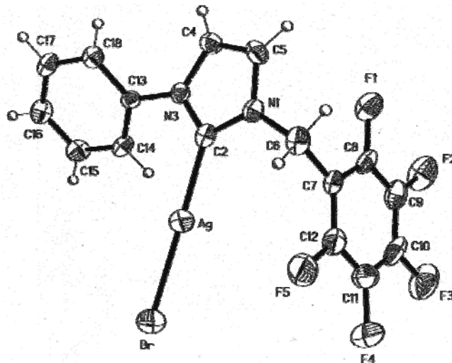
Figura 29. Estructura de rayos-X del compuesto 85e .
