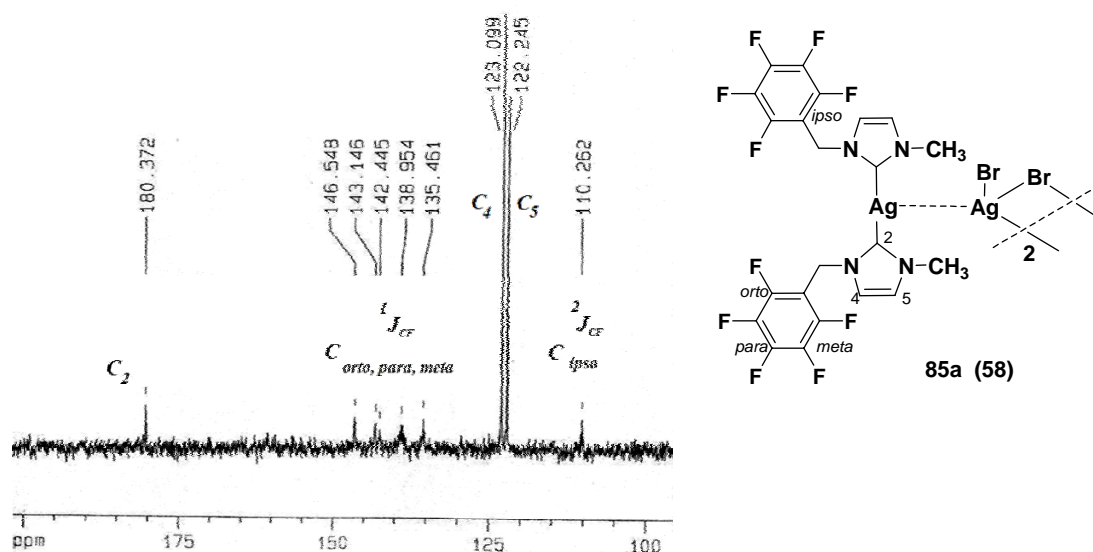
Figura 26. RMN ^{13}\text{C}\{^1\text{H}\} de 85a para C_2 -Ag, C -F ( orto , para , meta ), C_4 , C_5 y C_{ipso} .
