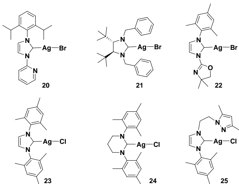
Figura. 7. Estructuras mononucleares tipo [\text{AgLX}] .
