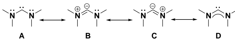
Esquema 3. Estructuras de resonancia para diaminocarbenos.
