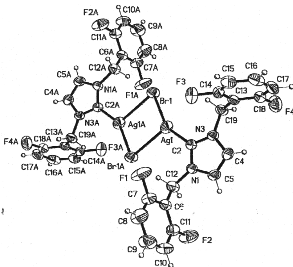
Figura 31. Estructura de rayos-X del compuesto 91b .
