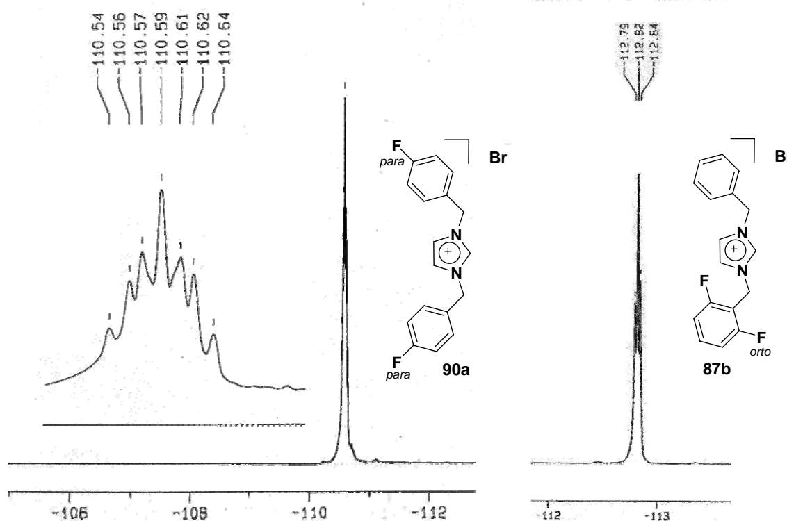
Figura 21. Señales en RMN ^{19}\text{F} : séptuple de 90a y triple de 87b .
