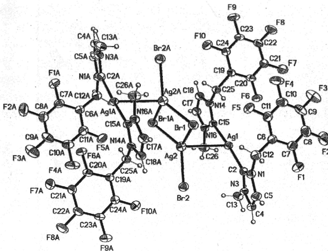
Figura 34. Estructura de rayos-X del compuesto 85a .
