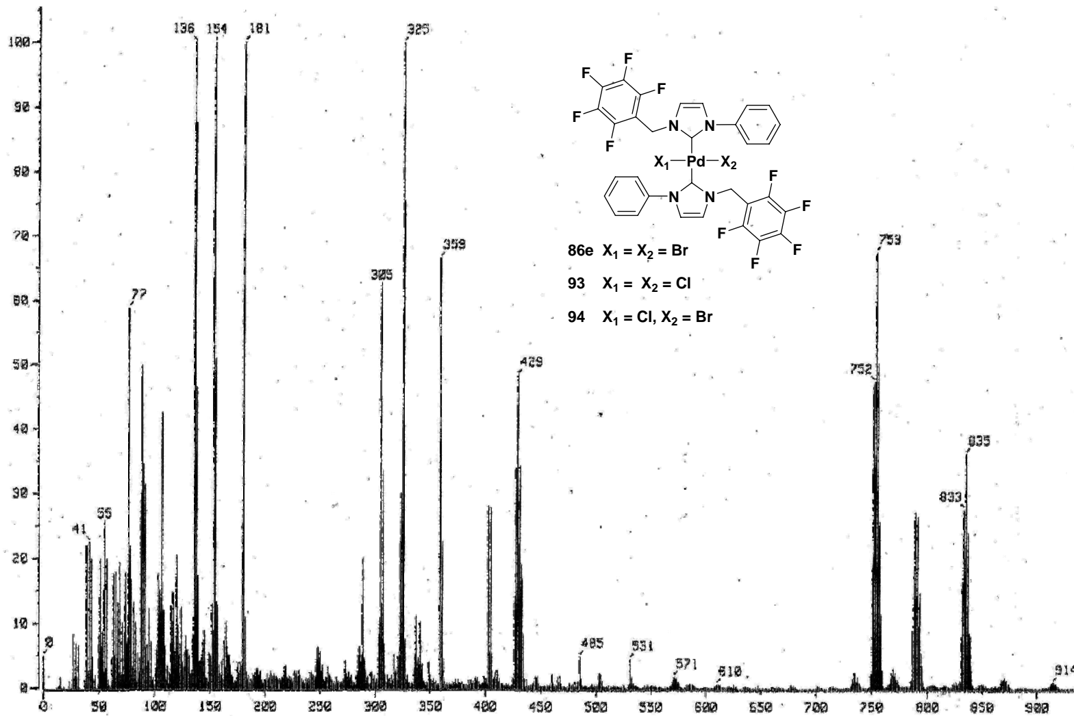
Apéndice I. EM-FAB + de la mezcla de compuestos 86e, 93 y 94.
