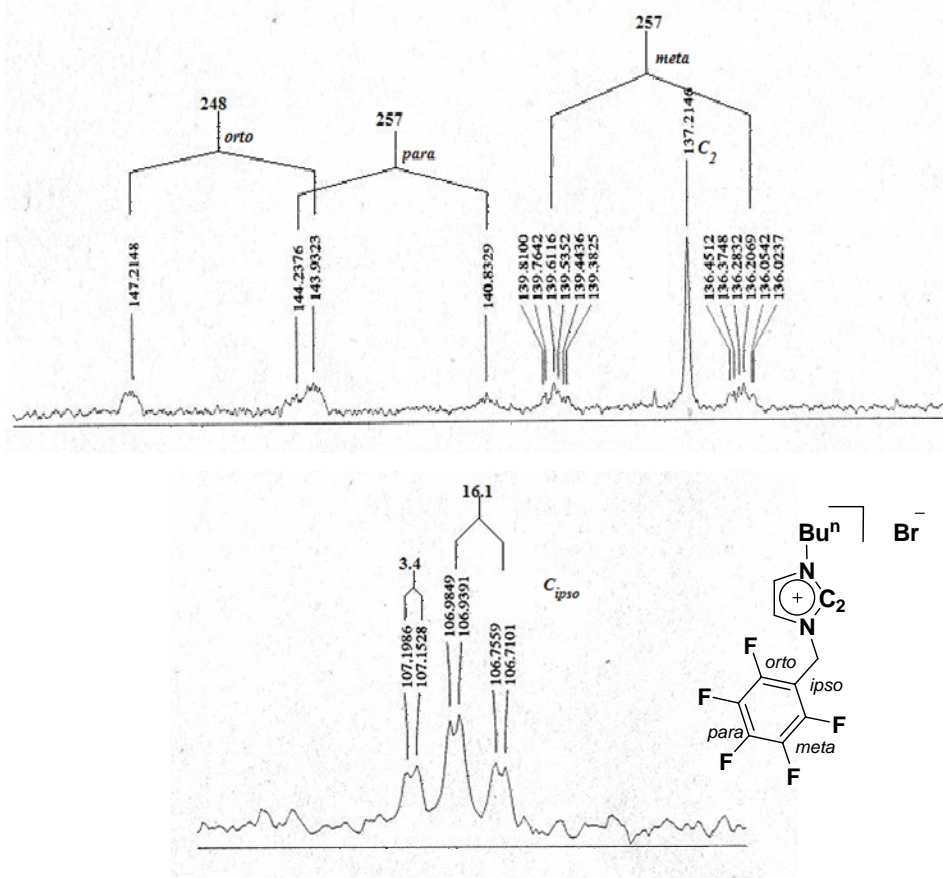
Figura 19. Ampliación del espectro de RMN ^{13}\text{C}\{^1\text{H}\} del compuesto 84d mostrando: (arriba) las señales correspondientes a C_{orto} , C_{para} , C_{meta} y C_2 (abajo) señal td correspondiente al C_{ipso} .
