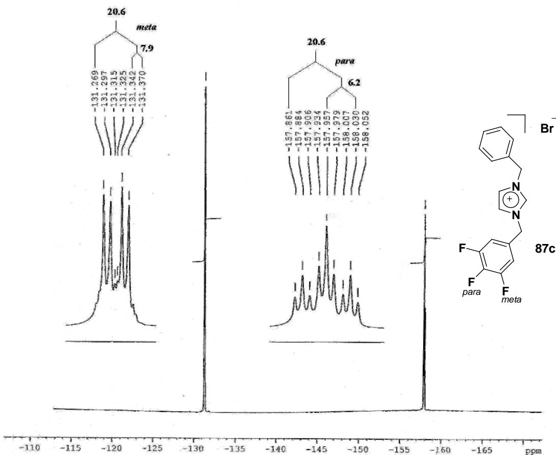
Figura 22. RMN ^{19}\text{F} del compuesto 87c.
