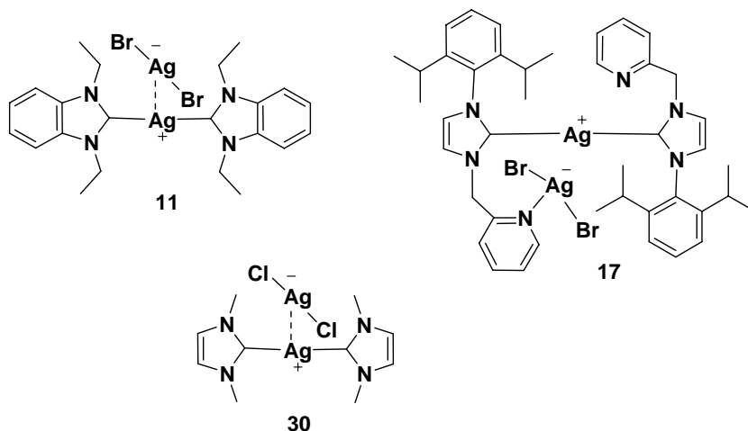
Figura 10. Estructuras multinucleares tipo [Ag(NHC)_2]^+[AgX_2]^- .
