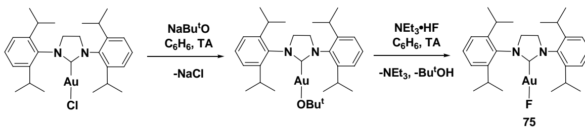
Esquema 22. Preparación del primer compuesto NHC de Au(I) que presenta el enlace Au-F .
