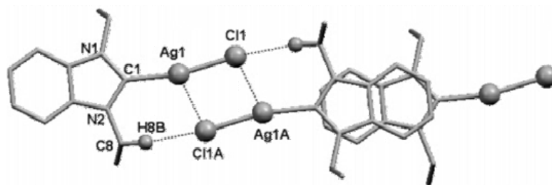
Figura 9. Interacciones intermoleculares CH\cdots Cl y \pi\cdots\pi de 28 . Para mayor claridad se omite C_{18}H_{37} .
