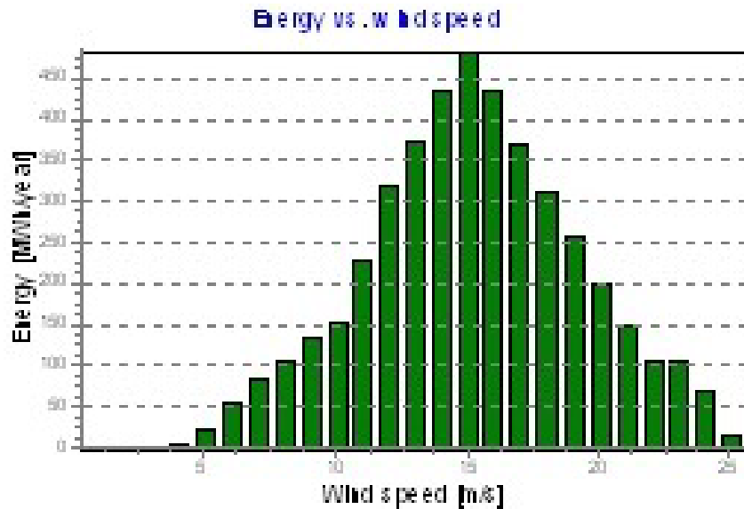
Figura V.15. Análisis Energía vs Velocidad de Viento
