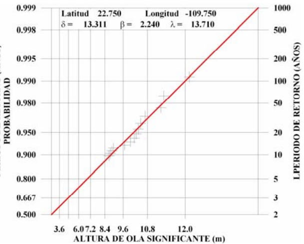
Figura 6-29 Distribución extremal de Weibull para altura de ola significativa
