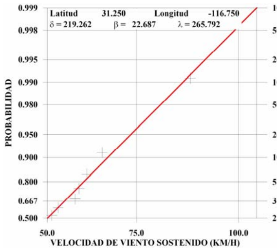
Figura 6-30 Distribución extremal de Weibull para velocidad de viento a 10 m SMM
