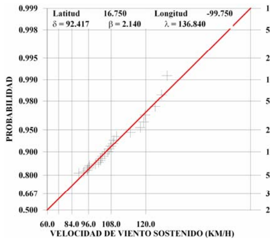
Figura 6-12 Distribución extremal de Weibull para velocidad de viento a 10 m SMM
