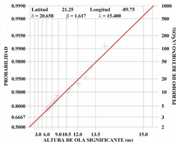
Figura 5-17 Distribución extremal de Weibull para altura de ola significativa
