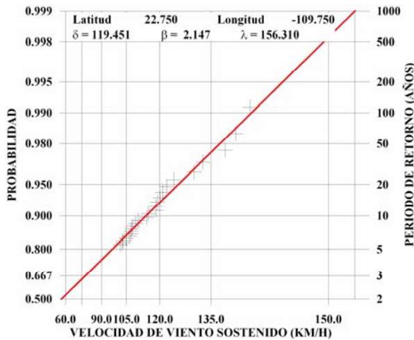
Figura 6-28 Distribución extremal de Weibull para velocidad de viento a 10 m SMM
