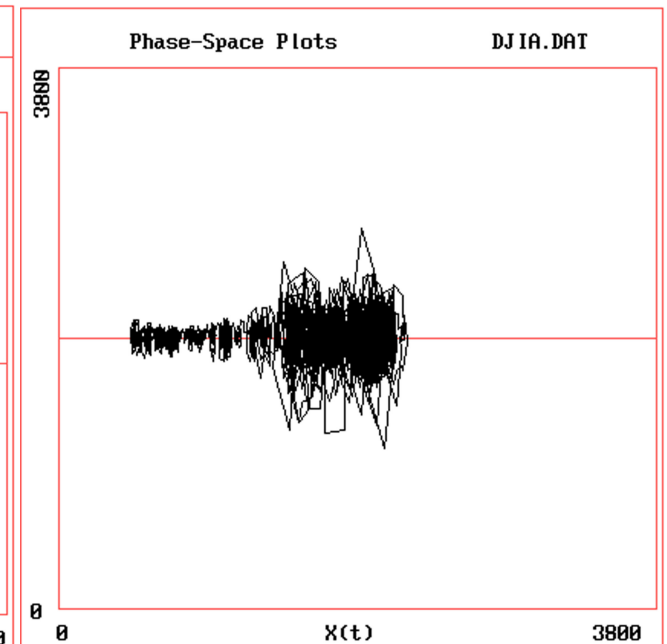
Figura 6.14 Atractor en dos planos DJIA
