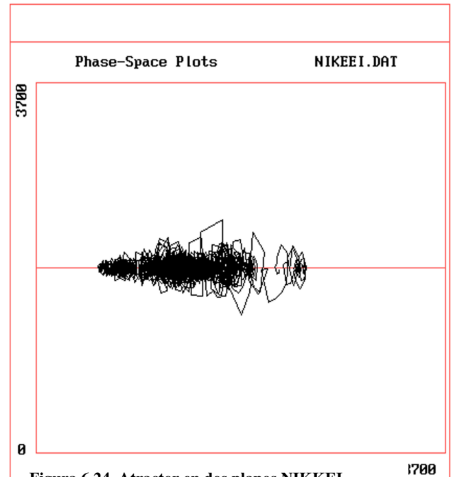
Figura 6.24 Atractor en dos planos NIKKEI
