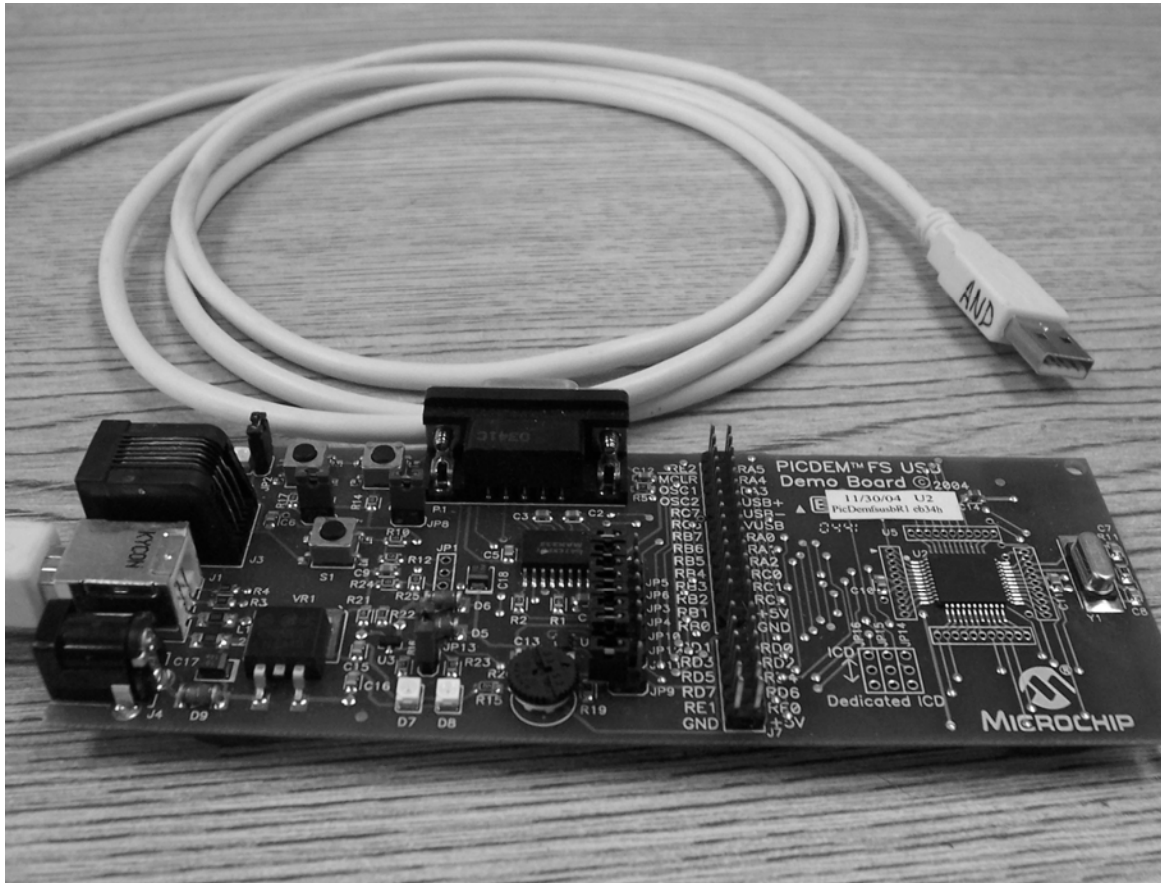
Figura 33. Tarjeta de evaluación de Microchip “PICDEM FS USB”, para el PIC184550.
