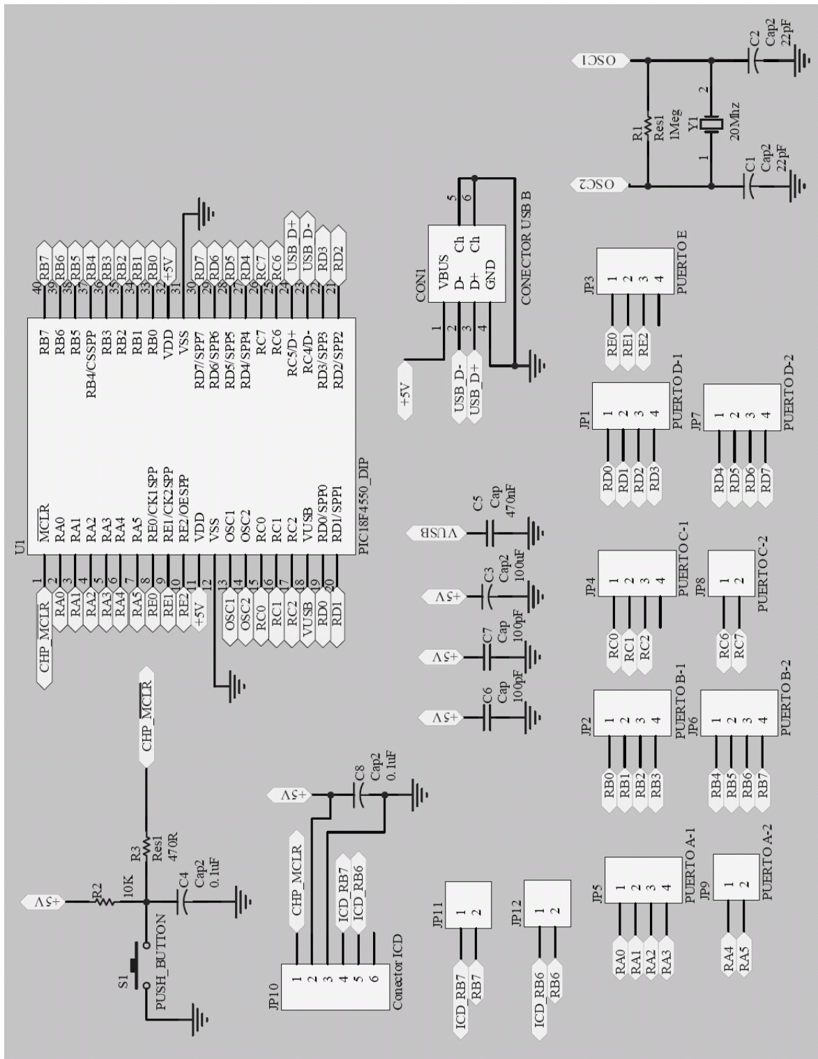
Figura 34. Diagrama de la interfaz USB.
