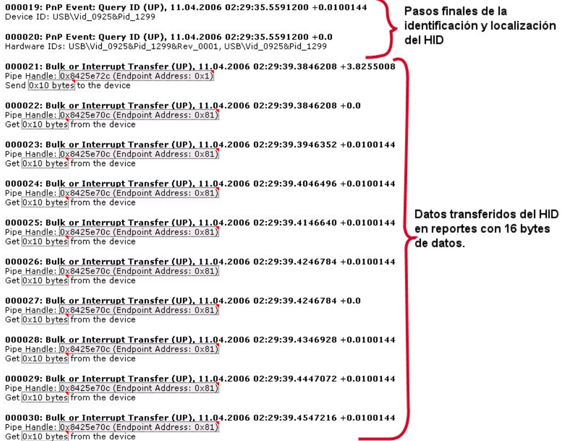
Figura 32. Análisis del microcontrolador con el firmware HID9 y el host con el software Interfaz1.
