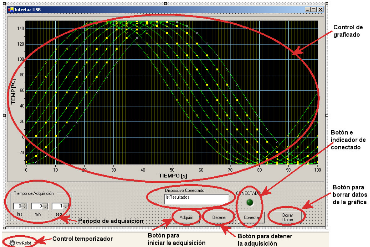
Figura 25. Interfaz final para el sistema de adquisición de temperatura.
