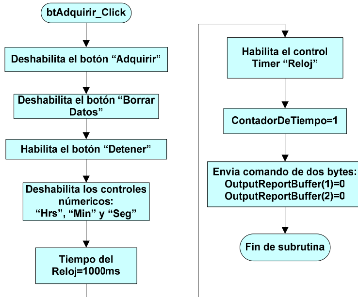
Figura 28. Función del botón "Adquirir".
