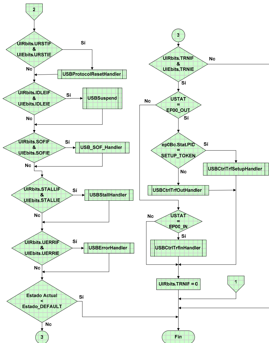
Figura 8. Segunda parte del diagrama de la función USBTasks .
