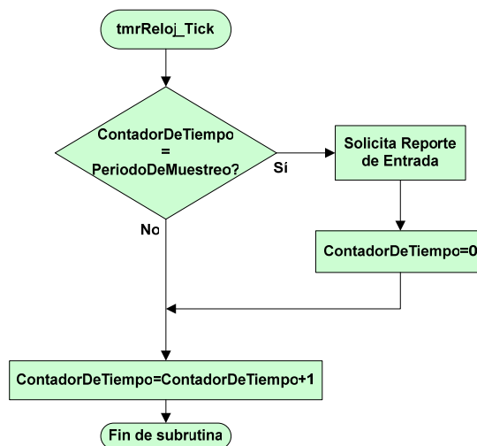
Figura 29. Función del control temporizador.
