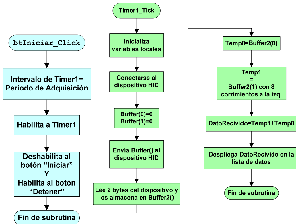
Figura 17. Funciones btIniciar_Click y Timer1_Tick de HIDCOMM2 .
