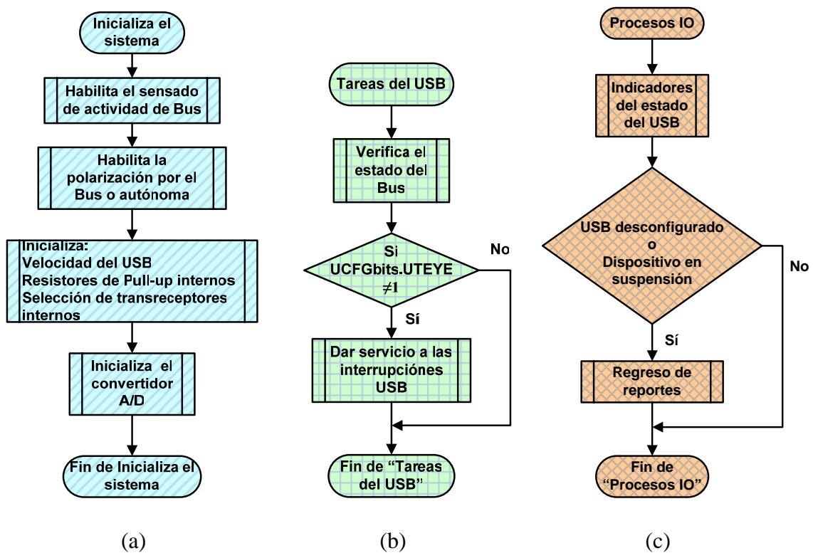
Figura 4. (a) Subrutina "Inicializa el sistema" (b) Subrutina "Tareas del USB" (c) Subrutina "Procesos IO".
