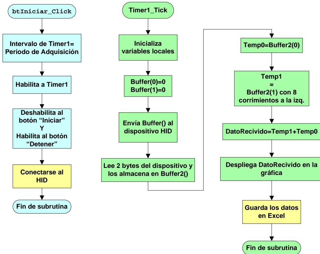
Figura 21. Funciones btIniciar_Click y Timer1_Tick de HIDCOMM4 .
