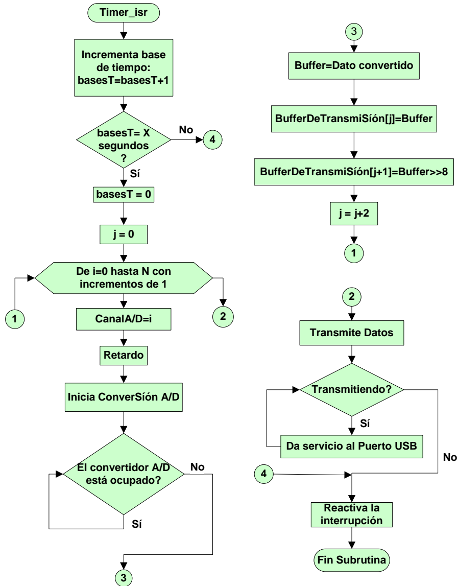
Figura 12. Subrutina de atención a la interrupción del Timer0.
