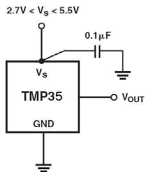
Figura 10. Aplicación típica.
