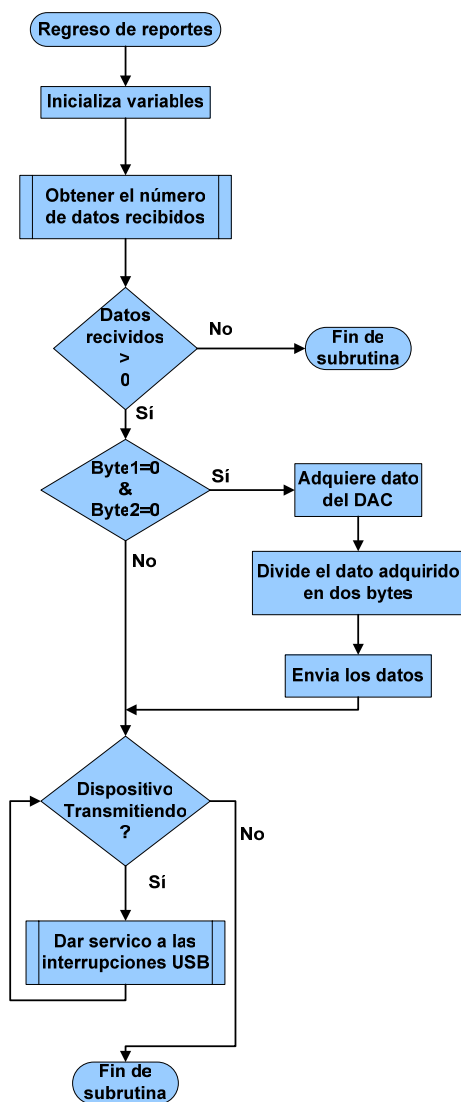
Figura 6. Subrutina “Regreso de reportes” del programa de prueba HID3.
