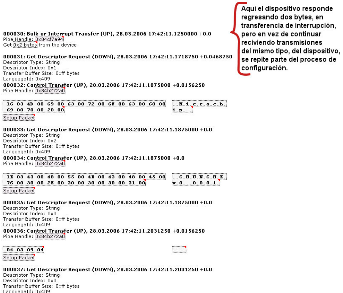
Figura 19. Análisis de la comunicación entre el software HIDCOMM2 y el firmware HID3 (segunda parte).
