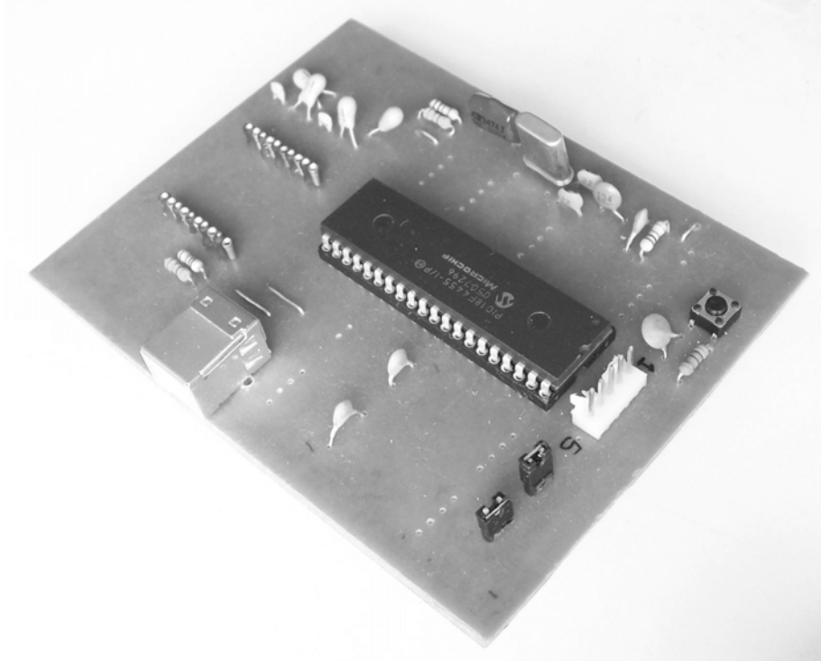
Figura 36. Primer prototipo de la interfaz USB (vista superior).
