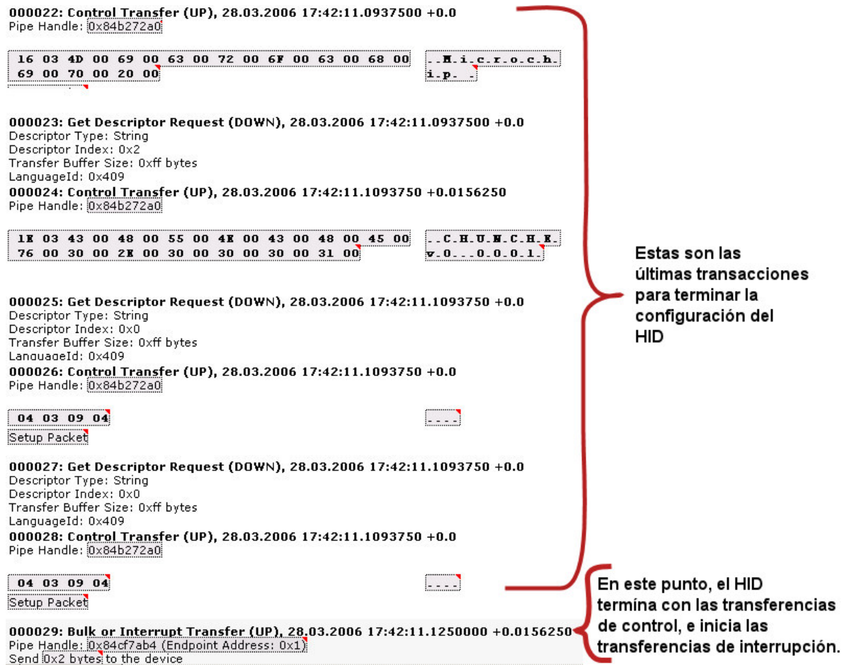
Figura 18. Análisis de la comunicación entre el software HIDCOMM2 y el firmware HID3.
