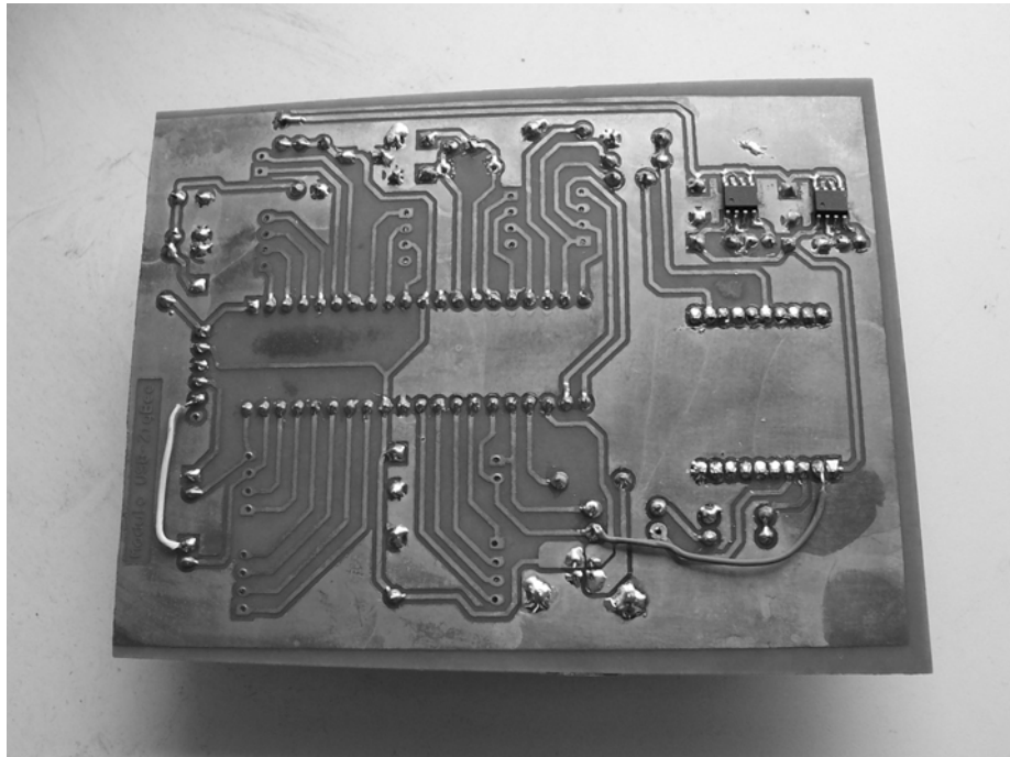
Figura 37. Primer prototipo de la interfaz USB (vista inferior).
