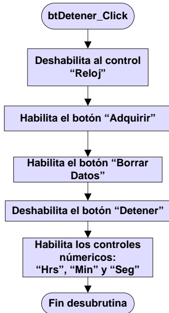
Figura 30. Función del botón “Detener”.
