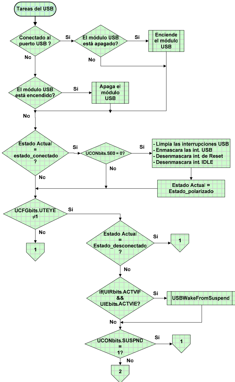
Figura 7. Primera parte del diagrama de la función “Tareas del USB” ( USBTasks ).
