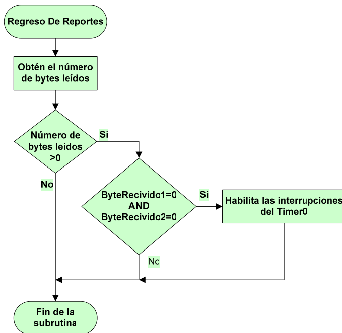
Figura 11. Diagrama de la función “Regreso De Reportes”, de la versión HID9.
