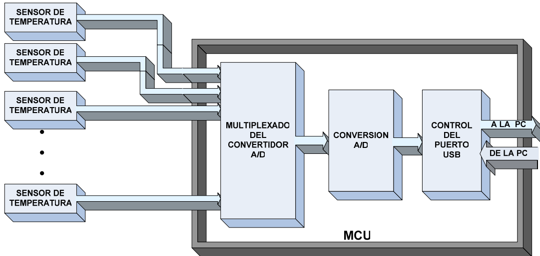
Figura 9. Sistema de monitoreo de temperatura.
