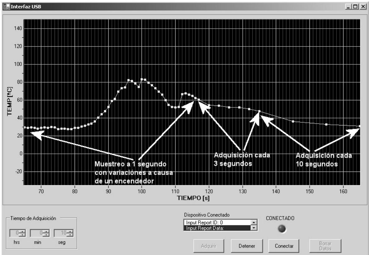
Figura 31. Corrida de la interfaz final, conectada al HID.
