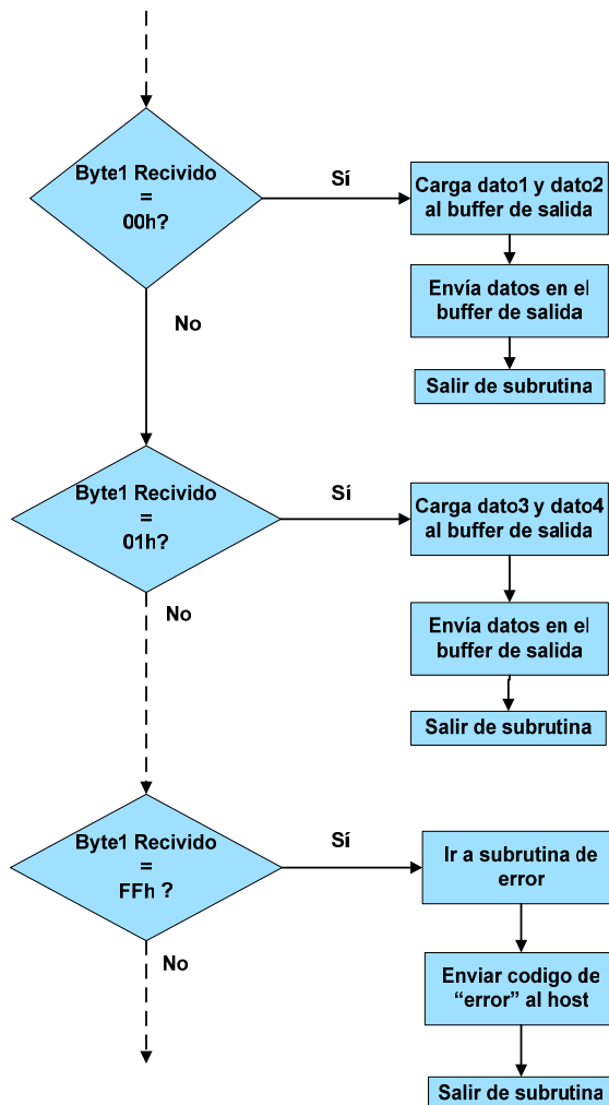
Figura 5. Diagrama simplificado de secuencia de comandos en el microcontrolador.
