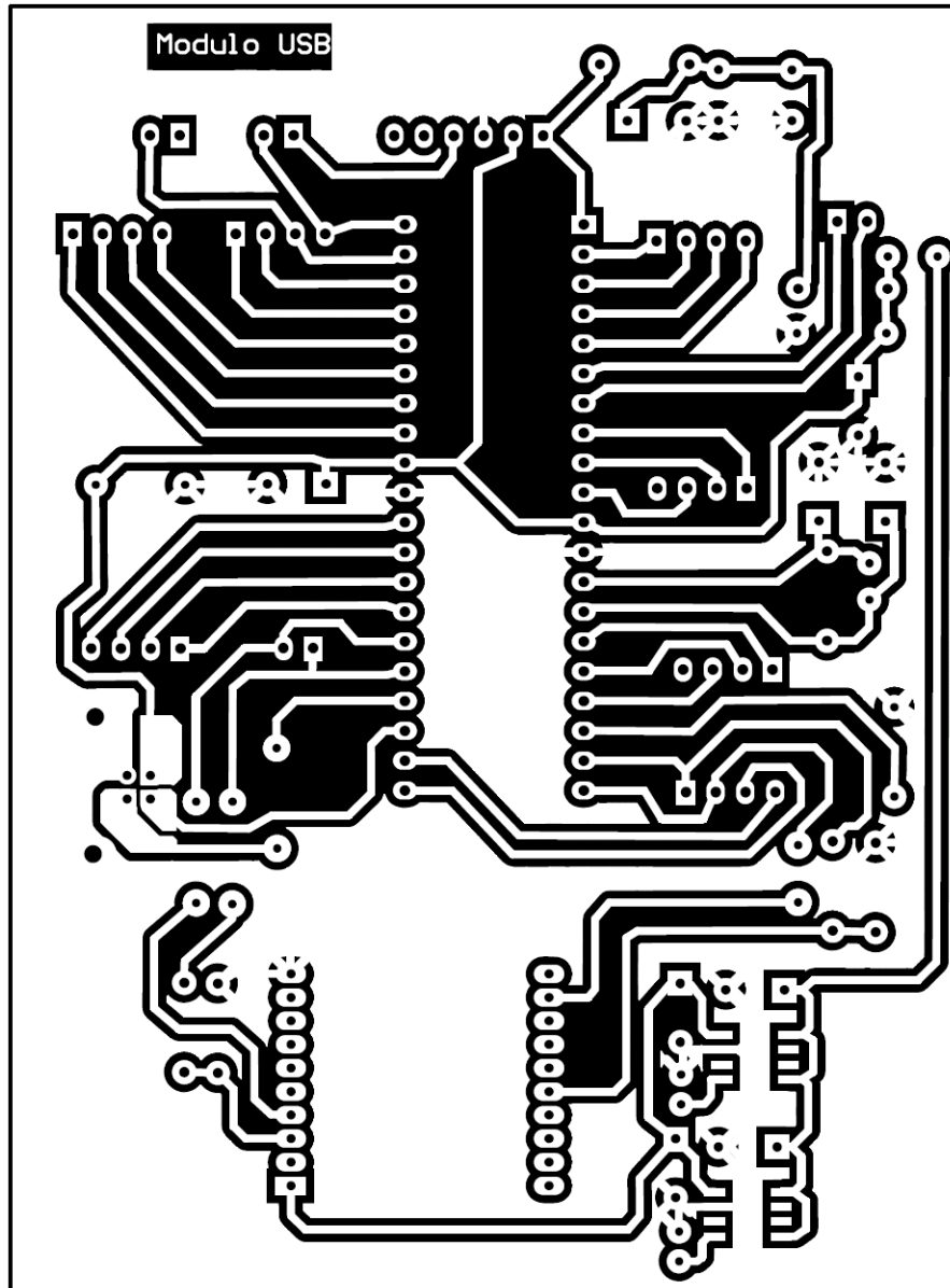
Figura 35. Diagrama del circuito impreso de la interfaz USB.
