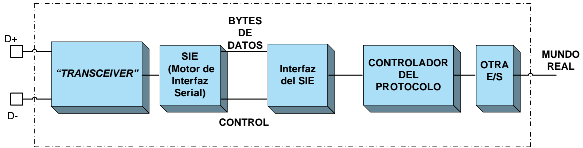
Figura 2. Diagrama de bloques de un dispositivo de E/S.
