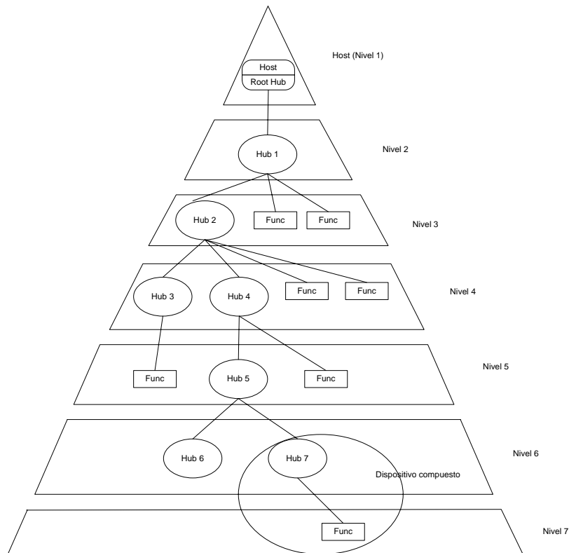
Figura 1. Topología del puerto USB.
