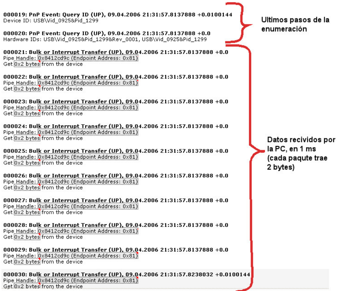
Figura 24. Análisis de la comunicación entre el dispositivo de interfaz humana con el firmware HID9 y el programa interfaz USBHIDIO5.
