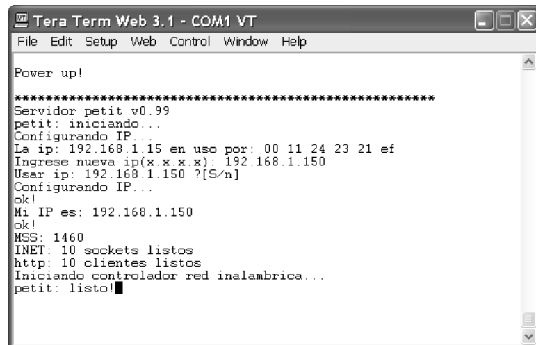
Figura 3.10: Captura de configuración de la dirección IP
