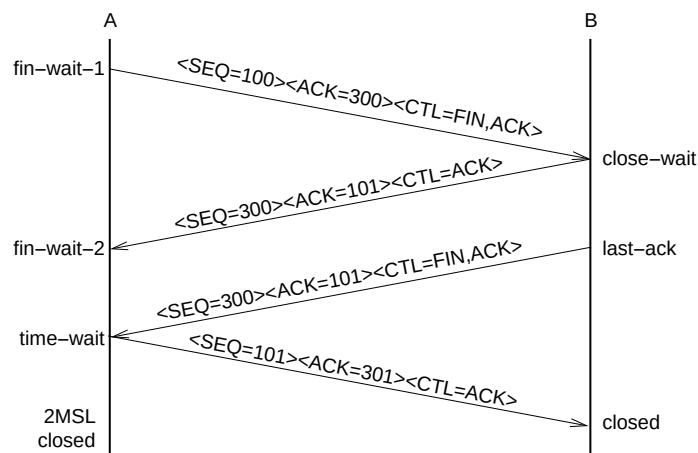
Figura 1.13: Cierre de conexión básico de 4 etapas de TCP
