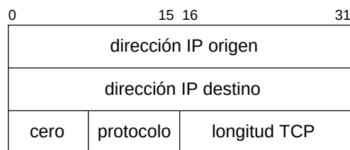
Figura 1.10: Pseudo cabecera TCP
