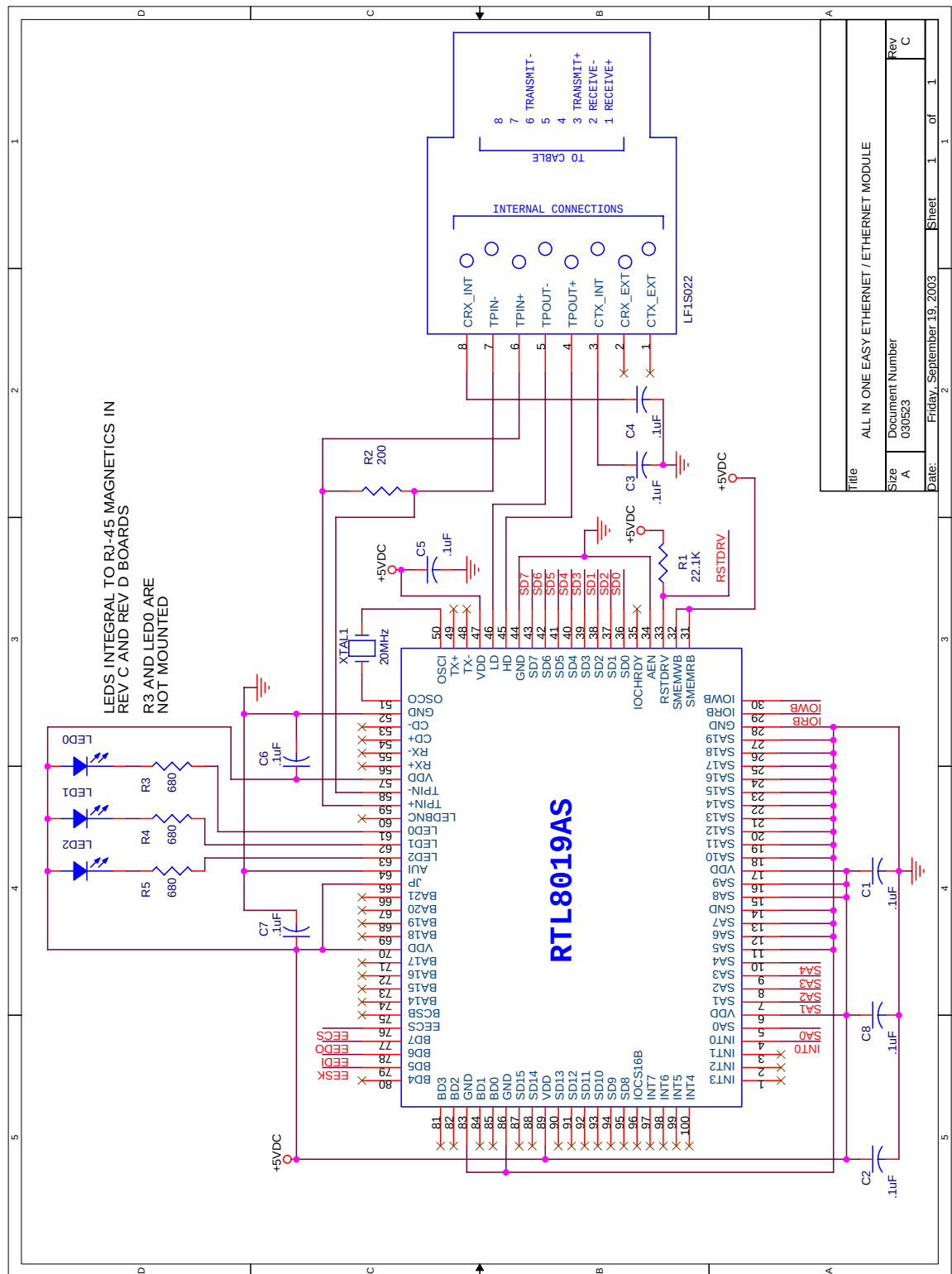
Figura D.3: Diagrama esquemático Easy Ethernet, página 2.
