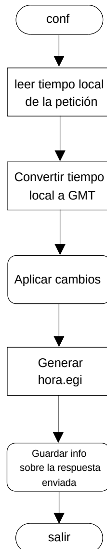
Figura 4.16: Diagrama de flujo del recurso ejecutable rtc.cgi
