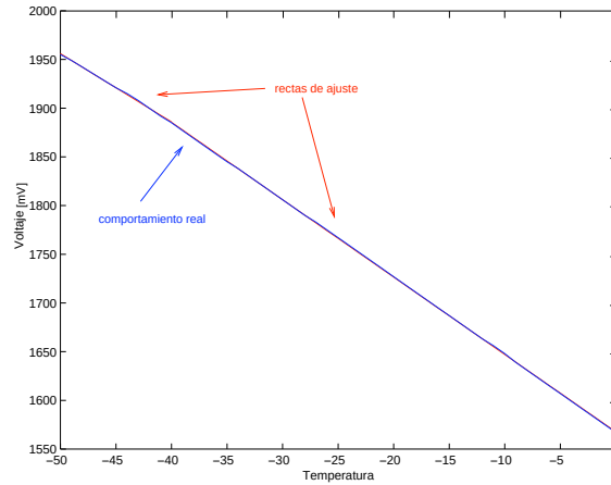
Figura 5.12: Ajuste mediante mínimos cuadrados, 5 rectas.
