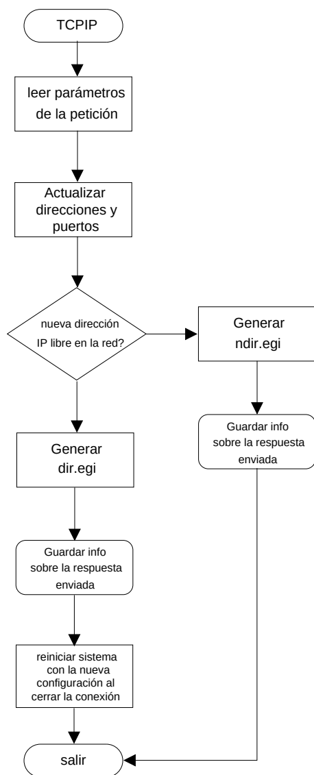
Figura 4.15: Diagrama de flujo del recurso ejecutable tcpip.cgi
