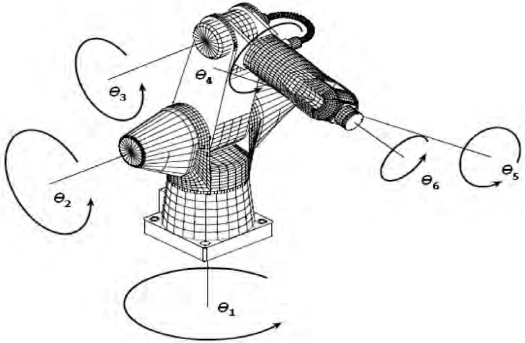
Figura 4.1: Robot manipulador CRS A465, indicando la localización de las juntas de rotación
