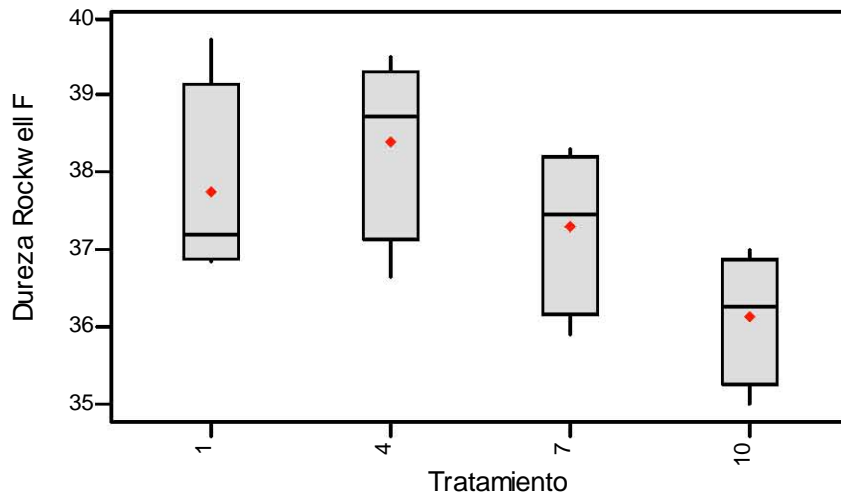
Fig. 3.23 Gráfico de caja del análisis de Dureza de las probetas de Mg AZ31 Con recubrimiento de pintura, con respecto al grupo de control que no fue expuesto a condiciones ambientales.
