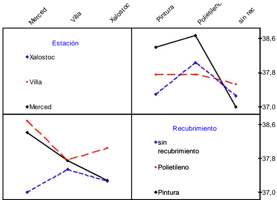
Fig. 3.20 Gráfico de interacción entre ambientes de exposición y recubrimientos de los especímenes de prueba, en donde el paralelismo demuestra que no existe correlación entre los ambientes de exposición y los recubrimientos, sin embargo existe un ligero cruce de líneas que, de acuerdo al análisis realizado es no significativo . T
