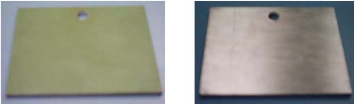
Fig. 2.14 la imagen muestra un espécimen de simple cara sin recubrimiento en el reverso y un recubrimiento de pintura en el anverso, de dimensiones 3.2 x 4.5 x 0,250 pulgadas aproximadamente.
