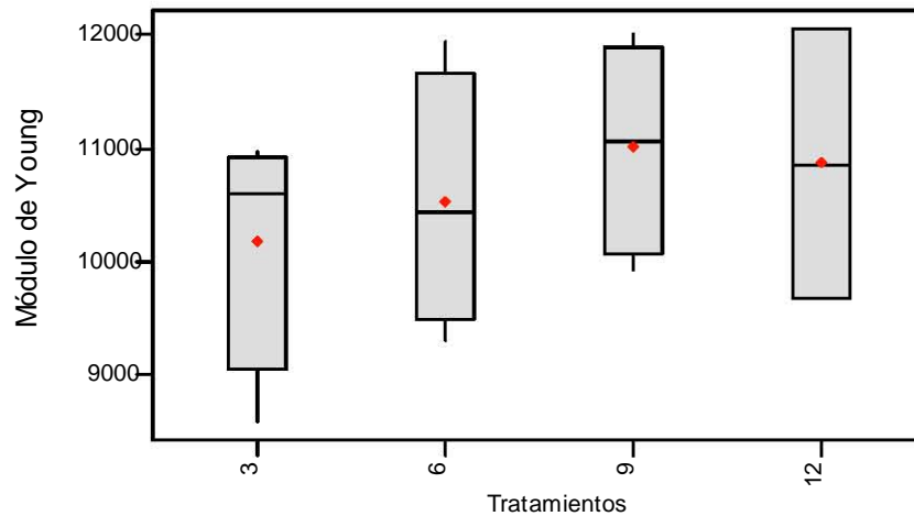
Fig. 3.18 Gráfico de caja del análisis del Módulo de Elasticidad de las probetas de Mg AZ31 sin recubrimiento, con respecto al grupo de control que no fue expuesto a condiciones ambientales.
