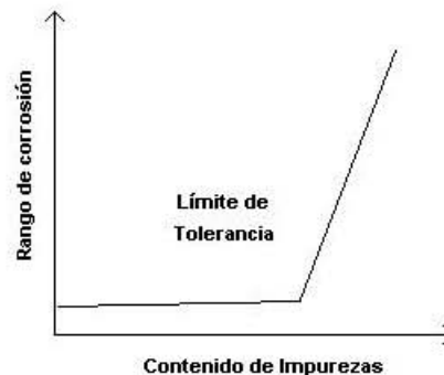
Fig. 1.9 Curva generalizada mostrando la influencia de los elementos X (Ni, Fe, Cu) en el rango de corrosión del magnesio.
