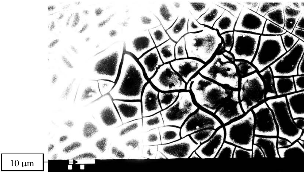
Fig. 3.31 Fotografía de la microscopía de barrido electrónico a 1000 aumentos, realizada a la muestra # 37, donde se aprecia claramente el ataque corrosivo en los límites de grano. La barra debajo de la imagen es de 10 micras de dimensión.
