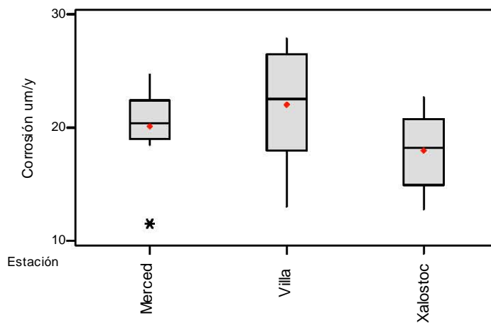
Figura 3.1 Gráfico de caja del análisis de la cantidad de corrosión del Mg AZ31 de acuerdo al sitio de exposición.
