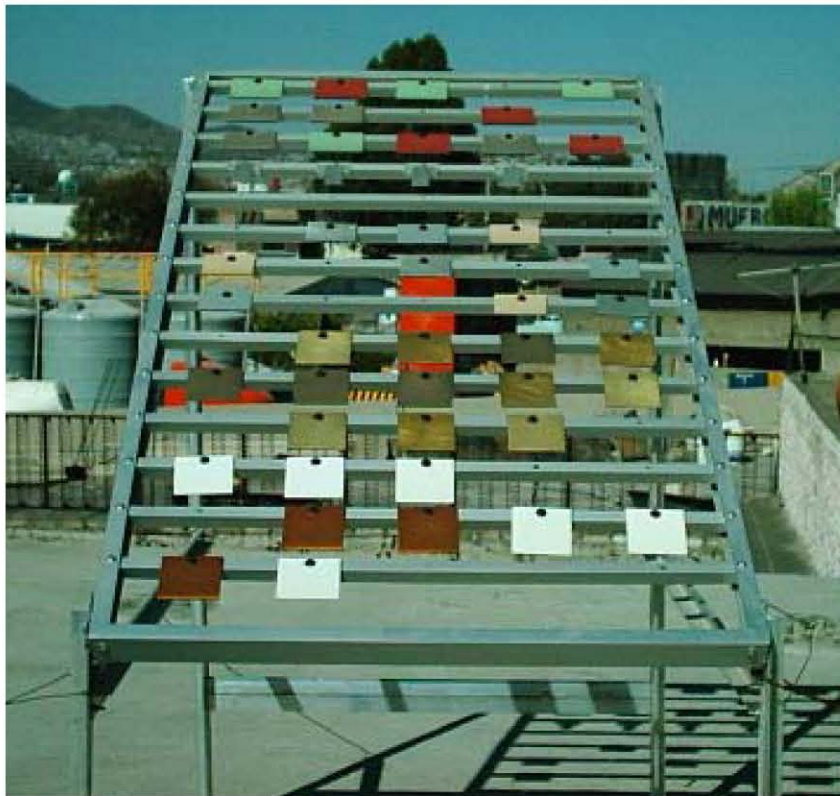
Fig. 2.22 Bastidor para pruebas de corrosión atmosférica montado en el ambiente industrial a los tres meses de exposición, en donde se aprecia claramente la colocación y tratamientos de las probetas en estudio.
