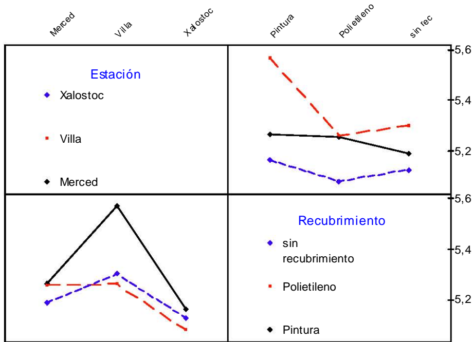
Fig. 3.6 Gráfico de interacción entre sitios de exposición y recubrimientos de las probetas, en donde el paralelismo demuestra que no existe correlación entre los sitios de exposición y los recubrimientos.
