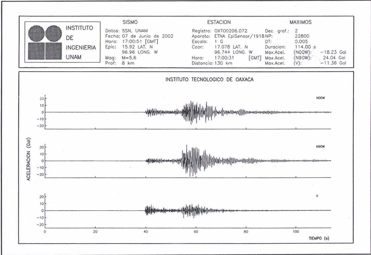
Figura 35. Acelerograma en formato ASCII estándar de aceleración (ASCIISTD)
