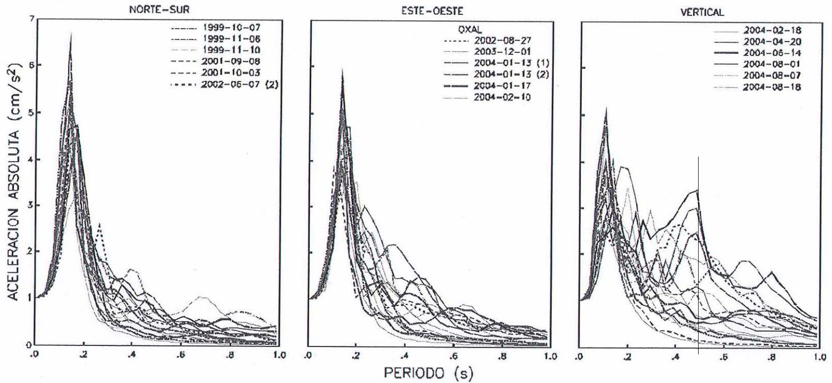
Figura 43. Espectros de Respuesta para los eventos registrados en la estación Oaxaca Alameda de León (OXAL)
