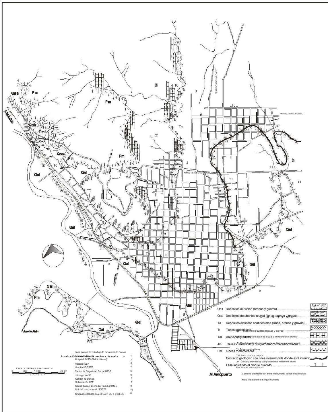
Figura 12. Estratigrafía y litología de la Ciudad de Oaxaca.
