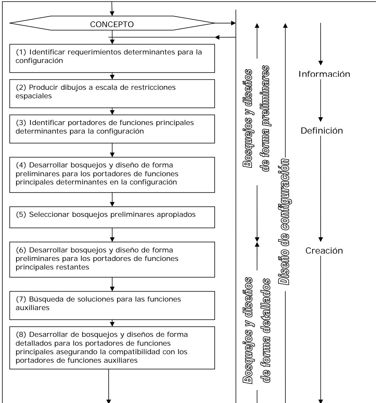
Figura 37-A. Diseño de configuración
