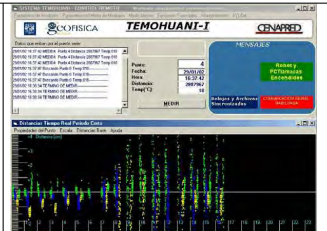
Figura 16. Pantalla de control y recepción de datos.
