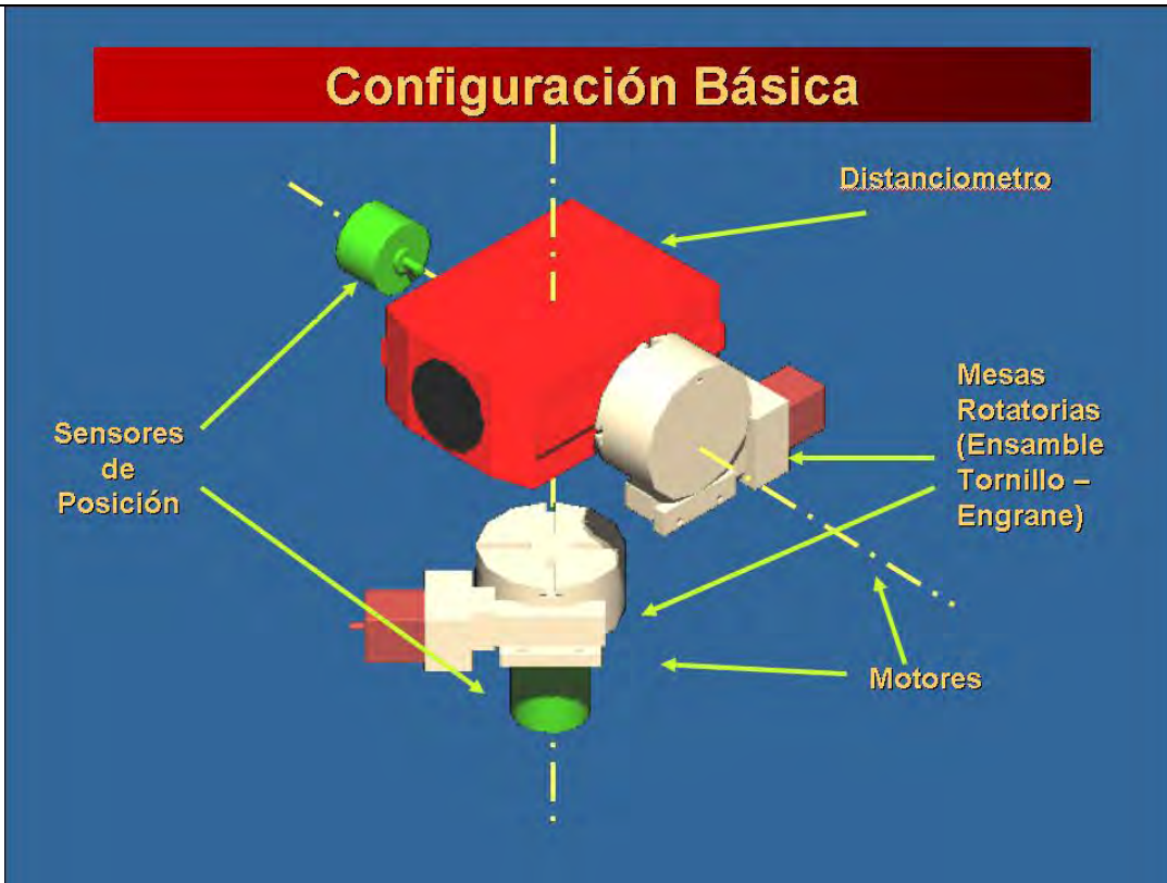
Figura 9, Distribución de componentes del sistema de movimiento.
