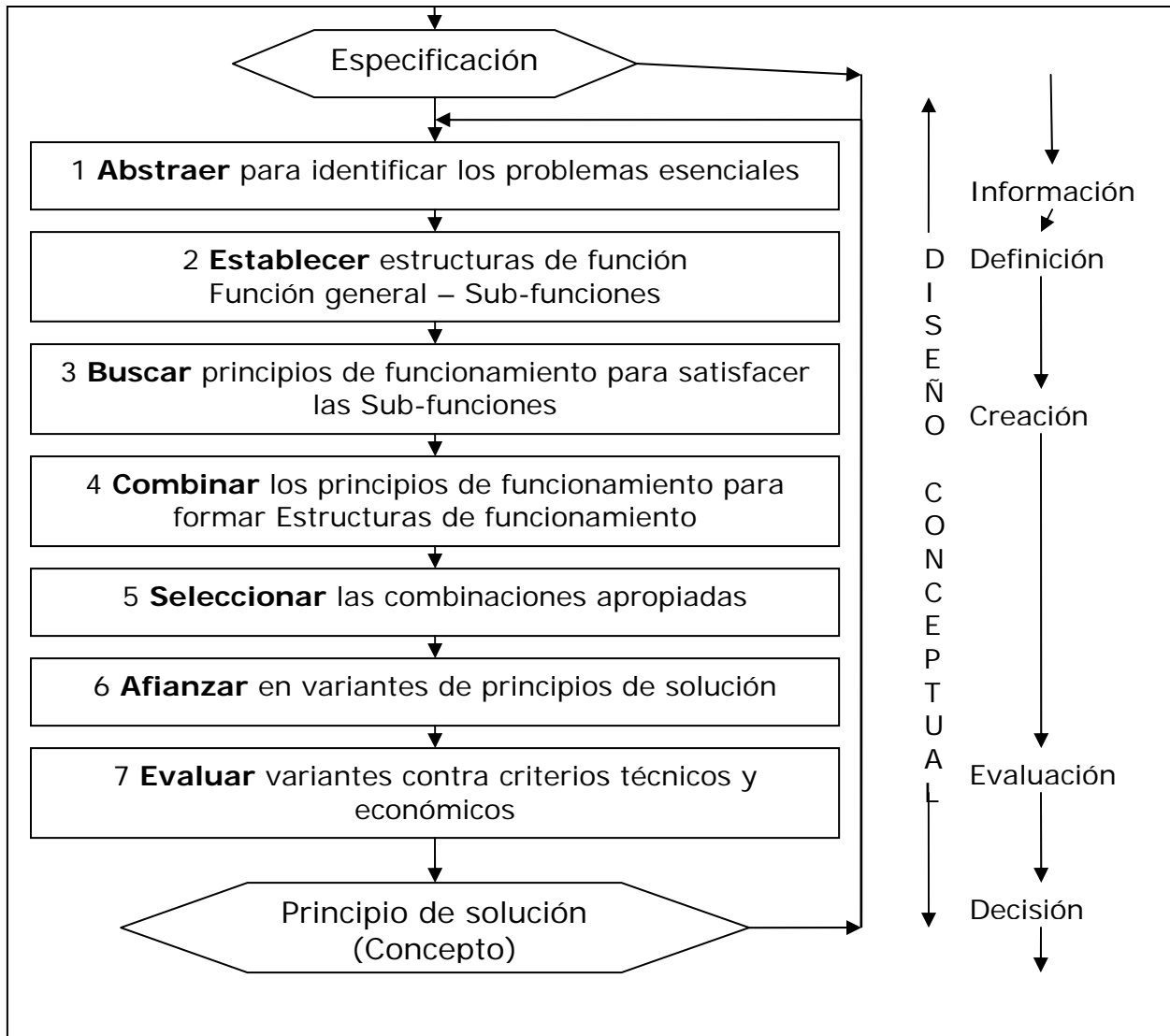
Figura 27. Diseño conceptual
