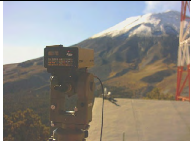
Imagen 8, EDM midiendo la distancia al prisma
