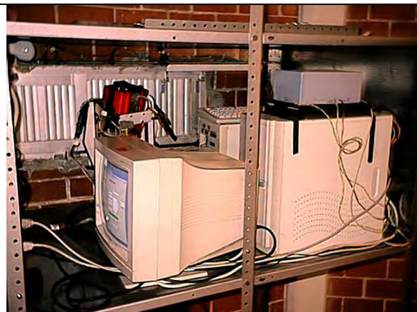
Imagen 12. Vista del sistema Temohuani I completo
