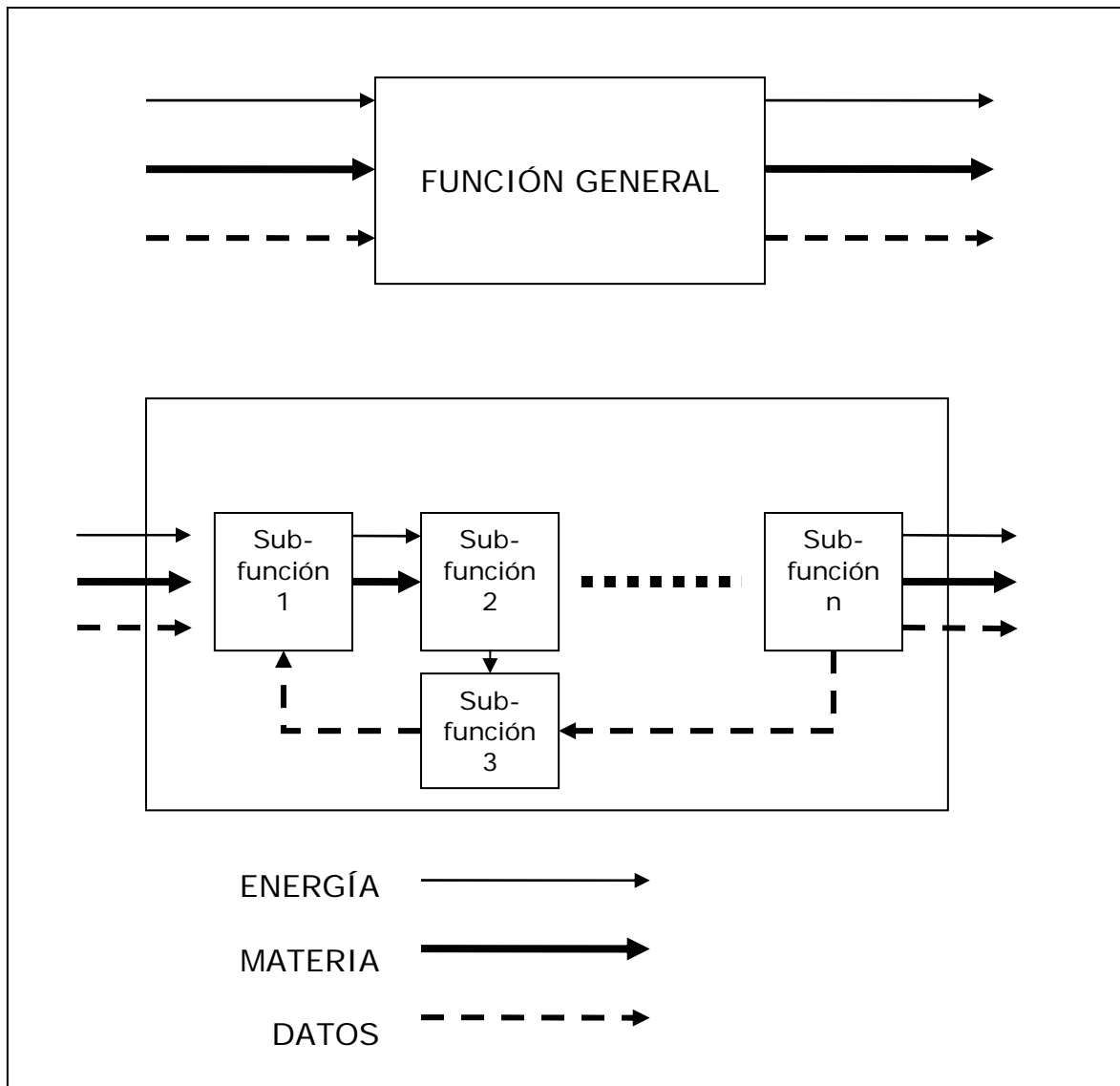
Figura 28. Estructura funcional
