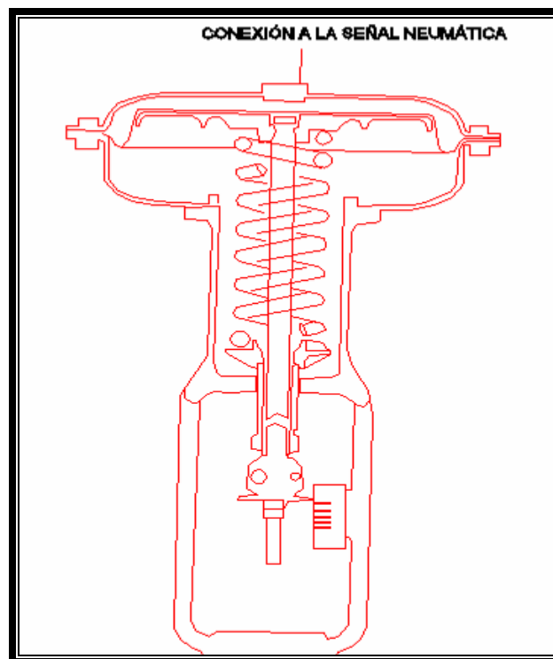
Figura 34.- Accionador de diafragma: abierto en falla, aire para cerrar. [18]
