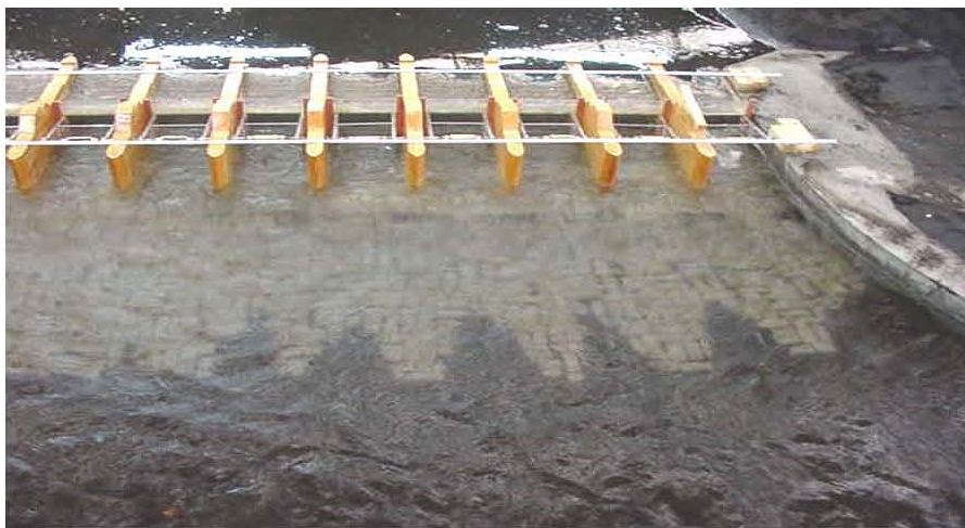
Figura 3.1.1 Condición del tapete después de la prueba, con NAME.
