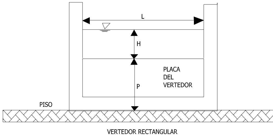
Figura 2.6.15 Vista frontal del Vertedor rectangular de cresta delgada, que abastece al modelo.
