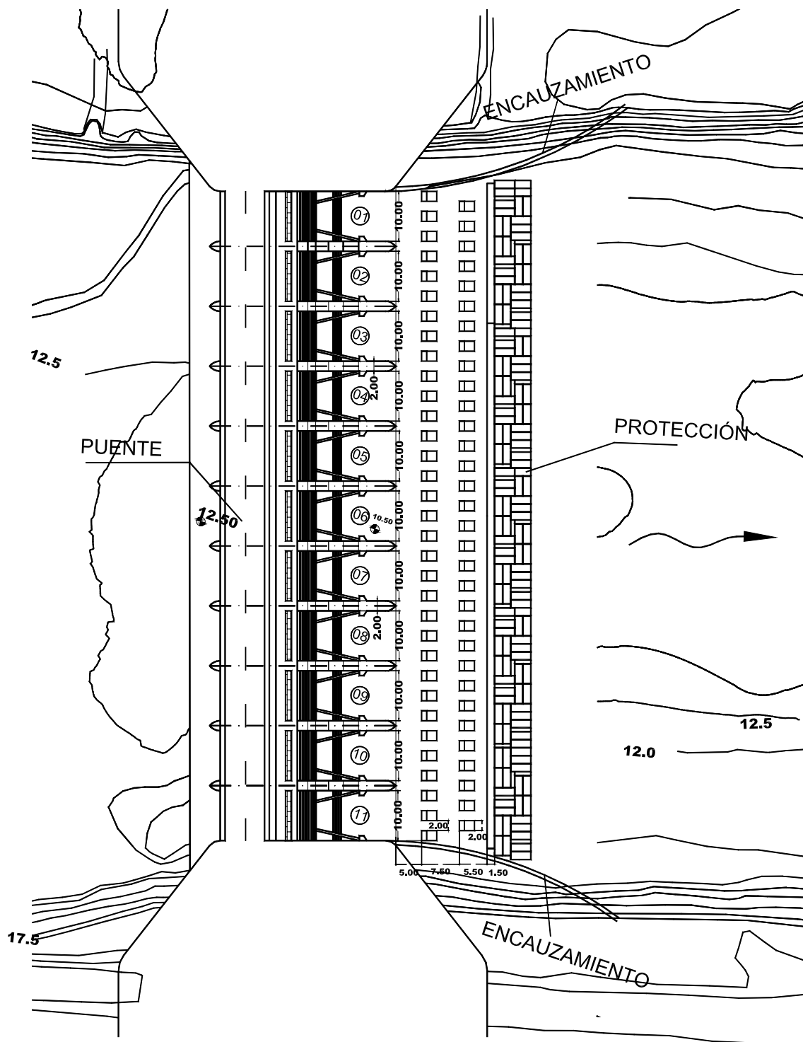
Fig. 3.4.3 Vista en planta de la estructura A3 modificada.
