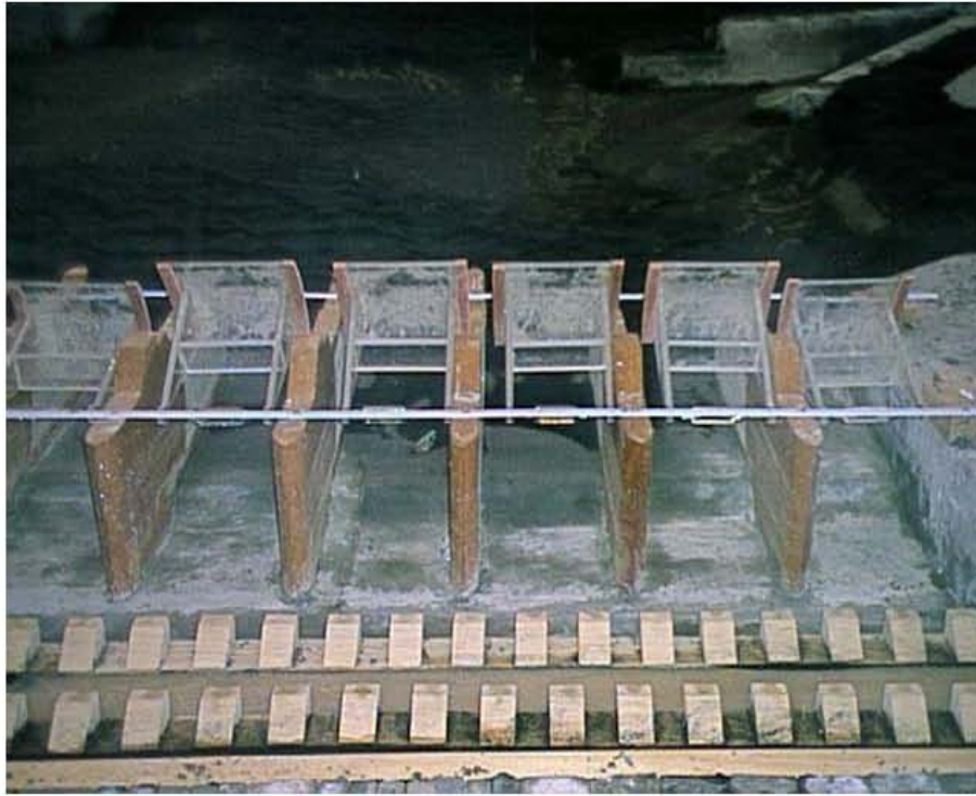
Figura 3.4.2 Detalle del tanque amortiguador con doble hilera de dientes.
