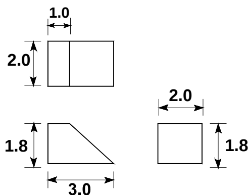
Fig. 3.4.1 Dimensiones de los dientes en metros, de la estructura terminal en prototipo.
