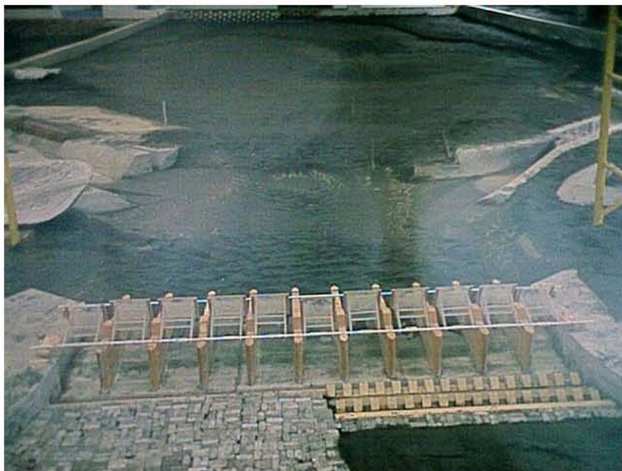
Fig. 3.4.5 Modificaciones hechas a la alternativa A3 en el modelo físico.
