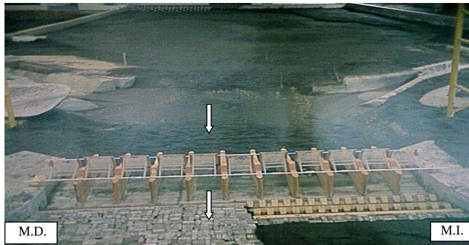
Figura 2.6.8 Estructura disipadora de energía en la estructura de control.
