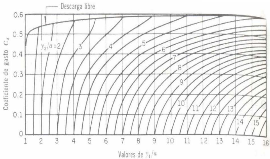
Figura 4.2.1 Para obtener el coeficiente de descarga de una compuerta plana (Sotelo A.G. 2002).
