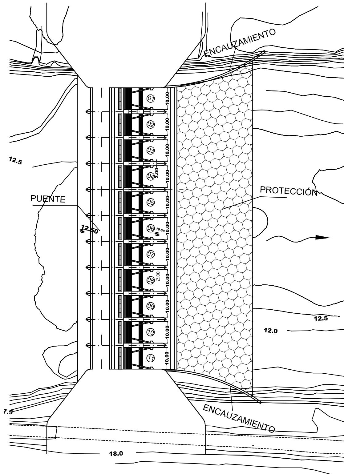
Fig.3.1.3 Vista en planta de la estructura de la alternativa A3.
