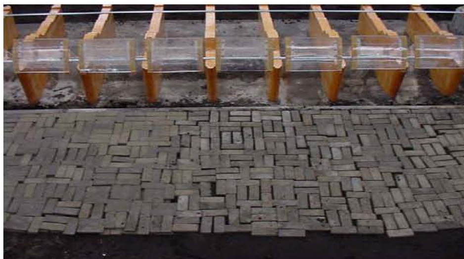
Fig. 3.4.6 Estructura disipadora de energía, simulada por sacos de concreto colocados en una capa.
