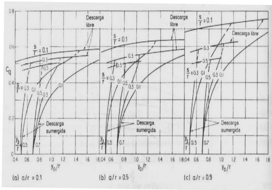
Figura 4.2.2 Para obtener el coeficiente de descarga ( C_d = C_q en la figura) para compuertas radiales (Sotelo A.G. 2002).
