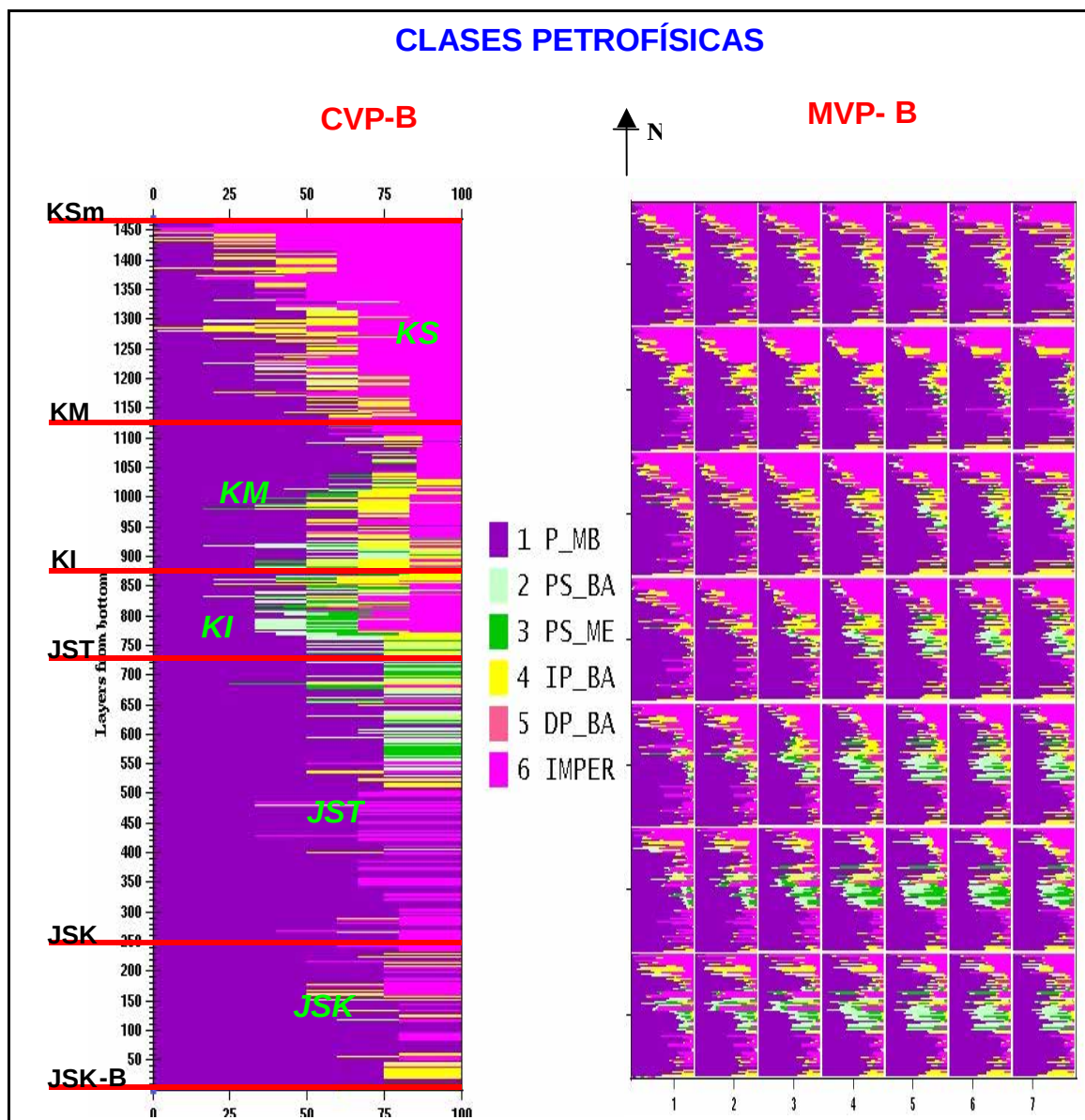
Figura 5.10. CVP y MVP de las clases petrofísicas del caso B.
