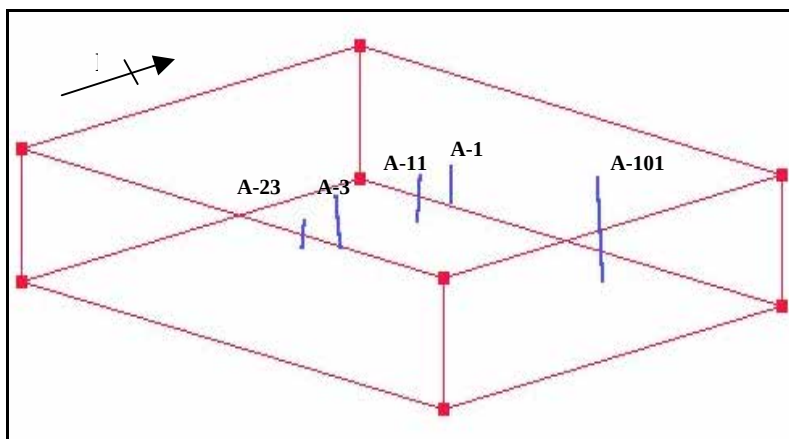
Figura 5.3. Cubo estocástico para el caso A.
