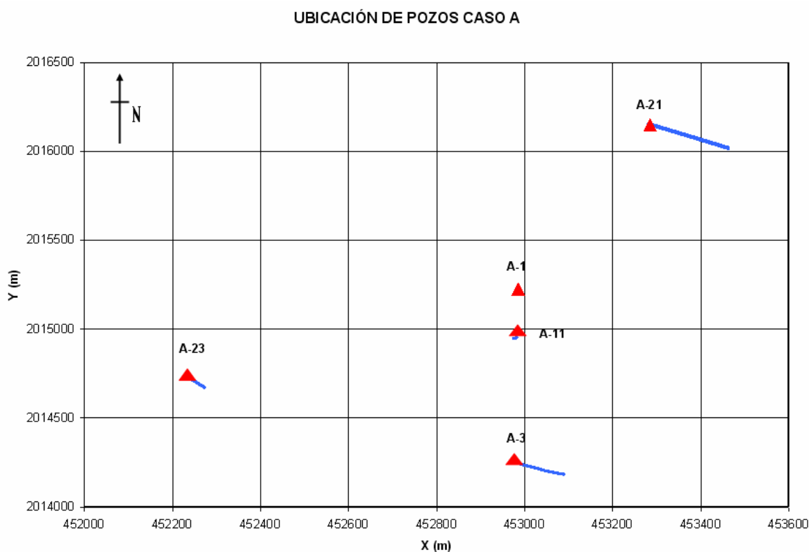
Figura 3.4. Ubicación de los pozos que constituyen al caso A.
