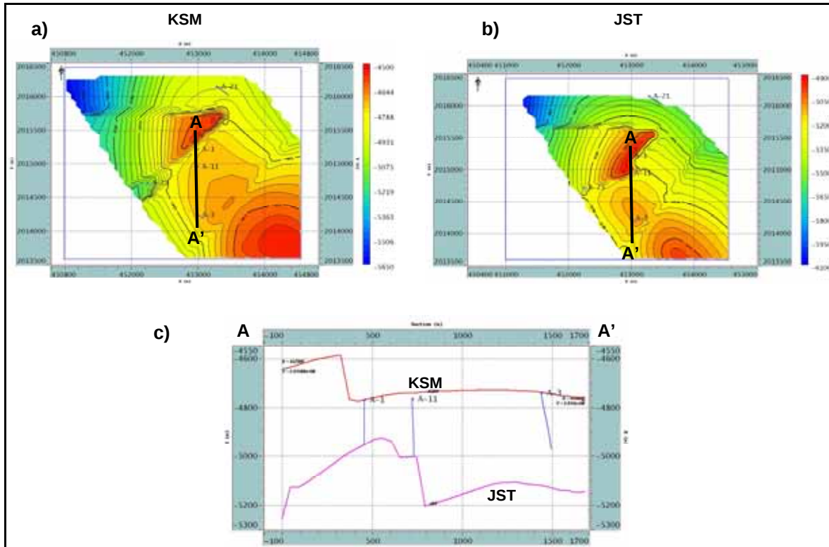
Figura 5.2. Configuraciones estructurales utilizadas para el análisis geoestadístico para el campo A. El inciso a) muestra la configuración estructural para el Cretácico Superior Medio (KSM), b) la configuración para el Jurásico Superior Tithoniano (JST), y c) unidad JST-KSM que se forma con la cima KSM y con la base JST.
