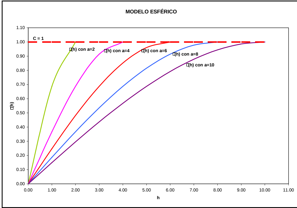
Figura 2.8. Gráfica del modelo esférico, con a = 2, 4, 6, 8 y 10 .
