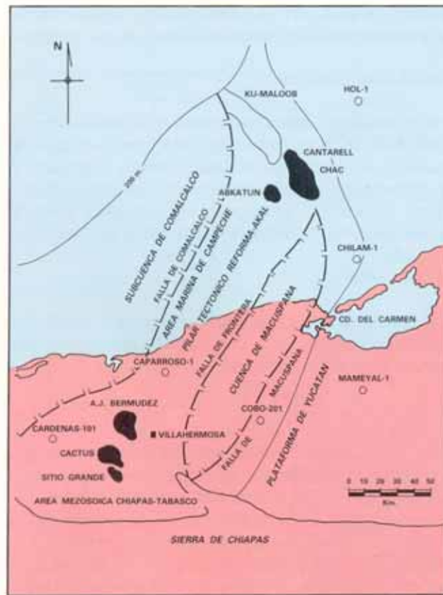
Figura 3.3. Límites estructurales y fisiográficos del Área Chiapas Tabasco. (Schlumberger, 1984).
