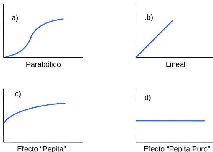
Figura 2.7. Formas teóricas de un variograma (modificado de Berlanga Gutiérrez y Obregón Andría, 1980).
