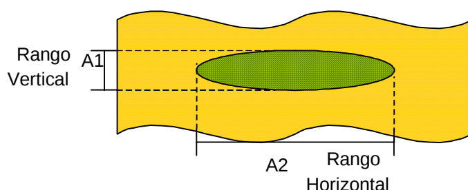
Figura 2.5. Lente mineralizado (modificado de Berlanga Gutiérrez y Obregón Andría, 1980).
