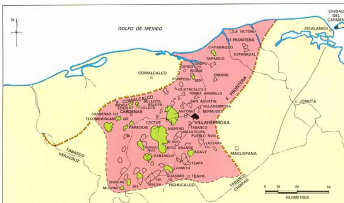
Figura 3.2. Ubicación del Área Chiapas Tabasco en la que se localizan los casos A, B y C. (Schlumberger, 1984).
