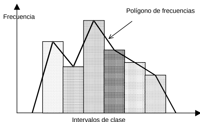
Figura 2.1. Histograma. Cada barra representa un grupo de valores con su determinada frecuencia dentro de una muestra.
