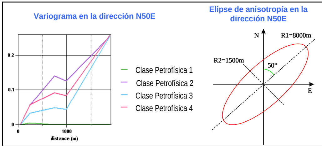
Figura 5.5. Dirección de mínima variabilidad y elipse de anisotropía.
