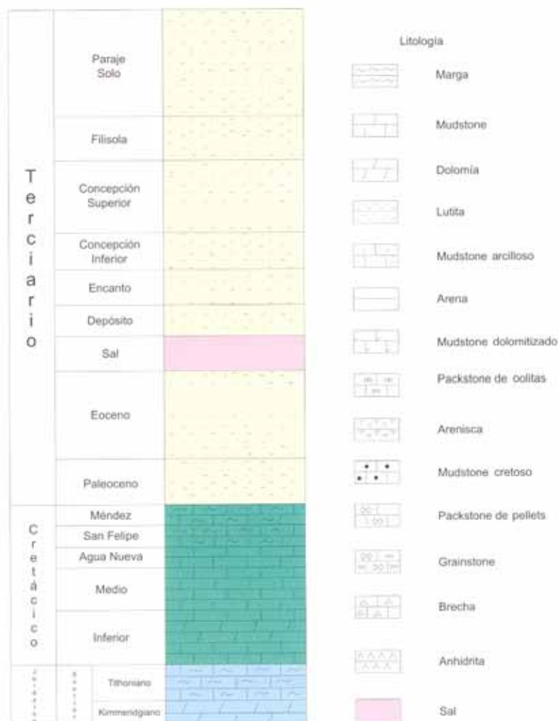
Figura 3.9. Columna geológica tipo del campo que pertenece al caso B. (PEMEX Exploración y Producción, 1999).
