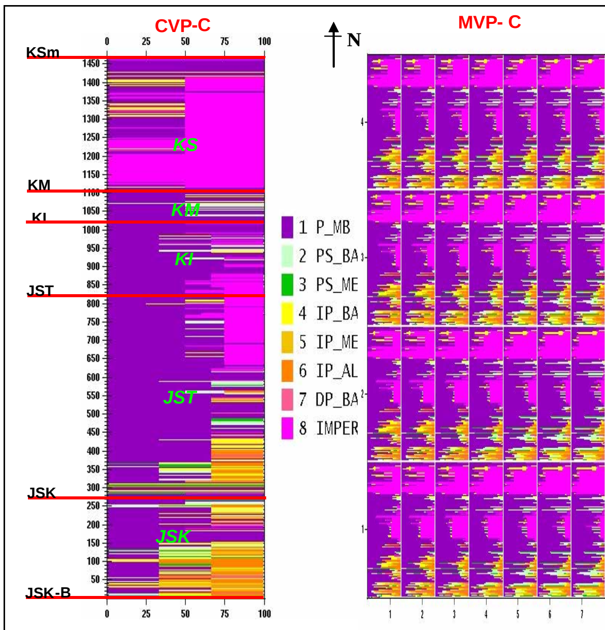
Figura 5.11. CVP y MVP de las clases petrofísicas del caso C.
