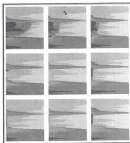
Figura 2.15. Matriz vertical de proporción. En este tipo de curvas, se dice que tienen un sentido tridimensional, ya que en cada CVP se tiene la proporción de las litofacies con respecto a la profundidad (z), y por otro lado, el conjunto de las CVP da la proporción lateral (x,y) de las litofacies. (Armstrong, Galli, Le Loc'h, Geffroy y Eschard, 2003).
