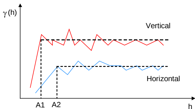
Figura 2.6. Variogramas en dirección vertical y horizontal (modificado de Berlanga Gutiérrez y Obregón Andría, 1980).
