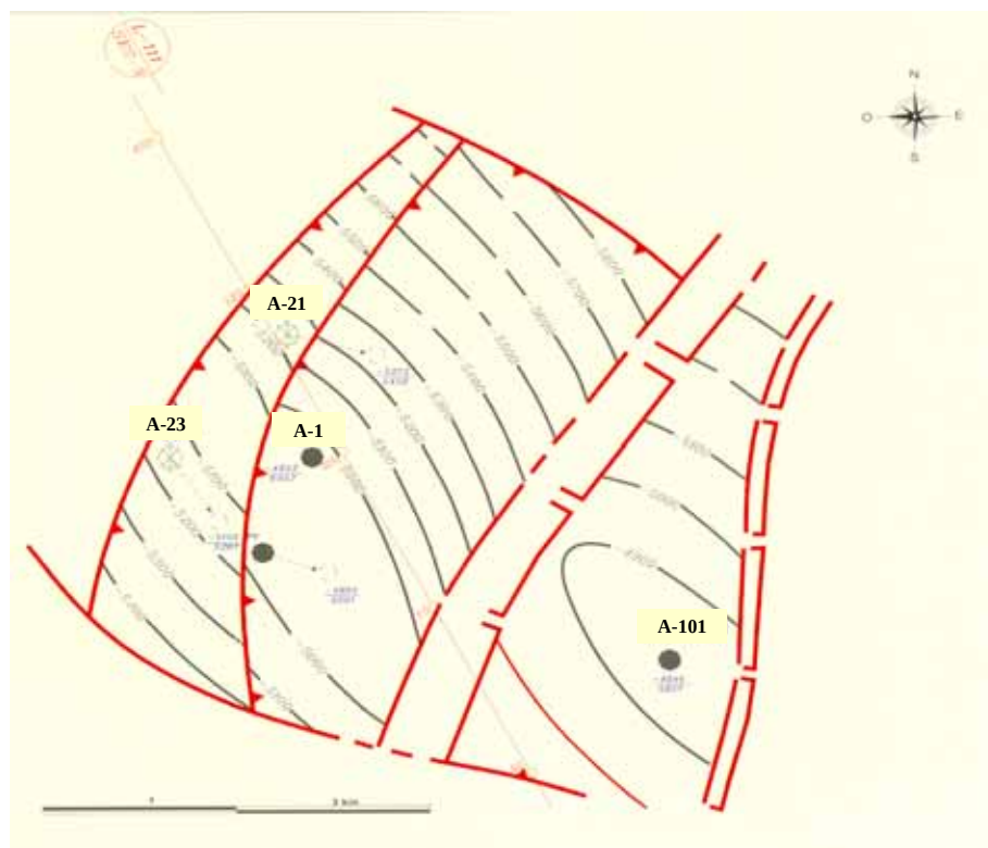
Figura 3.5. Anticlinal orientado de noreste a sureste en donde se encuentra el campo del caso A. (PEMEX Exploración y Producción, 1999).
