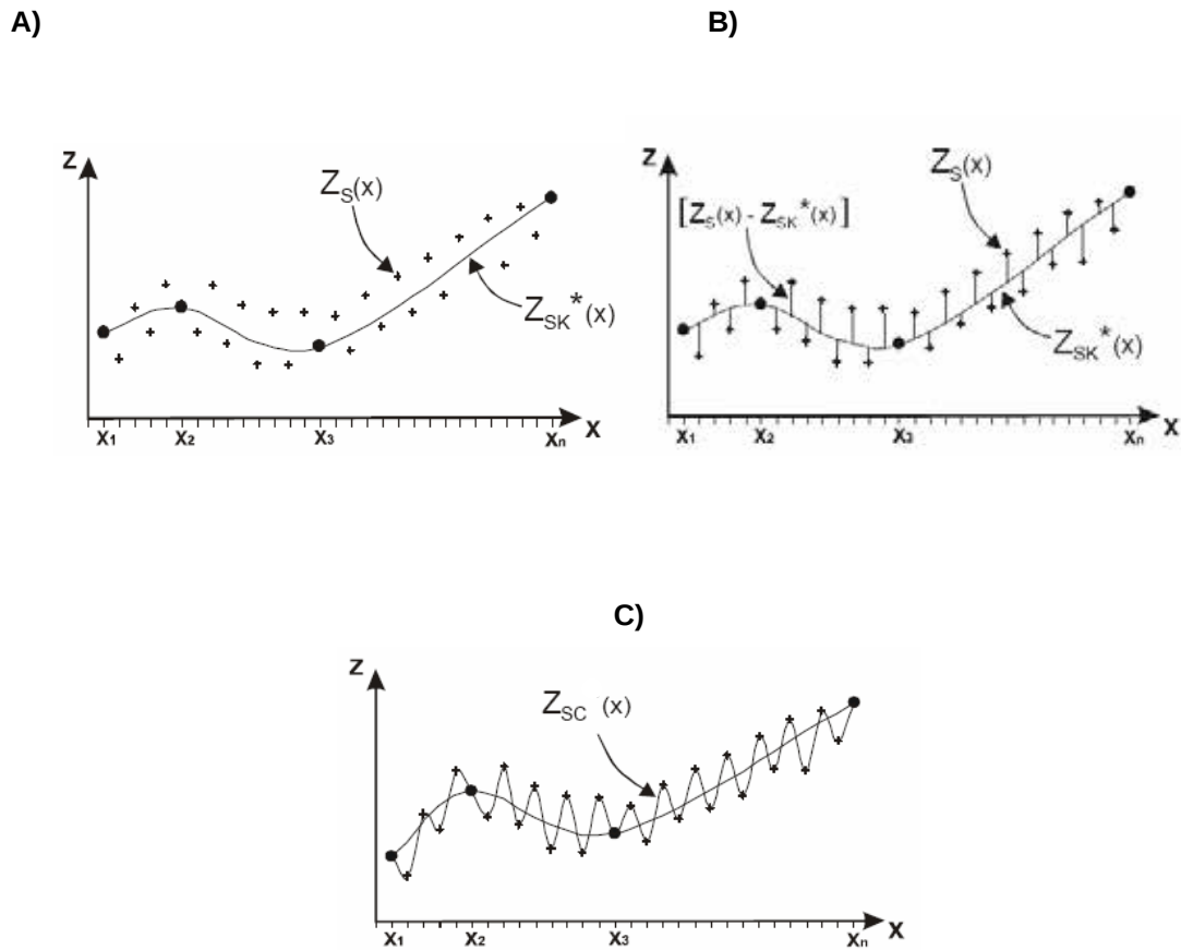
Figura 2.12. A) La línea continua representa la estimación Z_{SK}^*(x) de los valores simulados Z_S(x) . B) Se muestra la diferencia [Z_S(x) - Z_{SK}^*(x)] . C) La línea que une a los datos experimentales con las cruces es la simulación condicional Z_{SC}(x) resultante. (Cuador-Gil y Quintero-Silverio, 2001)
