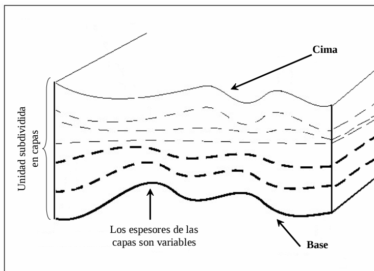
Figura 5.4. Subdivisión de una unidad litoestratigráfica de manera proporcional a cada punto.
