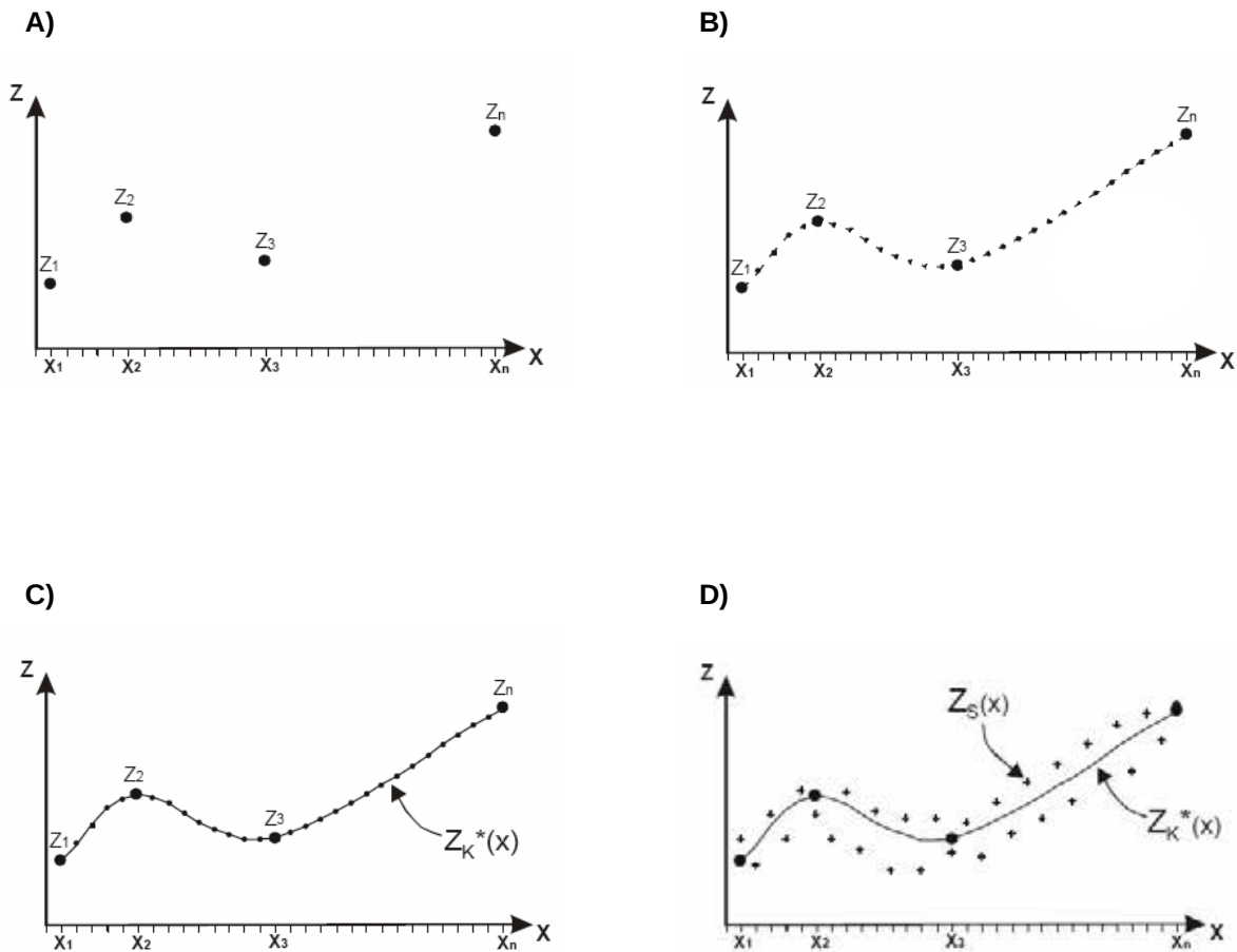
Figura 2.11. A) Distribución espacial de los datos experimentales z(x_i) a simular, los datos pueden estar dispuestos de forma regular, irregular o ambas a la vez . B) Localizaciones propuestas dentro del área en estudio en las que se simulará el fenómeno. C) Se observa los valores estimados por kriging Z_k^*(x) a partir de los datos experimentales. D) Los puntos en forma de cruz representan los valores simulados no condicionados Z_s(x) a partir de las características de variabilidad ( c(h) ó \gamma(h) ). (Cuador-Gil y Quintero-Silverio, 2001)
