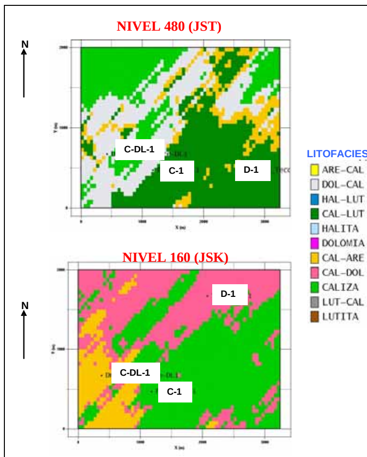
Figura 5.26. Niveles 480 y 160 de la unidad JSKBASE-KSM. (Resultados de la simulación gaussiana truncada sobre las litofacies en la dirección N50E).
