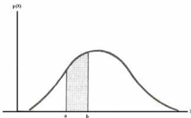
Figura 2.2. Distribución de probabilidad continua. El área sombreada representa la probabilidad de que x se encuentre entre a y b . (Spiegel, 1991)
