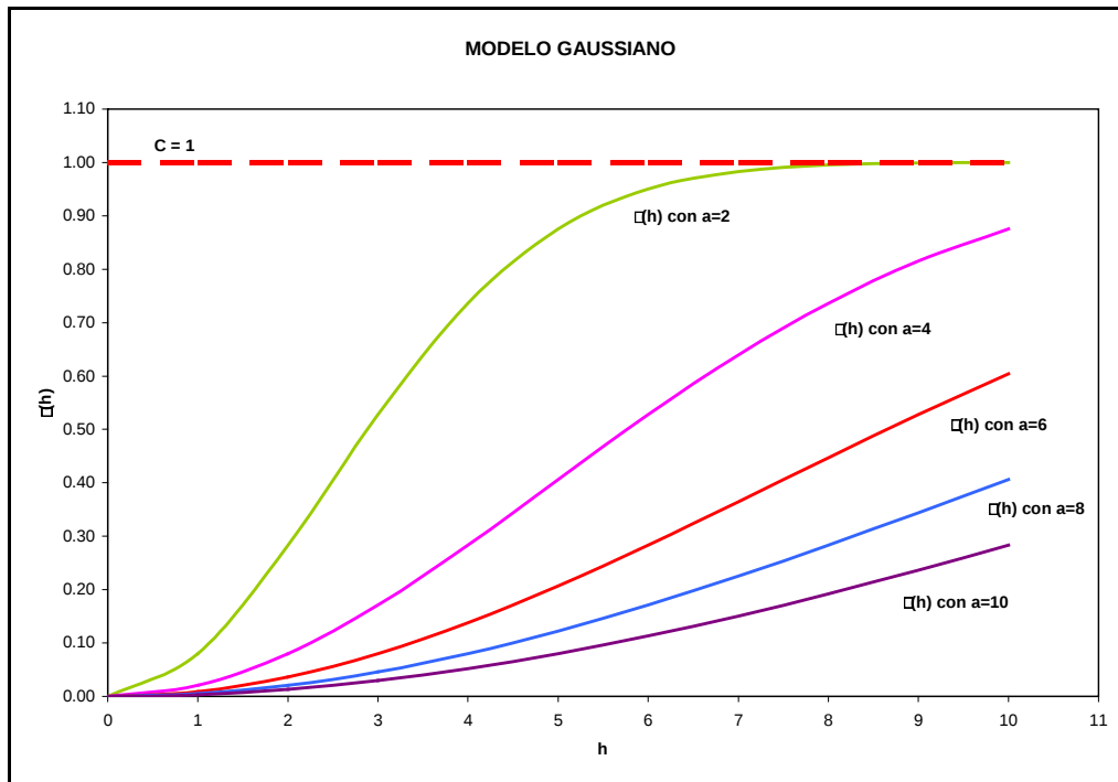
Figura 2.10. Gráfica del modelo gaussiano, con a = 2, 4, 6, 8 y 10 .
