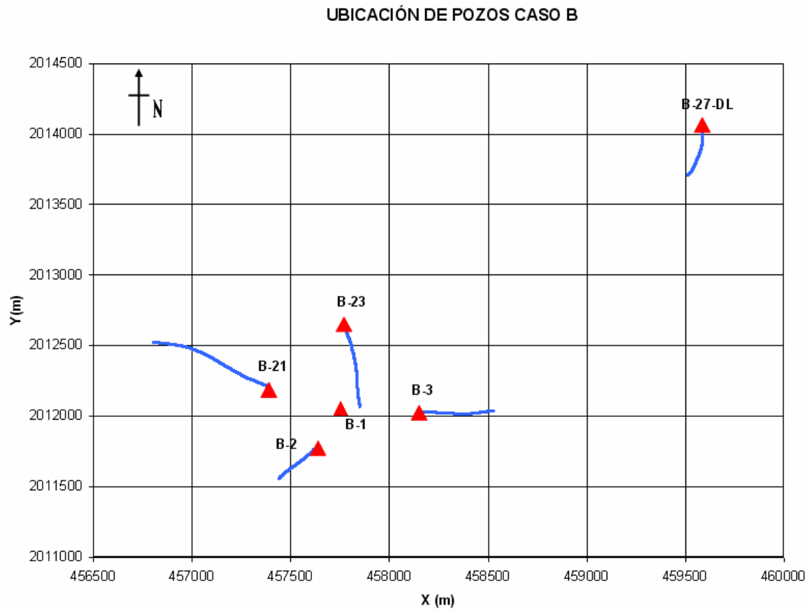
Figura 3.7. Ubicación de los pozos que conforman al campo del caso B
