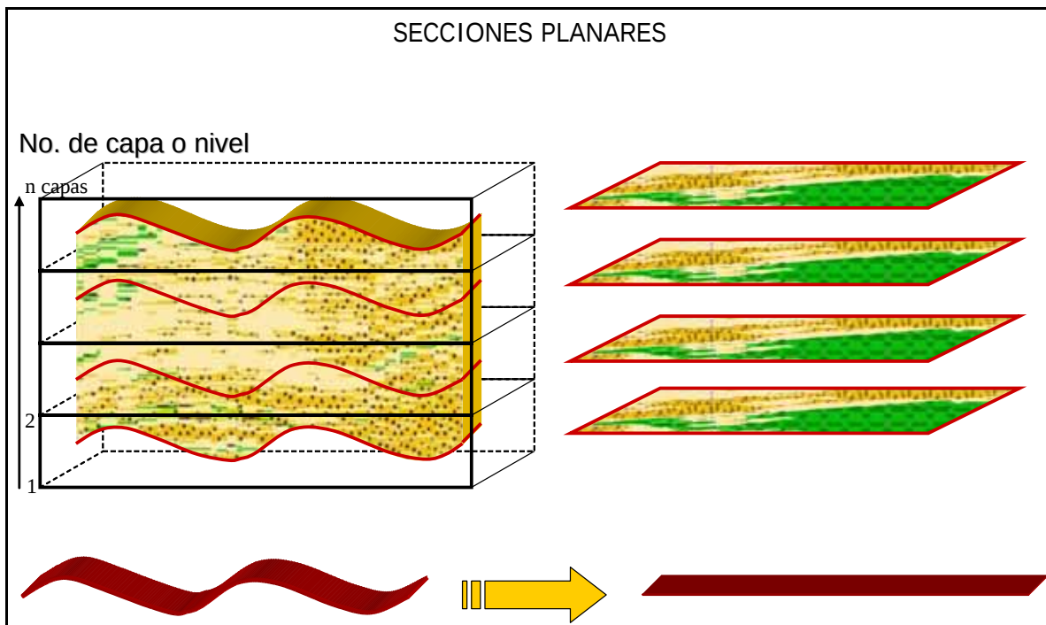
Figura 5.12. Se observa como se obtienen los mapas de los niveles que contienen la distribución de las facies, estos mapas siguen la morfología de la unidad.
