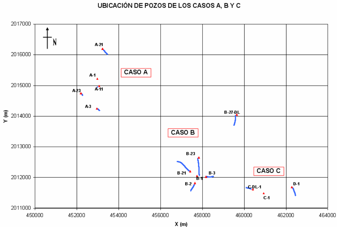
Figura 3.1. Muestra la ubicación de los casos A, B y C a los que se les aplico la simulación gaussiana truncada para obtener la distribución de litofacies, clases petrofísicas y de la relación Phisec * So.
