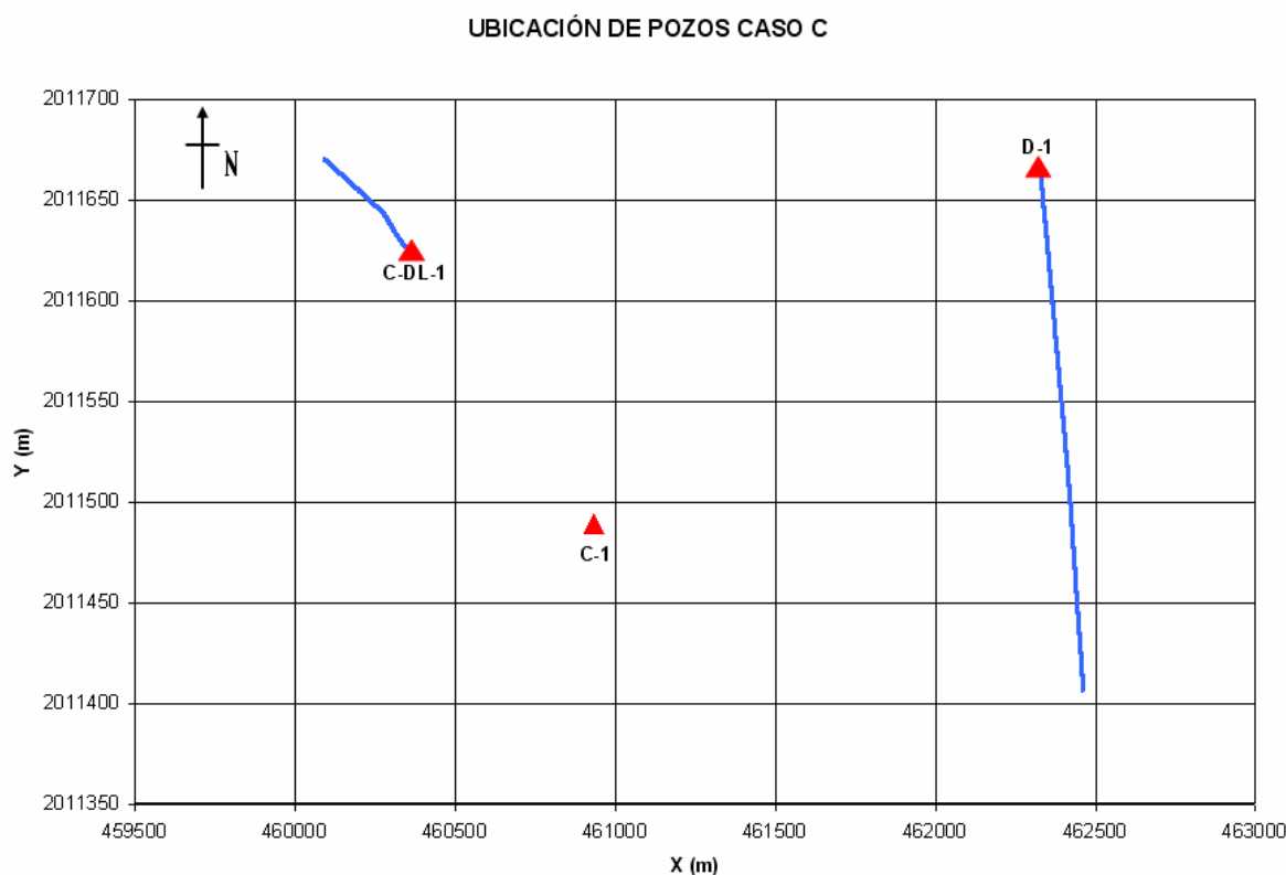
Figura 3.10. Distribución y ubicación de los pozos del campo del caso C.
