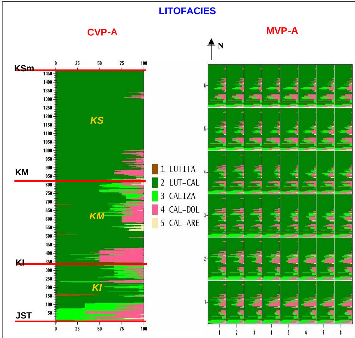
Figura 5.6. CVP y MVP de litofacies para el caso A.
