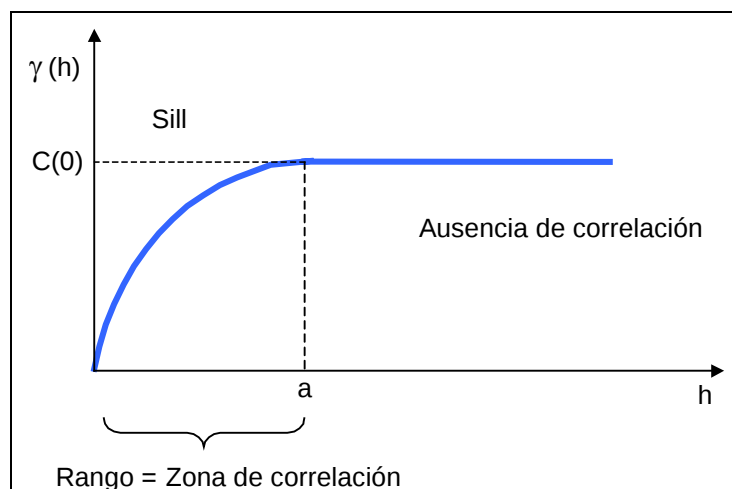
Figura 2.4. Variograma experimental.
