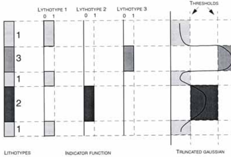
Figura 2.16. Se muestran las funciones indicadoras de las facies presentes en el pozo y las tendencias gaussianas generadas.
