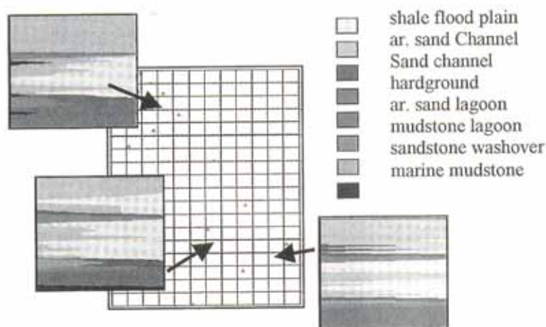
Figura 2.14. Malla regular en la que se estima mediante kriging las litofacies de las CVP por cada grupo de pozos (Armstrong, Galli, Le Loc'h, Geffroy y Eschard, 2003).
