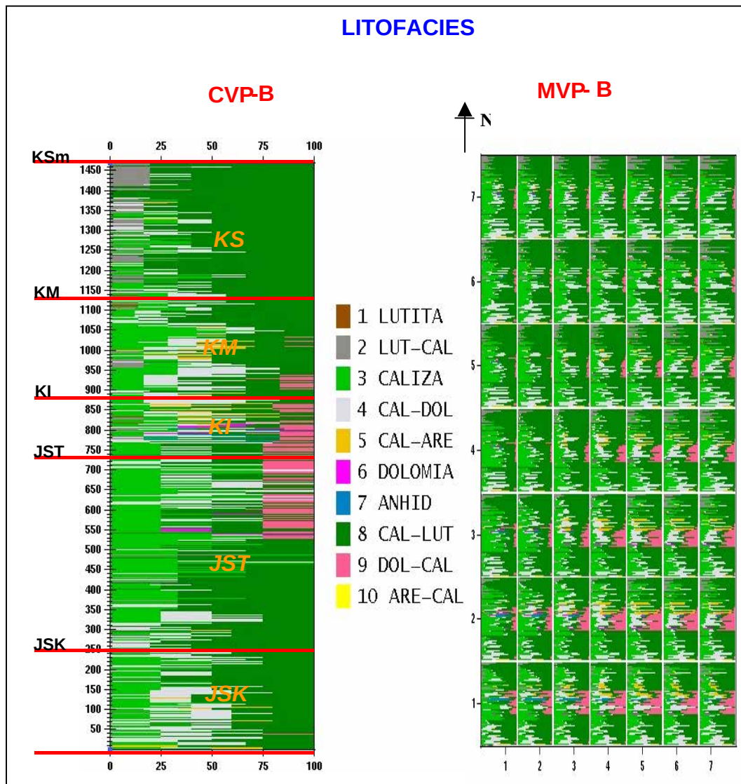
Figura 5.7. CVP y MVP de litofacies para el caso B.
