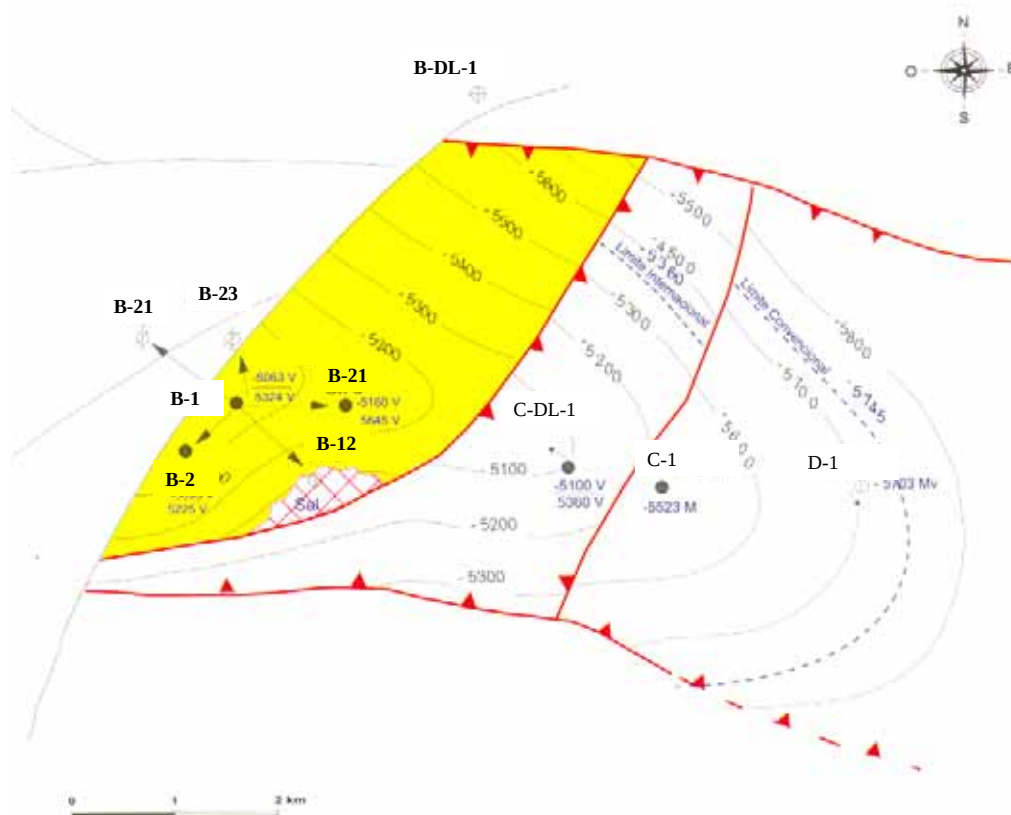
Figura 3.8. La estructura del caso B es un anticlinal semidómico orientado de noroeste a sureste. (PEMEX Exploración y Producción, 1999).
