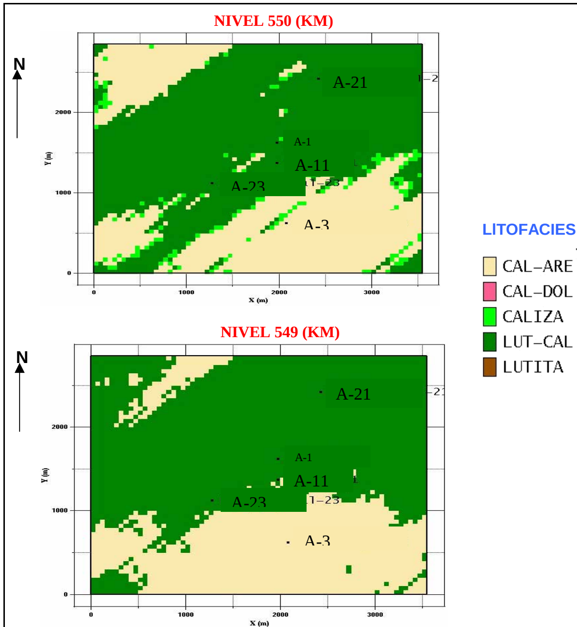
Figura 5.13. Niveles 550 (KM) y 549 (KM) de la unidad JST-KSM. Resultado de la simulación gaussiana truncada aplicando una dirección preferencial N 50° E, la cual es coincidente con la paleolínea del Golfo de México.
