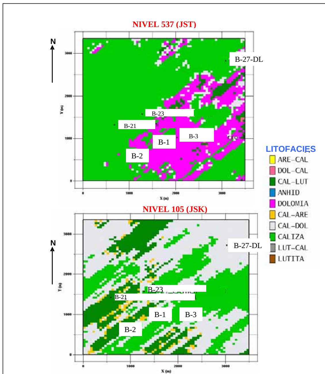
Figura 5.19. Niveles 537 (JST) y 105 (JSK) de la unidad JSKBASE-KSm. (Resultados de la simulación estocástica sobre las litofacies en la dirección N 50^{\circ} E ).
