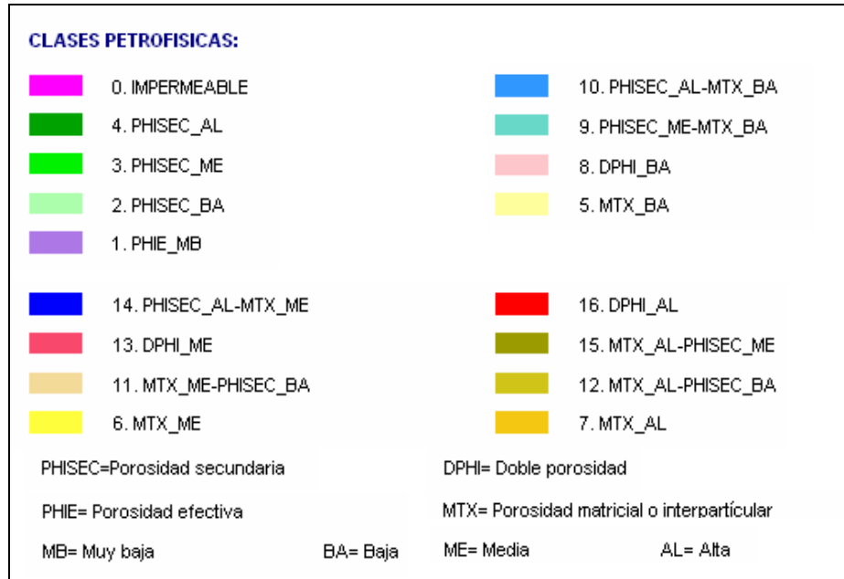
Figura 4.5. Clases petrofísicas generales. (IMP, 2004 a)
