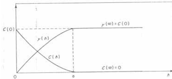
Figura 2.3. Covarianza y variograma. La covarianza c(h) decrece cuando el variograma \gamma(h) aumenta. El punto donde \gamma(h) alcanza su “estabilización” es llamado meseta o sill dentro de la distancia llamada rango ( a ). (Journel y Huijbregts, 1978).
