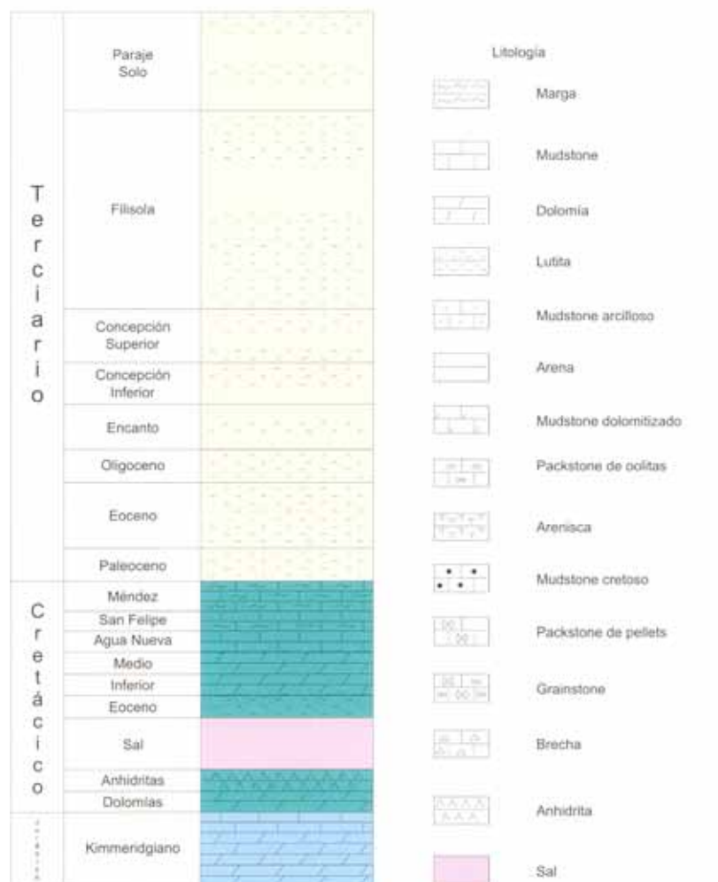
Figura 3.6. Columna Geológica tipo del caso A. (PEMEX Exploración y Producción, 1999).
