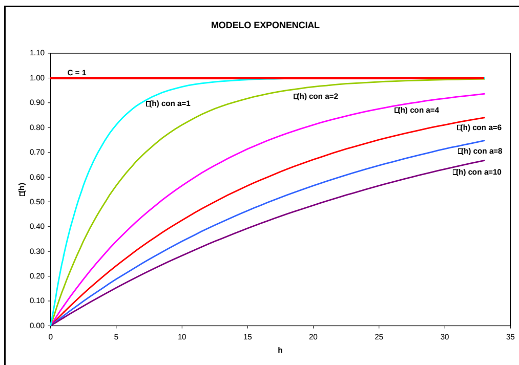
Figura 2.9. Gráfica del modelo exponencial, con a = 2, 4, 6, 8 y 10 .
