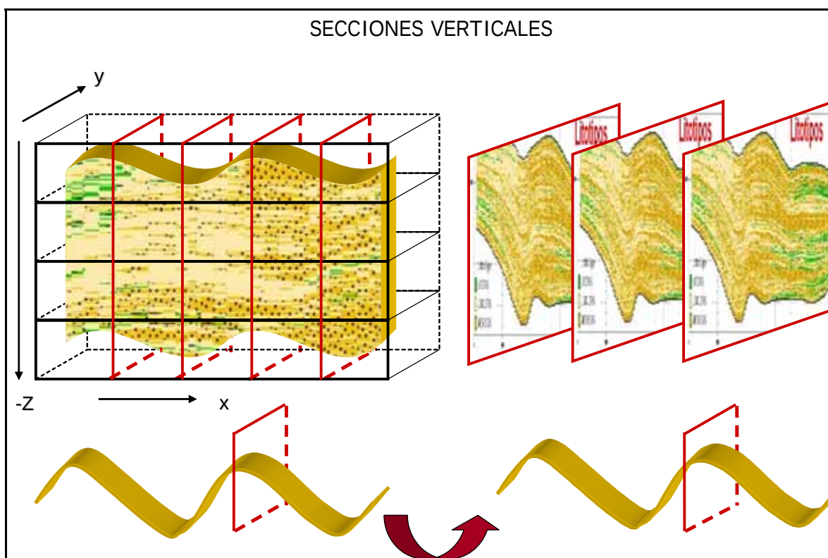
Figura 5.14. Forma de obtener las secciones verticales de la unidad estratigráfica.
