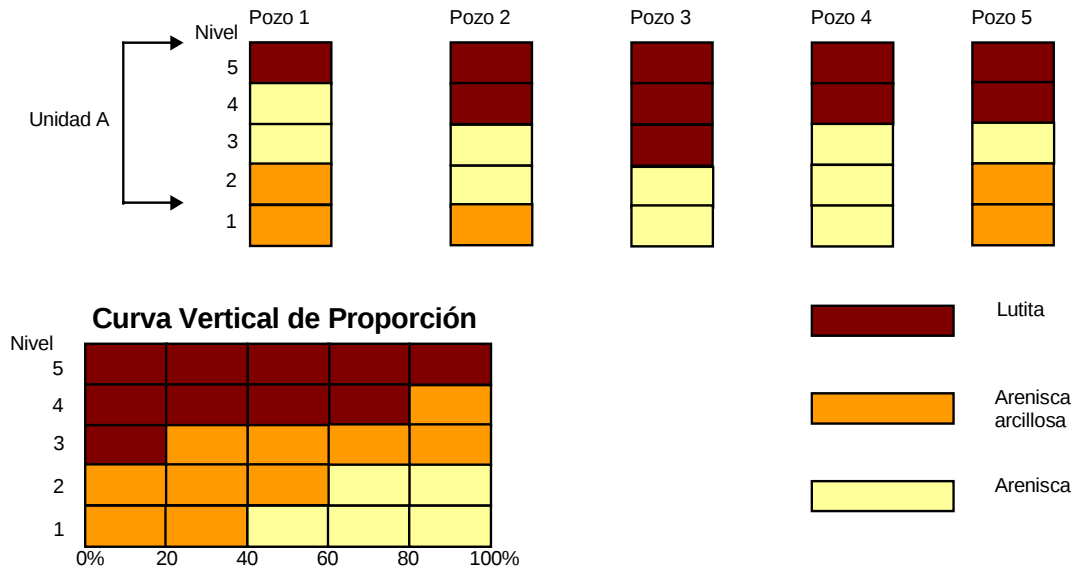
Figura 2.13. Generación de una curva vertical de proporción (CVP).
