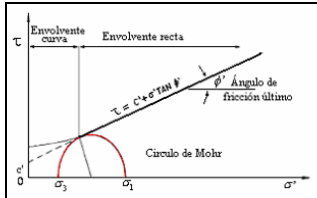
Figura II.2.5. Envolvente de falla o ley de resistencia Mohr-Coulomb
