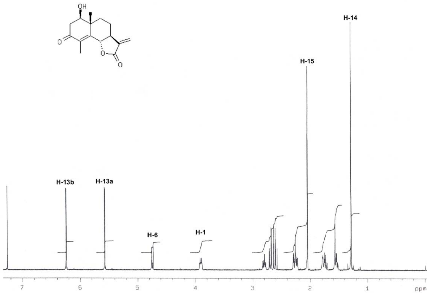
Espectro 10. Espectro de \text{RMN}^1\text{H} (500 MHz, \text{CDCl}_3 , TMS) de la Armexifolina.
