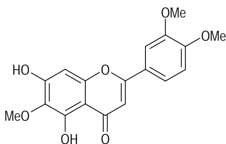
Figura 38. Eupatilina.
