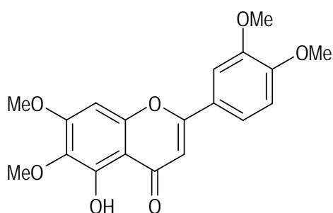
Figura 39. 5-hidroxi-3',4',6,7-tetrametoxiflavona.
