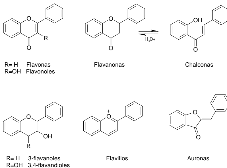
Figura 8. Diferentes grupos de flavonoides 18 .
