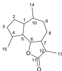
Figura 30. Esqueleto base del guayano.
