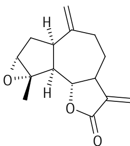
Figura 32. Estafiatina.
