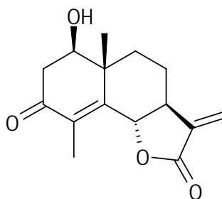
Figura 24. Arnefolina.
