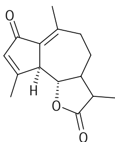
Figura 26. Achillina.
