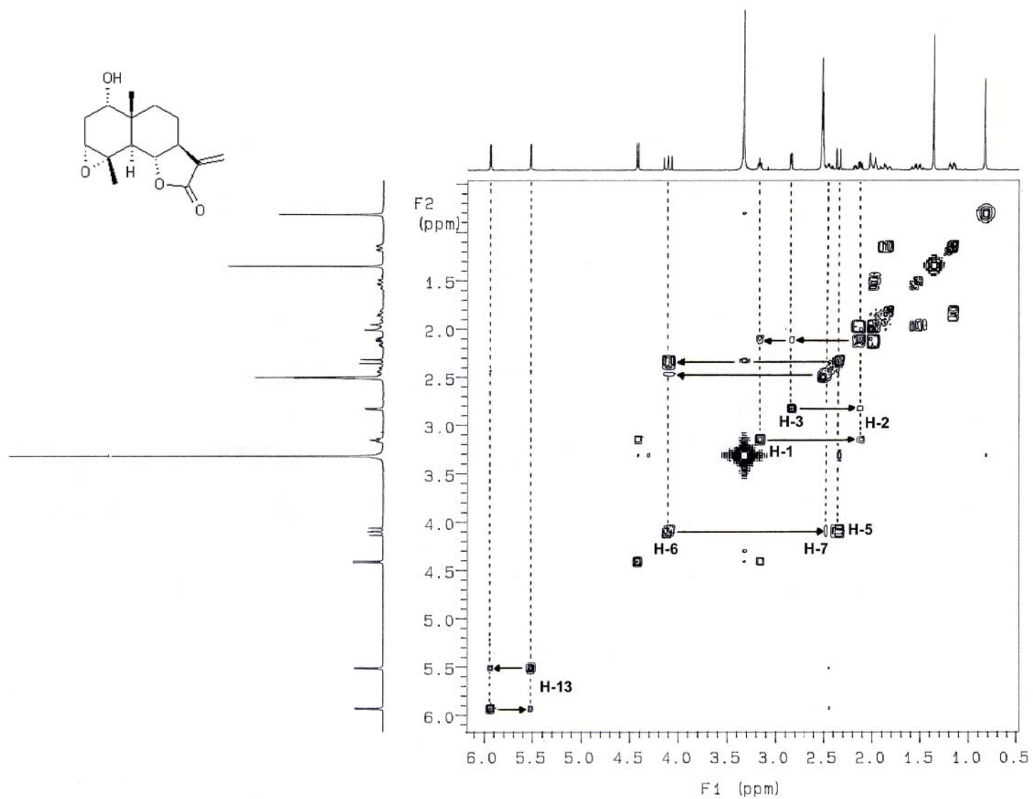
Espectro 6. Espectro COSY de la Ludovicina A.
