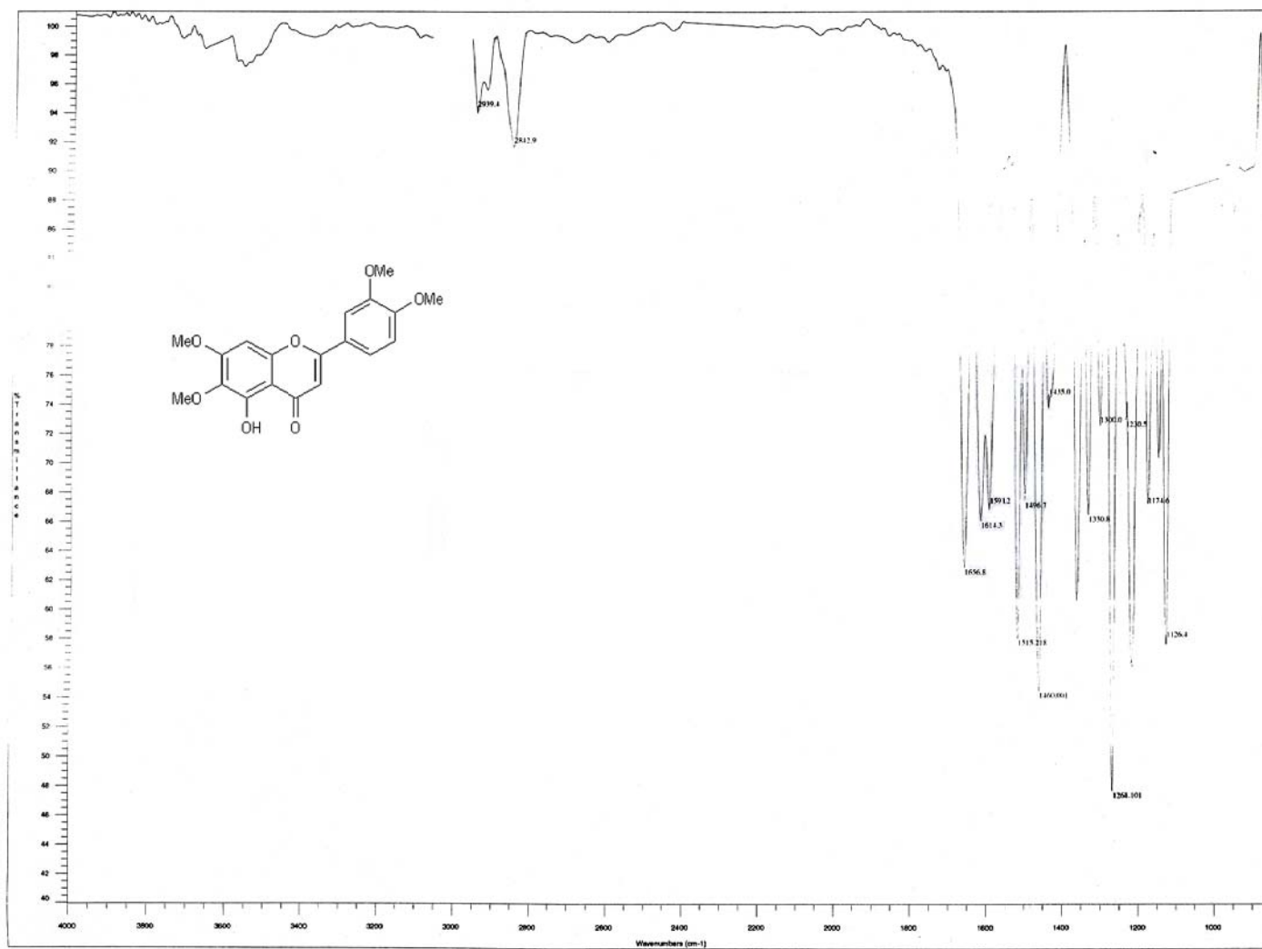
Espectro 30. Espectro de IR (Nujol) de la 5-hidroxi-3',4',6,7-tetrametoxiflavona.
