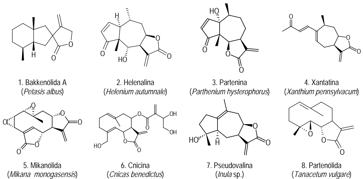
Figura 4. Estructuras de lactonas sesquiterpénicas con actividad biológica.
