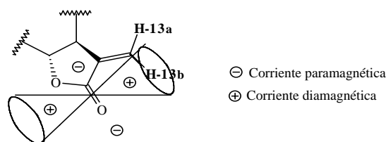
Figura 12. Posición de los hidrógenos H-13a y H-13b y efecto de anisotropía sobre H-13b.
