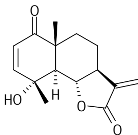
Figura 14. Arglanina.
