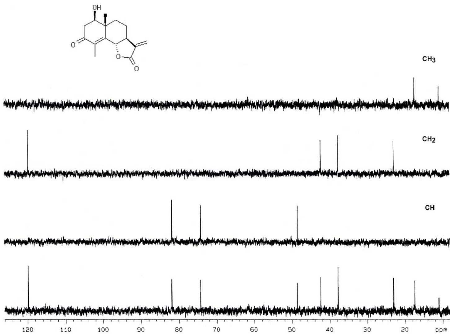
Espectro 9. Espectro DEPT de la Armexifolina.
