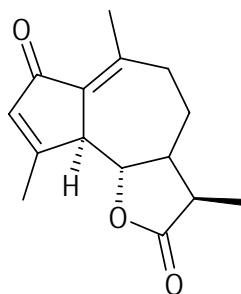
Figura 34. Achillina.
