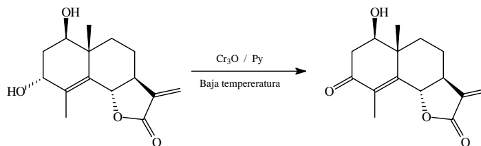
Figura 23. Reacción de oxidación de la Arnefolina.
