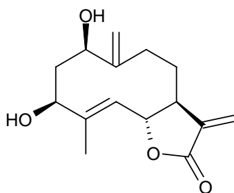
Figura 30. Ridentina.
