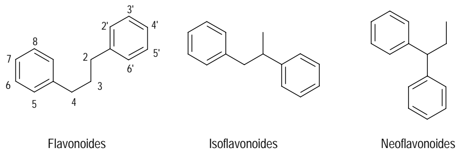
Figura 7. Estructuras básicas de los flavonoides.
