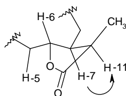
Figura 33. Posición del metilo C-13, de H-7 y H-11 en la lactona.
