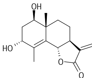
Figura 17. Arnefolina.
