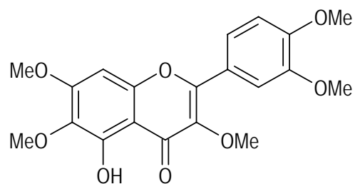
Figura 29. Artemetina.
