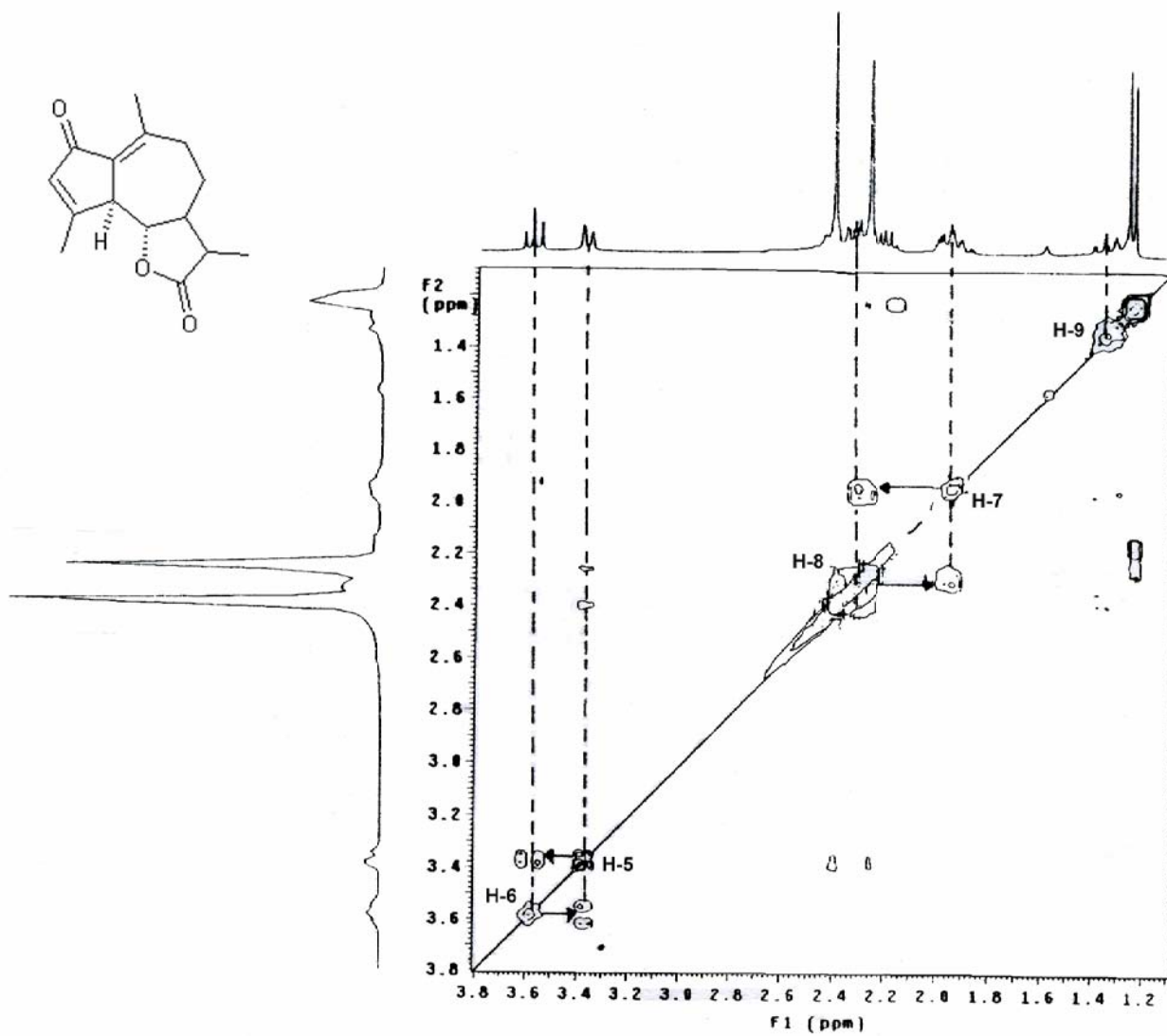
Espectro 25. Espectro COSY de la Achillina.
