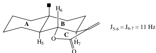
Figura 11. Disposición espacial de los hidrógenos H-5, H-6 y H-7.
