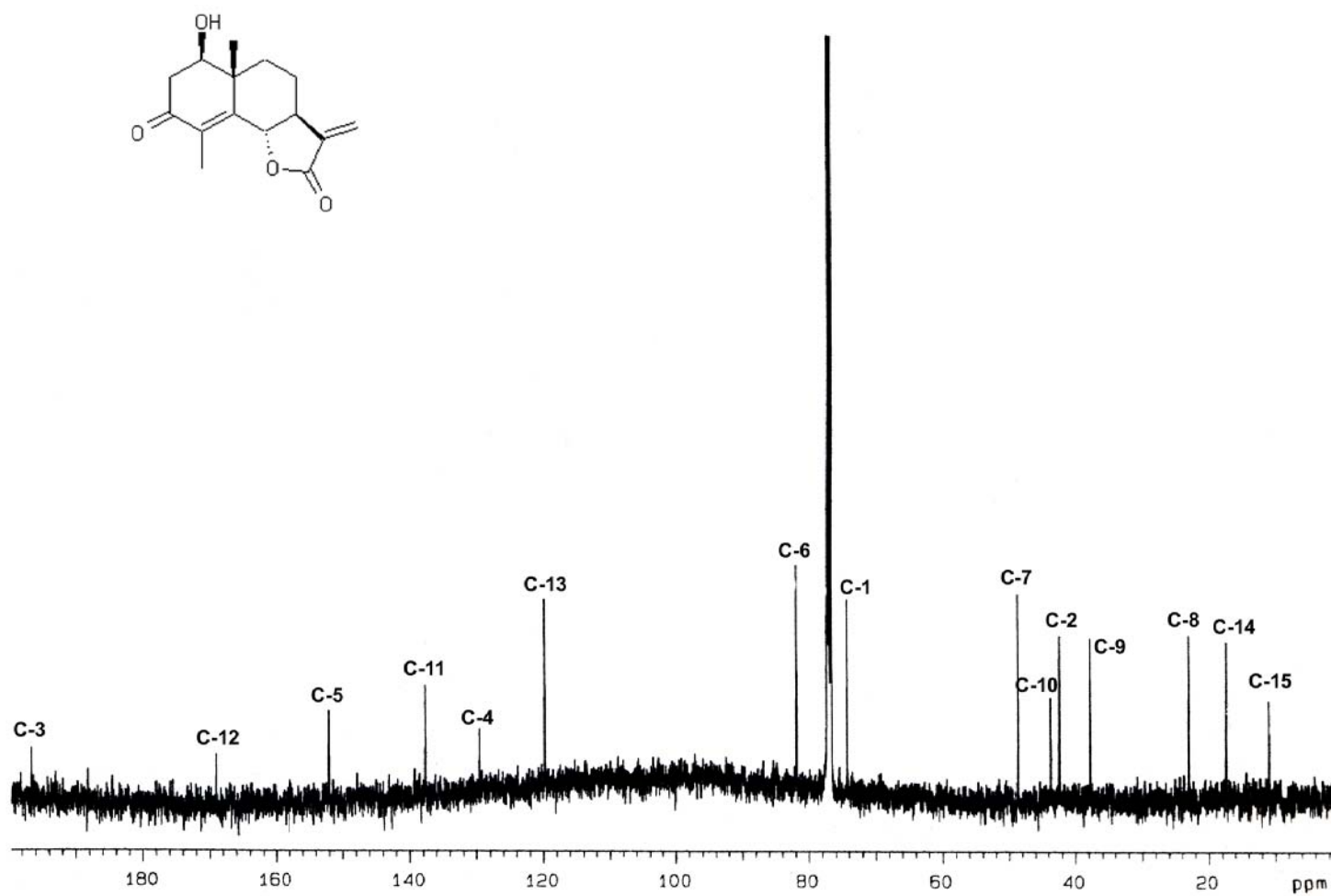
Espectro 8. Espectro de \text{RMN}^{13}\text{C} (500 MHz, \text{CDCl}_3 , TMS) de la Armexifolina.
