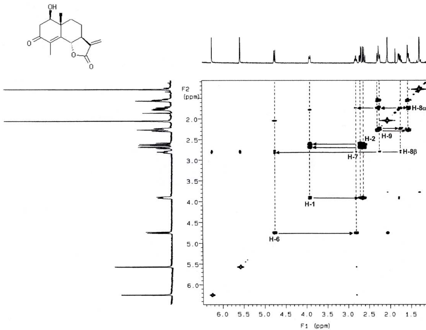
Espectro 11. Espectro COSY de la Armexifolina.
