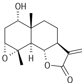
Figura 16. Ludovicina A.
