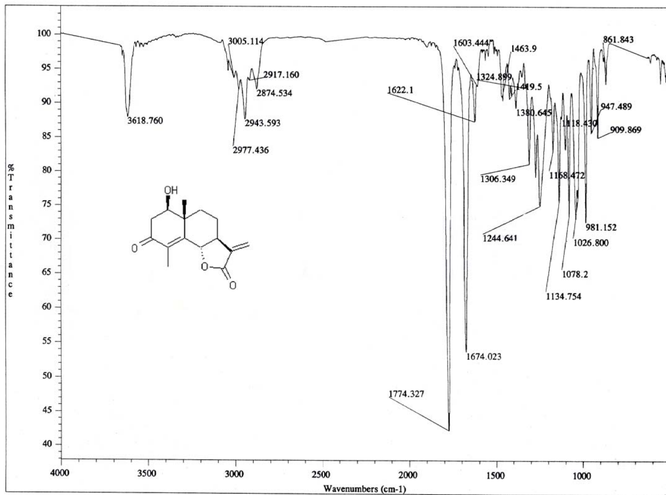
Espectro 7. Espectro IR (CHCl 3 ) de la Armexifolina.
