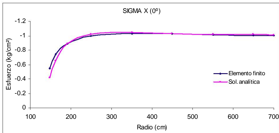
Figura 6.25 Malla final en remalleo # 3, esfuerzos \sigma_x en la línea horizontal
