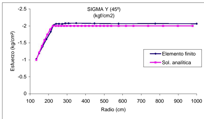
Figura 6.56 Gráfica Radio vs \sigma_y , malla remallada
