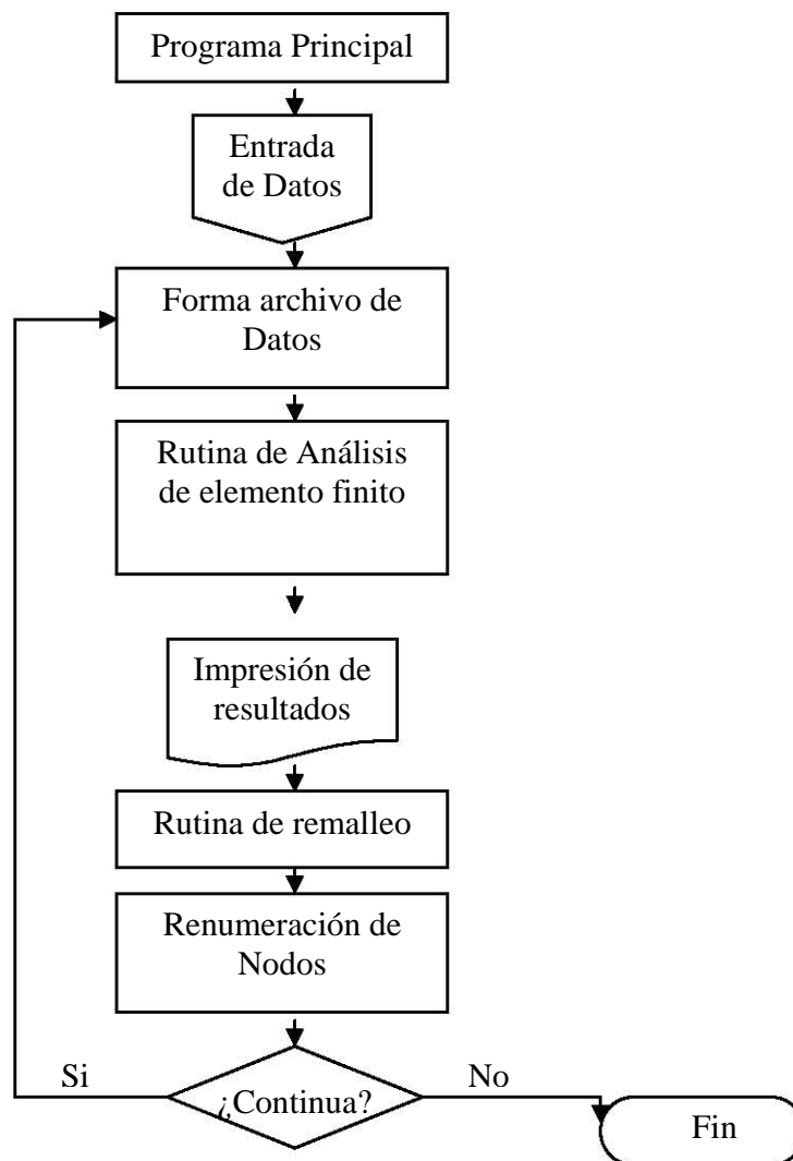
Figura 5.1 Diagrama de flujo del proceso de remalleo automático
