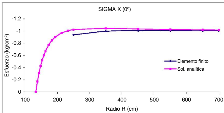
Figura 6.21 Malla burda, esfuerzos \sigma_x en la línea horizontal
