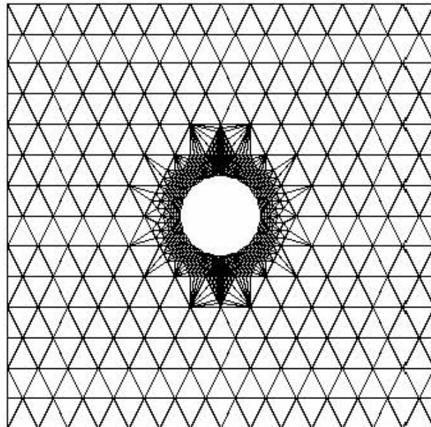
Figura 6.10 Remalleo 3 de 1692 elementos y 908 nudos
