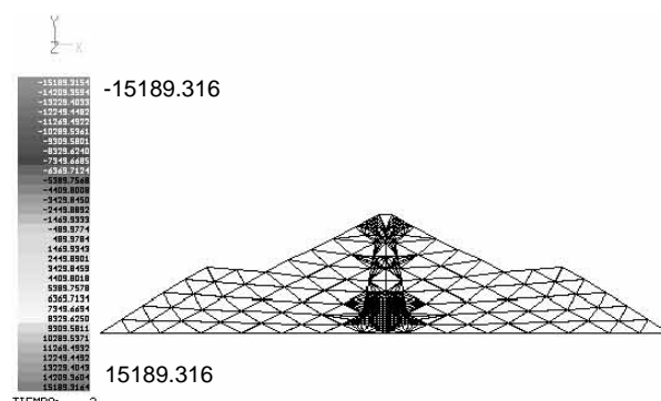
Remalleo 2 PRESA2A
