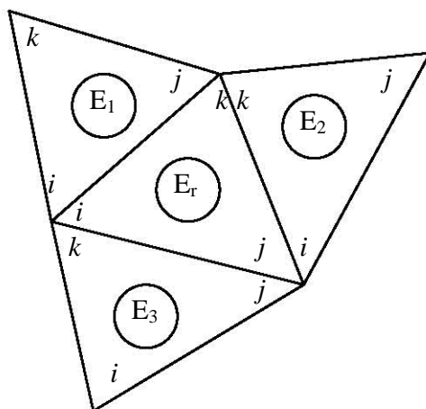
Figura 4.6 Incidencias y conexión local entre el elemento a remallar y sus contiguos
