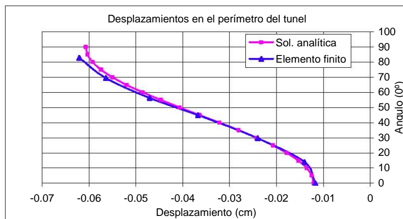
Figura 6.32: Desplazamientos en la circunferencia, malla fina
