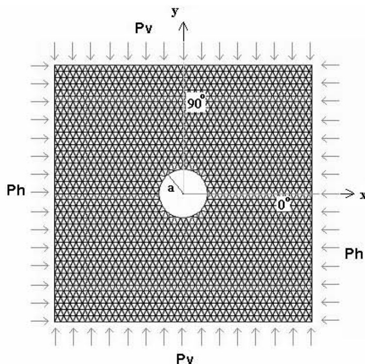
Figura 6.6 Malla de 3470 elementos y 1870 nudos
