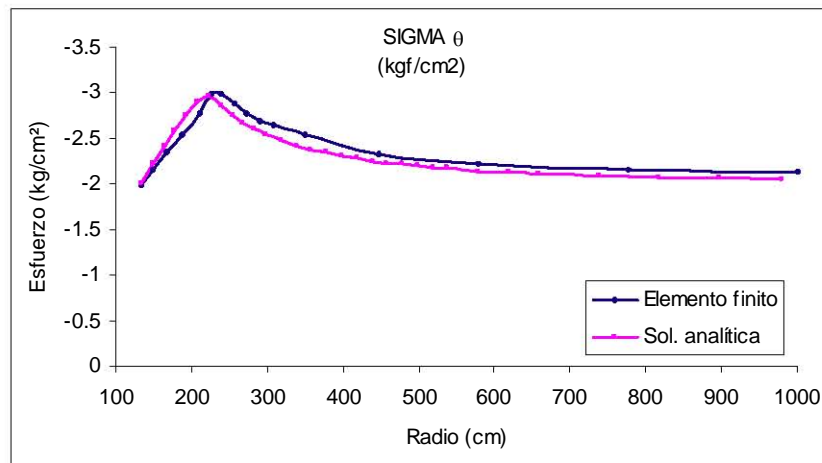
Figura 6.52 Gráfica Radio vs \sigma_\theta , malla remallada
