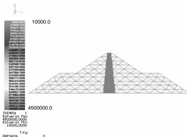
Figura A.47 Modelo de presa con elementos finitos y distribución de materiales. La coloración indica la magnitud del modulo de elasticidad en \text{kgf/m}^2 .
