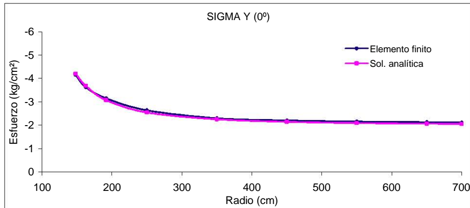
Figura 6.29 Malla final en 3 er remalleo, esfuerzos \sigma_y en la línea horizontal
