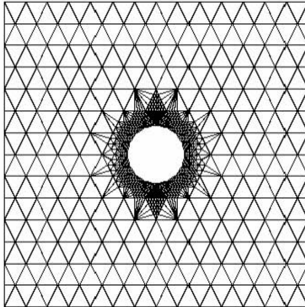
Figura 6.9 Remalleo 2 de 1588 elementos y 856 nudos
