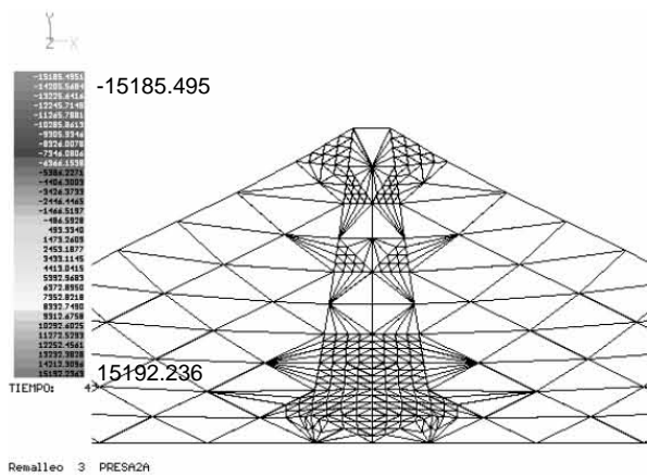
Figura A.58 Remalleo # 3
