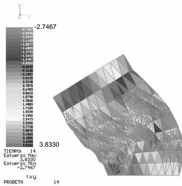
Figura A.17 Estado de esfuerzos \tau_{xy} en la iteración # 14
