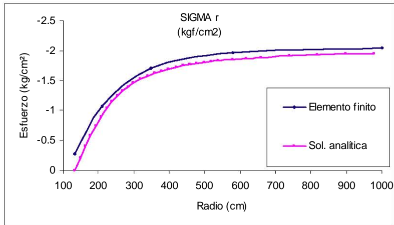
Figura 6.45 Gráfica Radio vs Esfuerzo Radial para la malla burda
