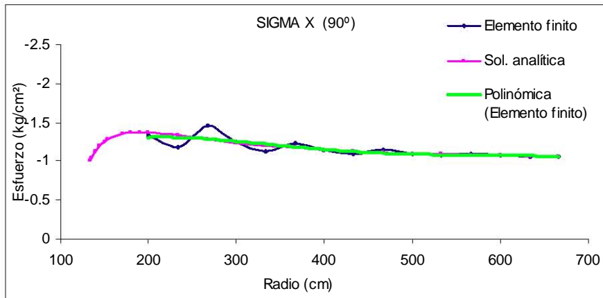
Figura 6.12 Malla intermedia, esfuerzos \sigma_x en la línea vertical
