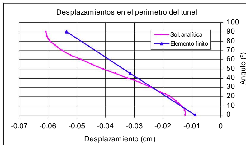
Figura 6.30: Desplazamientos en la circunferencia, malla burda
