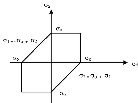
Figura 5.4 Estado de esfuerzo, teoría de Tresca.
