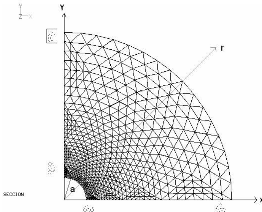
Figura 6.40 Malla fina de 1152 elementos y 625 nodos
