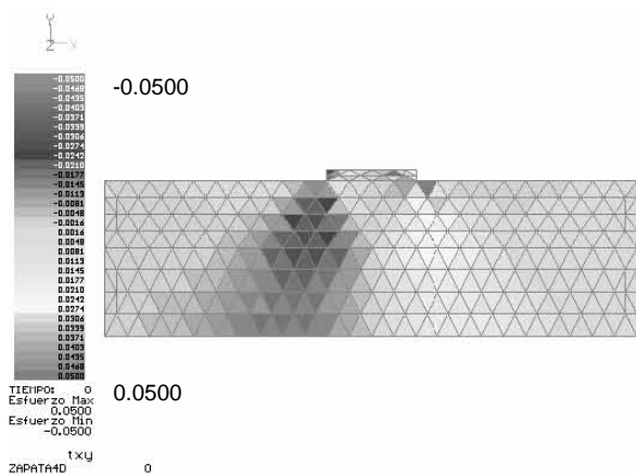
Figura A.33 Estado de esfuerzos \tau_{xy} inicial
