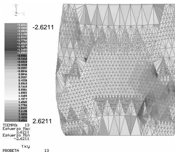
Figura A.11 Iteración # 13, estado de esfuerzos \tau_{xy} con acercamiento
