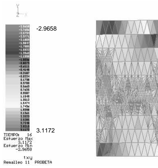
Figura A.31 Estado de esfuerzos \tau_{xy} en remalleo # 11
