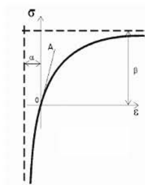
Figura A.1 Modelo hiperbólico de Kondner
