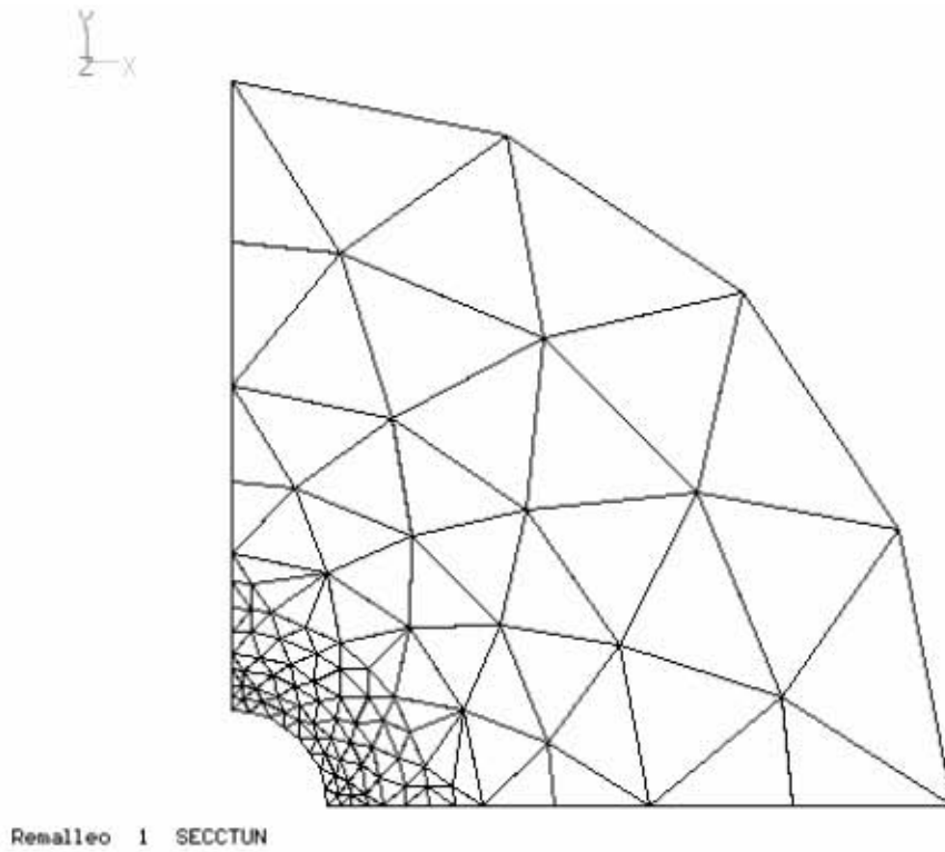
Figura 6.41 Primer remalleo en análisis elastoplástico
