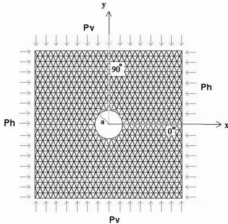
Figura 6.5 Malla de 1550 elementos y 855 nudos
