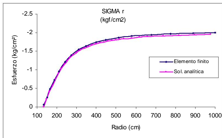
Figura 6.47 Gráfica Radio vs Esfuerzo Radial para la malla fina
