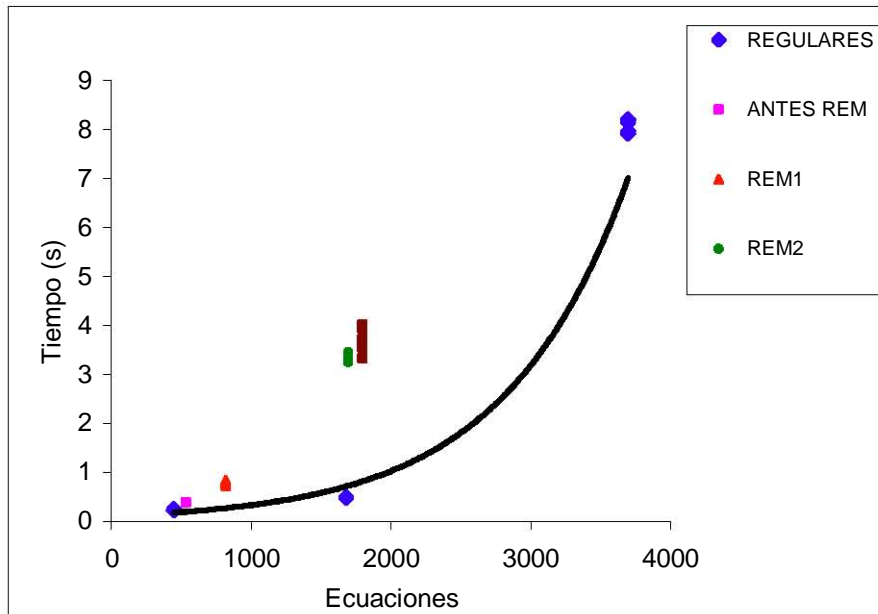
Figura 6.35 Gráfica número de ecuaciones vs Tiempo
