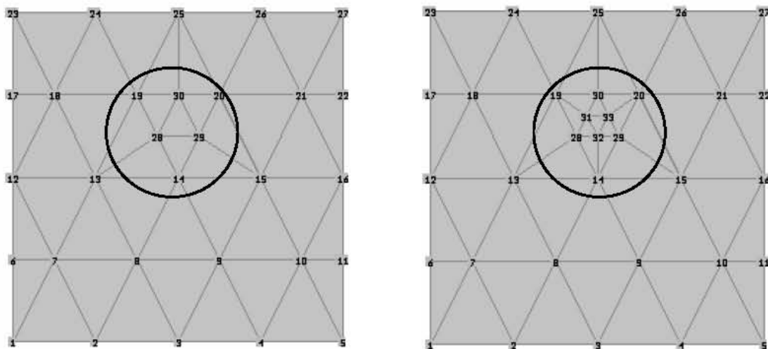
Figura 4.3 Malla de elemento finito refinada.
