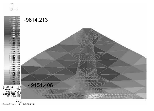
Figura A.61 Estado de esfuerzos \tau_{xy} , remalleo # 9
