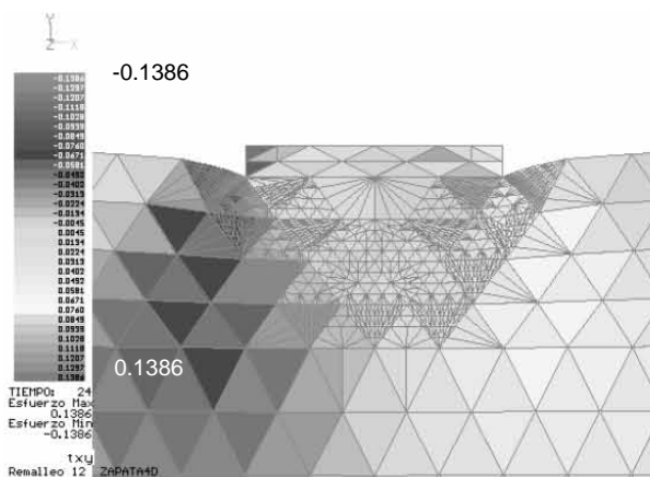
Figura A.45 Acercamiento del estado de esfuerzos \tau_{xy} , remalleo # 12
