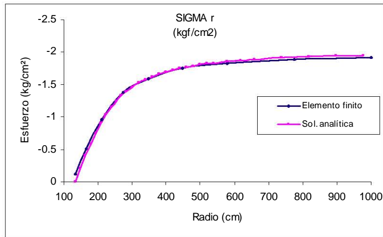
Figura 6.46 Gráfica Radio vs Esfuerzo Radial para la malla intermedia
