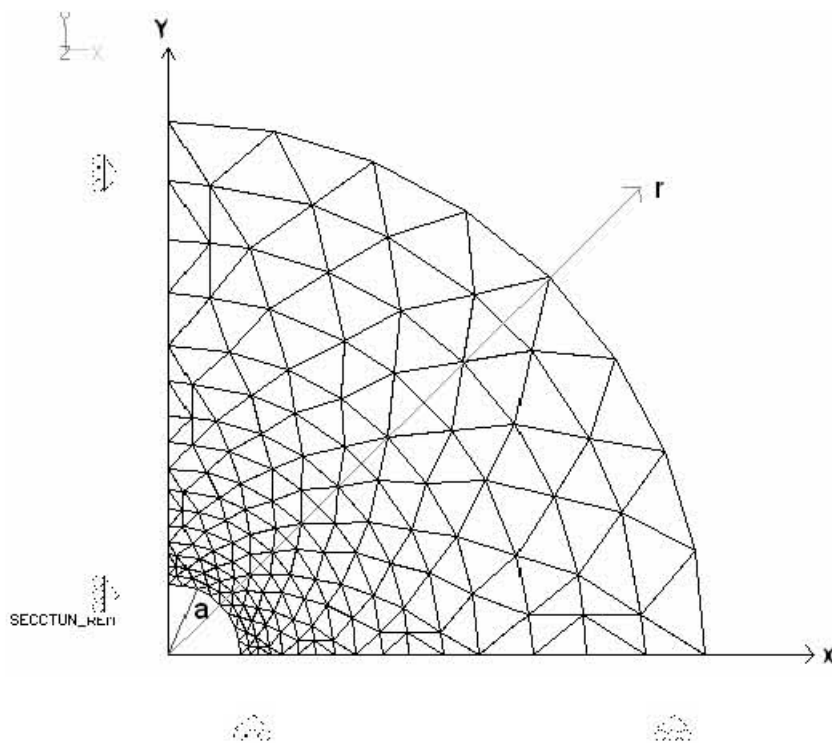
Figura 6.39 Malla intermedia de 288 elementos y 169 nodos
