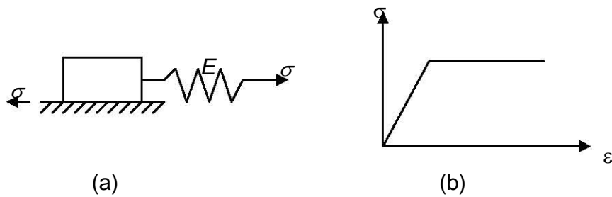
Figura 6.2 Material St. Venant. (a) Modelo, (b) Gráfica esfuerzo deformación.
