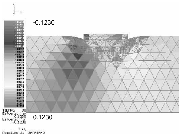
Figura A.38 Estado de esfuerzos \tau_{xy} correspondiente al remalleo #21
