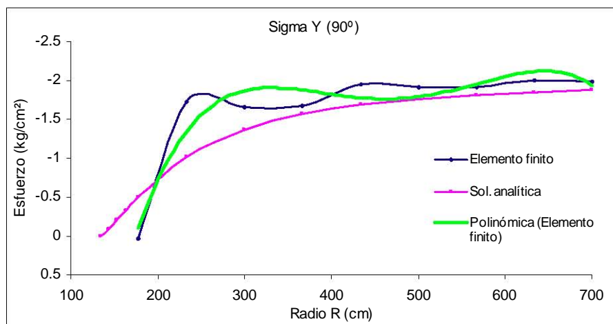
Figura 6.16 Malla burda, esfuerzos \sigma_y en la línea vertical sobre el túnel
