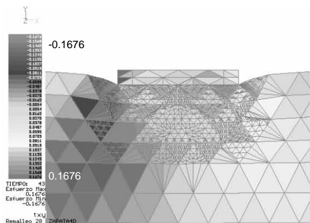
Figura A.46 Remalleo # 2A. Estado de esfuerzos \tau_{xy}
