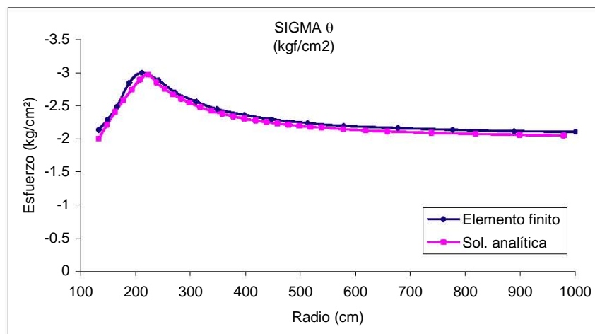
Figura 6.51 Gráfica Radio vs \sigma_{\theta} , malla fina
