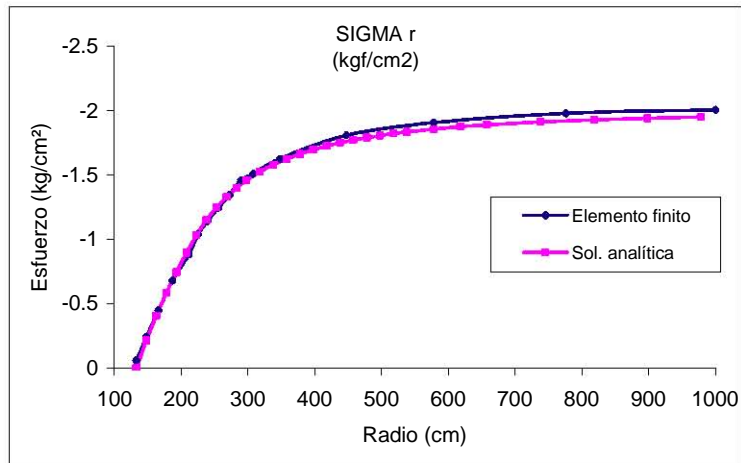
Figura 6.48 Gráfica Radio vs Esfuerzo Radial en el remalleo
