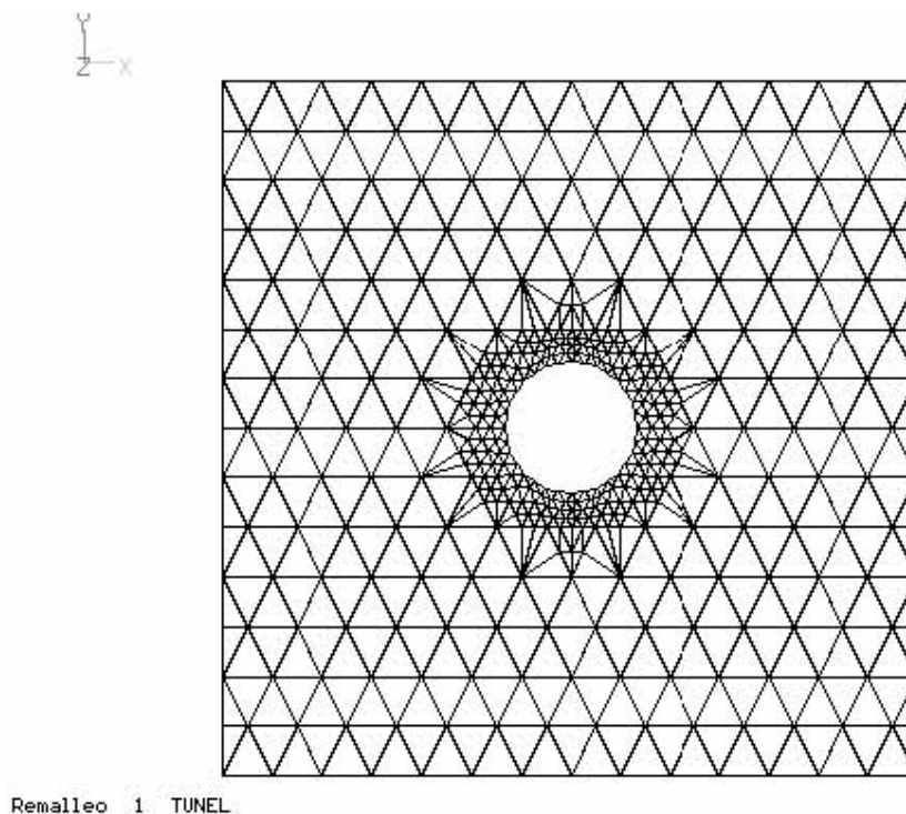
Figura 6.8 Remalleo 1 de 744 elementos y 418 nudos
