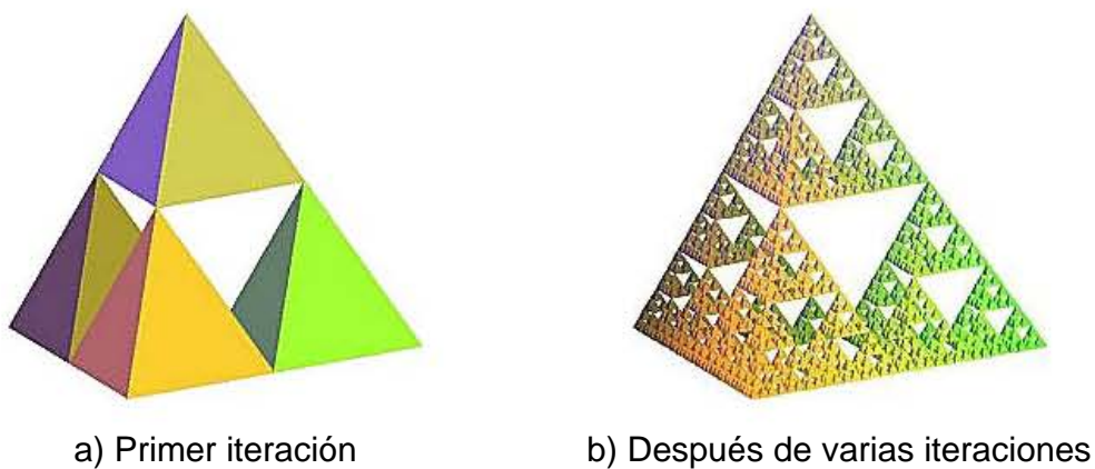
Figura 2.13 Tetraedro de Sierpinski
