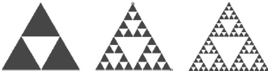
Figura 4.1 Proceso de generación del triángulo de Sierpinsky
