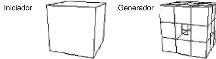
Figura 2.14 Iniciador y generador del fractal Esponja de Menger
