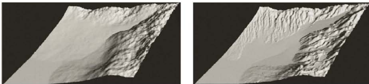
Figura 2.7 Modelación con fractales, erosión de un terreno
