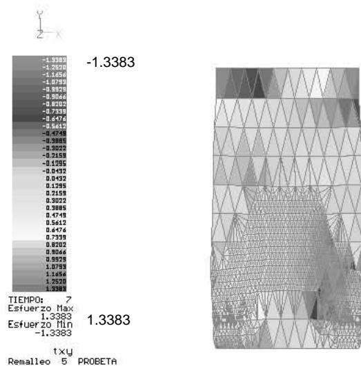
Figura A.7 Remalleo #5, esfuerzos \tau_{xy}
