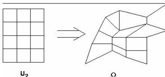
Figura 2.17 Transformación del cuadrado unitario ( U_2 ) en una región irregular ( \Omega ).
