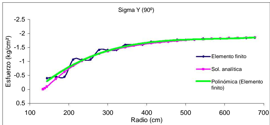
Figura 6.18 Malla fina, esfuerzos \sigma_y en la línea vertical
