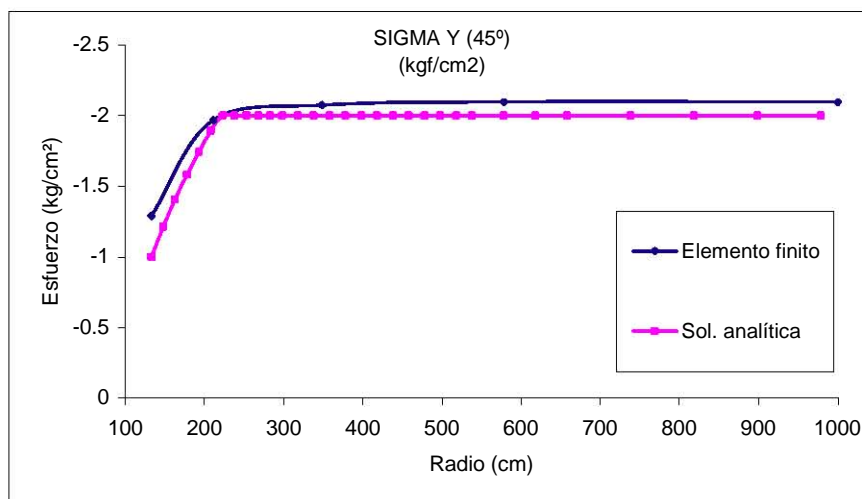
Figura 6.53 Gráfica Radio vs \sigma_y , malla burda
