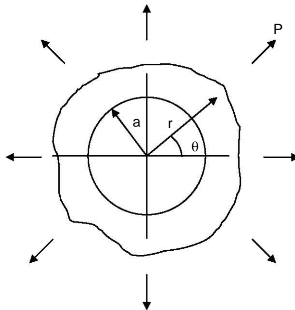
Figura 6.3 Túnel circular en una masa infinita bajo presión hidrostática
