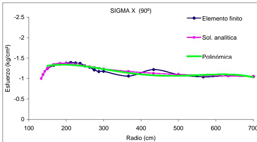
Figura 6.15 Malla final en 3 er remalleo, esfuerzos \sigma_x en la línea vertical
