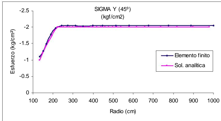
Figura 6.55 Gráfica Radio vs \sigma_y , malla fina
