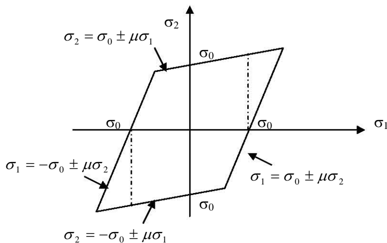
Figura 5.5: Estado de esfuerzos, teoría de Saint-Venant
