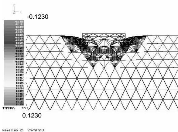
Figura A.37 Remalleo # 21, acercamiento
