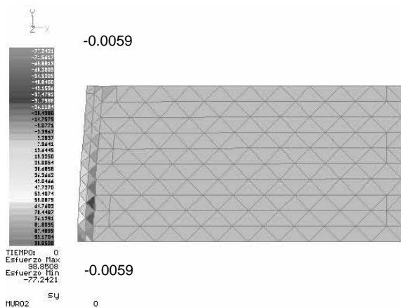
Figura A.71 Estado de esfuerzos \sigma_y inicial
