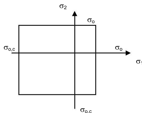
Figura 5.3 Estado de esfuerzos en la resistencia máxima
