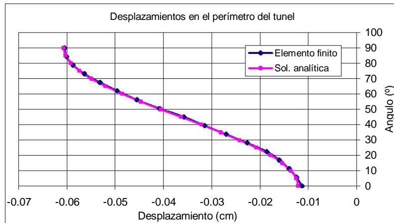
Figura 6.34: Desplazamientos en la circunferencia, malla final en 3 er remalleo
