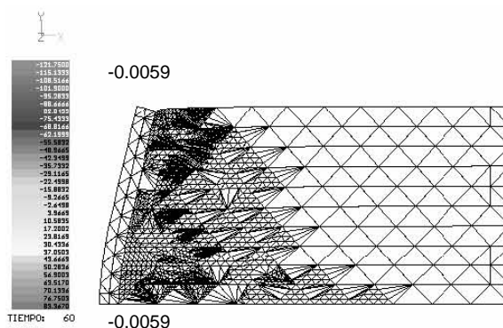
Remalleo 40 MURO2
