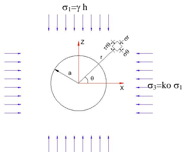
Figura 6.1 Análisis de un túnel en un medio infinito
