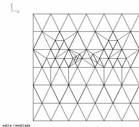
Figura 4.4 Remalleo asimétrico en un análisis lineal
