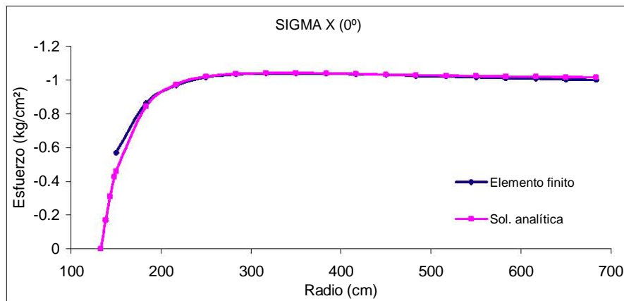
Figura 6.23 Malla fina, esfuerzos \sigma_x en la línea horizontal
