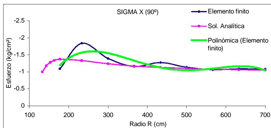
Figura 6.11 Malla burda, esfuerzos \sigma_x en la línea vertical
