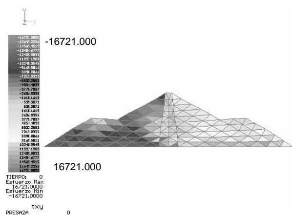
Figura A.48 Estado de esfuerzos \tau_{xy} inicial, debido a peso propio
