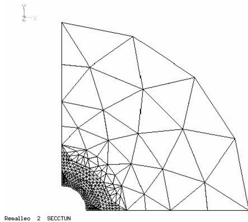
Figura 6.42 Remalleo 2 en la malla de elemento finito
