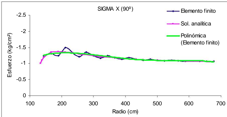
Figura 6.13 Malla fina, esfuerzos \sigma_x en la línea vertical
