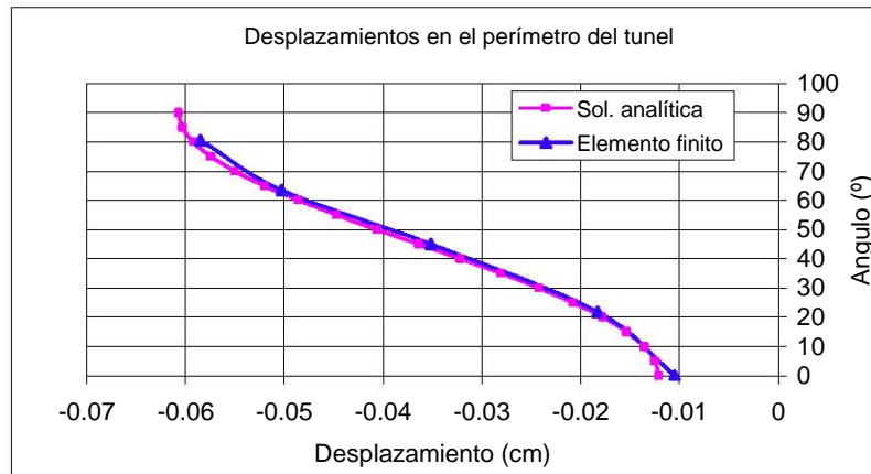
Figura 6.31: Desplazamientos en la circunferencia, malla intermedia
