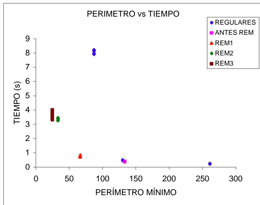
Figura 6.37 Gráfica perímetro del elemento menor vs tiempo
