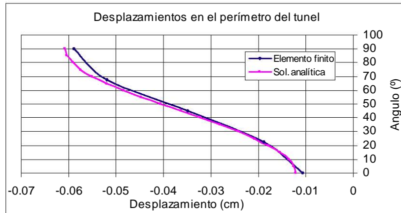
Figura 6.33: Desplazamientos en la circunferencia, malla inicial en remalleo
