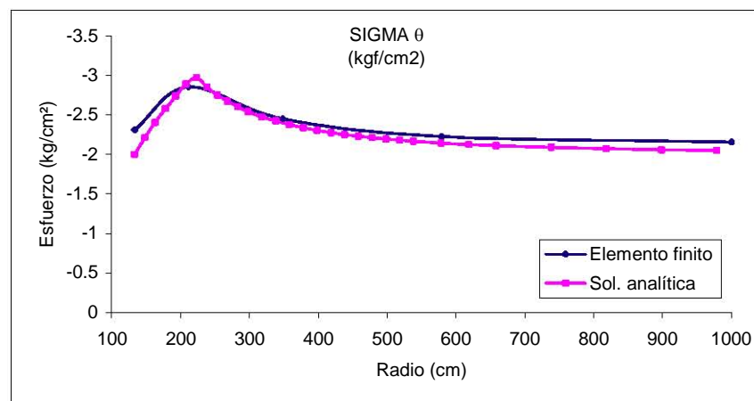
Figura 6.49 Gráfica Radio vs \sigma_{\theta} , malla burda
