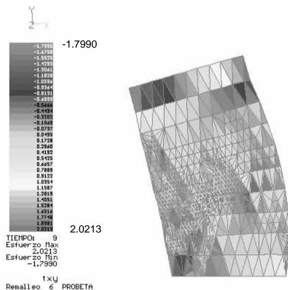
Figura A.15 Estado de esfuerzos \tau_{xy} en el remalleo # 6
