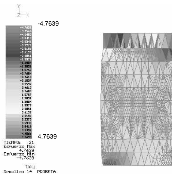
Figura A.25 Remalleo # 14, estado de esfuerzos \tau_{xy}
