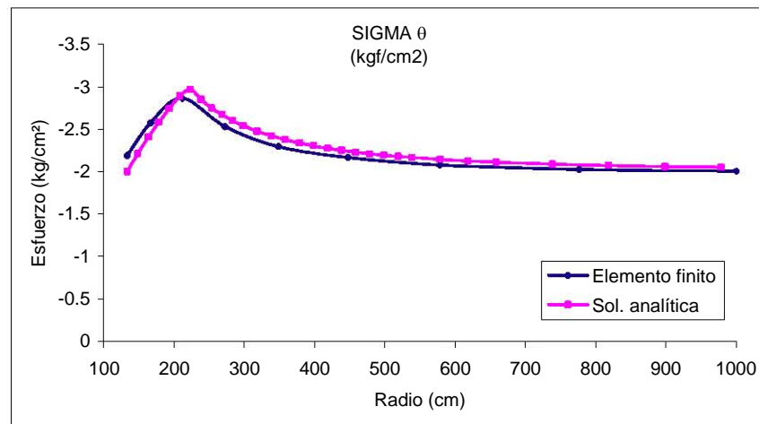
Figura 6.50 Gráfica Radio vs \sigma_{\theta} , malla intermedia
