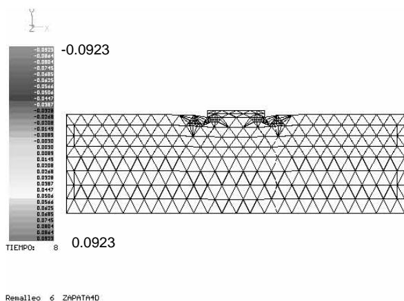
Figura A.35 Remalleo # 6
