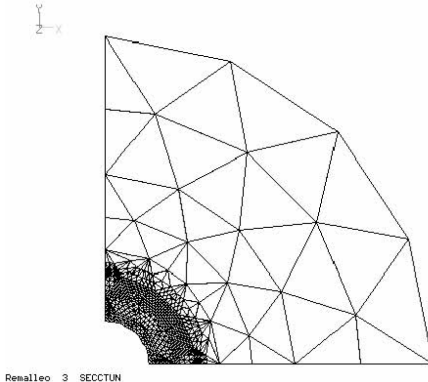
Figura 6.43 Remalleo 3 en la malla de elemento finito
