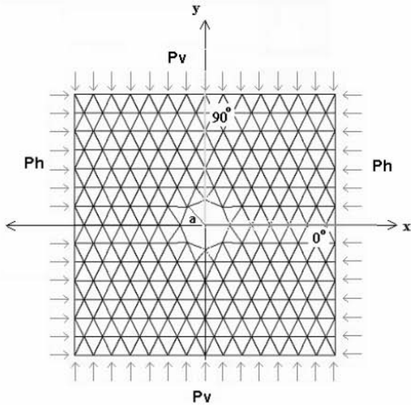
Figura 6.4 Malla de 396 elementos y 232 nudos
