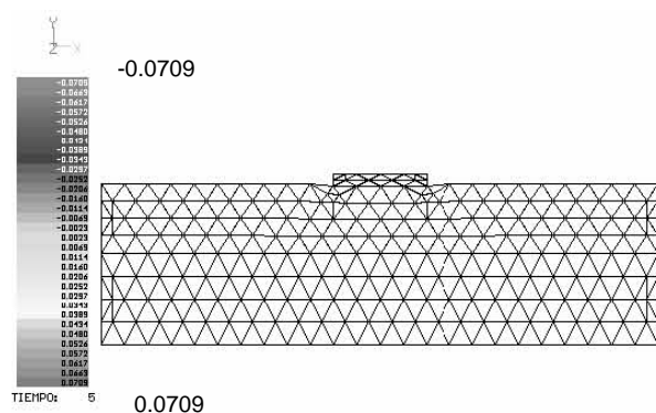
Figura A.39 Remalleo inicial
