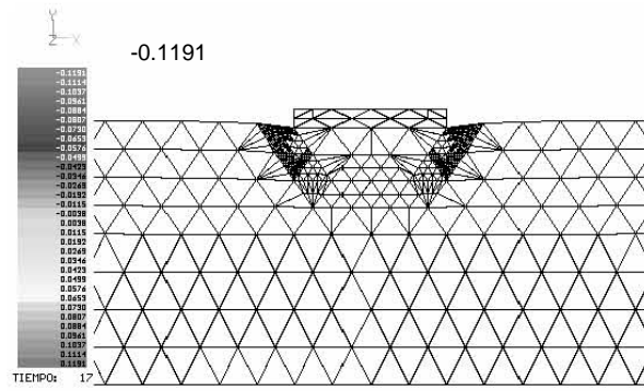
Figura A.42 Remalleo # 7
