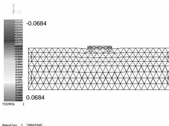
Figura A.34 Primer remalleo
