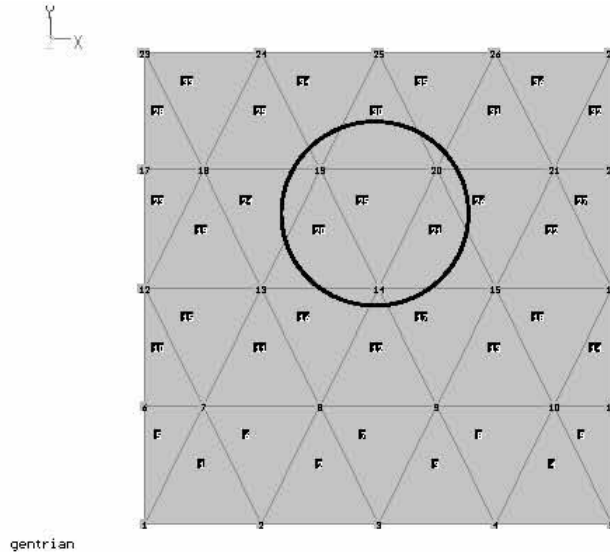
Figura 4.2 Malla de elemento finito inicial
