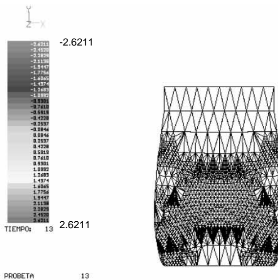
Figura A.9 Remallo en Iteración # 13
