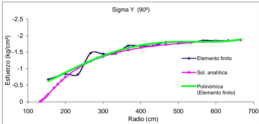
Figura 6.17 Malla intermedia, esfuerzos \sigma_y en la línea vertical sobre el túnel
