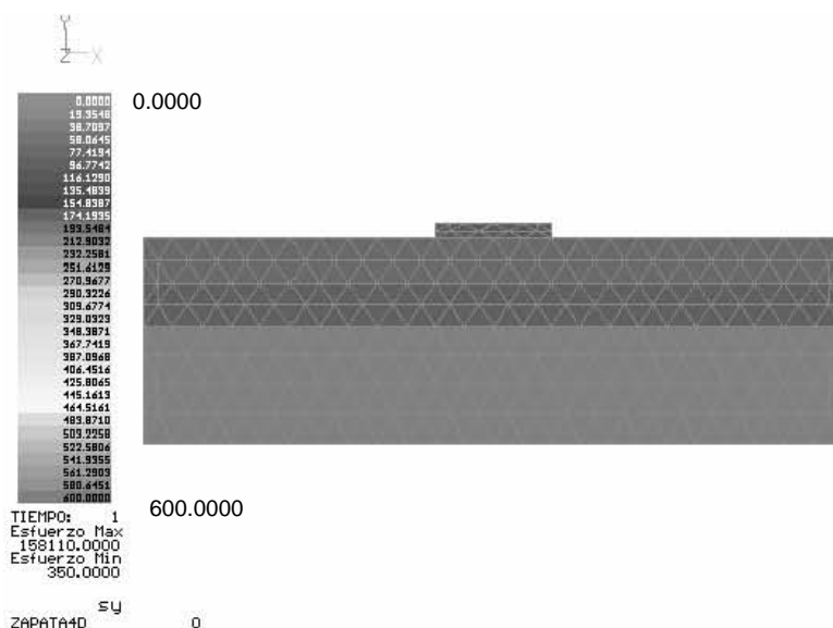
Figura A.32 Modelación de una zapata aislada. La escala de colores indica el módulo de elasticidad del suelo, en \text{kgf/cm}^2 .
