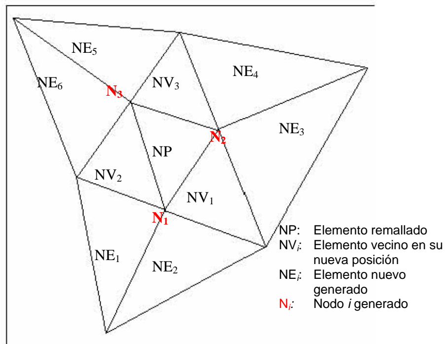
Figura 4.7 Fragmentación del elemento a remallar y de los elementos vecinos
