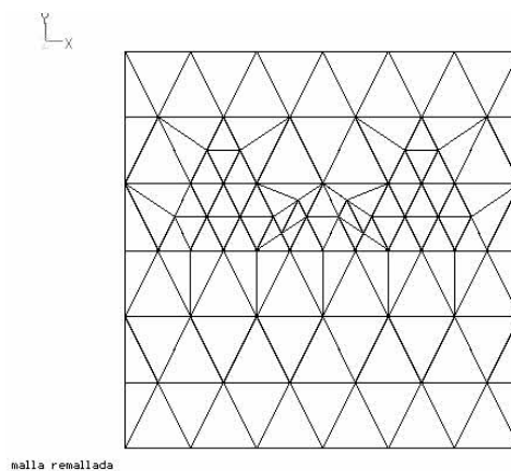
Figura 4.5 Remalleo simétrico en un análisis lineal
