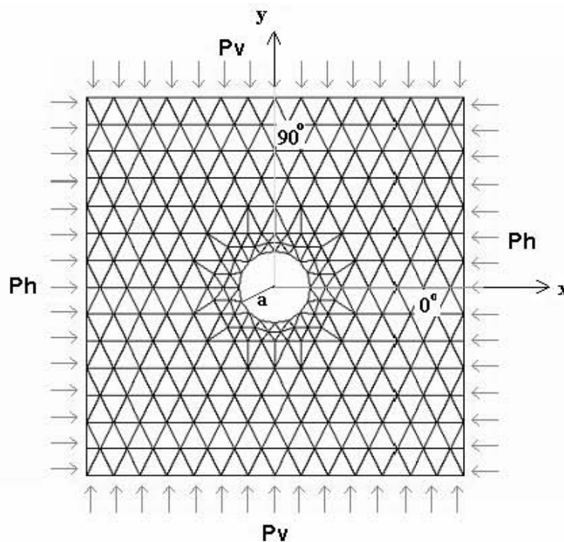
Figura 6.7 Malla de 476 elementos y 276 nudos
