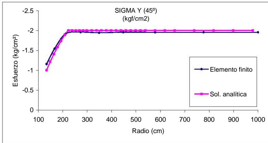
Figura 6.54 Gráfica Radio vs \sigma_y , malla intermedia
