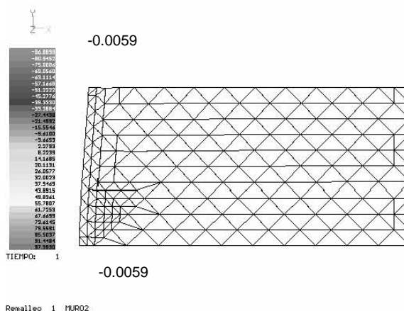
Figura A.72 Primer remalleo
