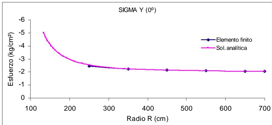
Figura 6.26 Malla burda, esfuerzos \sigma_y en la línea horizontal
