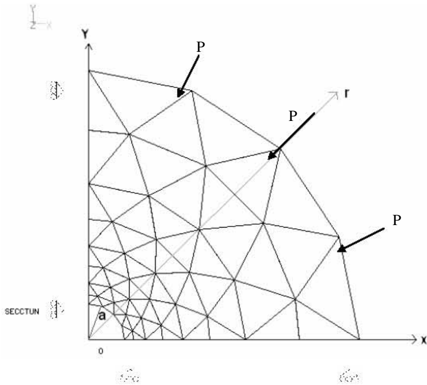
Figura 6.38 Malla burda de 72 elementos y 49 nodos.
