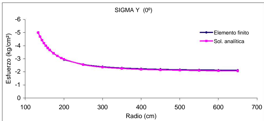
Figura 6.27 Malla intermedia, esfuerzos \sigma_y en la línea horizontal
