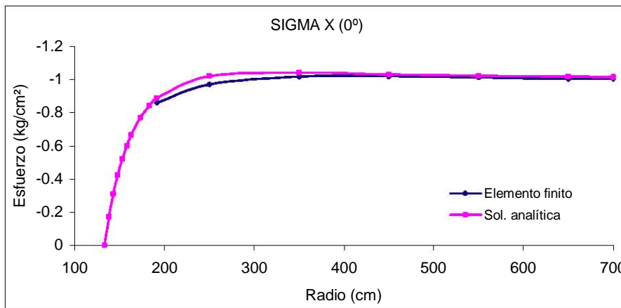
Figura 6.24 Malla inicial en remalleo, esfuerzos \sigma_x en la línea horizontal
