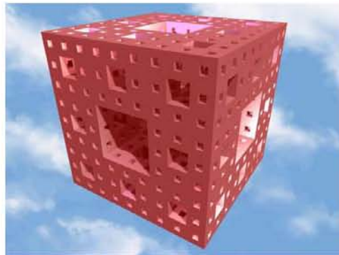
Figura 2.15 Esponja de Menger
