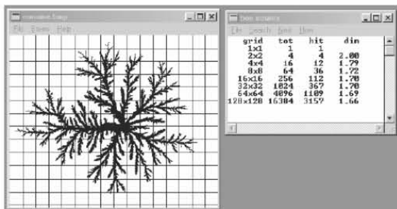
Figura 2.3 Método de conteo de cajas para calcular la dimensión fractal.
