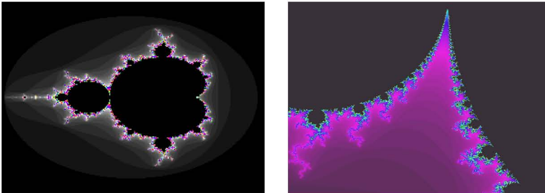
Figura 2.1 Conjunto de Mandelbrot
