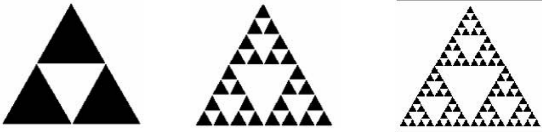
Figura 2.12 Generación del triángulo de Sierpinski
