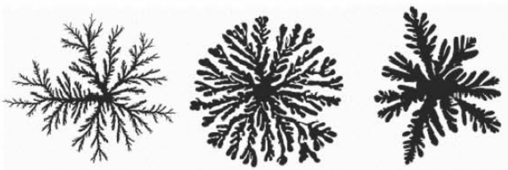
Figura 2.5 Configuraciones fractales
