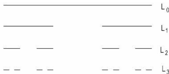
Figura 2.8: Conjunto de Cantor
