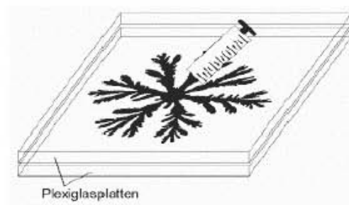
Figura 2.4 Experimento de Henry S. Hele-Shaw
