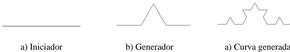
Figura 2.10 Construcción de la curva de Koch.
