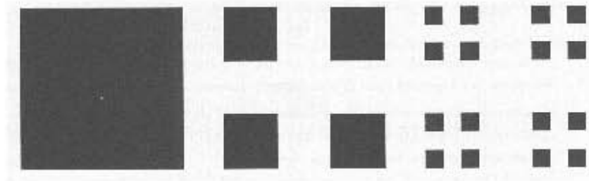
Figura 2.9 Conjunto de Cantor en el plano
