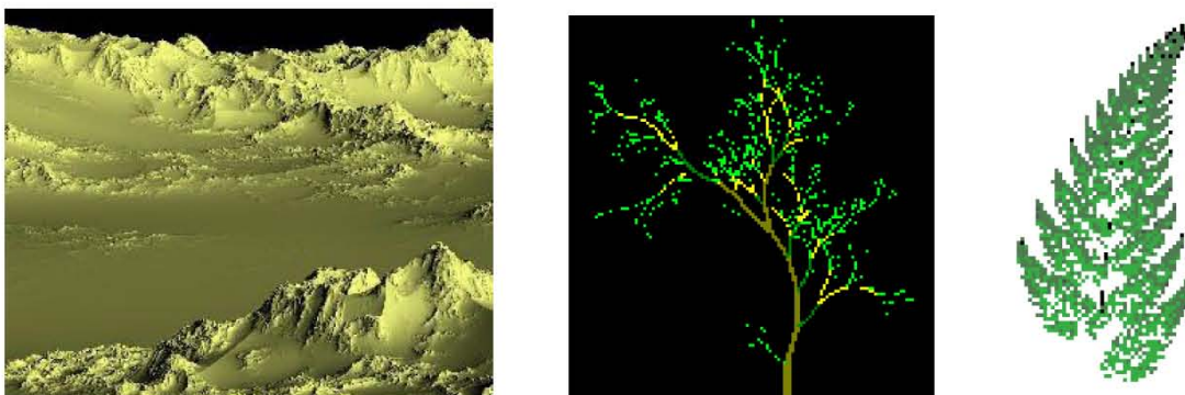
Figura 2.2 Simulación de formas naturales mediante fractales
