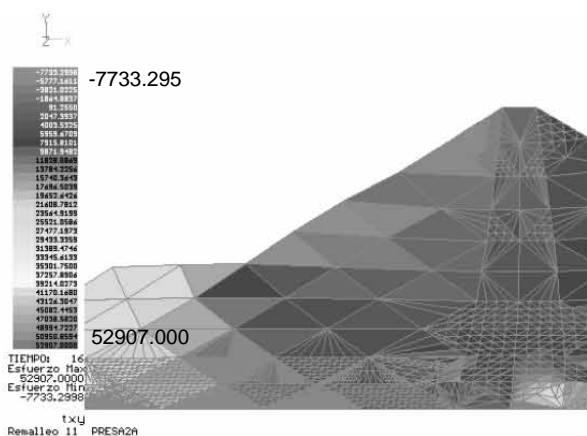
Figura A.55 Estado de esfuerzos \tau_{xy} en remallo # 11
