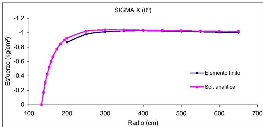
Figura 6.22 Malla intermedia, esfuerzos \sigma_x en la línea horizontal
