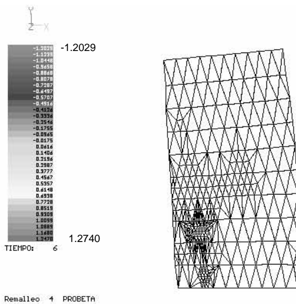
Figura A.13 Remalleo #4
