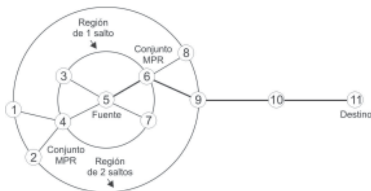
Figura 3.13.- Descubrimiento de ruta con MPR
