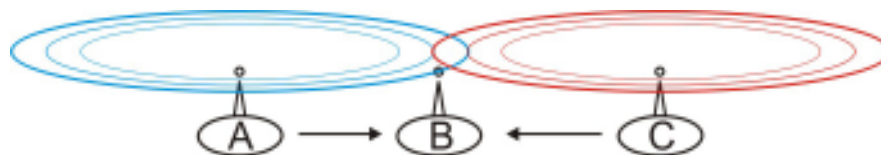
Figura 3.1 .- El nodo A es una terminal oculta para C
