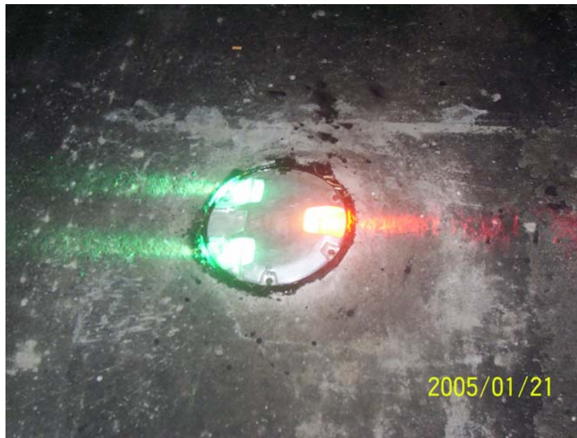
Fotografía V.38.- Unidad rasante para umbral (luces color verde) y extremo de pista (luz color roja)
