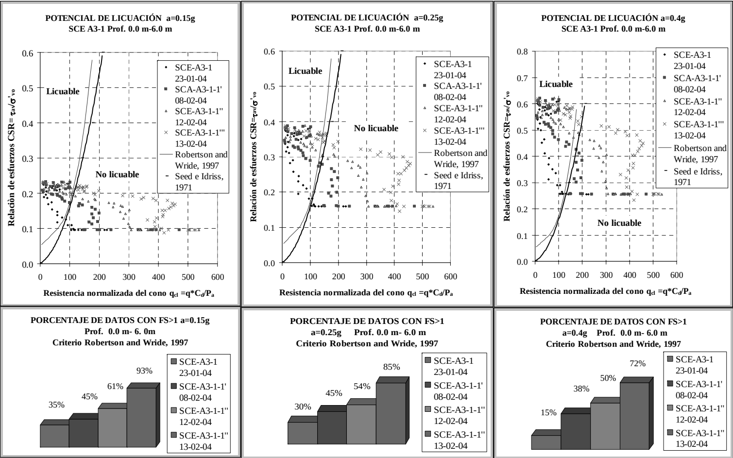
Figura 6.7 Efecto de la aceleración máxima en el potencial de licuación de los materiales del Sector 1
