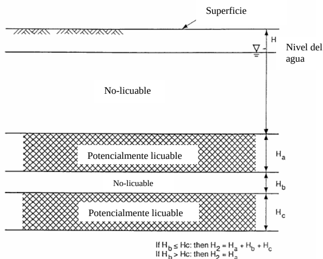
Figura 4.18 Esquema para determinar H_1 y H_2 , Ishihara (1985)
