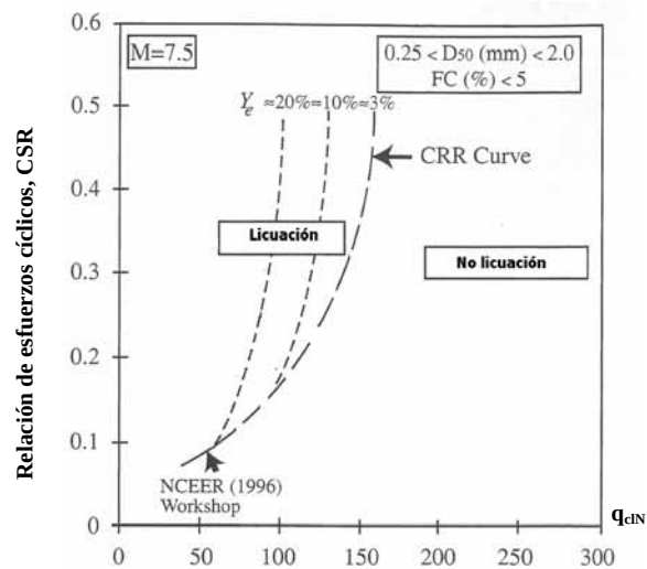
Figura4.16 Valores tentativos de las deformaciones al cortante generadas por licuación, con base en q_{clN} , Seed et al. (1985)
