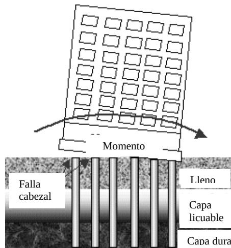
Figura 3.14 Falla de la conexión entre el cabezal de los pilotes y la superestructura
