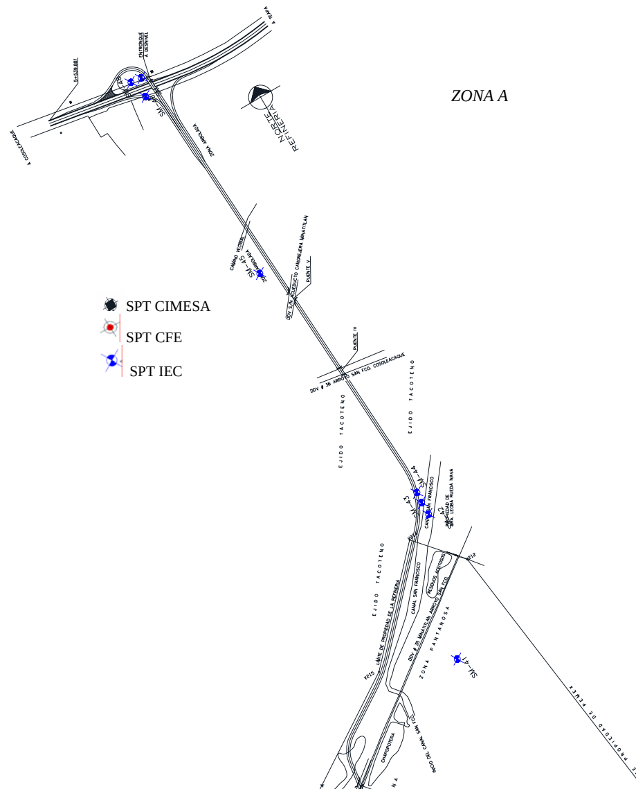
Figura A2.1 Detalle de localización de pruebas SPT en el área de estudio, Zona A
