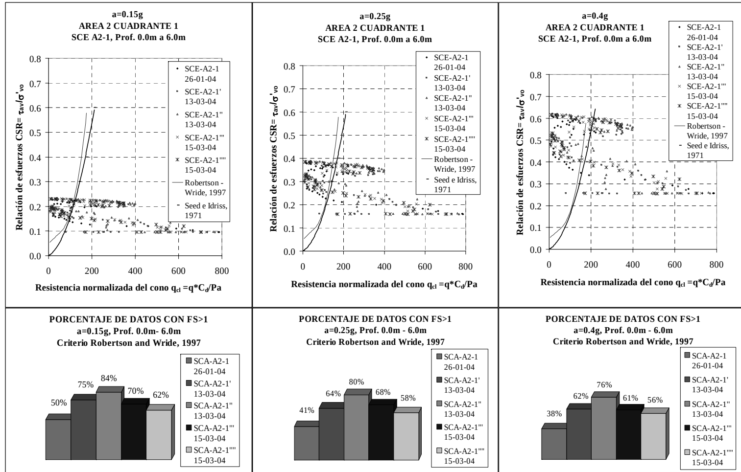
Figura 6.17 Efectividad de la vibroflotación para reducir la licuabilidad de los estratos superficiales, hasta 6m de profundidad (primer cuadrante)
