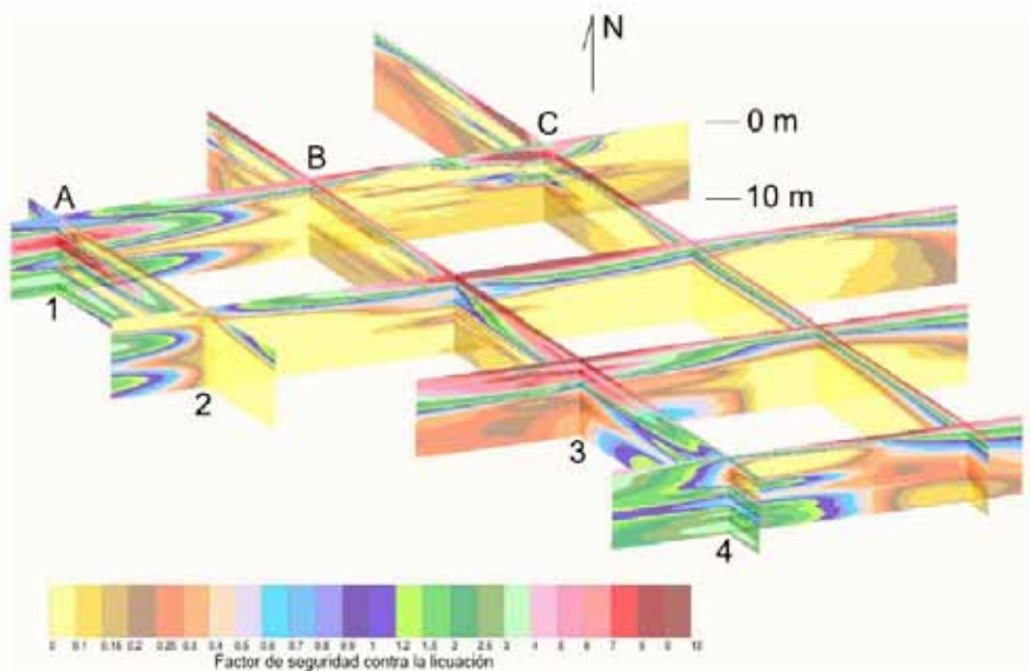
Figura 2.2 Vista en 3D de los siete cortes del factor de seguridad contra la licuación, profundidad 0 a 10 m, Auvinet et al. (2005)
