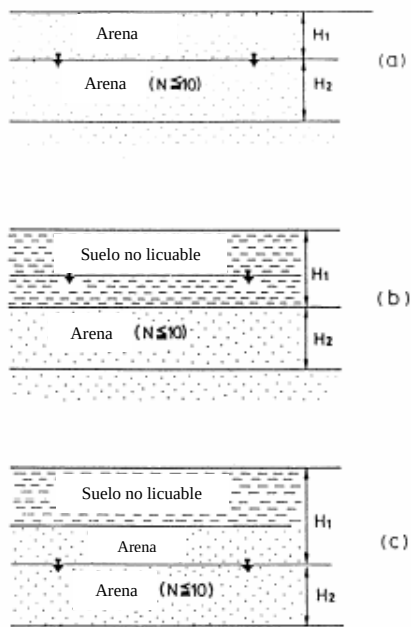
Figura 4.19 Definición de las capas licuables y no licuables, Ishihara (1985)
