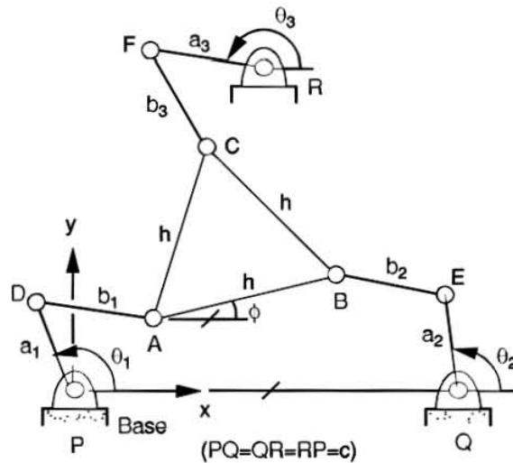
Fig. 22 Robot paralelo plano de 3 grados de libertad con estructura 3RRR
