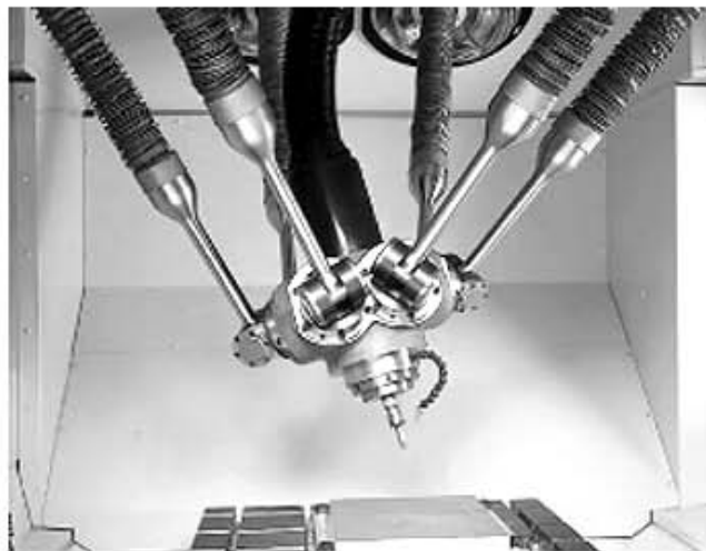
Fig. 7 Hexápodo
