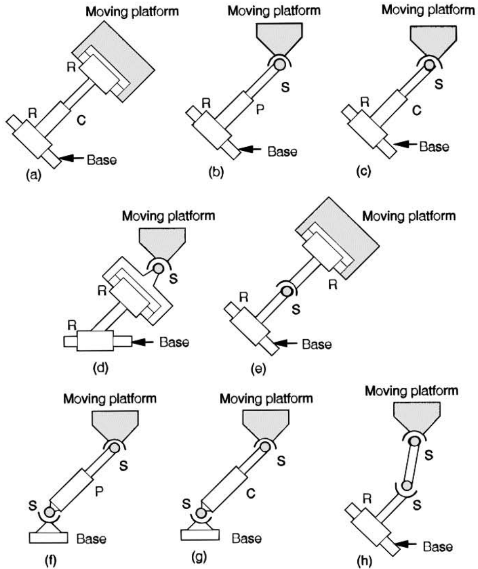
Fig.25 Ocho posibles configuraciones de miembros.
