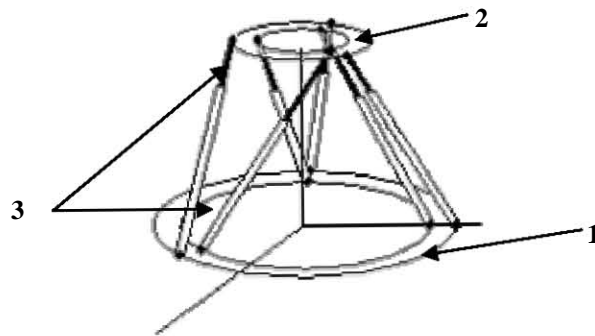
Fig. 28 El mecanismo con piernas cruzadas (CL). 1.- Base, 2.- Plataforma móvil, 3.- Piernas cruzadas
