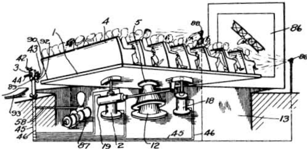
Fig.1 Posiblemente el primer mecanismo paralelo espacial, patentado en 1931 (US patent No.1,789,680)
