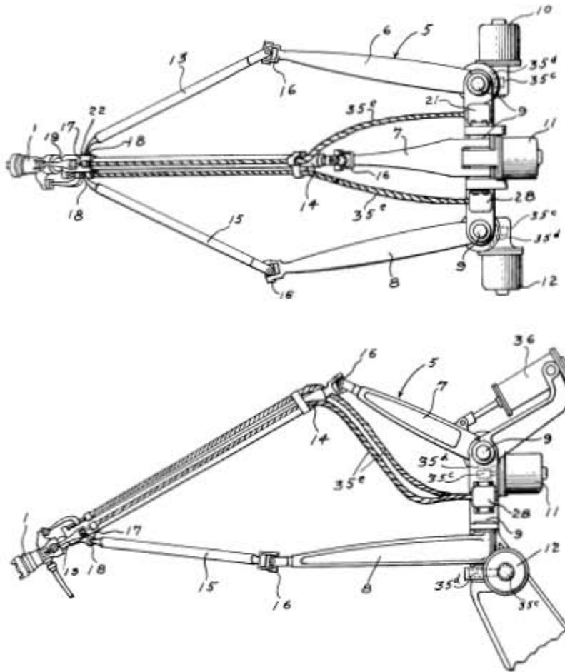
Fig.2 Primer robot industrial paralelo, patentado en 1942 (US patent No. 2, 286,571)
