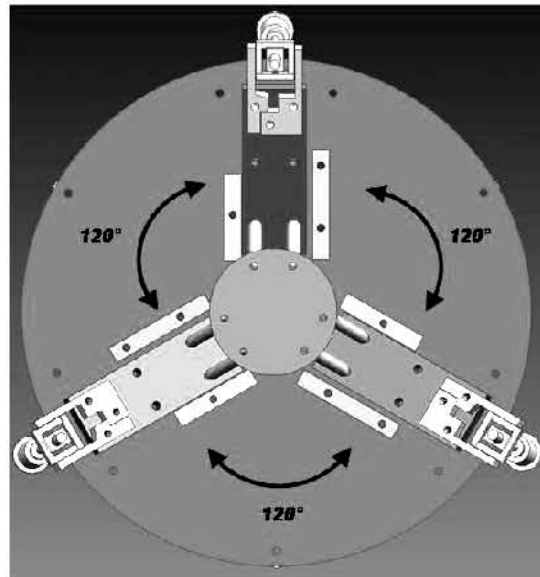
Fig. 37 Vista superior
