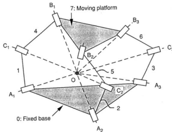
Fig. 24 Manipulador esférico con estructura 3RRR
