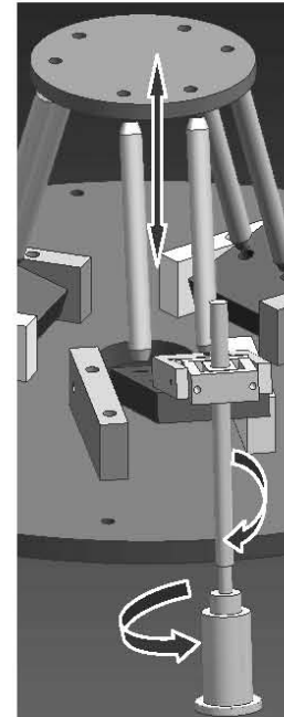
Fig. 38c Cadena cinemática
