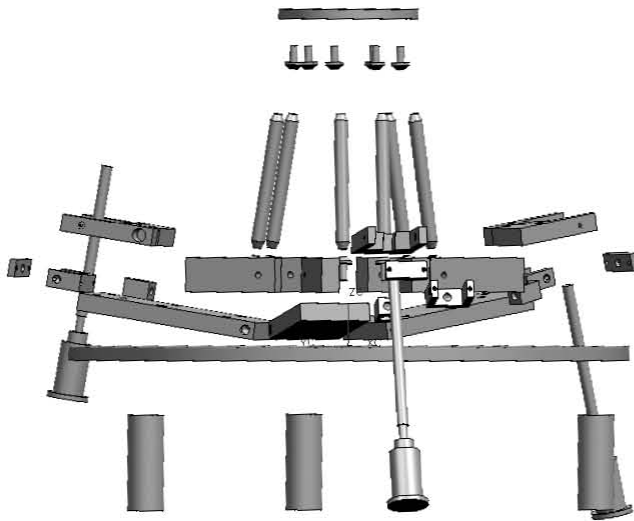
Fig.40a Micromanipulador paralelo Vista frontal
