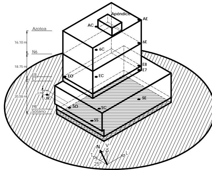
Fig 1.14 – Esquema de ubicación de los acelerógrafos en el edificio
