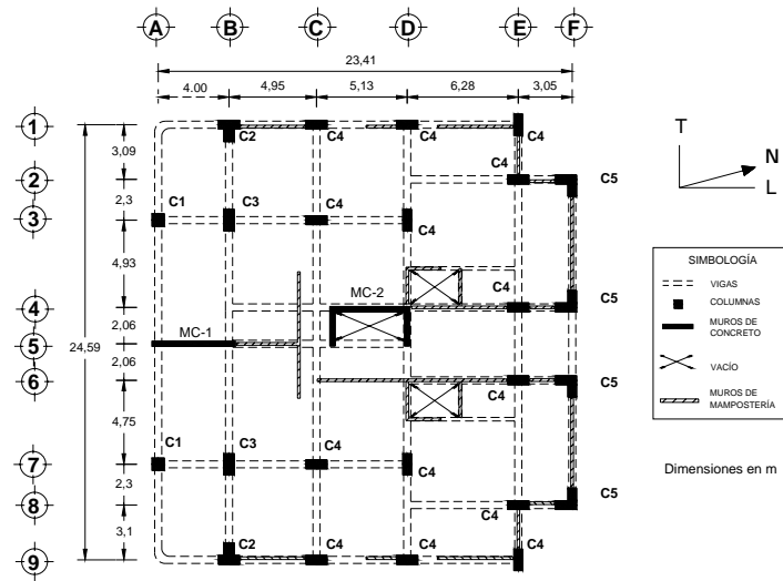
Fig 1.18 - Planta tipo
