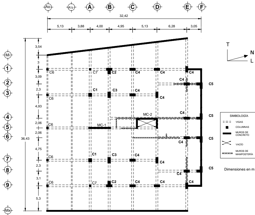
Fig 1.19 - Planta del sótano
