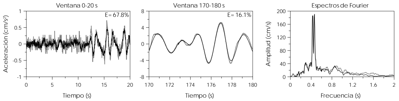
Fig D.22 – Ajuste del modelo 3D-TRAS en el componente L para el evento 99-3
