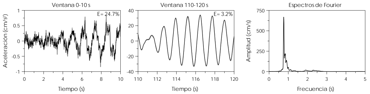
Fig D.14 – Ajuste del modelo 3D-SIST-Ch del edificio SIS en el componente T para el evento 03-1
