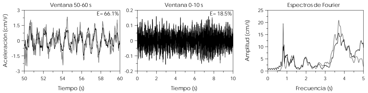
Fig D.12 – Ajuste del modelo 3D-SIST-Ch del edificio SIS en el componente R para el evento 02-2
