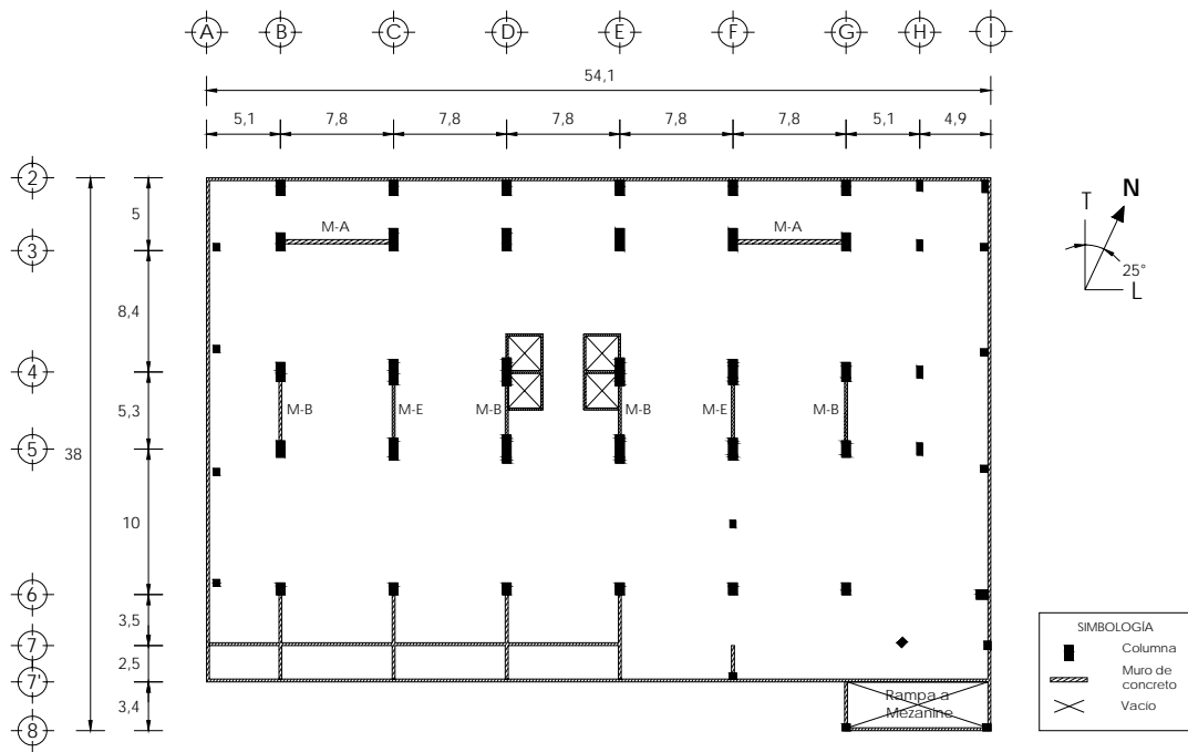
Fig 1.10 – Planta del sótano
