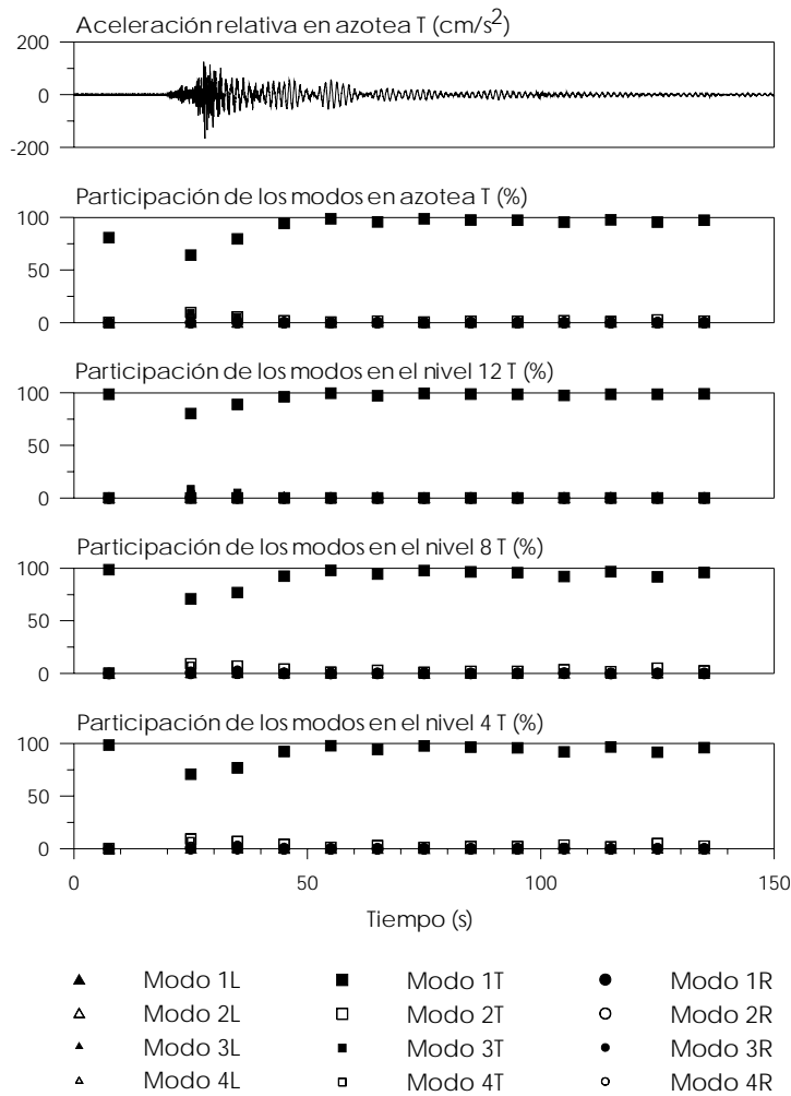
Fig 3.18 – Factores de participación de los modos identificados en las respuestas en T del modelo 3D-SIST-G T
