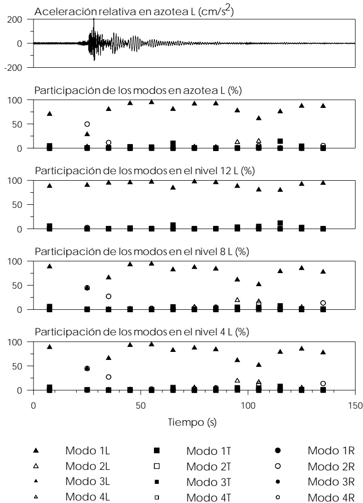
Fig 3.17 – Factores de participación de los modos identificados en las respuestas en L del modelo 3D-SIST- G_{LR}
