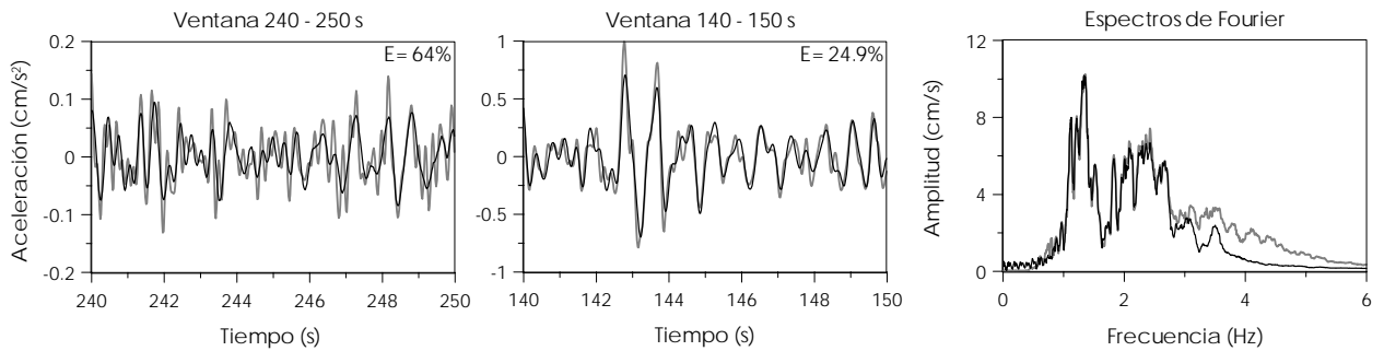
Fig D.25 – Ajuste del modelo 2D-CAB-V en el componente T para el evento 99-3
