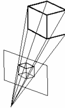
ILUSTRACIÓN IV.7 Proyección polar
