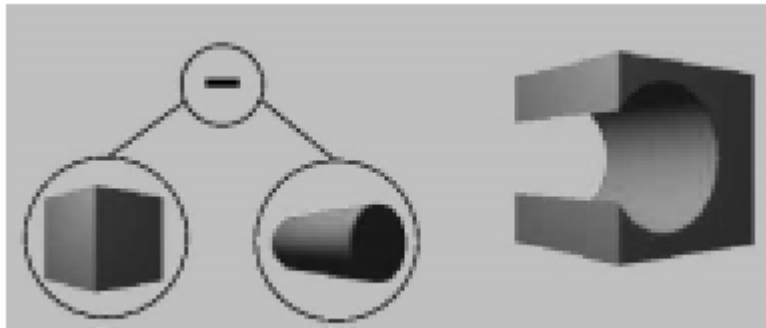
ILUSTRACIÓN IV.4 Operación booleana
