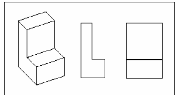
ILUSTRACIÓN IV.6 Proyecciones paralelas
