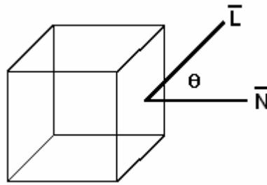
ILUSTRACIÓN IV.9 Componente Difusa
