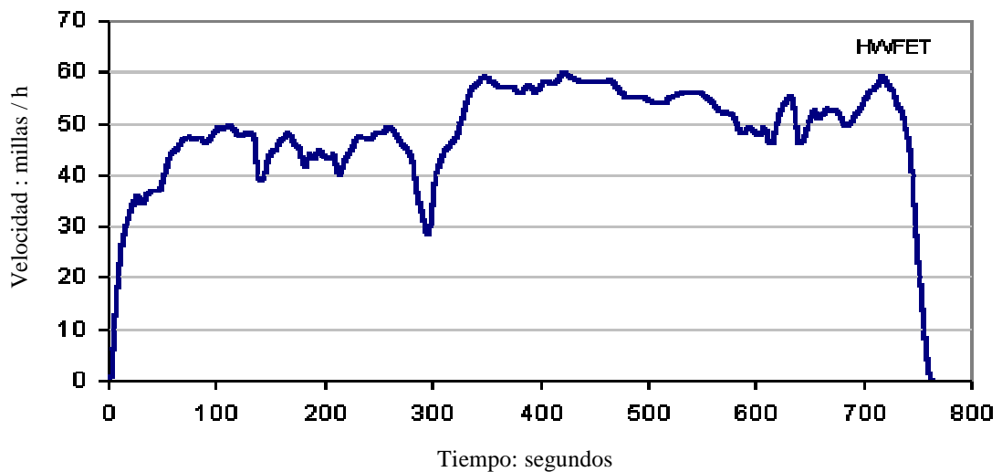
Figura 6.9 Ciclo de manejo en carretera HWFT.
