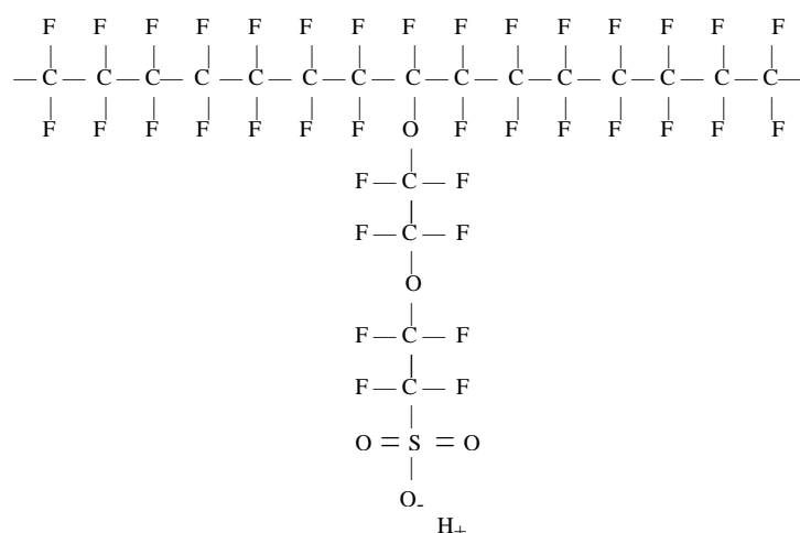
Figura 3.1 Estructura de un fluoroetileno sulfonado (también llamado copolímero ácido perfluorosulfónico).
