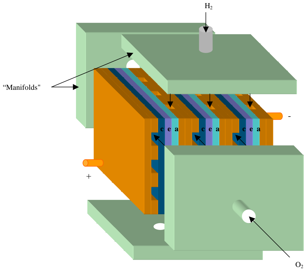
Figura 2.4 Armado básico de una pila de celdas de combustible o “ manifolding externo ”.
