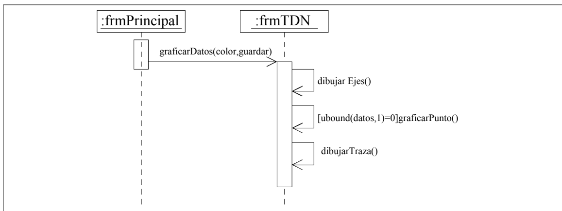
Figura 4.11: Diagrama de secuencia del caso de uso 6.
