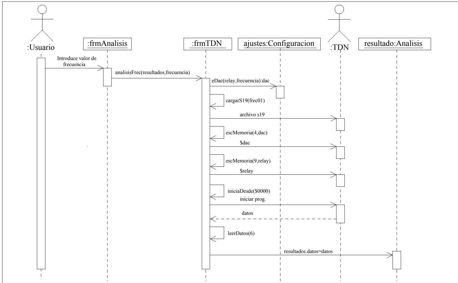
Figura 4.7: Diagrama de secuencia del caso de uso 2.
