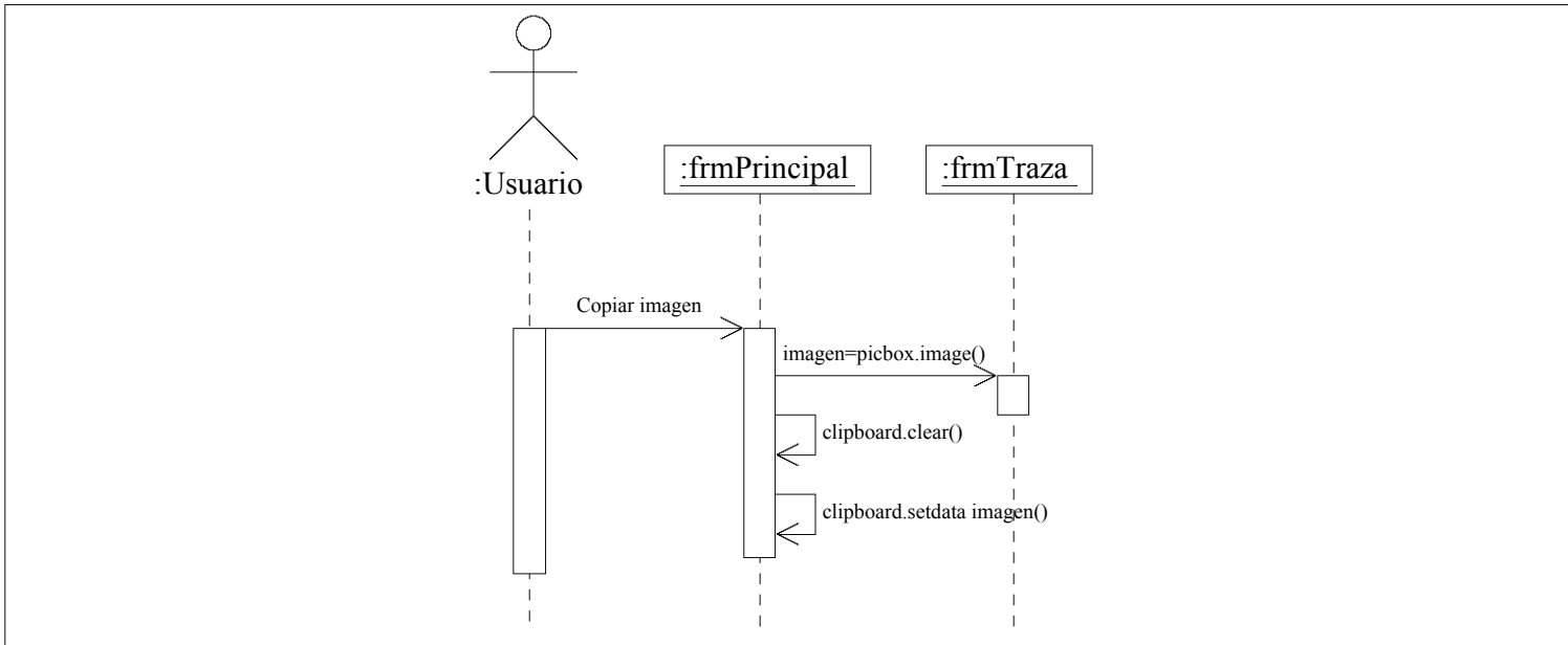
Figura 4.16: Diagrama de secuencia del caso de uso 11.
