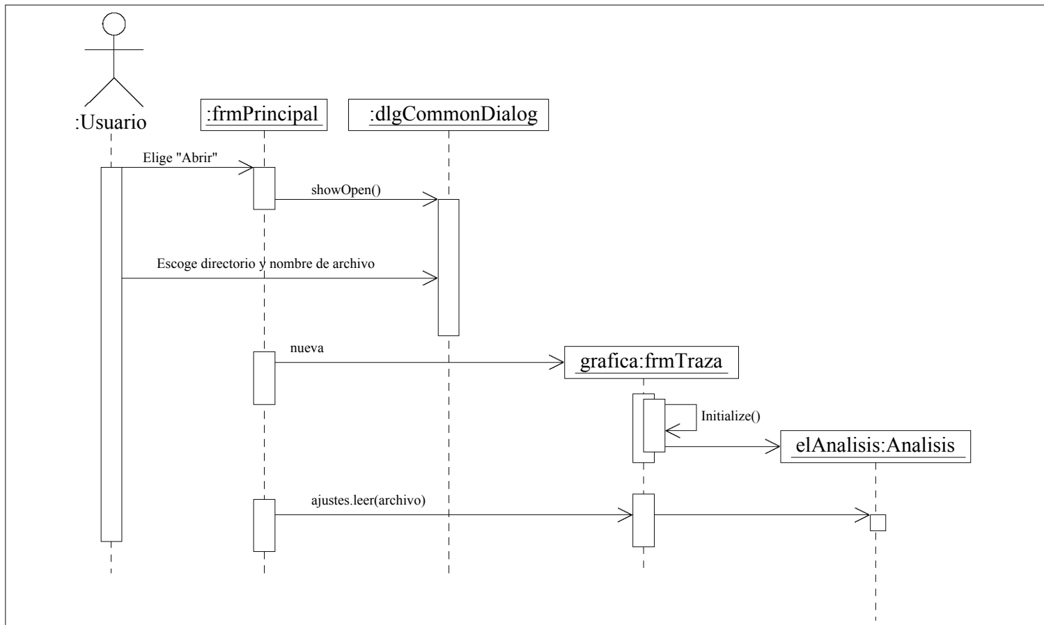
Figura 4.9: Diagrama de secuencia del caso de uso 4.
