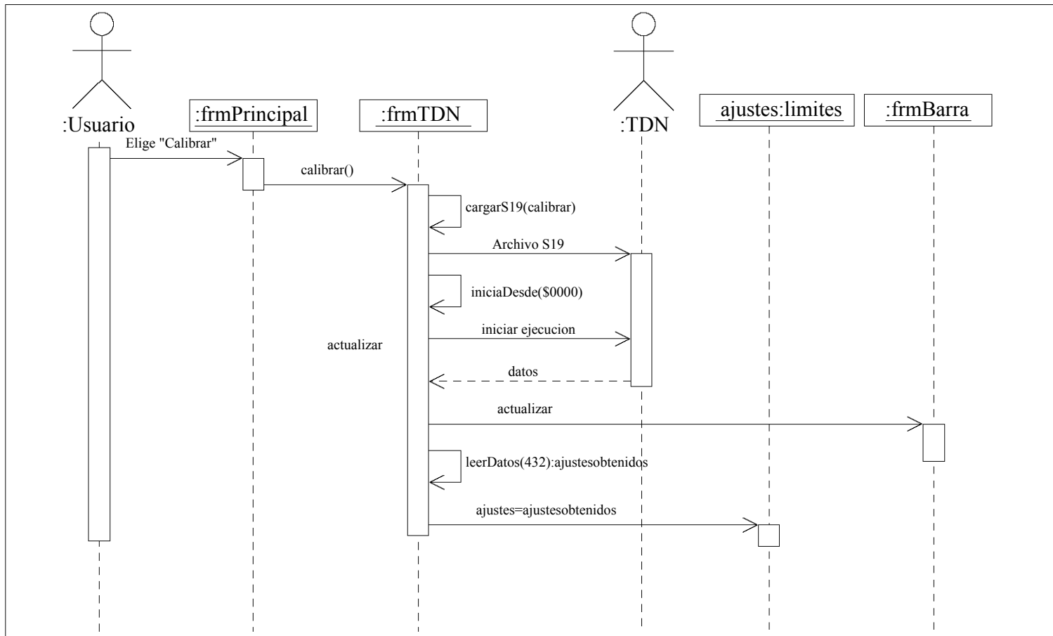
Figura 4.12: Diagrama de secuencia del caso de uso 7.
