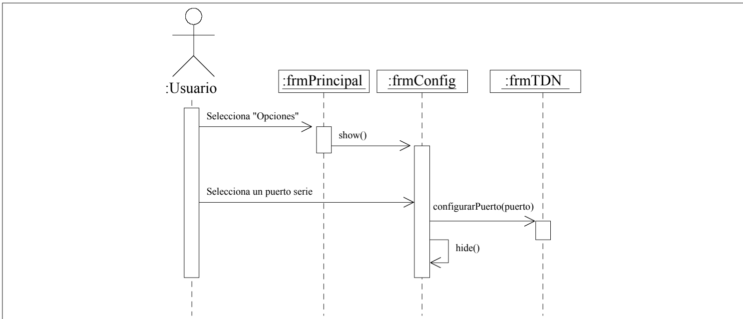
Figura 4.13: Diagrama de secuencia del caso de uso 8.
