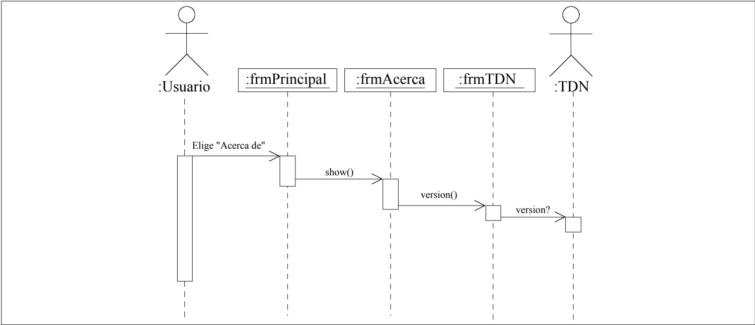
Figura 4.15: Diagrama de secuencia del caso de uso 10.
