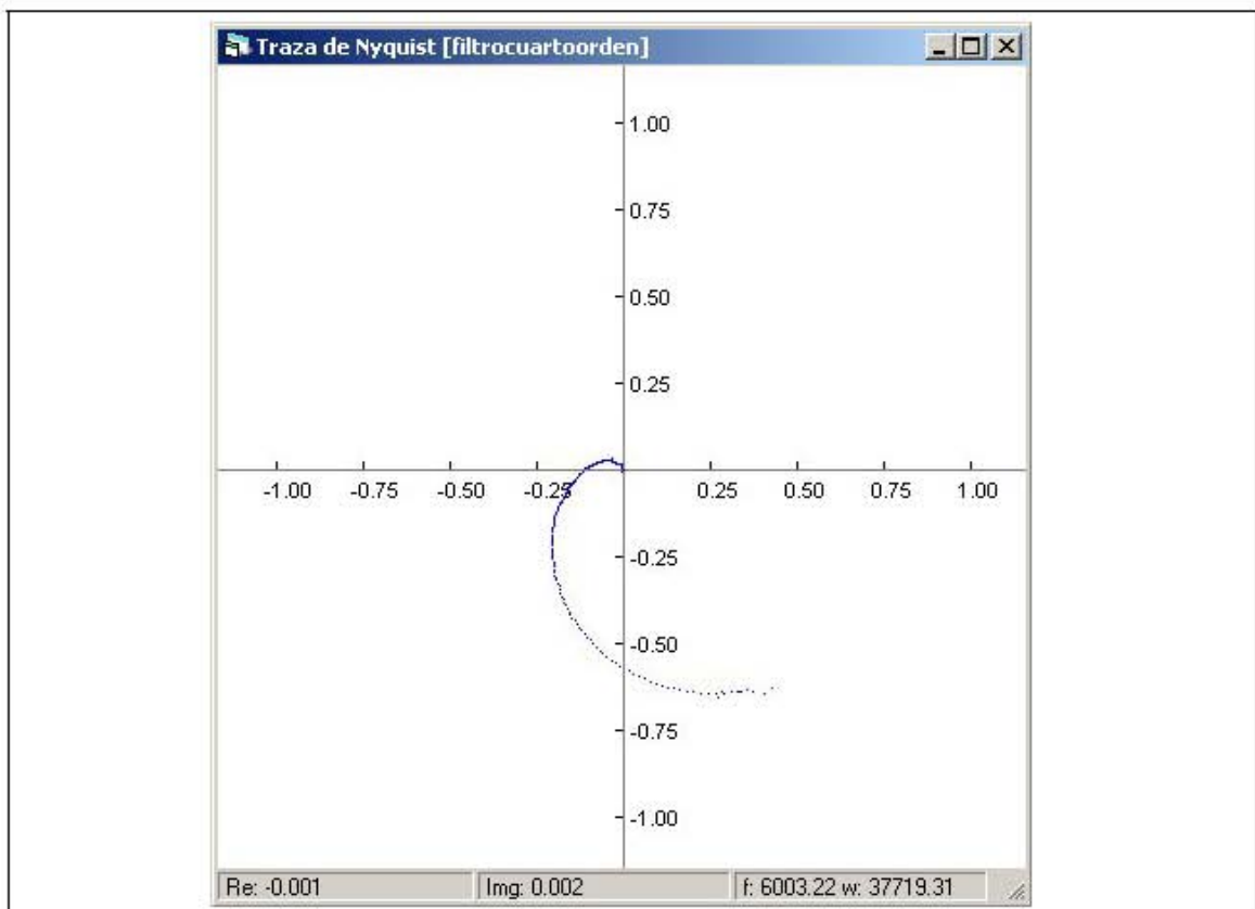
Figura 5.10: Análisis de un filtro paso-bajas de cuarto orden mediante el TDN
