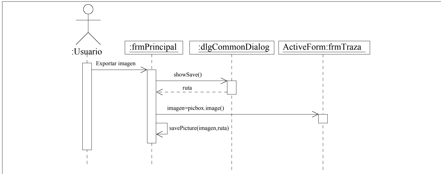
Figura 4.17: Diagrama de secuencia del caso de uso 12.
