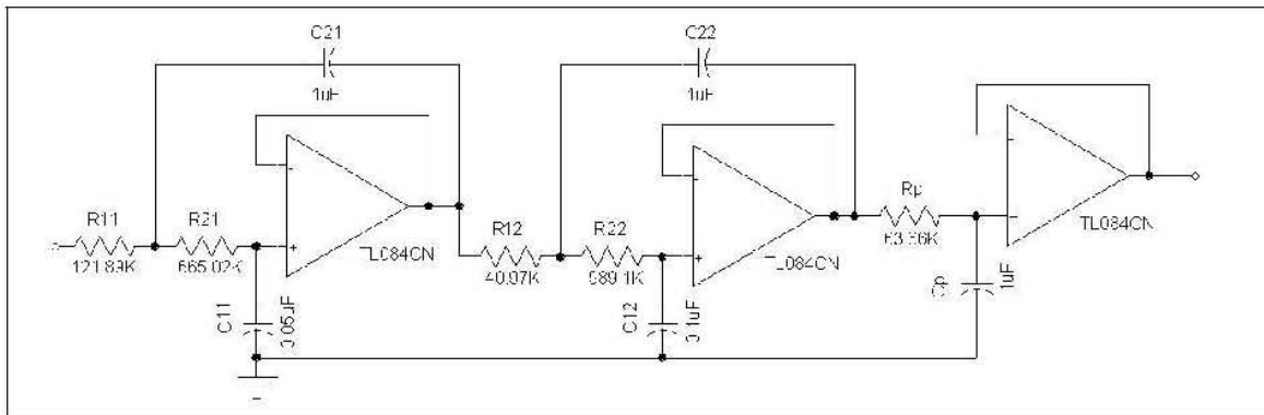
Figura 2.8: Filtro paso-bajas
