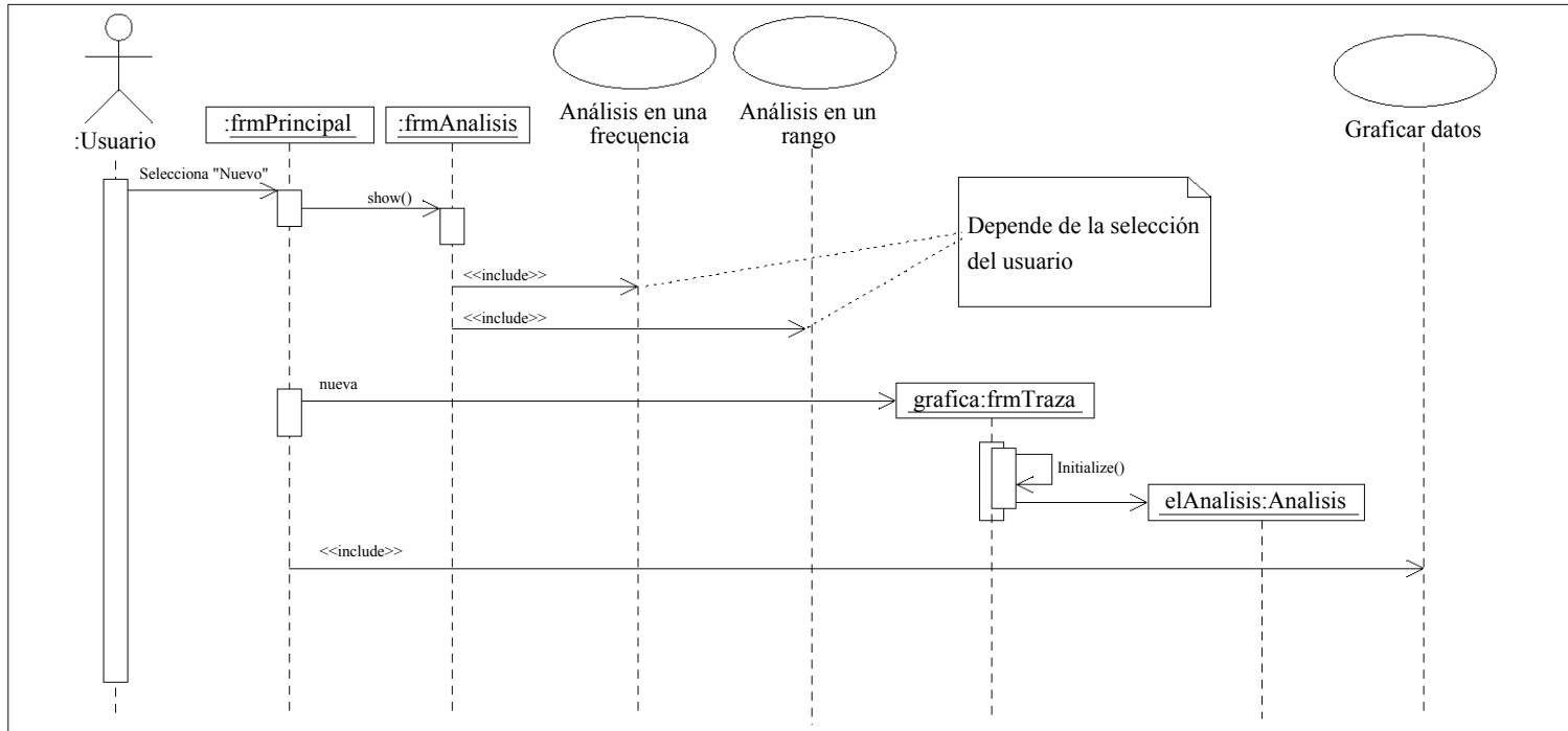
Figura 4.6: Diagrama de secuencia del caso de uso 1.
