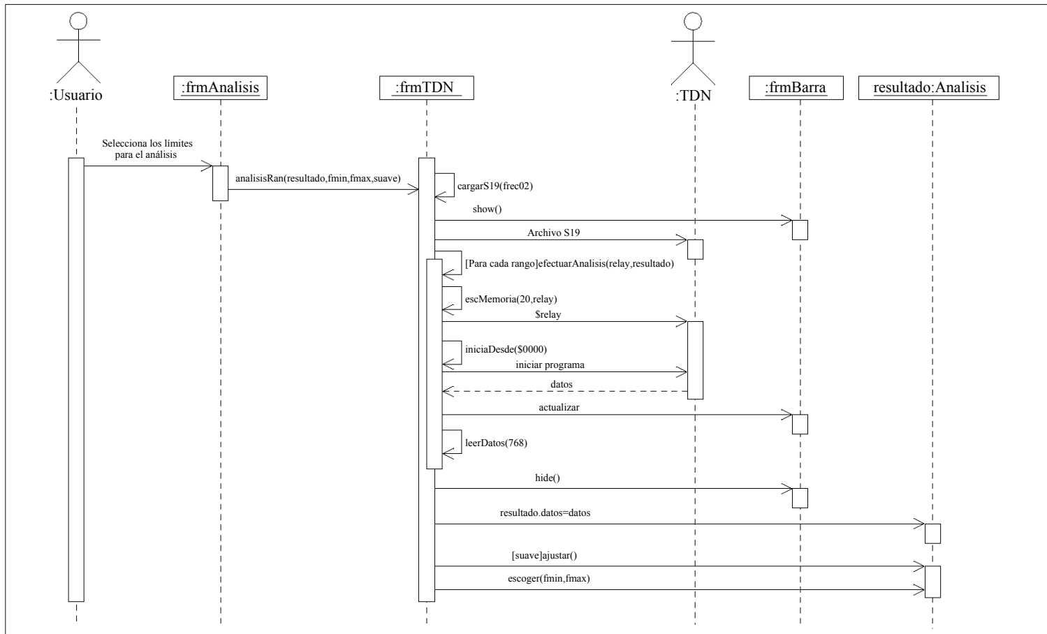
Figura 4.8: Diagrama de secuencia del caso de uso 3.
