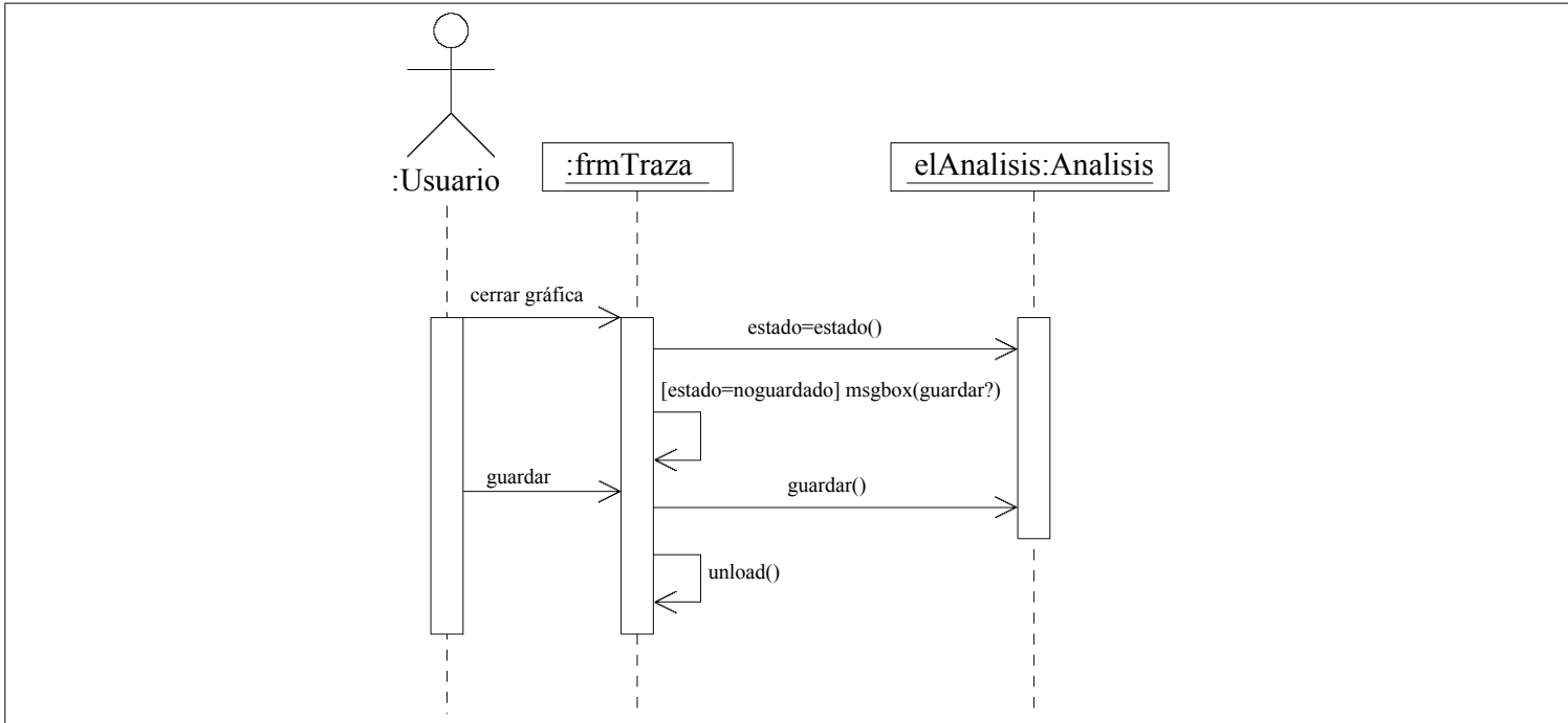
Figura 4.14: Diagrama de secuencia del caso de uso 9.
