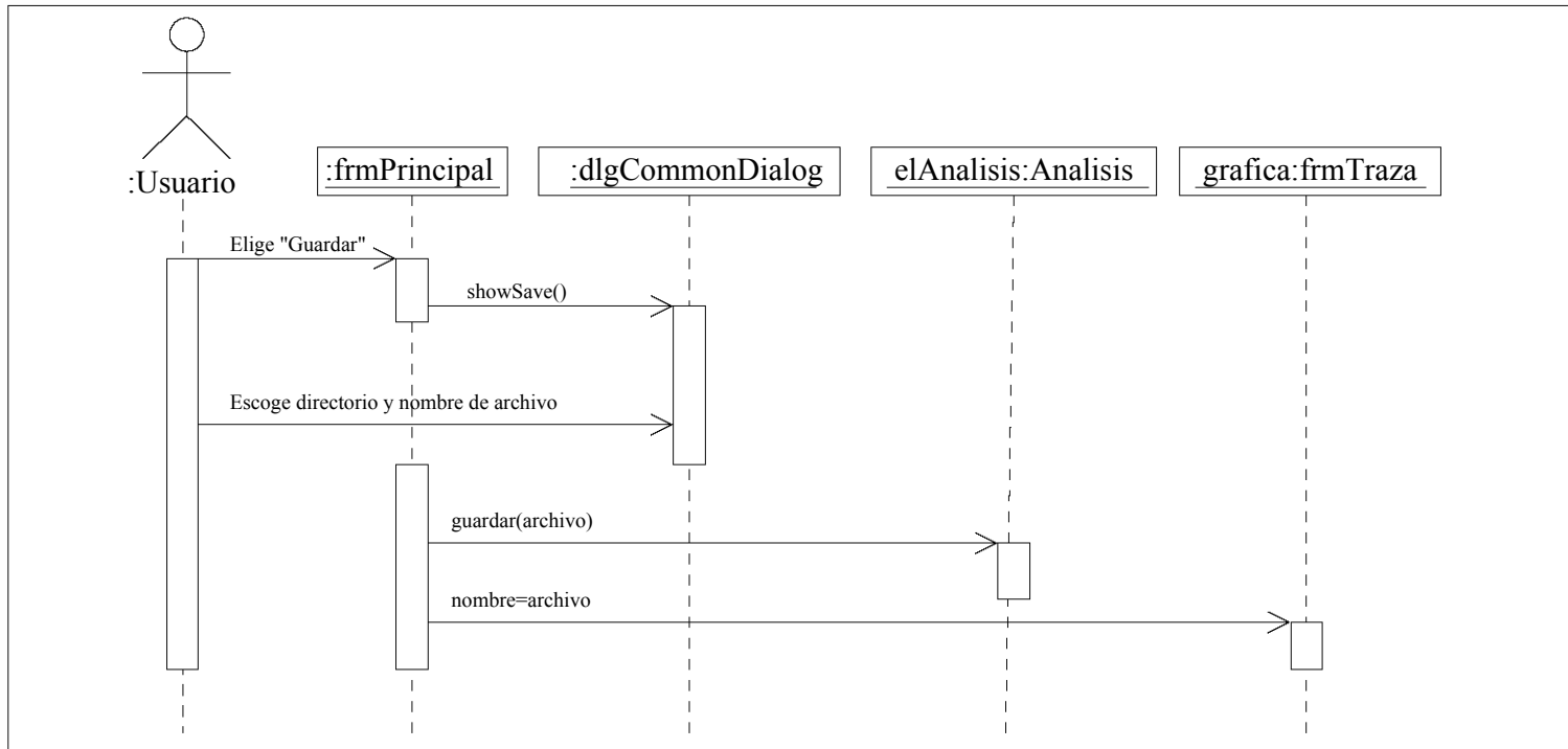
Figura 4.10: Diagrama de secuencia del caso de uso 5.
