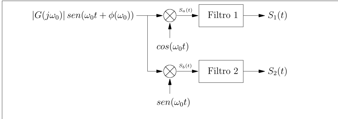
Figura 1.2: Multiplicación por las señales \cos(\omega t) y \sen(\omega t)
