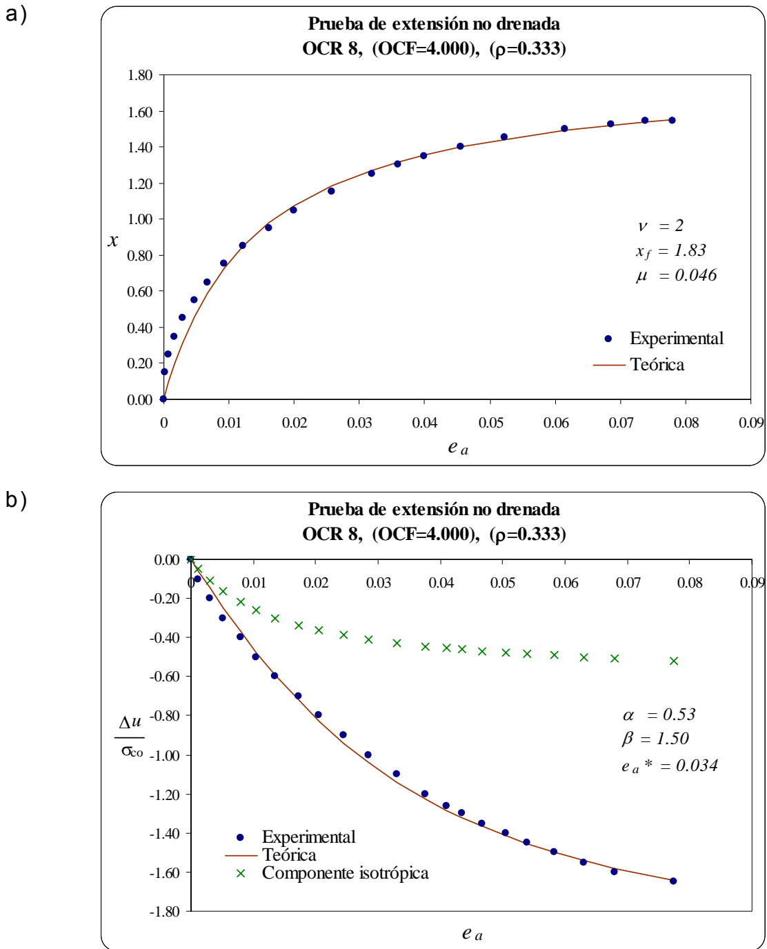
Figuras 3.11 Prueba triaxial de extensión no drenada, arcilla de Weald, OCR=8. a) Esfuerzo desviador – Deformación desviadora, b) Presión de Poro – Deformación desviadora.
