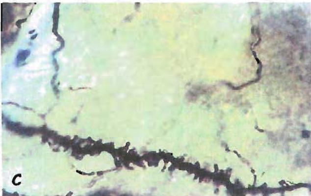
Fig. 6. Fotomicrografías de neuronas espinosas medianas del estriado del grupo control ♂. (A) 400x, (c) 1000x y del grupo control ♀ (B) 400x (D) 1000x.
