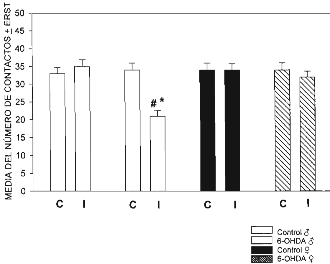
GRÁFICA 4. En esta gráfica se muestra la media del número de contactos con espina dendrítica de los caudados ipsi ( I ) y contralateral ( C ) a la lesión de los cuatro grupos analizados.
