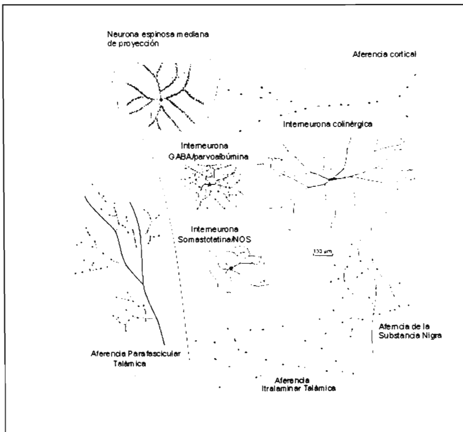
Fig. 3. Fibras aferentes y neuronas de proyección del estriado. Tomado de Wilson (1998).
