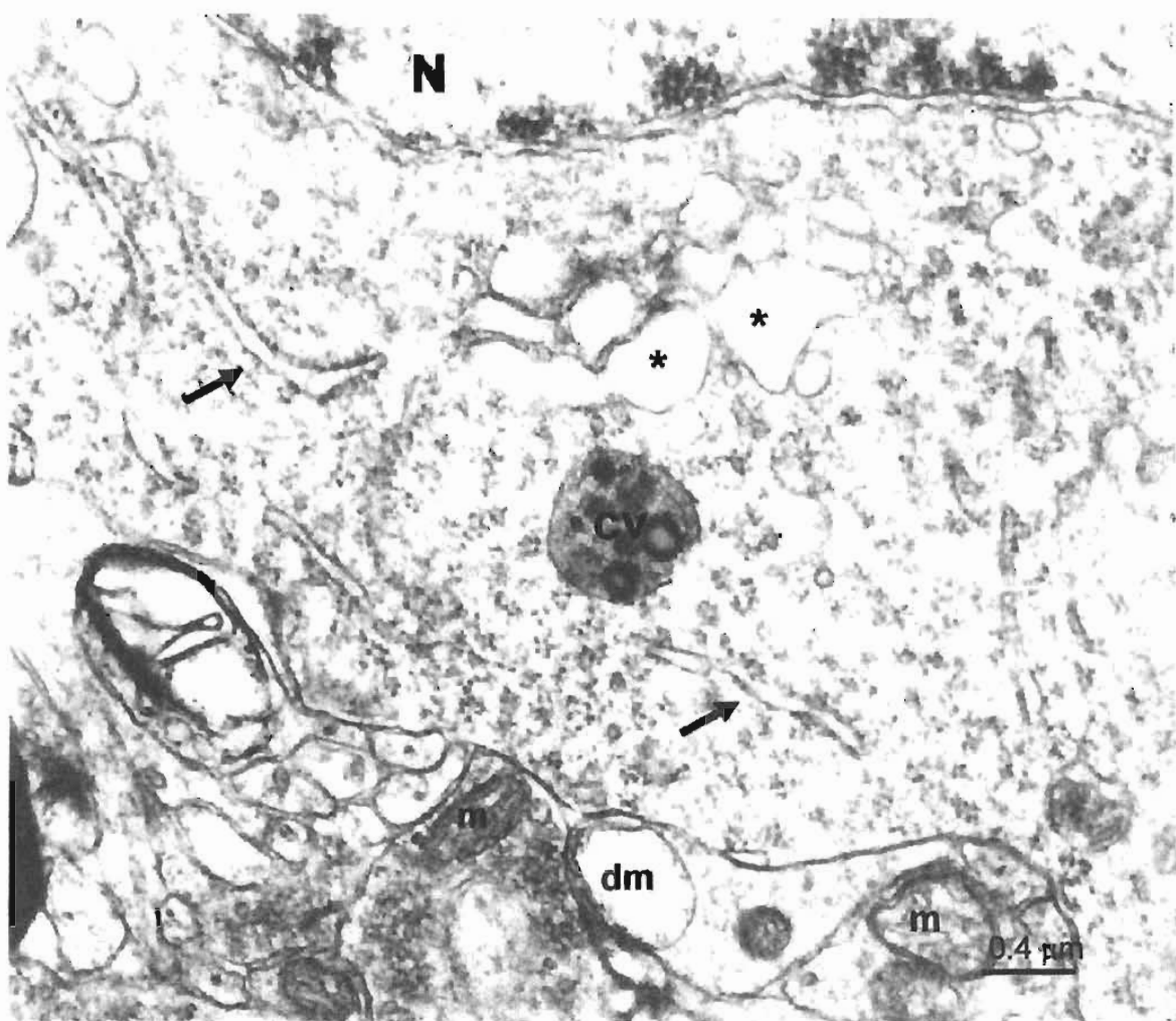
Fig. 10. Fotomicrografía de una parte de una neurona del estriado de un animal del grupo lesionado ♀ con signos evidentes de neurodegeneración, caracterizado por presencia de vacuolas (*) rodeando al núcleo (N), mitocondria (m), retículo endoplásmico ( → ), degeneración de mitocondrias (dm), cuerpo multivesicular (CV). Magnificación 20000 X.
