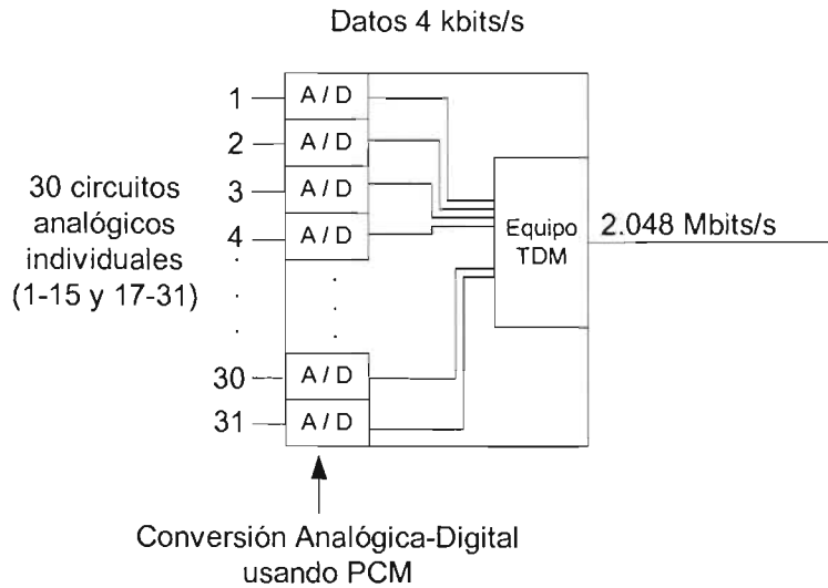
Figura 1.15. Multiplexor primario.
