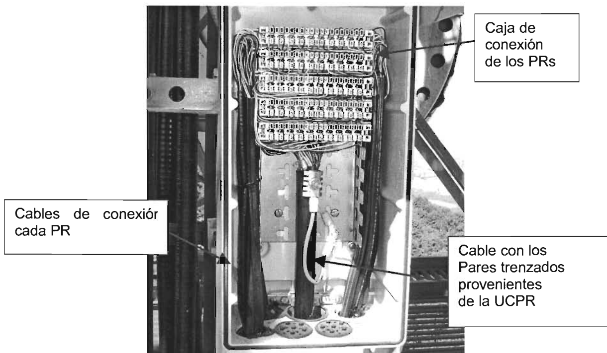
Figura 4.22. Caja de conexión en la torre.
