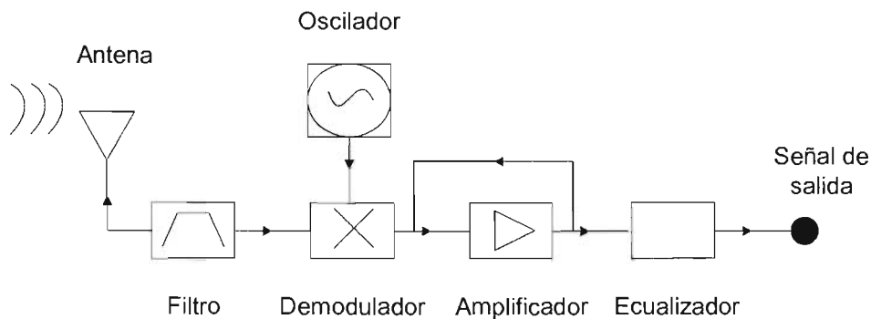
Figura 1.25. Receptor simple de radio.
