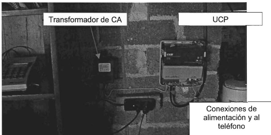
Figura 4.36. Instalación de la UPC.
