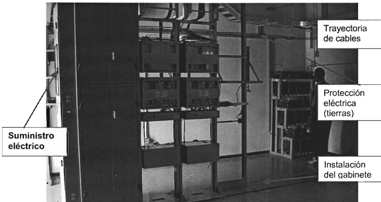
Figura 4.5. Sala donde se instalará el SMG.
