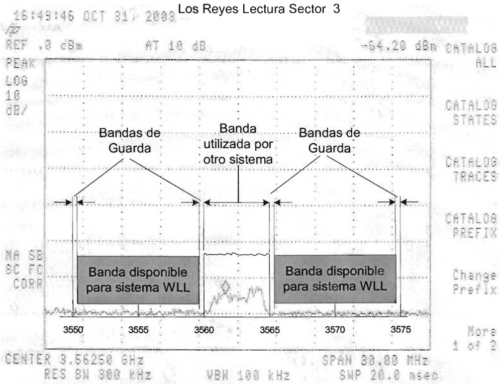
Figura 4.11. Tercera lectura del ancho de banda del sitio Los Reyes.
