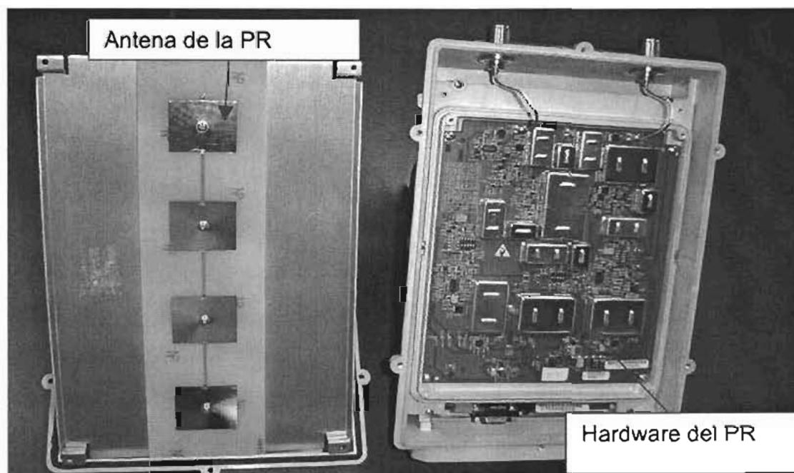
Figura 3.3. Antena PR.
