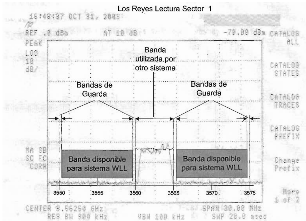
Figura 4.9. Primera lectura del ancho de banda del sitio Los Reyes.
