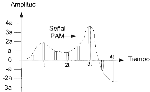
Figura 1.9. Modulación por amplitud de pulsos.
