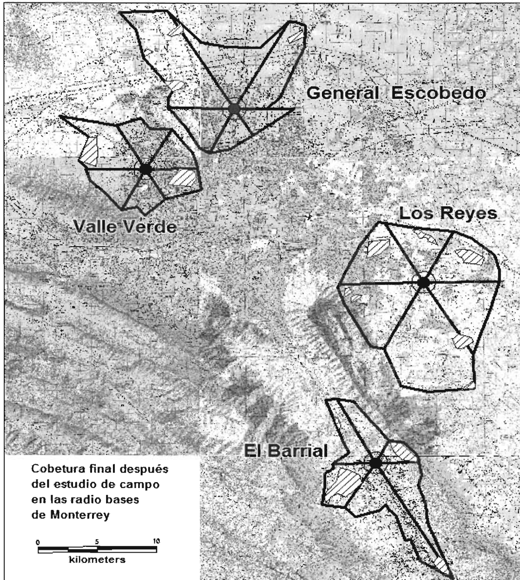
Figura 4.8. Cobertura de las cuatro radio bases.
