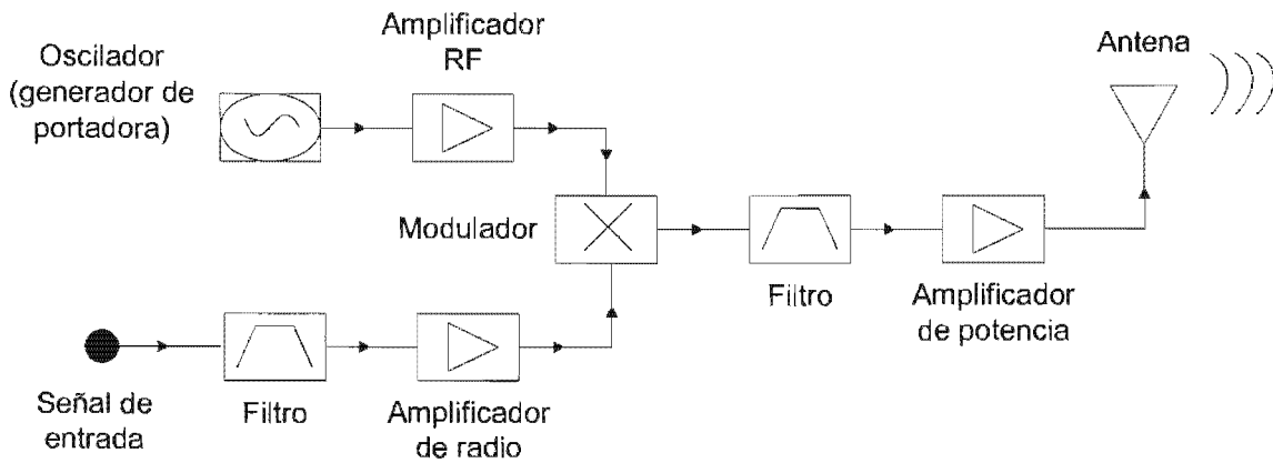
Figura 1.21. Transmisión simple de radio.
