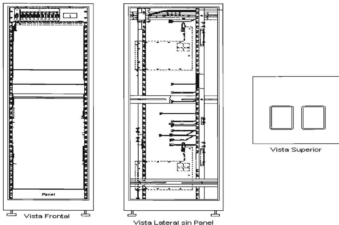
Figura 4.15. Bastidor del SMG.
