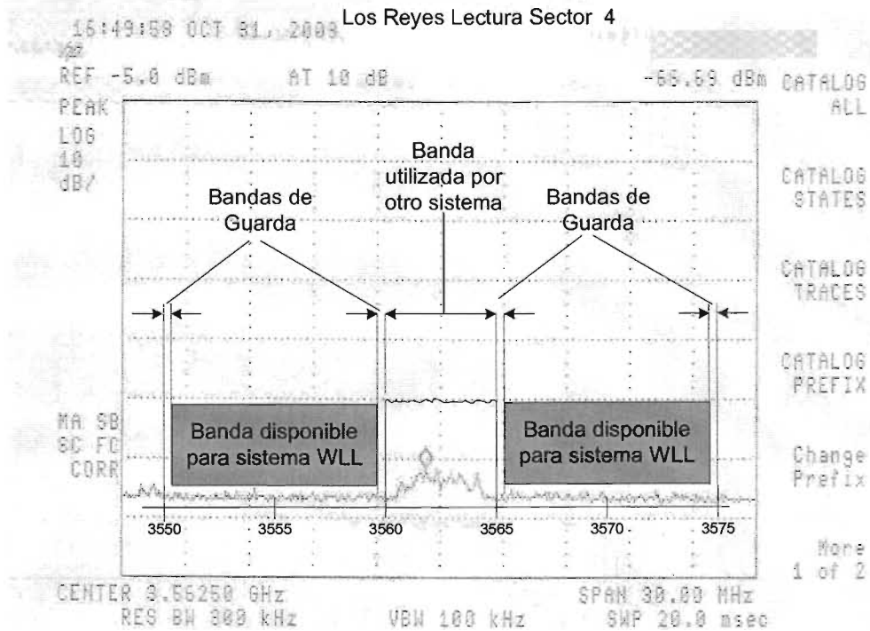
Figura 4.12. Cuarta lectura del ancho de banda del sitio Los Reyes.
