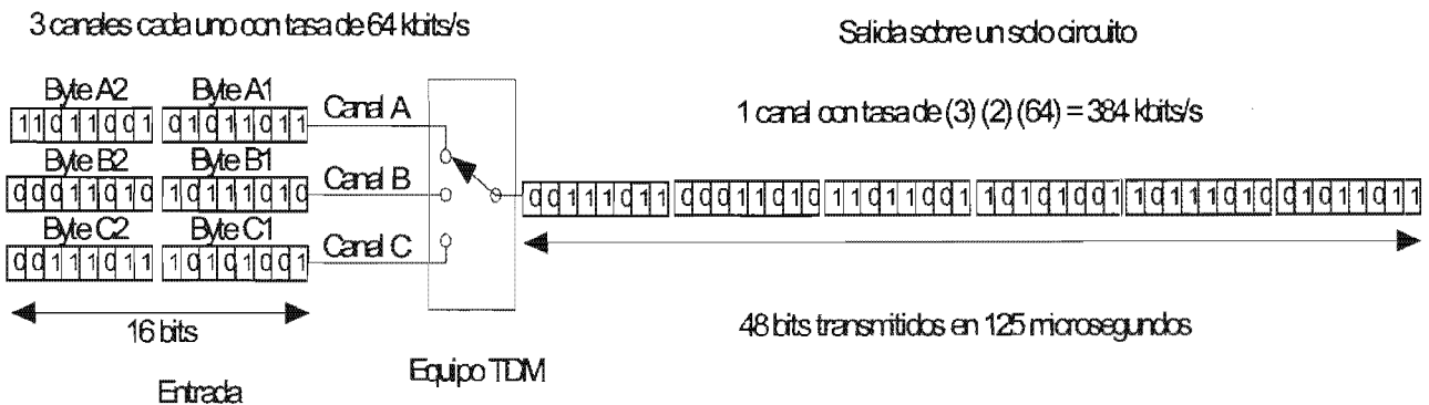
Figura 1.14. Principio de multiplexaje por división de tiempo.
