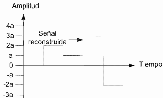
Figura 1.8. Reconstrucción de la forma de onda.
